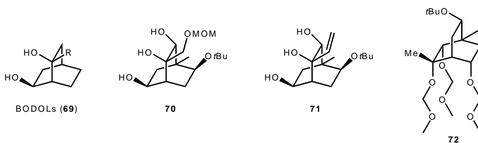
Figure 7 : Les BODOLs de Frejd et trois exemples de ligands tridentates synthésisés au laboratoire.
