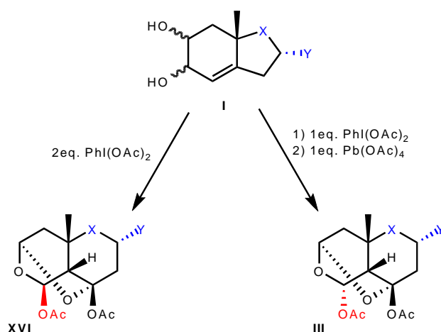
Schéma 115 : Différence de réactivité entre le \text{Pb}(\text{OAc})_4 et le \text{PhI}(\text{OAc})_2 .
