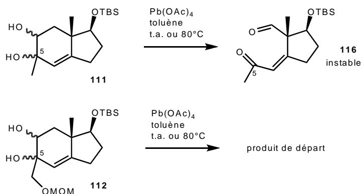
Schéma 31 : Une fonctionnalisation de la position 5 n'est pas favorable à la réaction domino.
