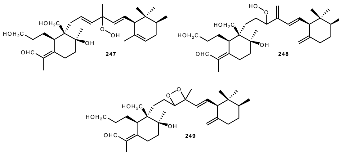
Figure 27 : Intermédiaires possibles de la formation des irones.
