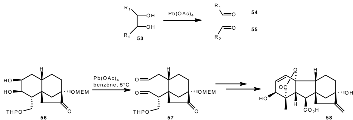
Schéma 13 : Réaction de fission du glycol et son utilisation dans la synthèse de l'acide Gibbérellique par Corey.
