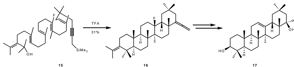
Schéma 4 : Synthèse biomimétique du Sophoradiol
