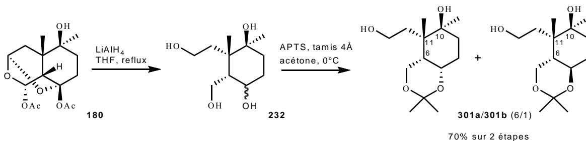
Schéma 70 : Réduction de la "cascade" 180 et protection sous forme d'acétonide.
