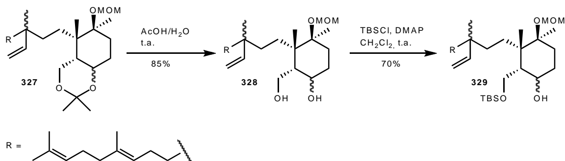
Schéma 86 : Synthèse de l'alcool 329 .
