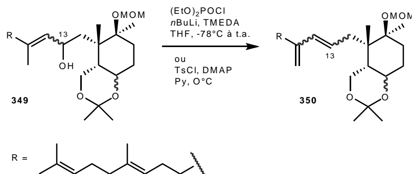
Schéma 99 : L'alcool allylique en C13 est très instable.
