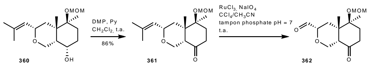
Schéma 108 : Nouvel essai de formation de la lactone.
