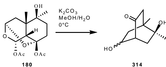
Schéma 78 : Formation très rapide du bicyclic 314.
