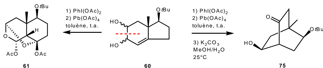
Schéma 20 : Deux possibilités de réaction domino.
