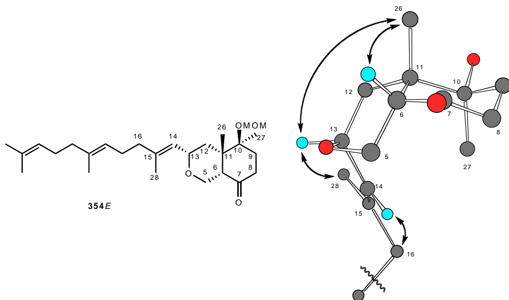
Figure 45 : Confirmation des configurations de la cétone 354E par expérience ^1\text{H} -RMN-NOESY (représentation du conformère de plus basse énergie).
