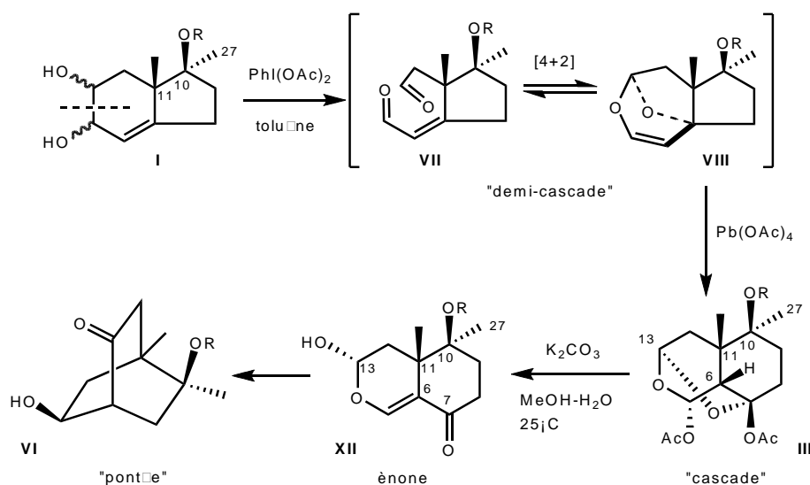
Schéma 76 : Rappel de la réaction domino du laboratoire.
