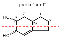
Figure 11 : Les différentes positions fonctionnalisables de la partie "nord".
