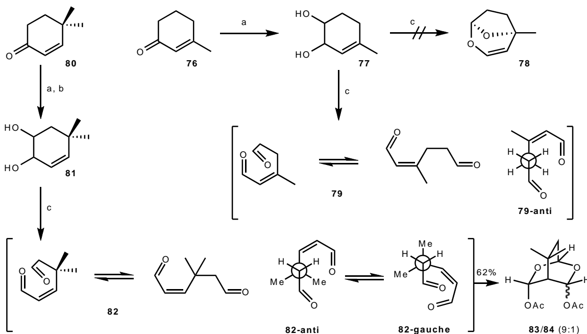
Schéma 23: Réactifs et conditions: a) \text{Pb}(\text{OAc})_4 , benzène, 90°C, 4 jours; b) \text{LiAlH}_4 , \text{Et}_2\text{O} , 0°C; c) 2,4 eq. \text{Pb}(\text{OAc})_4 , MeCN, -30°C à 25°C.
