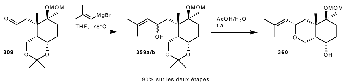
Schéma 107 : Synthèse d'un bicyclic ne comportant pas l'intégralité de la chaîne homofarnésyle.
