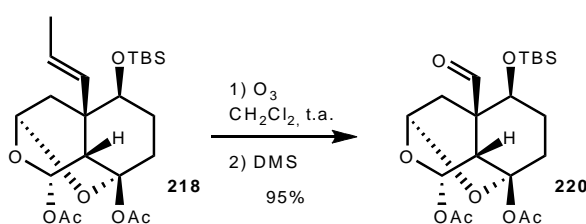
Schéma 53 : Ozonolyse du composé 218 .
