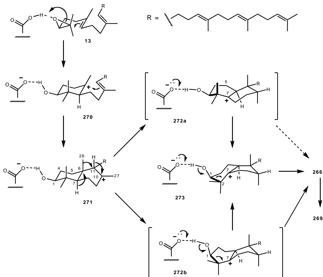
Figure 37 : Mécanisme de formation de l'alcool 269.
