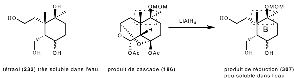
Schéma 111 : Utilisation bénéfique de la "cascade" 186 comportant l'alcool tertiaire protégé.
