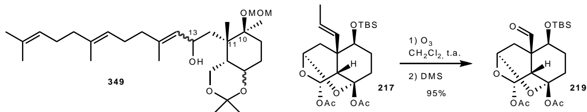
Schéma 120 : Deux méthodologies nous donnant accès aux spiroiridals.
