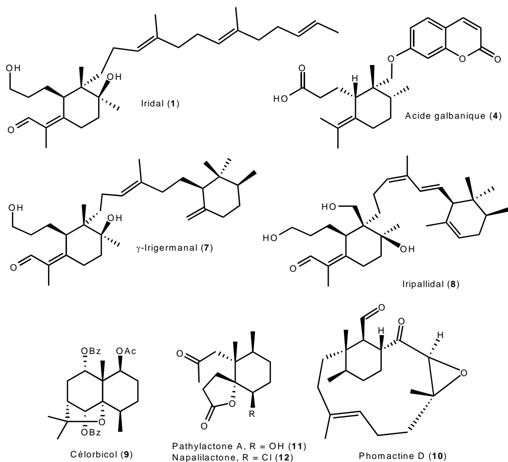
Figure 4 : Quelques terpènes.
