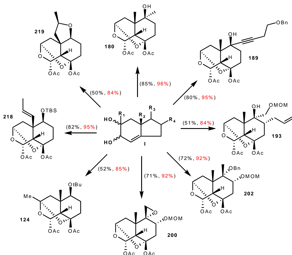
Figure 5 : Quelques exemples de produits pouvant être obtenus par la réaction domino initiée par le \text{Pb}(\text{OAc})_4 (rendement obtenu, rendement moyen par transformation dans la réaction domino ).
