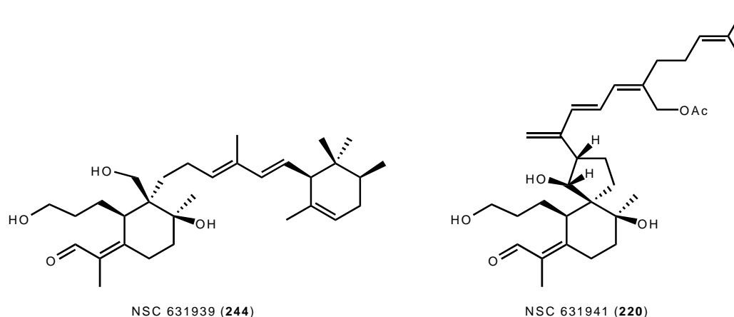
Figure 33 : Deux iridals issus du programme de criblage du NCI.
