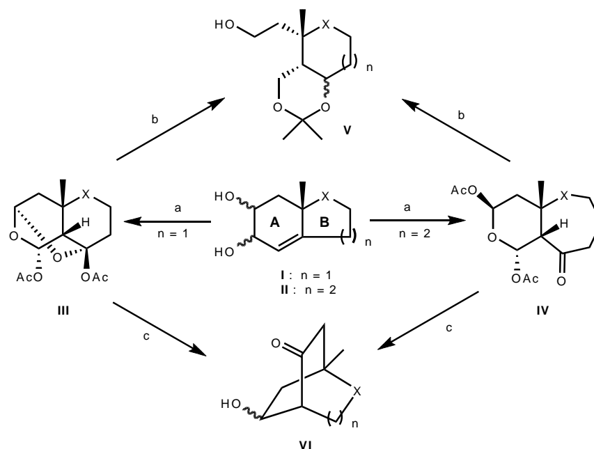
Schéma 1 : Produits obtenus par réaction domino. a) 2.5 eq. Pb(OAc) 4 , CH 3 CN, 25 °C. b) LiAlH 4 , Et 2 O, 0 °C puis p -TsOH, acétone. c) K 2 CO 3 , MeOH:H 2 O (8:1), 25 °C.
