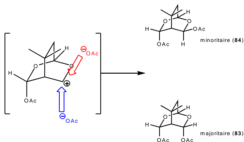
Figure 8 : Deux attaques possibles pour le groupement acétate.
