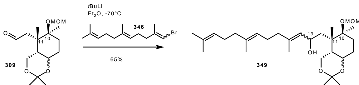
Schéma 98 : Réaction de couplage par échange halogène-lithium.
