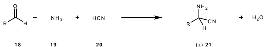
Schéma 5 : La première réaction domino: la réaction de Strecker
