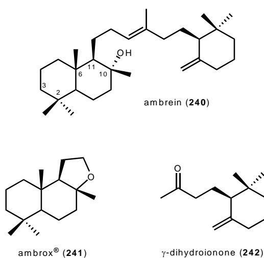
Figure 24 : L'odeur d'ambre gris provient de la dégradation de l'ambrein.
