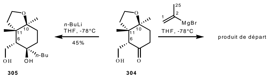
Schéma 73 : Additions sur la cétone 304.
