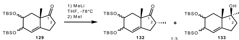
Schéma 38 : Vérification du caractère basique du MeLi par arrêt de la réaction à l'aide de MeI.
