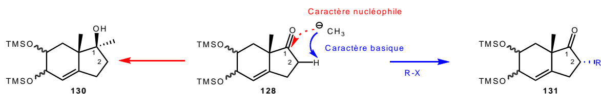
Figure 12 : Caractère nucléophile et basique (l'anion est piégé par ajout de RX) du MeLi.
