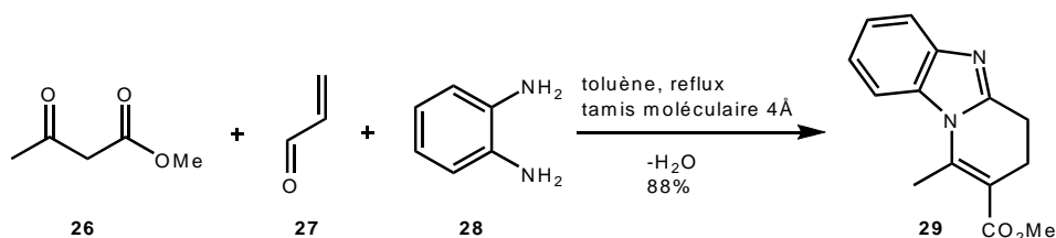
Schéma 8 : Synthèse de polyhétérocycles par réaction domino.
