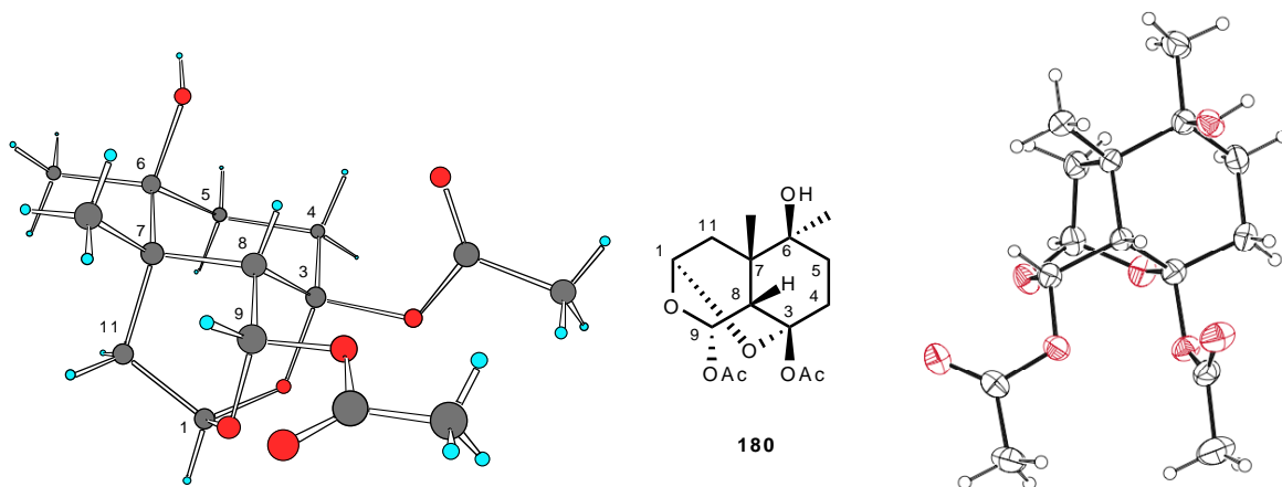
Figure 13 : Rayon X de la "cascade" 180 (vue en Chem3D et en ellipsoïde).
