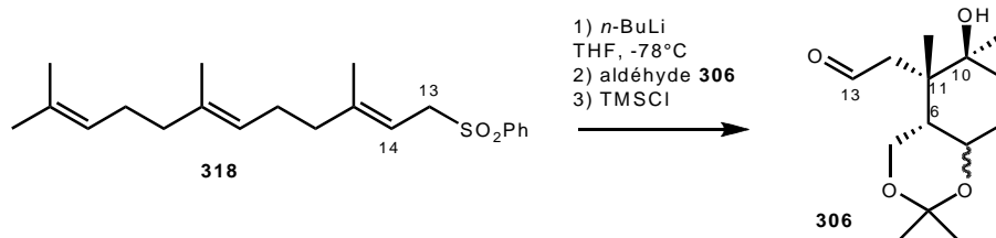
Schéma 82 : Absence d'addition de la sulfone.
