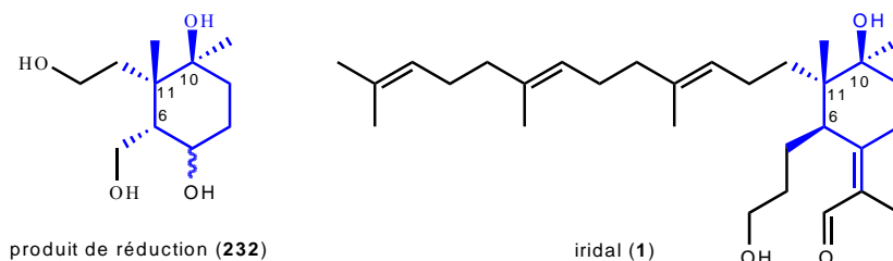
Figure 40 : Une ressemblance évidente.
