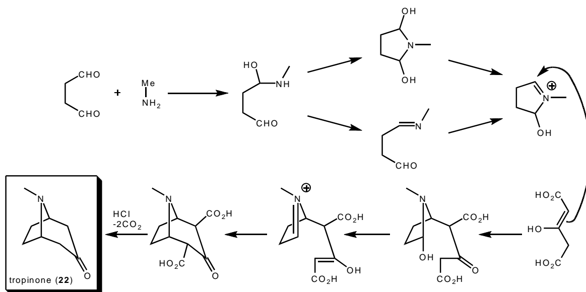
Schéma 6 : Synthèse domino de la tropinone.
