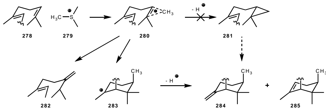
Schéma 65 : Insertion du groupement méthyle.
