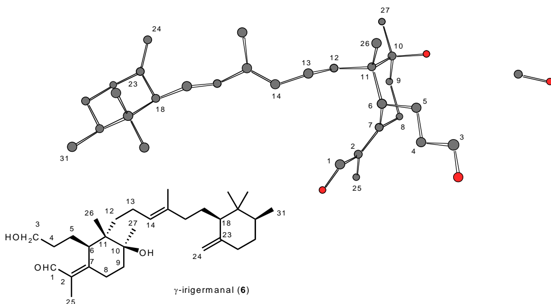
Figure 30 : Rayons X du \gamma -irigermanal 6 obtenu par Marner.
