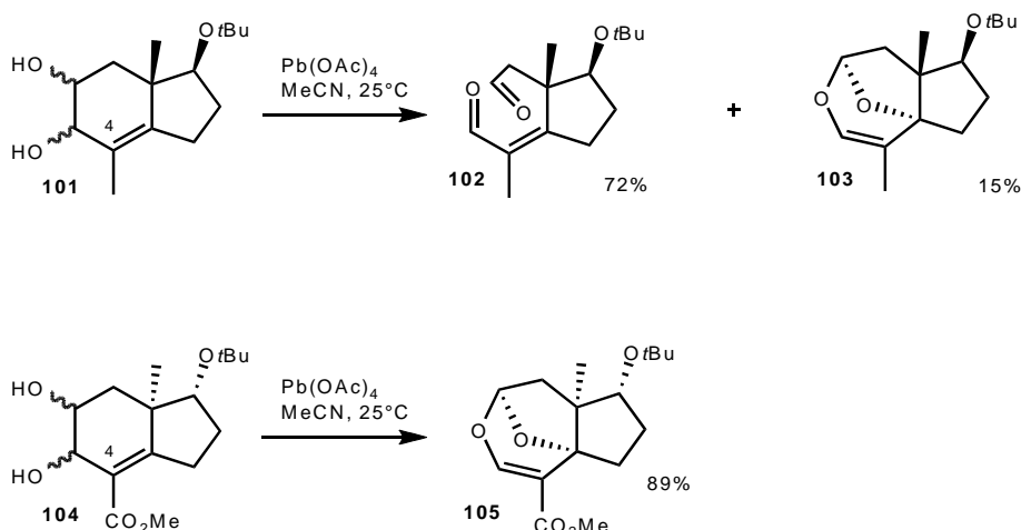
Schéma 27 : Influence du substituant en position 4 sur la réaction domino.
