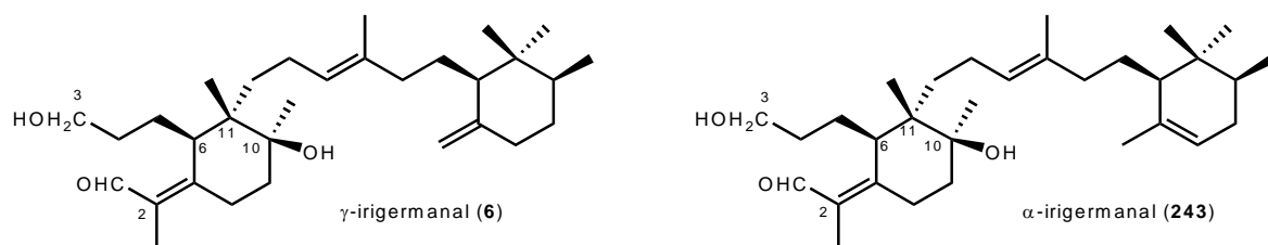
Figure 25 : Les deux premiers Iridals décrits.
