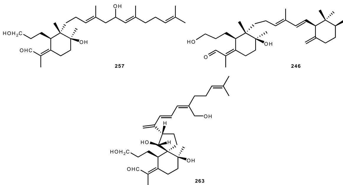
Figure 34 : Un exemple de chacune des trois sous-familles des iridals.
