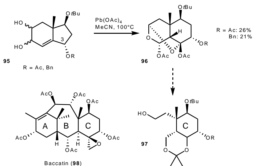
Schéma 26 : La réaction de cascade peut avoir lieu avec un substituant en position 3.
