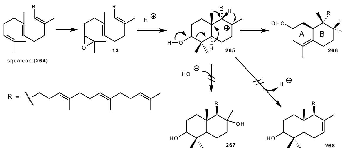
Schéma 62 : Biosynthèse proposée de l'iridal.
