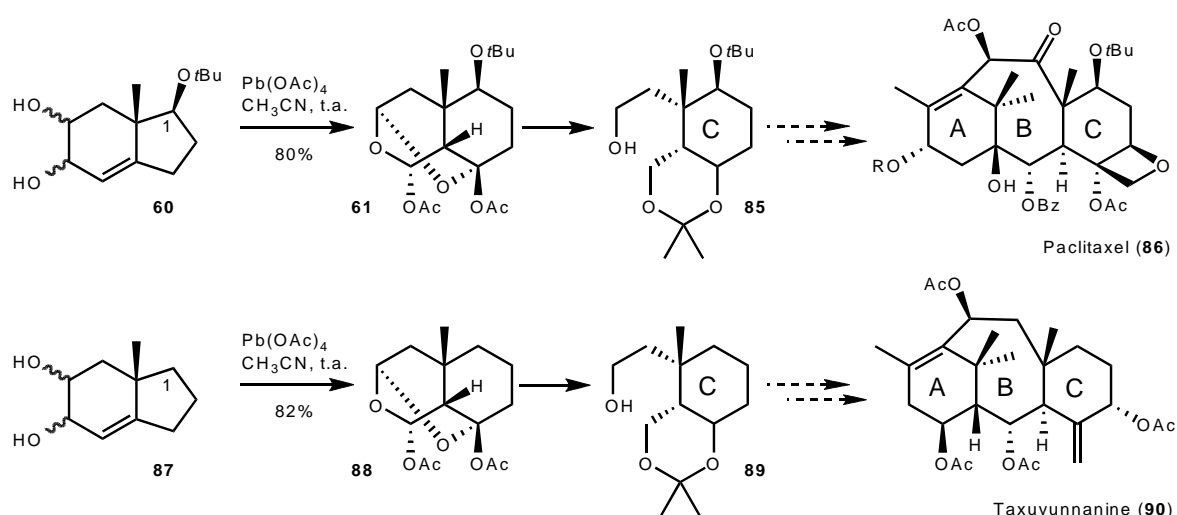
Schéma 24 : Les premières réactions de "cascade" avaient pour but la synthèse taxoïde.
