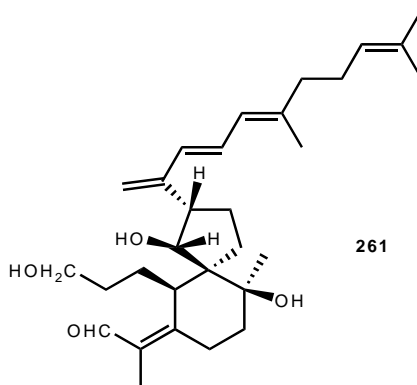
Figure 29 : Un spiroiridal.
