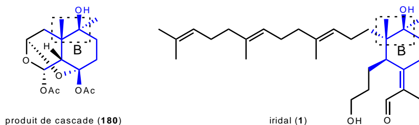
Figure 39 : Les centres quaternaires déjà définis.
