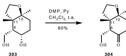
Schéma 72 : Oxydation du diol 303.
