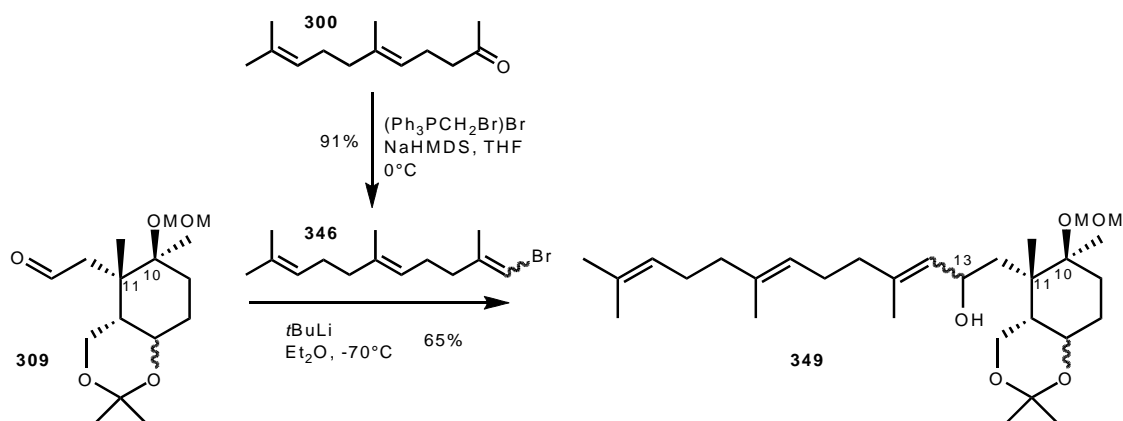
Schéma 112 : Synthèse de la chaîne homofarnésyle.
