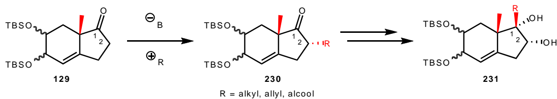
Schéma 58 : Insertion d'un troisième centre asymétrique et contrôle du deuxième centre quaternaire.
