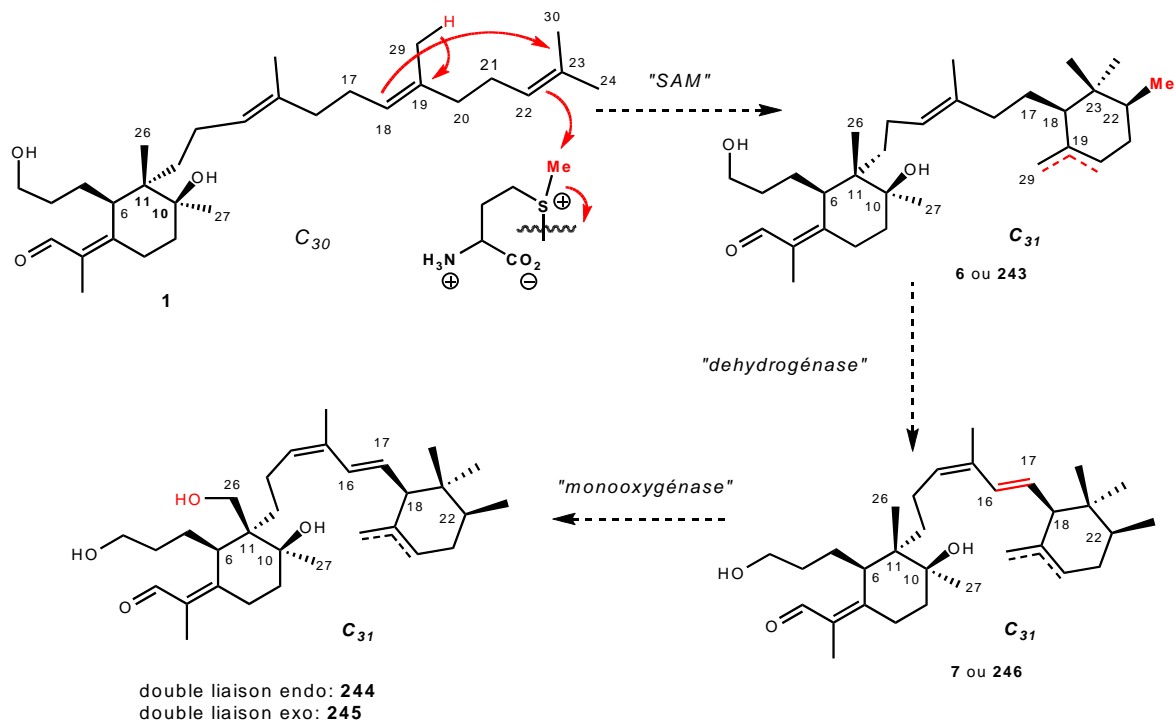
Schéma 64 : Biosynthèse probable des cycloiridals à partir de l'iridal (1), selon Marner.
