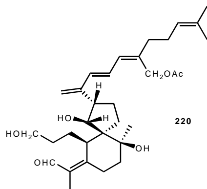
Figure 31 : 29-acétoxy-spiroiridal.
