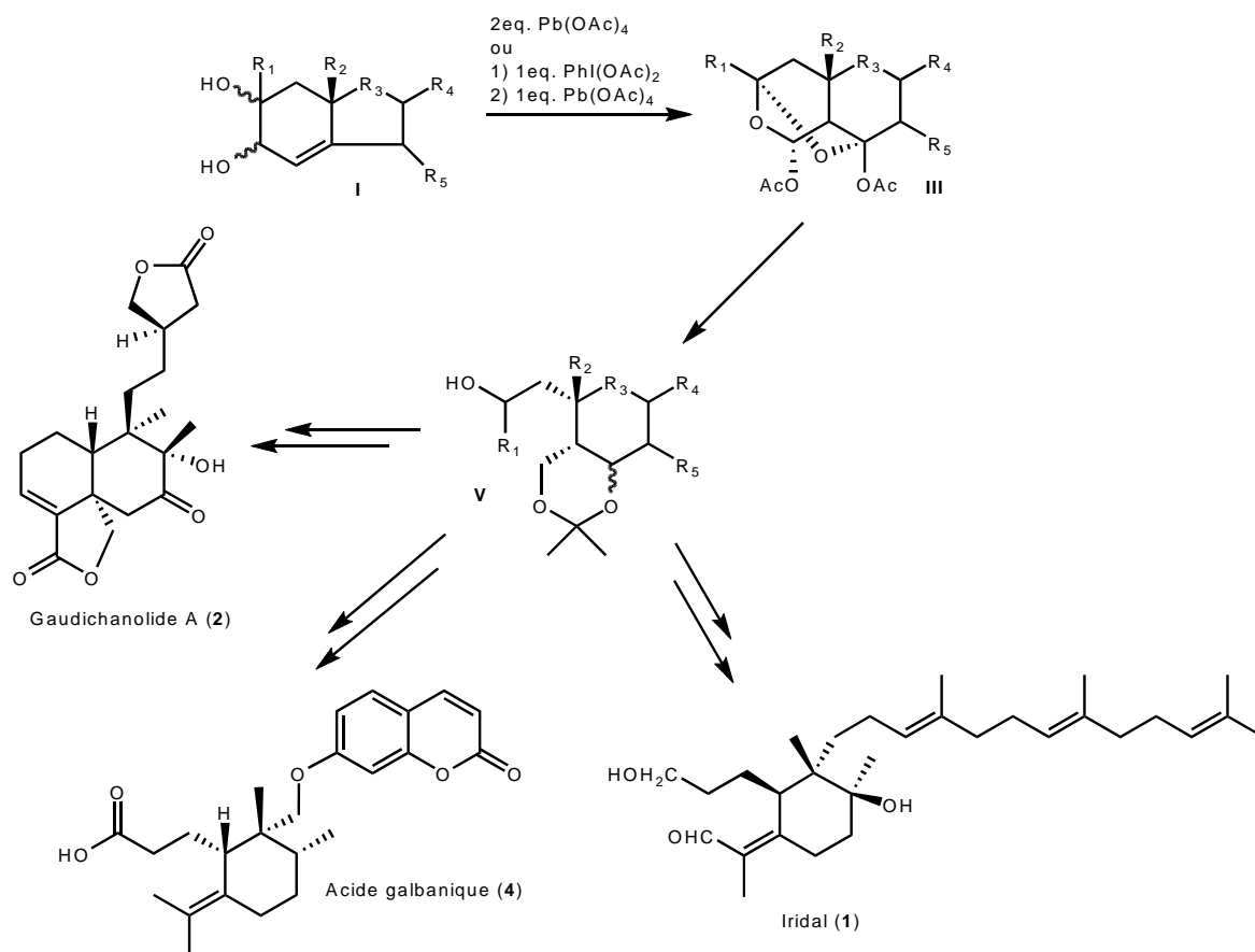
Schéma 2 : Une grande variété structurale accessible.
