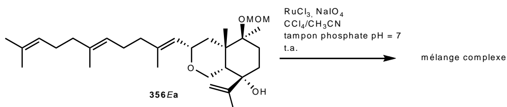
Schéma 105 : Essai de formation de la lactone en C5.
