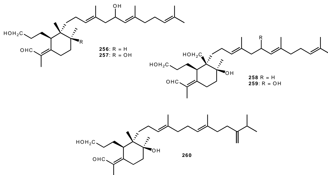
Figure 28 : Quelques exemples d'iridals.
