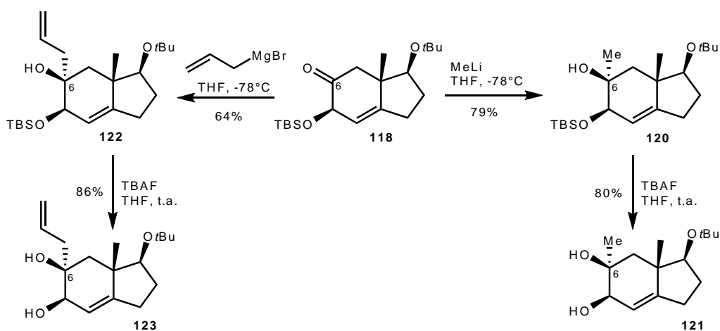
Schéma 34 : Synthèse des diols fonctionnalisés en position 6.
