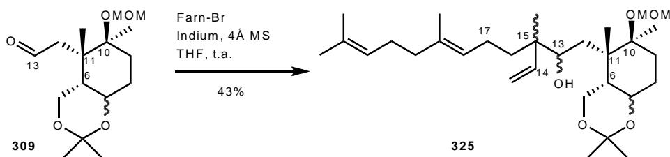
Schéma 84 : Couplage par l'indium. Addition en \gamma du bromure de farnésyle.
