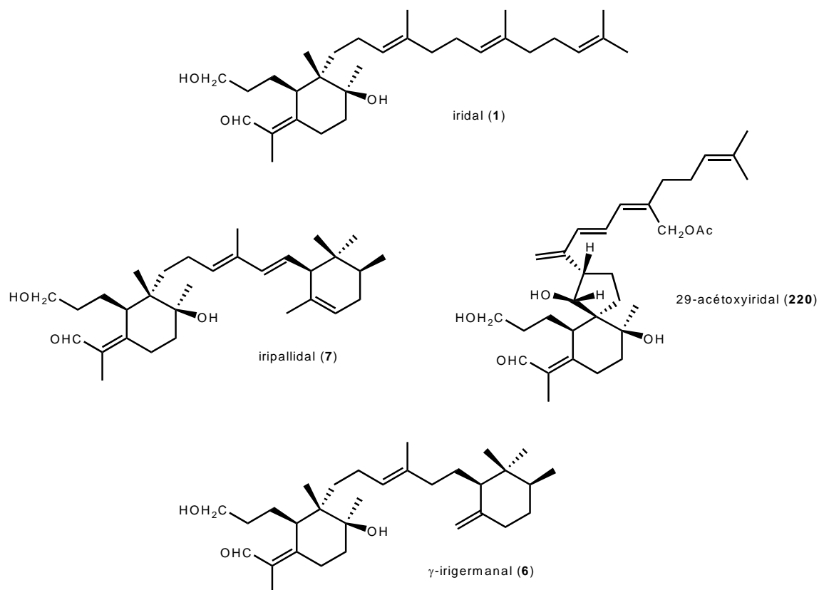
Figure 18 : Quelques exemples des trois sous-familles des iridals.
