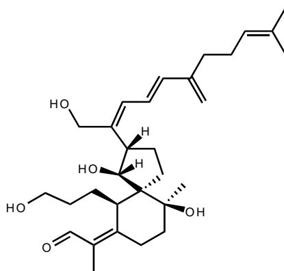
28-deacetylbelamcandal ( 262 )
