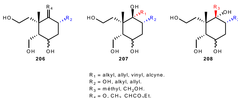
Figure 14 : Des cyclohexanes hautement fonctionnalisés.
