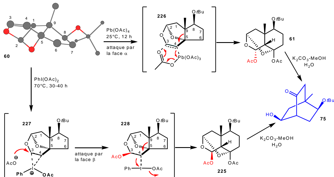
Schéma 55 : Chemin réactionnel possible expliquant la différence de réactivité entre le \text{PhI}(\text{OAc})_2 et le \text{Pb}(\text{OAc})_4 .
