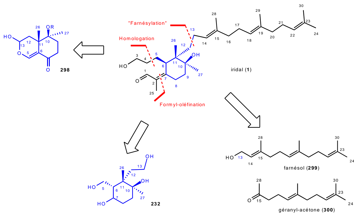
Schéma 68 : Rétrosynthèse proposée de l'iridal.
