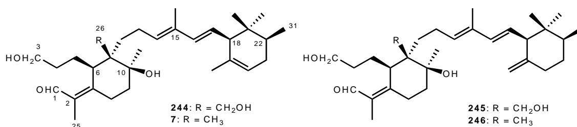
Figure 26 : Des précurseurs des irones.
