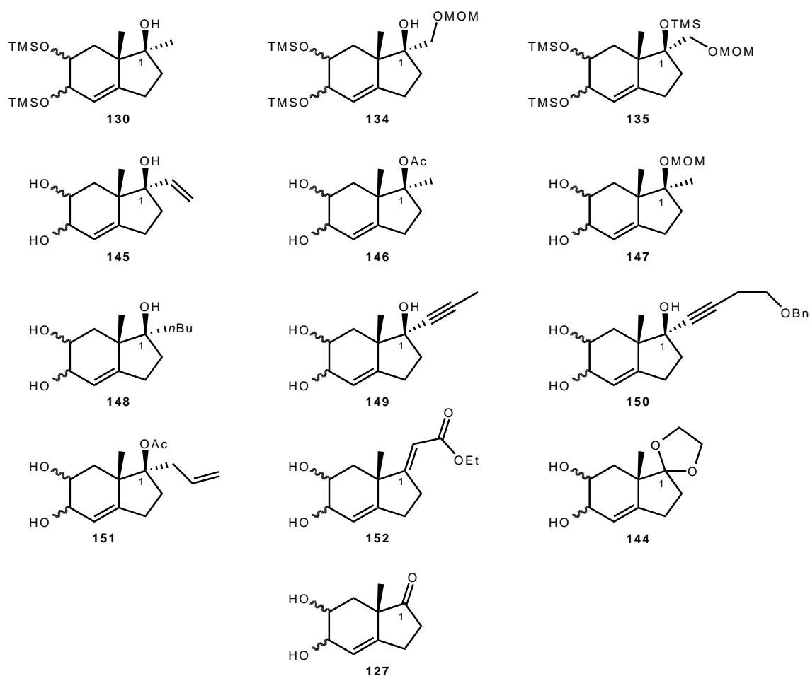
Schéma 41 : 13 diols insaturés dont 10 comportant deux centres quaternaires stéréodéfinis.
