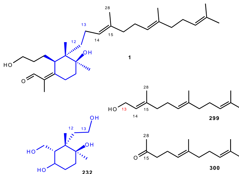
Figure 42 : Un carbone de trop ou un de moins.
