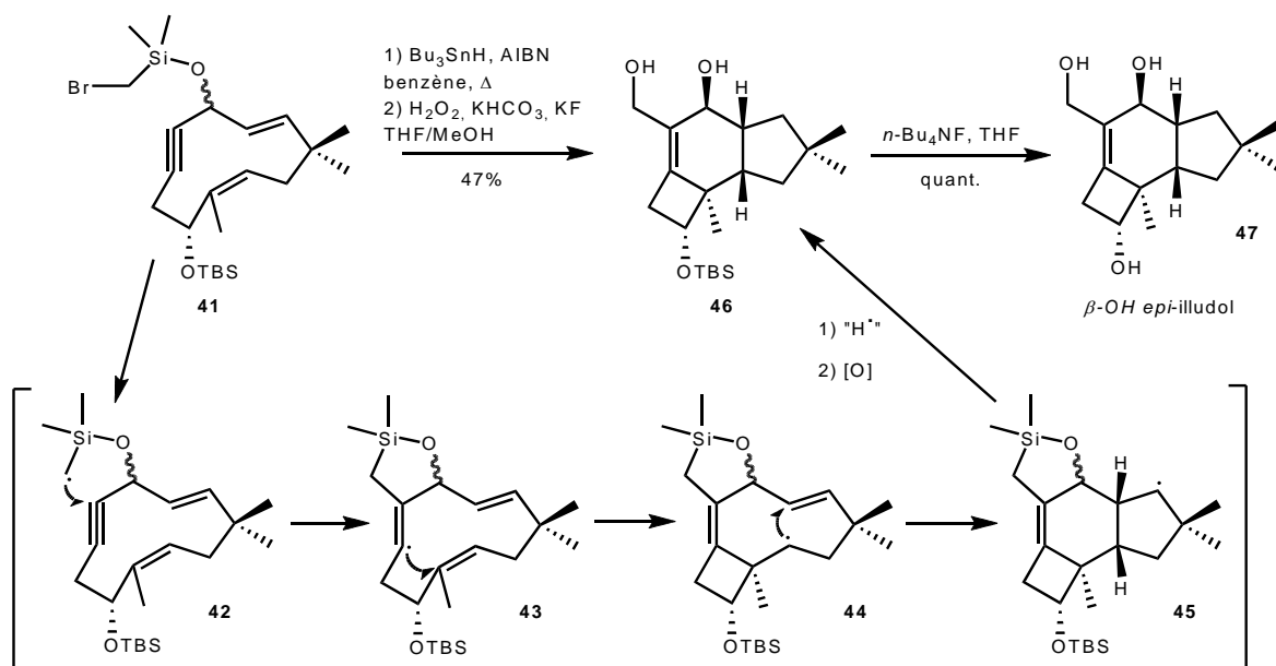
Schéma 11 : Réaction domino de type radicalaire. Synthèse de l'épi-illudol.
