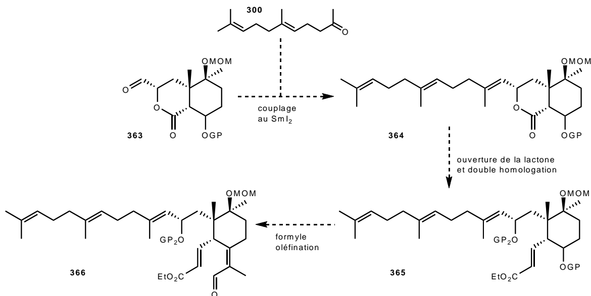
Schéma 109 : Voie de synthèse envisageable avec un couplage au samarium.
