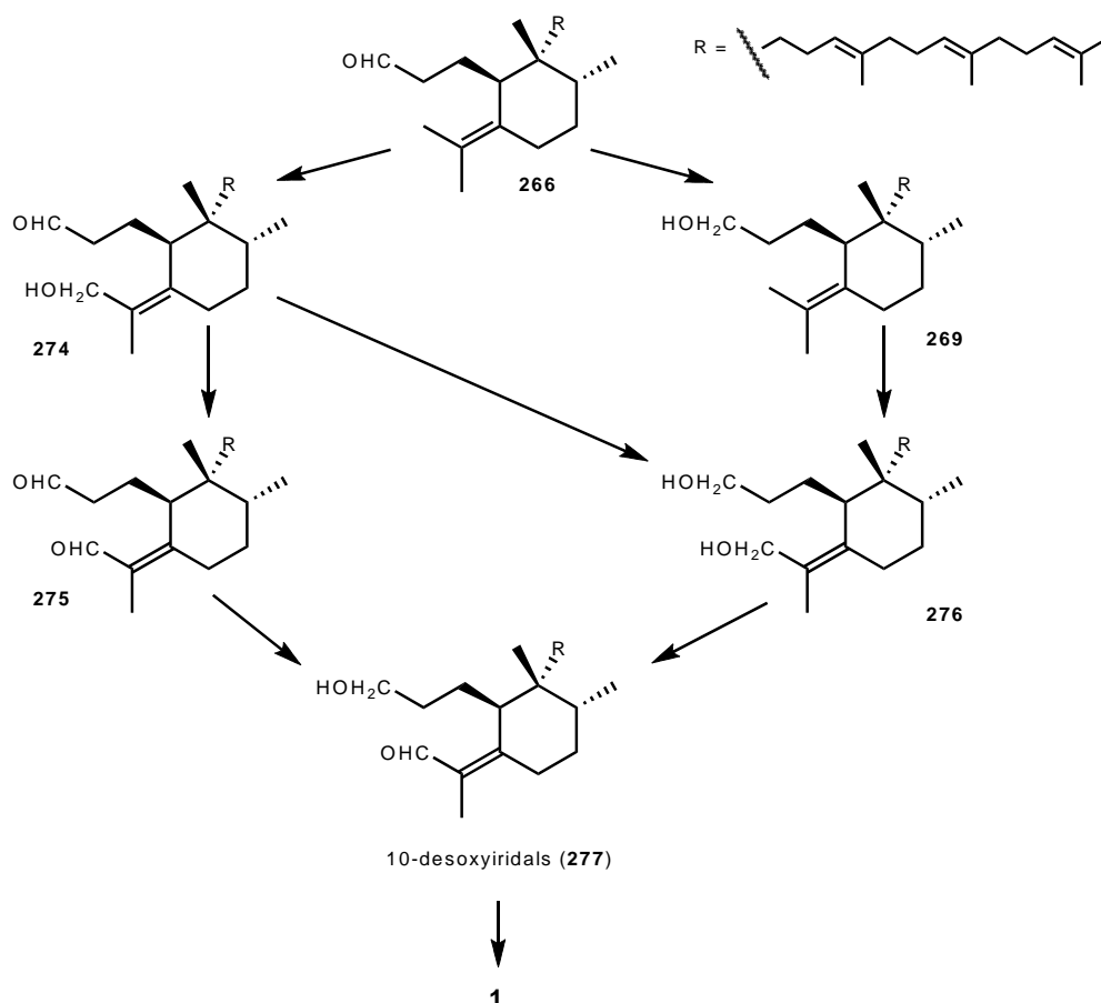
Schéma 63 : Intermédiaire attendu lors de l'inhibition de la synthèse de spiroiridals.
