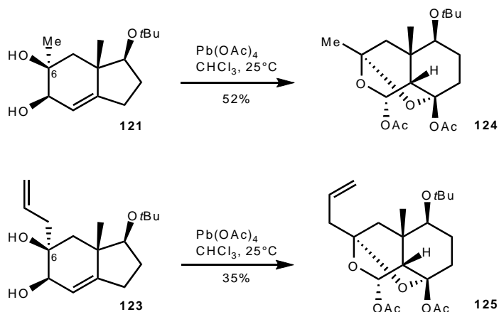
Schéma 35 : Réactions domino avec un substituant en position 6.
