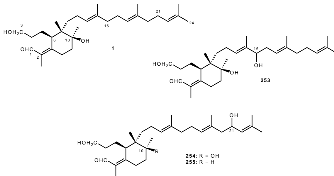
Schéma 61 : Quelques iridals à chaîne ouverte.
