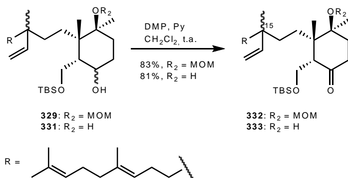
Schéma 88 : Oxydation de Dess-Martin.
