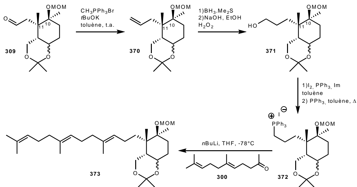
Schéma 122 : Couplage envisagé de la chaîne homofarnésyle.
