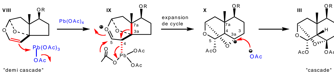
Schéma 18 : Le plomb agit comme acide de Lewis.
