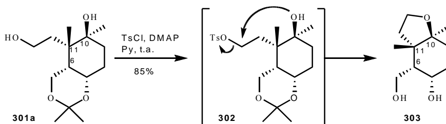
Schéma 71 : Formation du furane 303 .
