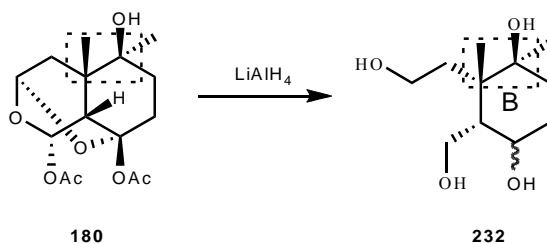
Schéma 110 : Réduction de la "cascade" 180 pour obtenir le cyclohexane 232 .
