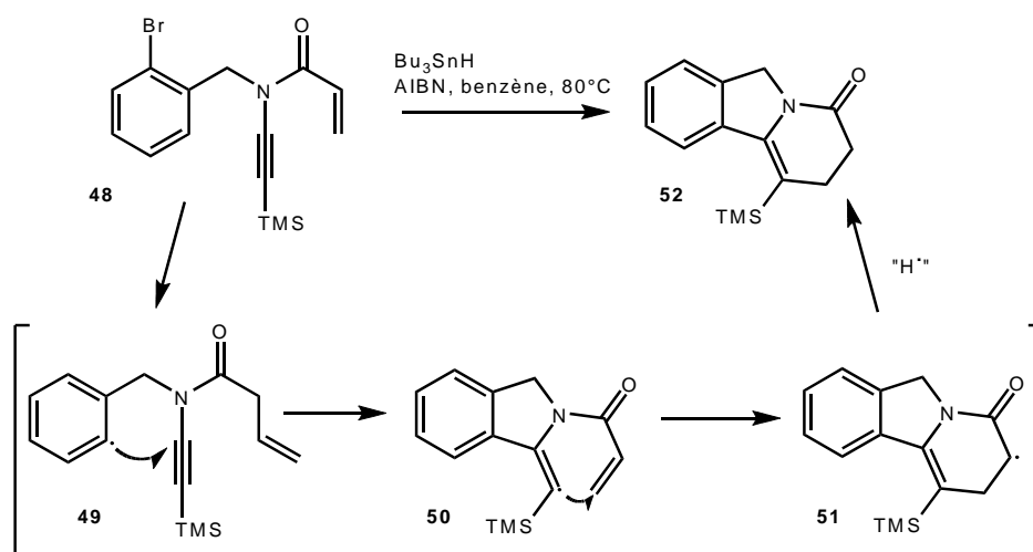
Schéma 12 : Exemple de polyhétérocycle obtenu par réaction domino radicalaire.
