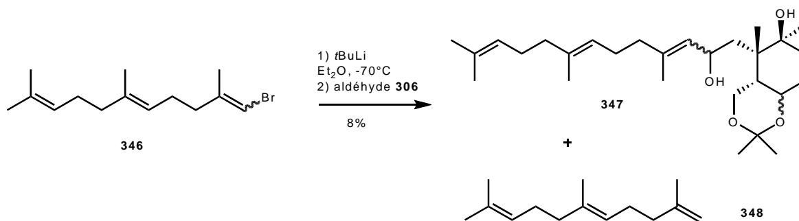
Schéma 97 : Couplage par échange halogène-lithium.
