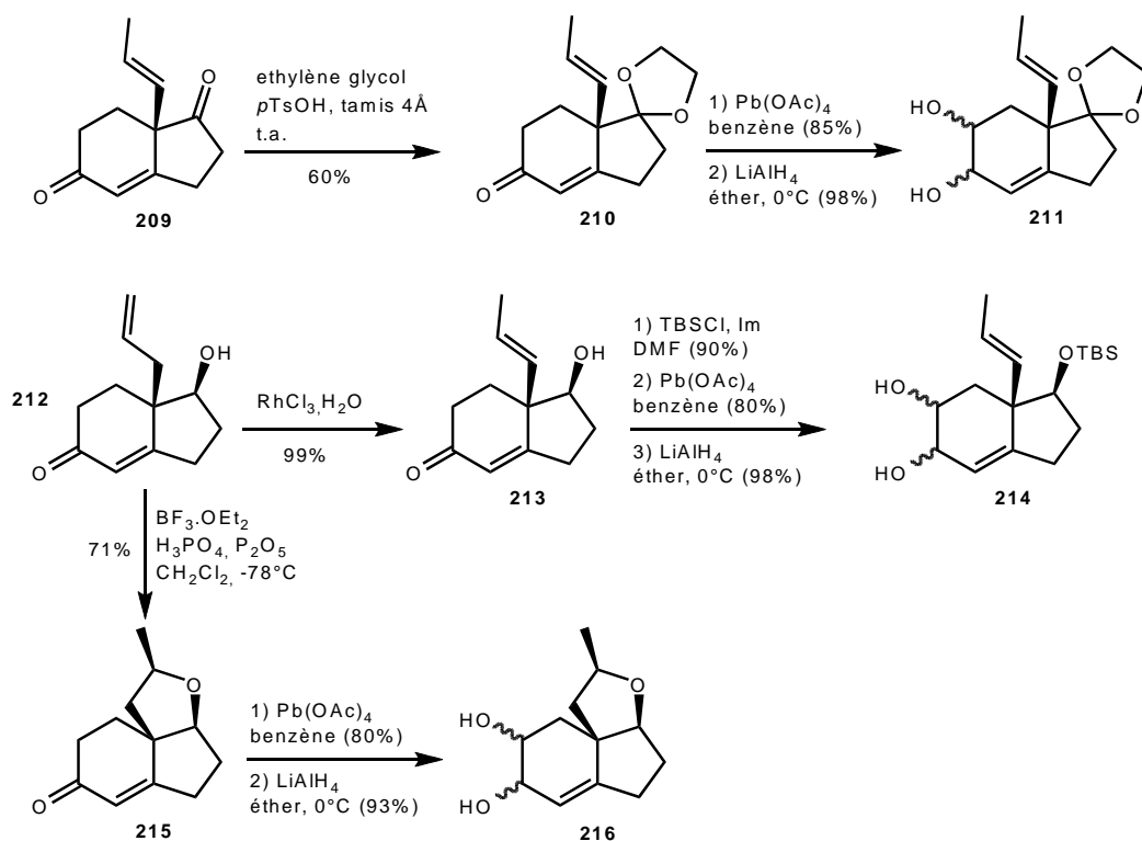
Schéma 51 : Synthèse de 3 diols fonctionnalisés en position 7a.
