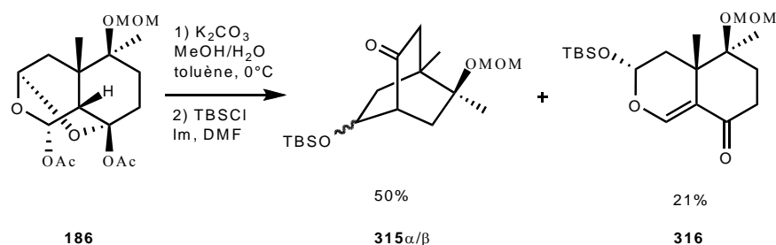
Schéma 79 : Synthèse de l'énone 316.
