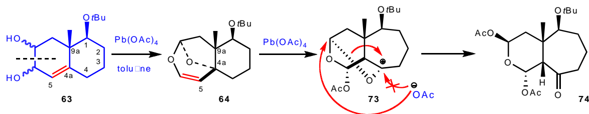
Schéma 19: Réaction domino avec la série Wieland-Miescher.
