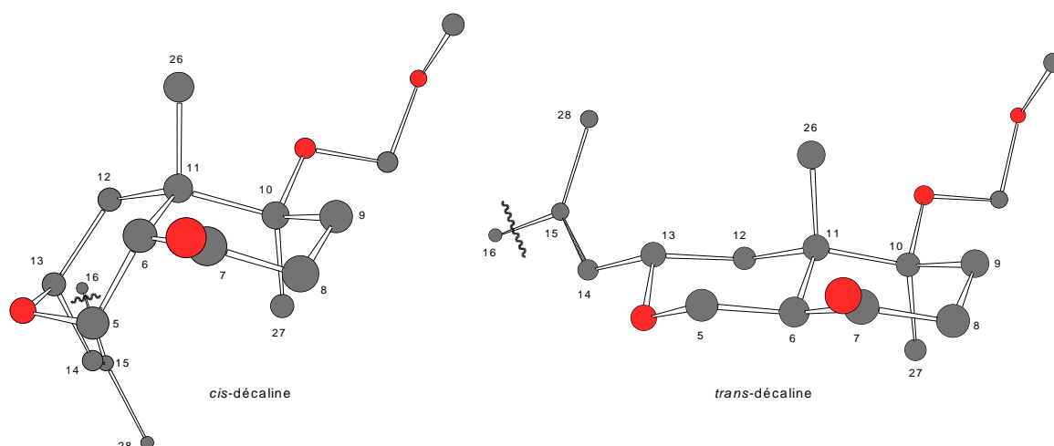
Figure 47 : Conformères de plus basse énergie de la cétone 354E : forme cis et trans .
