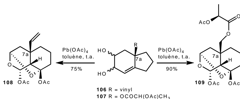
Schéma 28 : Des réactions de cascade avec un groupement différent de méthyle, en position 7a.
