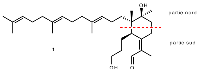
Schéma 69 : Découpage de l'iridal.
