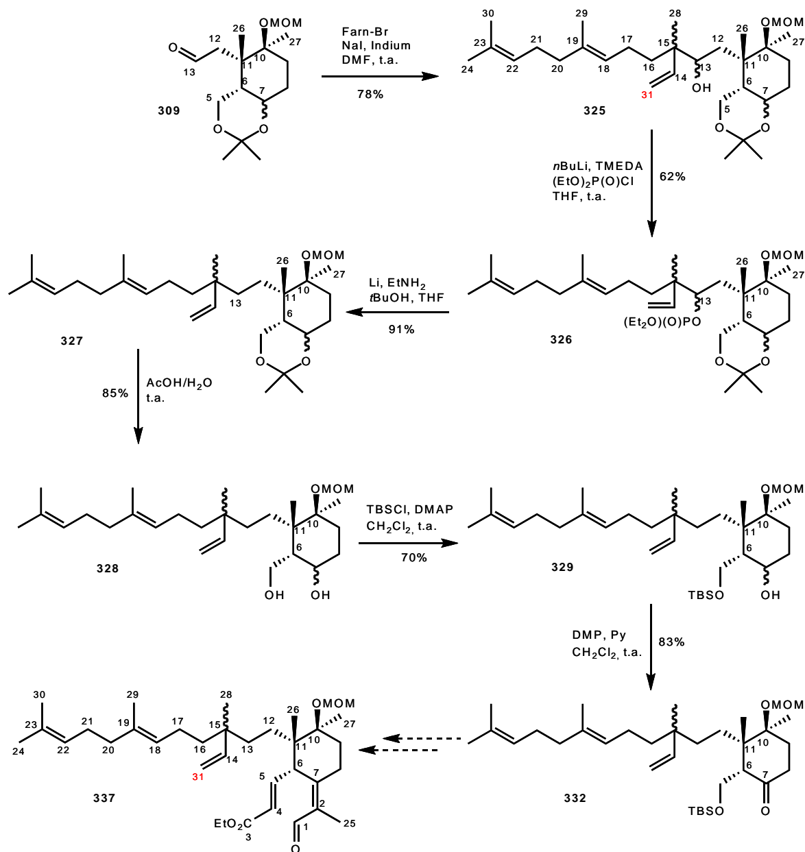
Figure 20 : Voie de synthèse avec couplage à l'indium.
