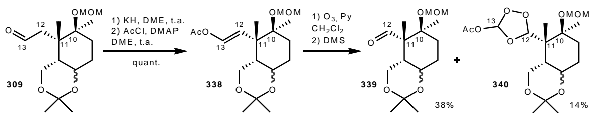
Schéma 90 : Ozonolyse.
