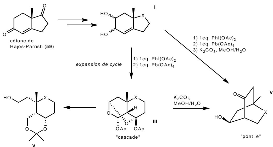
Schéma 114 : La réaction domino initiée par le \text{Pb}(\text{OAc})_4 mène à une grande diversité structurale.
