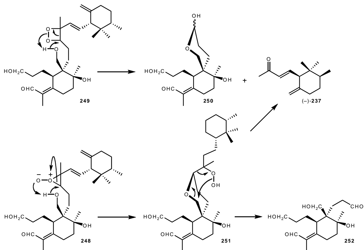
Schéma 60 : Participation possible de l'alcool en C26 dans la formation des irones.
