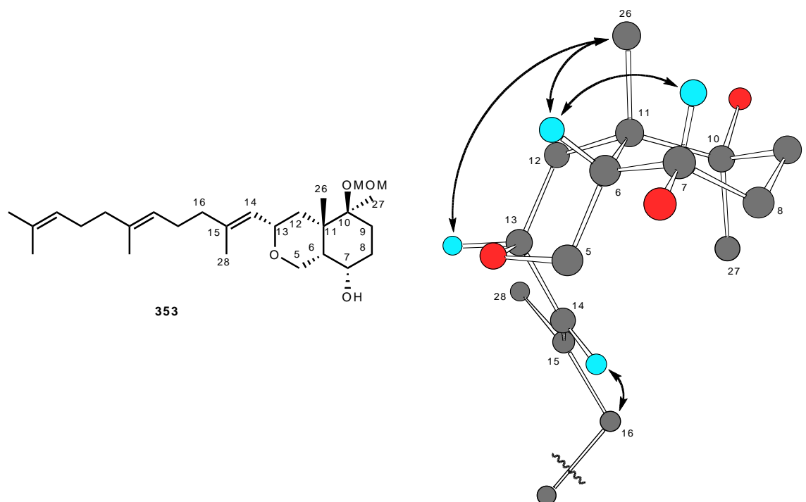
Figure 44 : Confirmation des configurations de l'alcool 353 par expérience ^1\text{H} -RMN-NOESY (représentation du conformère de plus basse énergie).
