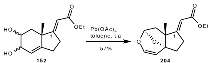
Schéma 49 : Un produit de "demi-cascade" isolable.
