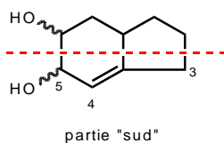
Figure 10 : Les différentes positions fonctionnalisables de la partie "sud".
