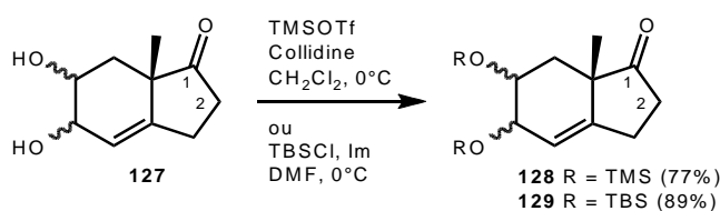
Schéma 37 : Protection du diol 127 .
