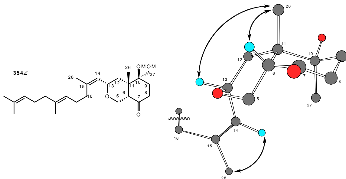
Figure 46 : Confirmation des configurations de la cétone 354Z par expérience ^1\text{H} -RMN-NOESY (représentation du conformère de plus basse énergie).
