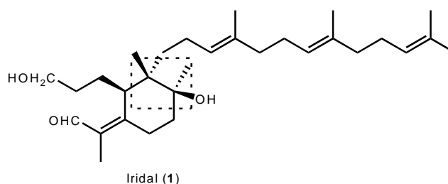
Figure 1 : L'iridal.
