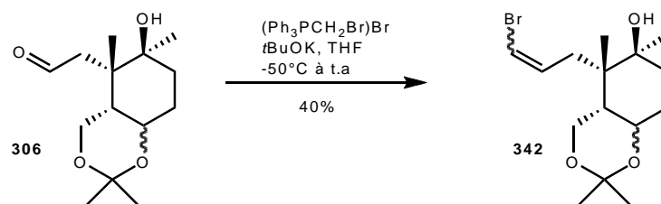
Schéma 93 : Bromométhylenation.
