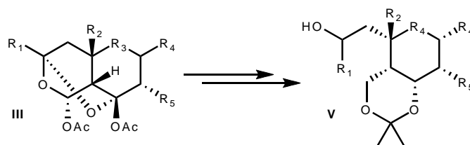
Schéma 59 : Des cycles à six chaînons très fonctionnalisés.
