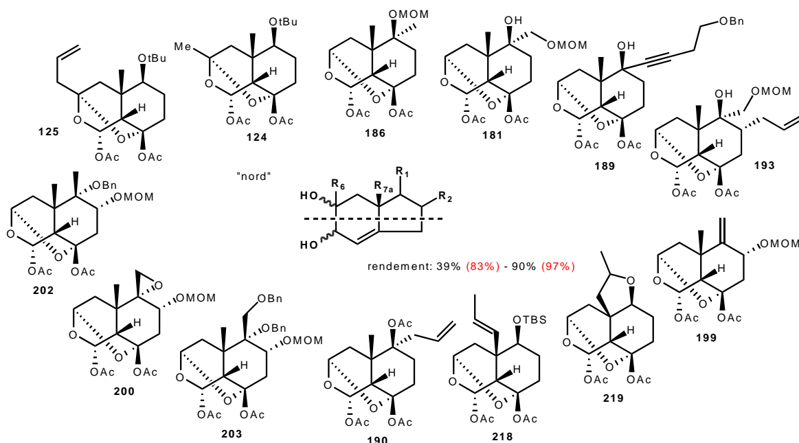
Schéma 117: La partie "nord" accepte une grande diversité fonctionnelle (rendement de la réaction, rendement moyen par transformation de la réaction domino).
