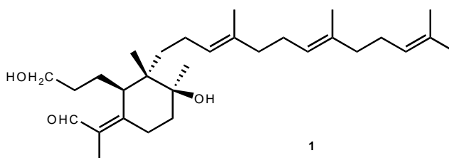
Figure 15 : L'iridal.
