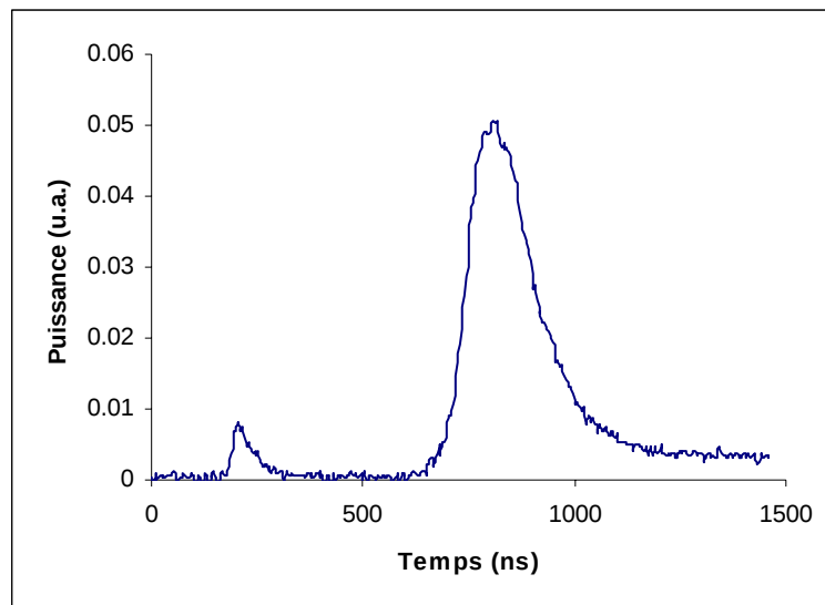
Figure V-1. Impulsions en sortie de laser déclenché à base de \text{Nd}:\text{GdVO}_4 .
