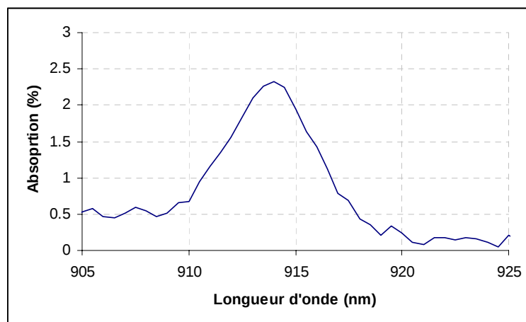
Figure III-21. Spectre d'absorption sur un passage autour de 914 nm d'un cristal de \text{Nd:YVO}_4 dopé à 0.1 % et long de 5 mm.
