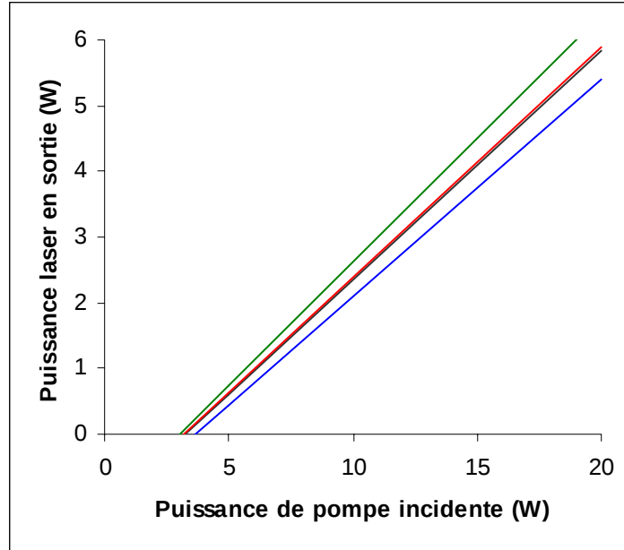
Figure II-17. Comparaison des performances laser calculées en régime continu d'un cristal de \text{Nd}:\text{GdVO}_4 (courbe noire) avec celle de cristaux possédant la section efficace d'émission (courbe bleue), sa section efficace d'absorption (courbe bleue) ou la répartition de population de son niveau fondamental (courbe rouge) du \text{Nd}:\text{YVO}_4 .
