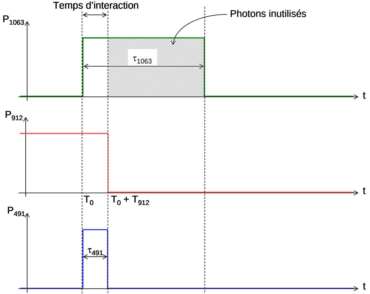
Figure IV-9. Evolution des puissances instantanées à 1063 nm, 912 nm et 491 nm dans le cas d'impulsions de forme carrée lorsque T_{912} < \tau_{1063} .
