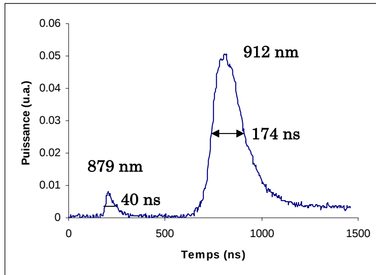
Figure V-12. Impulsions en régime déclenché à 879 nm et 912 nm avec un cristal de \text{Nd}:\text{GdVO}_4 et un coupleur de sortie de 4.7 %.
