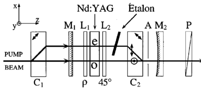
Figure III-2. Source micro-onde basée sur un laser bi-longueur d'onde utilisant un élément biréfringent [Brunel 97].
