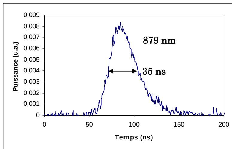
Figure V-13. Impulsion déclenchée à 879 nm avec un cristal de \text{Nd}:\text{GdVO}_4 et un coupleur de sortie de 25.5 %.
