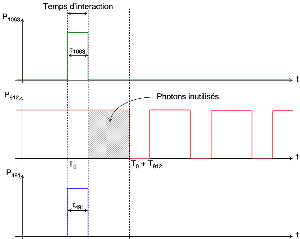
Figure IV-8. Evolution des puissances instantanées à 1063 nm, 912 nm et 491 nm dans le cas d'impulsions de forme carrée lorsque \tau_{1063} < T_{912} .
