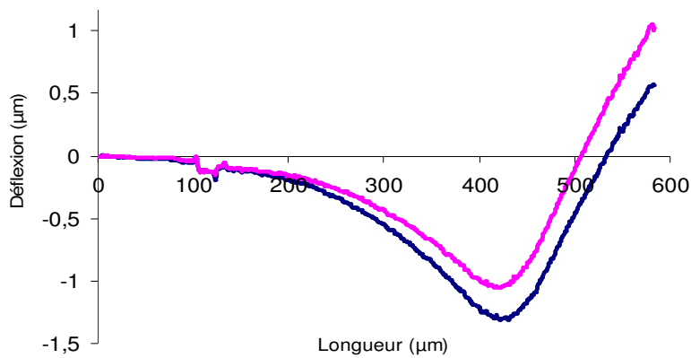
Figure III-10: Profil de la micropoutre aux extremums du 1 er mode de résonance (F1=11069Hz, V PZT =10V)
