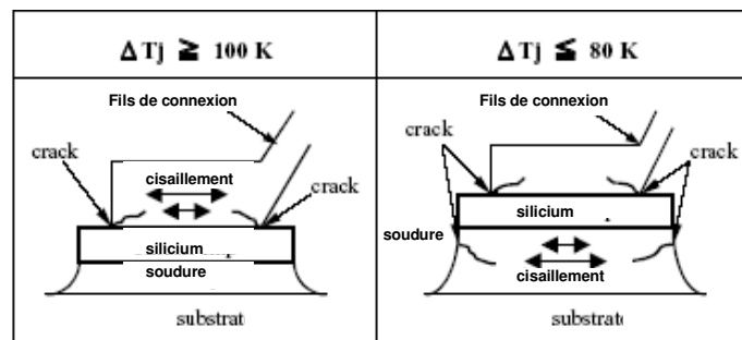
Figure I-30: Illustration des mécanismes de défaillance en fonction de la température [MOR01]
