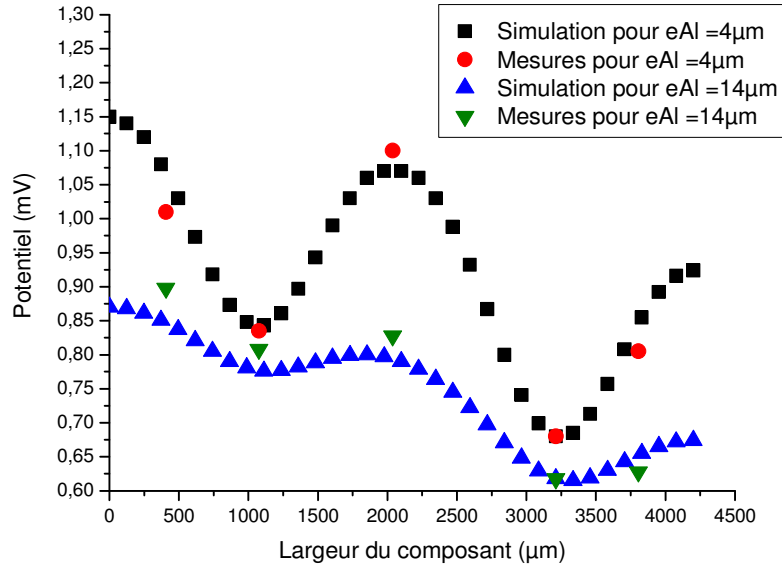
Figure IV-13 : Mesures et simulations des potentiels à la surface du métal pour un double contact fil-métallisation
