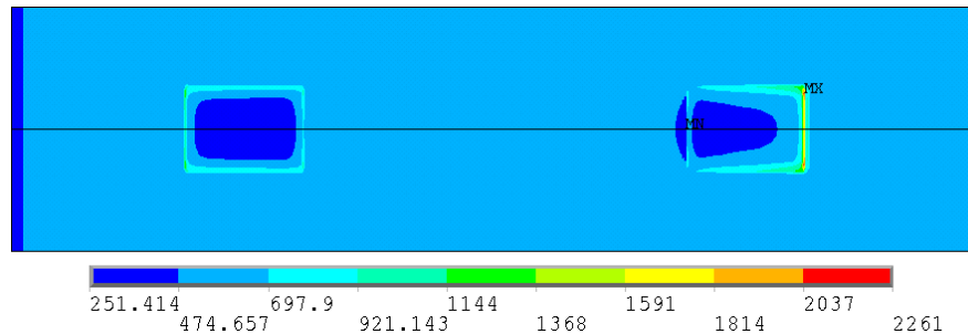
Figure IV-34 : Contraintes de Von Mises (MPa) sur 1/8 ème de la métallisation (eAl= 4µm)
