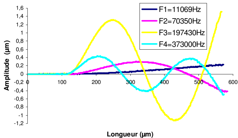
Figure III-11: Déflexions de la micropoutre pour les quatre premiers modes de résonance (V PZT =10V)
