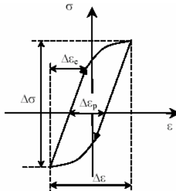
Figure I-28: Illustration d'un cycle contrainte déformation, élastique et plastique
