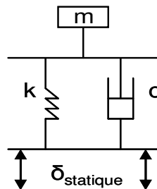
Figure I-21: Oscillateur amorti avec excitation à la base
