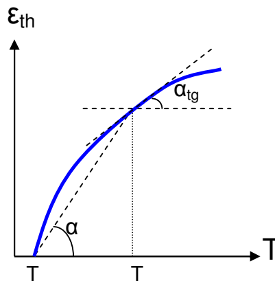
Figure I-4 : Représentation graphique du coefficient de dilatation thermique
