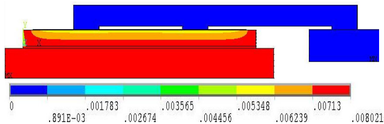
Figure IV-10 : Distribution des potentiels (V) sur le modèle pour I_{DS}=5A
