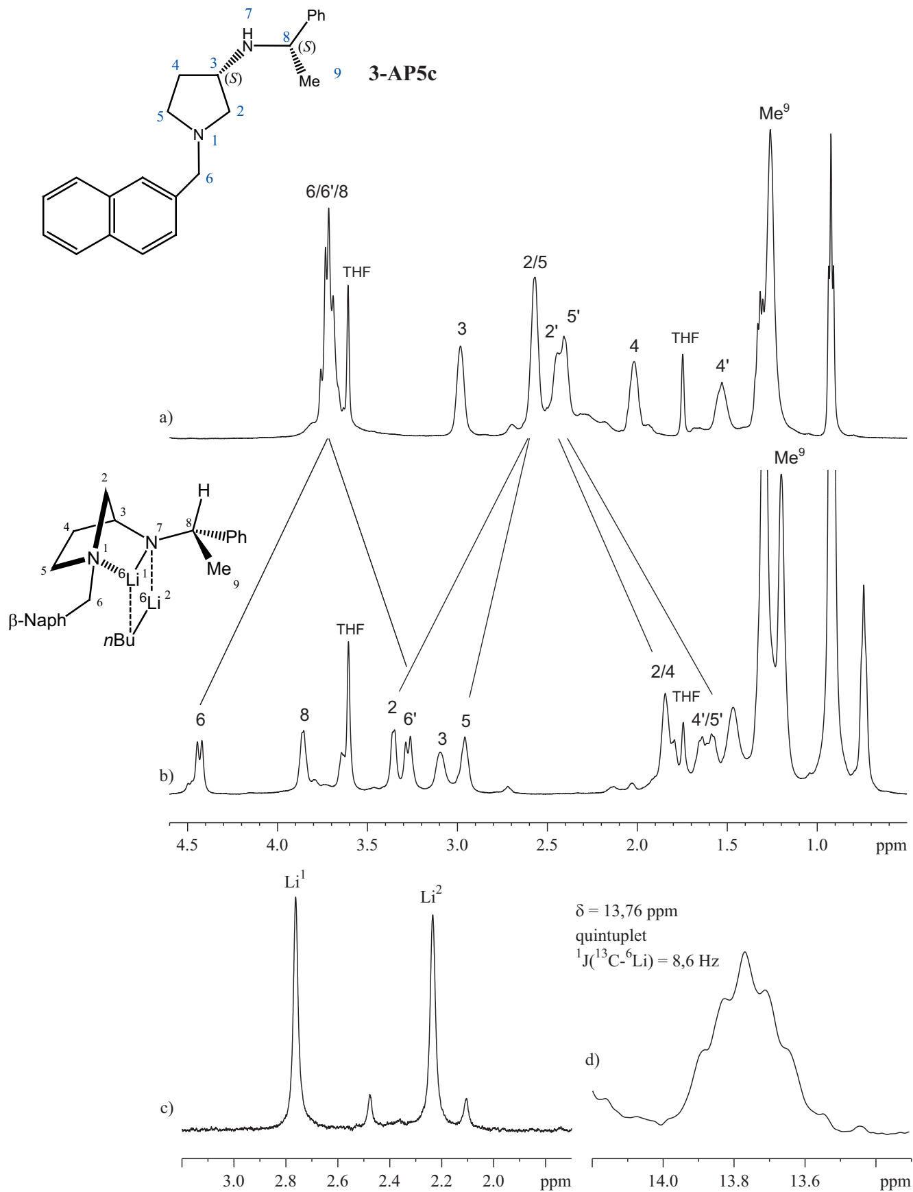
Figure 40. Spectres RMN à une dimension de l'amine et du complexe dans le \text{THF-}d_8 à T = 195\text{K} a) Spectre 1D ^1\text{H} de l'amine 3-AP5c ; b) Spectre 1D ^1\text{H} , c) Spectre 1D ^6\text{Li} , d) Spectre 1D ^{13}\text{C} de l'agrégat 3-AP5c / n\text{Bu}^6\text{Li} .
