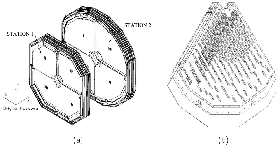
FIG. 0.1 –: (a) Vue schématique de l’assemblage des quarts de chambres des stations 1 et 2. Les lettres B et NB situées sur les faces indiquent respectivement les plans bending et non-bending . Le sens ( X, Y, Z ) des coordonnées est également indiqué. (b) Vue artistique d’un quart de chambre.
