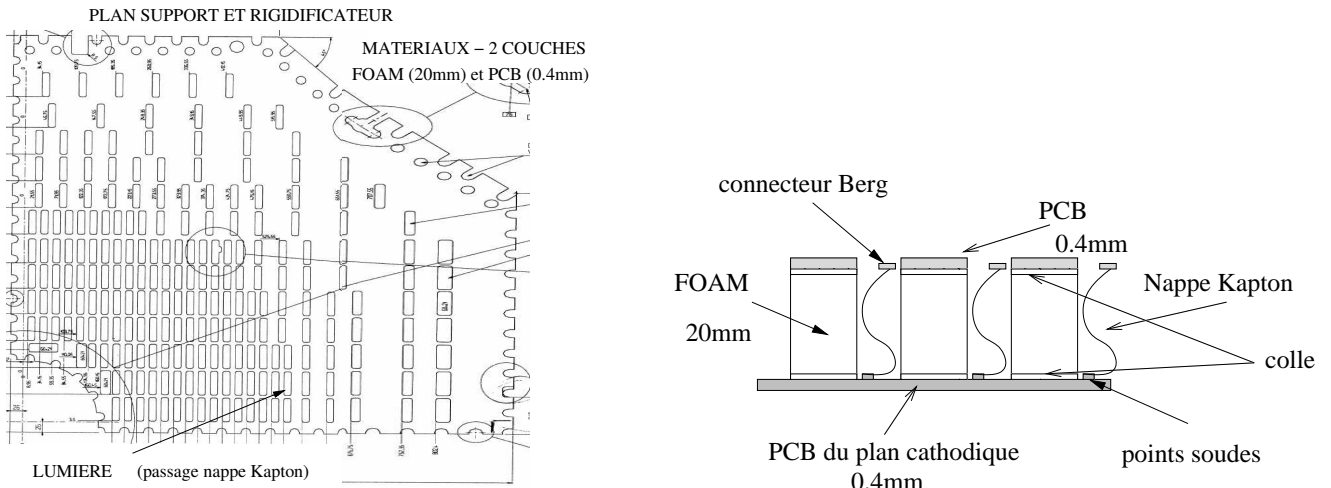
(a) Plan de principe qui montre la configuration géométrique de lumières.
