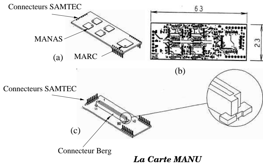
FIG. 0.14 –: Vue schématique de l'emplacement des puces et des connecteurs SAMTEC sur les cartes filles (a). Les dimensions sont portées sur la figure (b) et l'emplacement du connecteur Berg, posé sur le dessous des cartes, est visible dans la partie (c).
