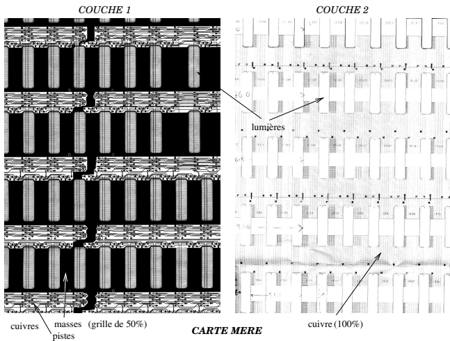
FIG. 0.10 –: Une partie des couches cuivrées de la carte mère. Le dessin de gauche correspond à la couche de masse et aux pistes de transmission des signaux, tandis que celui de droit représente le plan des alimentations.
