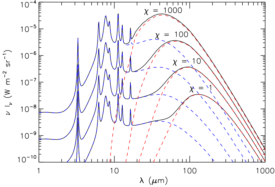
FIG. 2.6 – Spectre d'émission des poussières excitées par 1, 10, 100 et 1000 fois le champ de rayonnement interstellaire moyen de Mathis et al. (1983) et pour N_H = 10^{20} \text{ cm}^{-2} . Les spectres en tirets bleus et rouges sont respectivement les contributions des grains chauffés stochastiquement et des grains à l'équilibre thermique. Ces spectres sont obtenus avec le modèle DUSTIAS décrit au chapitre 6.
