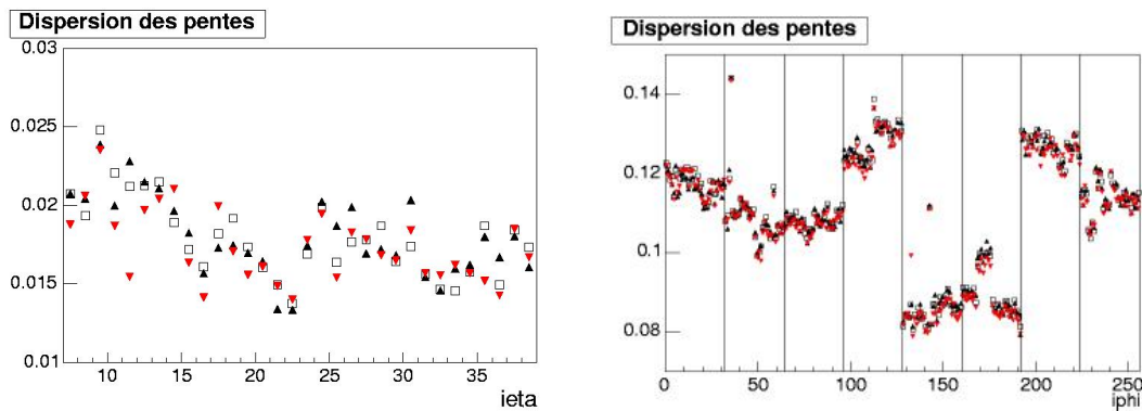
FIGURE 5.21 – Dispersion des valeurs des pentes des rampes, divisée par la pente moyenne, en fonction du numéro de cellule en \eta (gauche) et en \phi (droite) dans le compartiment du milieu d'un des bouchons du calorimètre électromagnétique. Les gains haut (triangles), moyen (carrés) et bas (triangles inversés) sont représentés. La dispersion correspond à la largeur d'un ajustement gaussien pour \eta ; la statistique étant faible pour \phi , un tel ajustement n'a pas pu être effectué et l'écart type a été utilisé. Les limites entre modules sont indiquées pour \phi .
