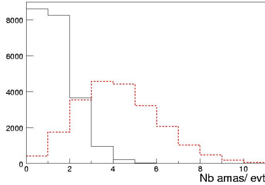
FIGURE 5.26 – Nombre d'amas reconstruits par l'algorithme LArMuID, avec un seuil large (100 et 50 MeV), en utilisant cinq (ligne rouge pointillée) ou vingt-neuf (ligne noire pleine) coefficients de filtrage optimal.
