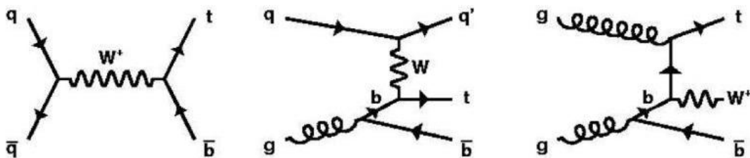
FIGURE 2.4 – Diagrammes de production de tops par interaction faible (“tops seuls” ou single tops), au premier ordre.
