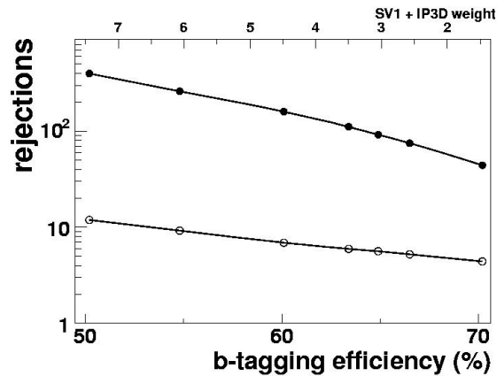
FIGURE 4.9 – Facteur de rejet des jets légers (points) et des jets c (cercles) en fonction de l'efficacité d'étiquetage des jets de b . La méthode utilisé est SV1+IP3D .
