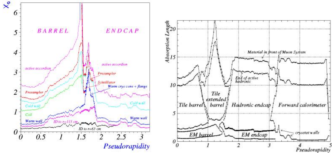
FIGURE 3.10 – Gauche : quantité de matière, exprimée en longueurs de radiation X_0 , de chaque composant placé en amont du calorimètre électromagnétique d’ATLAS, en fonction de la pseudo-rapidity \eta . Droite : équivalent en quantité de matière, exprimée en longueurs d’absorption \lambda_I , de chaque partie du système de calorimétrie d’ATLAS, en fonction de la pseudo-rapidity \eta .
