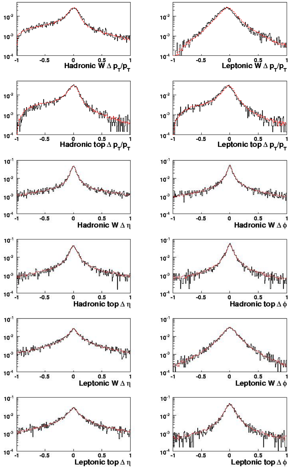
FIGURE 4.17 – Résolutions globales pour l'impulsion transverse ( \frac{\Delta p_T}{p_T} ) et la direction ( \Delta\eta et \Delta\phi ) des bosons W et quarks top reconstruits. Les courbes pleines noires correspondent à la simulation détaillée, et les courbes rouges en pointillé à la simulation simplifiée.
