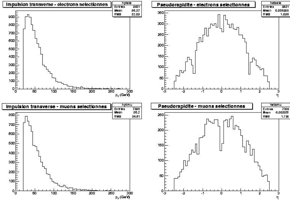
FIGURE 4.6 – Distributions de l'impulsion transverse et de la pseudo-rapidité \eta pour le lepton isolé sélectionné. En haut : électron, en bas : muon.
