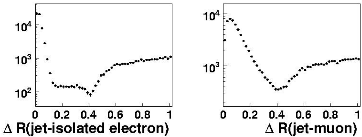
FIGURE 4.7 – Distance ( \Delta R ) entre le lepton et le jet le plus proche. À gauche, le lepton est l'électron isolé sélectionné ; à droite, tous les muons de l'événement avec p_T > 3 GeV.
