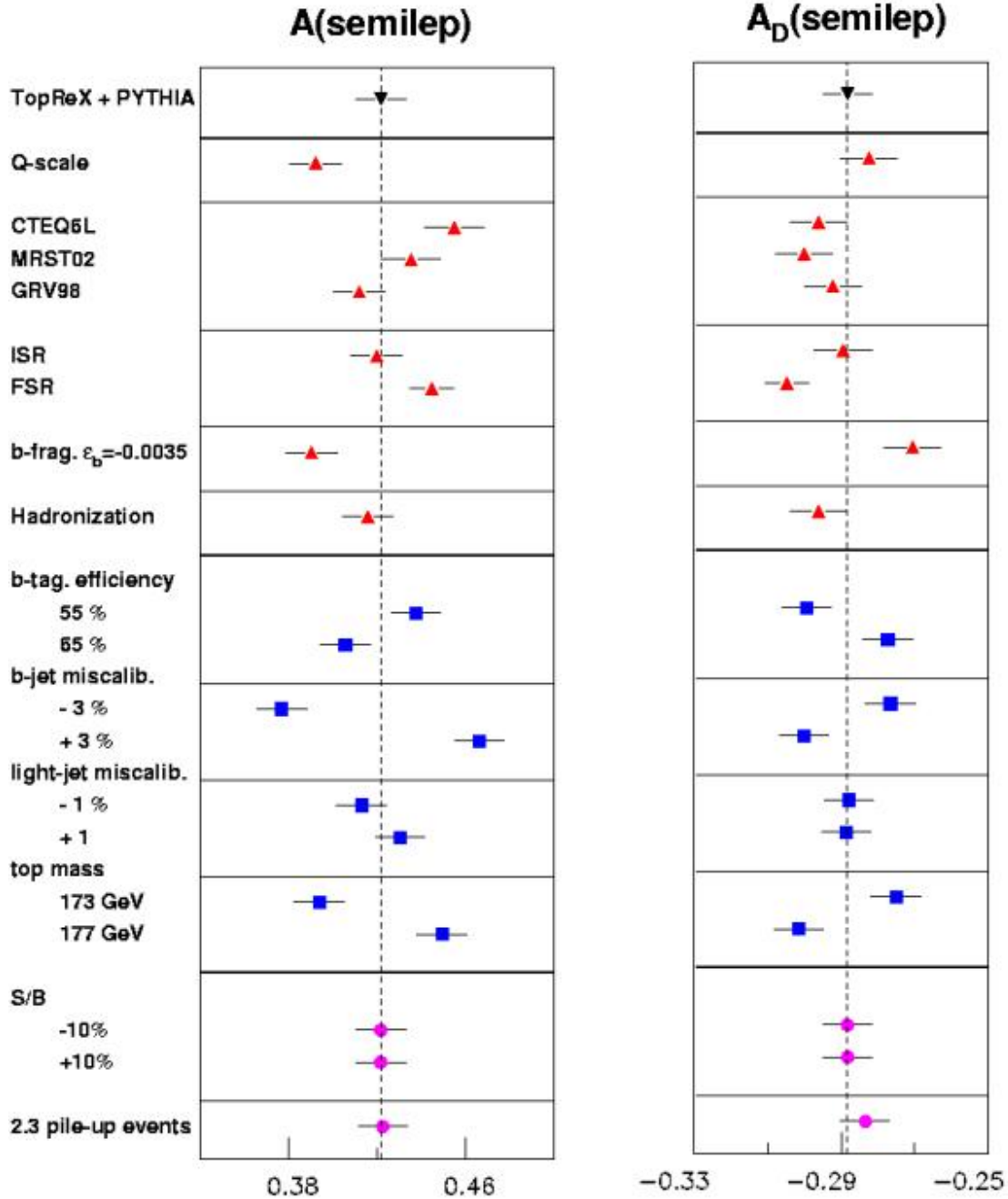
FIGURE 4.26 – Incertitudes systématiques sur la mesure des asymétries A et A_D , calculées en simulation simplifiée pour des événements t\bar{t} semileptoniques.
