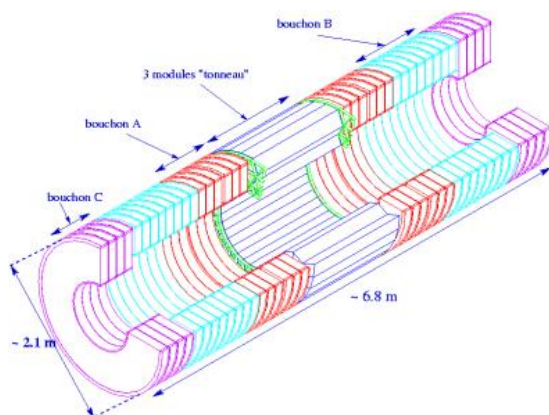
FIGURE 3.8 – Gauche : représentation schématique du trajectographe à rayonnement de transition (TRT). La longueur totale a été réduite à |\eta| < 2.0 par rapport à la conception initiale. Droite : vue du TRT tonneau, installé avec le SCT tonneau.
