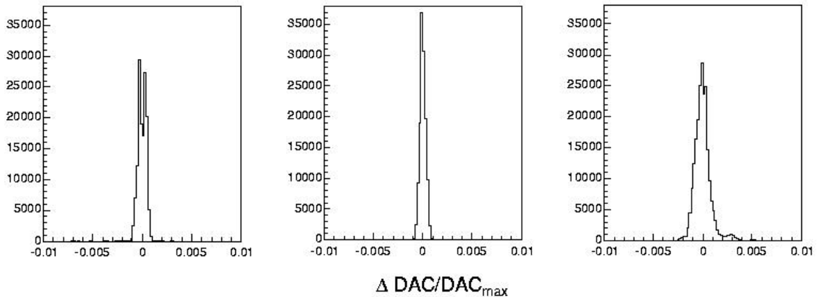
FIGURE 5.18 – Écart relatif \frac{DAC_{cal}-DAC_{int}}{DAC_{max}} entre la valeur de DAC utilisée dans l'étalonnage et celle issue de l'interpolation linéaire de la rampe. Ces valeurs correspondent au compartiment du milieu d'un des bouchons du calorimètre. Les gains haut, moyen et bas sont représentés de gauche à droite.
