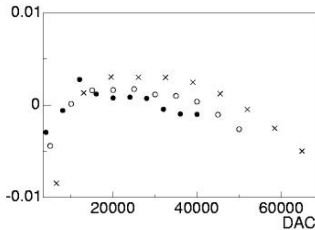
FIGURE 5.19 – Écart relatif \frac{A_{reco} - A_{ij}}{A_{reco}} entre la valeur d'amplitude reconstruite et l'interpolation linéaire A_{ij} = f(DAC) , en fonction de la valeur du DAC, en bas gain. Ces valeurs sont des moyennes sur le compartiment du milieu d'un des bouchons du calorimètre. Les trois gammes de valeurs utilisées pour les différents lots de données sont représentées : 4000-40000 (disques), 5000-50000 (cercles) et 6500-65000 (croix).
