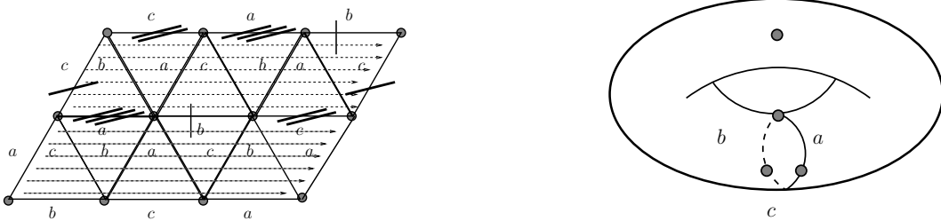
La surface de translation \Sigma_\theta lorsque \theta est non singulière.
