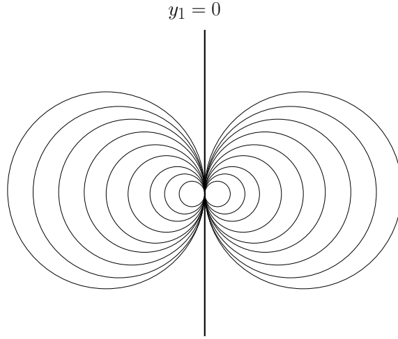
\mathcal{F}_{a,\lambda,\theta=0} sur un droite invariante d_1 .
