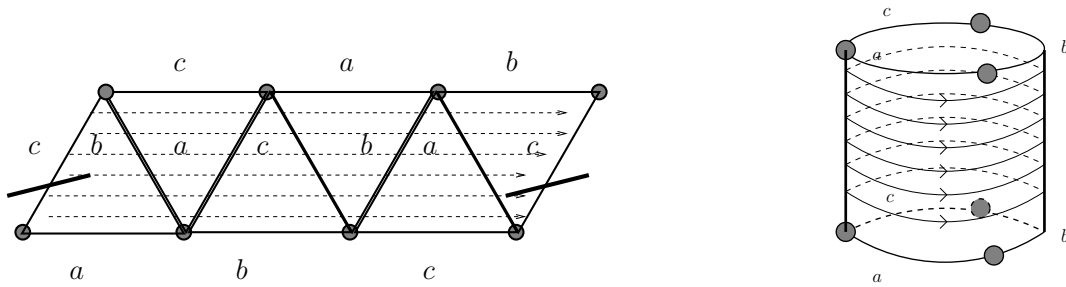
La surface de translation \Sigma_\theta lorsque \theta est non singulière.
