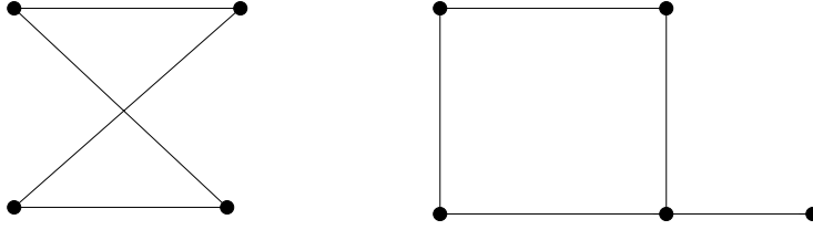
Polygones dégénérés.
