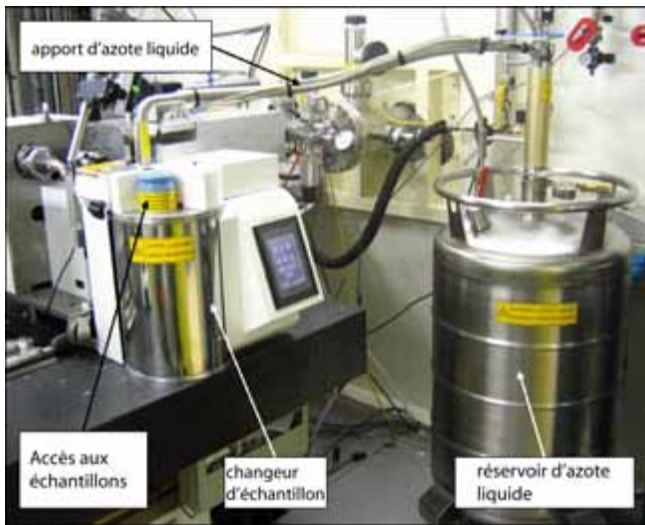
(a) Vue d'ensemble de la ligne de lumière avec changeur d'échantillon
