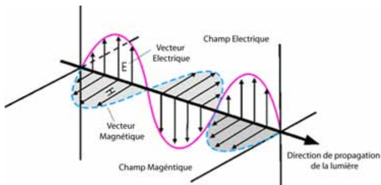
FIG. 9.1: La lumière est une onde électromagnétique (OEM) formée d’une composante électrique et d’une composante magnétique perpendiculaire.
