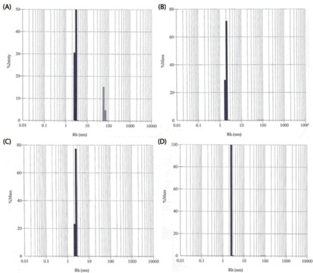
FIG. 11.5: Influence de la nature du tampon et de la présence d'Ugi sur l'homogénéité de l'échantillon. (A) UNG \Delta 24 seule. (B) UNG \Delta 24 + 10 mM DTT. (C) UNG \Delta 24 + Ugi. (D) UNG \Delta 24 + 10 mM DTT + Ugi.
