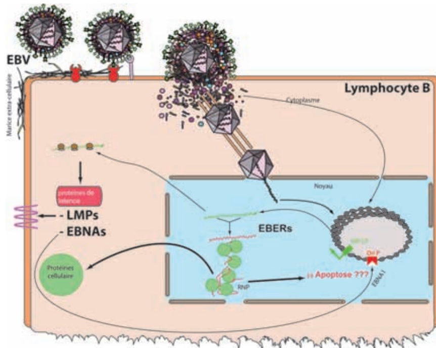
FIG. 2.5: Infection latente des lymphocytes B. EBNA1 interagit avec l'origine de réplication Orip et maintient le génome sous formes épisomale. Les gènes correspondants aux autres protéines EBNA sont transcrits à partir des promoteurs Wp ou Cp. Les EBERS restent majoritairement dans le noyau. Leurs rôles vont de l'inhibition de l'apoptose à la stimulation de la prolifération cellulaire. La protéine membranaire LMP1 est essentielle pour le processus de transformation.
