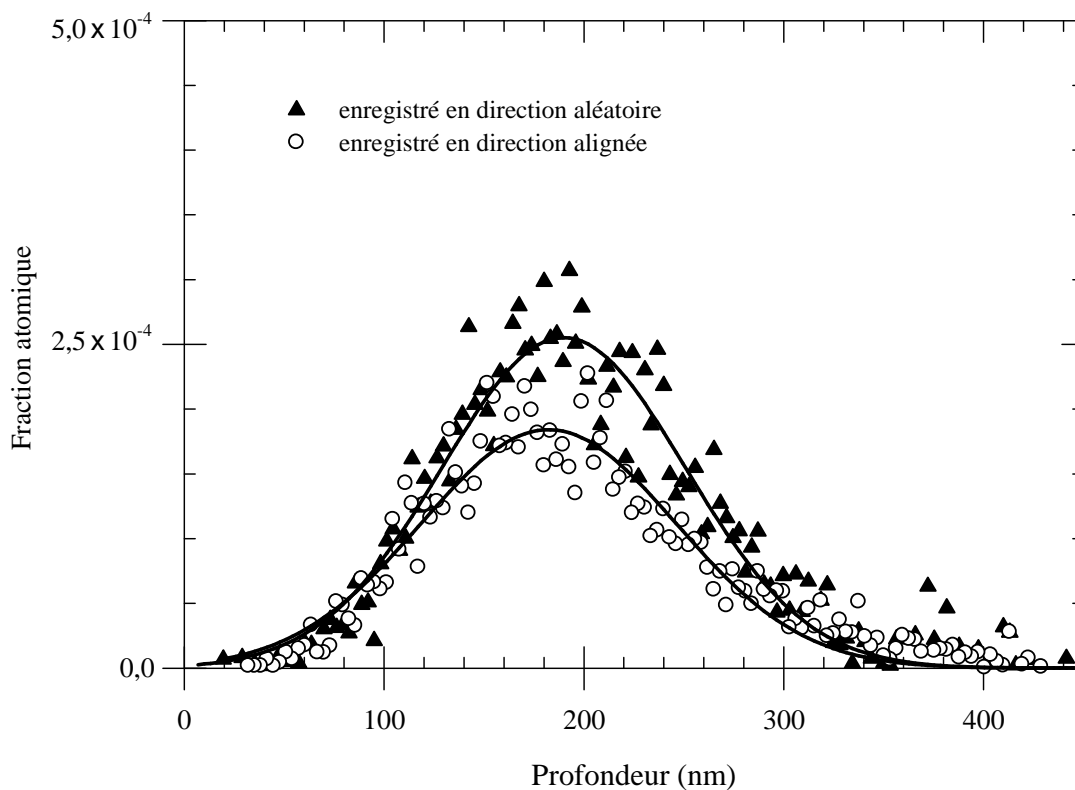
Figure 31 : Profils d'iode obtenus après implantation à la fluence de 3,8 \times 10^{14} \text{ cm}^{-2} à 400^\circ \text{C} par l'analyse des spectres RBS enregistrés en direction aléatoire et de canalisation. Les courbes sont les ajustements des points expérimentaux par des gaussiennes.
