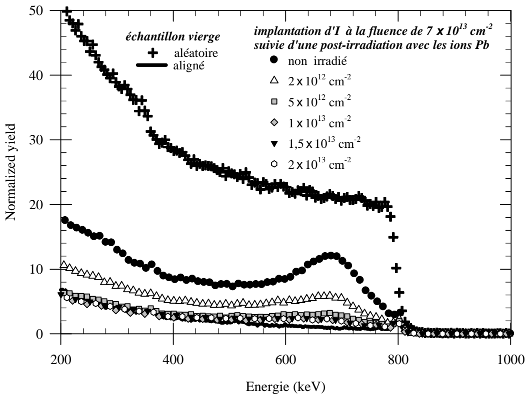
Figure 29 : Spectres RBS enregistrés en directions aléatoire et de canalisation sur des échantillons endommagés par l'implantation d'une fluence d'iode de 7 \times 10^{13} \text{ cm}^{-2} puis irradiés avec différentes fluences de Pb de 860 MeV.
