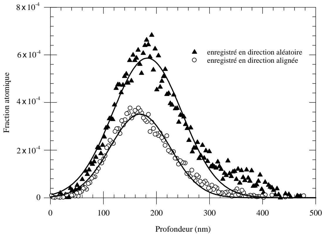
Figure 32 : Profils d'iode obtenus après implantation à la fluence de 9,6 \times 10^{14} \text{ cm}^{-2} à 600 \text{ °C} par l'analyse des spectres RBS enregistrés en direction aléatoire et de canalisation.
