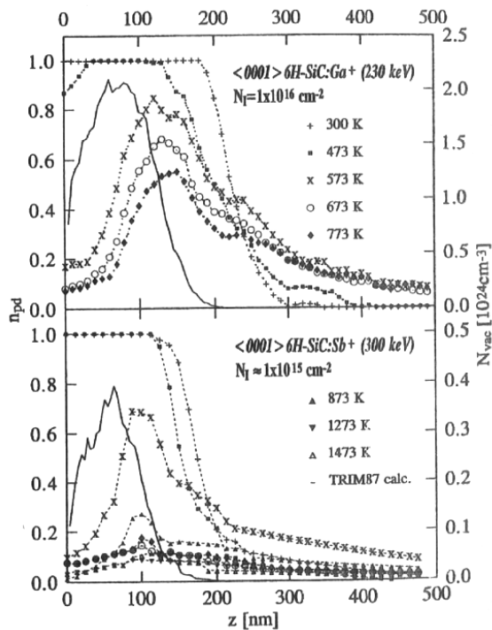
Figure 24 : Distribution en profondeur de la densité relative de défauts n_{pd} dans SiC implanté avec des ions \text{Ga}^+ et \text{Sb}^+ à différentes températures et distribution des lacunes produites dans les cascades primaires calculée par TRIM87 [C1-63].
