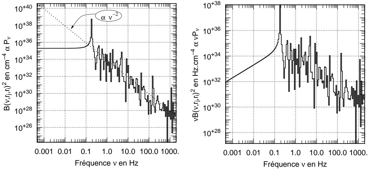
Fig. 53. Tracé de B^2 et vB^2 en fonction de la fréquence \nu : on constate l'existence d'un plateau à basse fréquence (bruit à bande limitée où "BLN"), d'un pic à \nu_{QPO} \simeq 0.41c_s/r_j puis d'une décroissance en \nu^{-2} à partir de la fréquence de coupure \nu_b \sim \nu_{QPO} . On a pris ici c_s = 4 \times 10^8 \text{ cm.s}^{-1} , r_i = 10^7 \text{ cm} et r_j = 10^9 \text{ cm} . On remarquera aussi la présence de nombreux pics secondaires liés aux oscillations des fonctions de Bessel.
