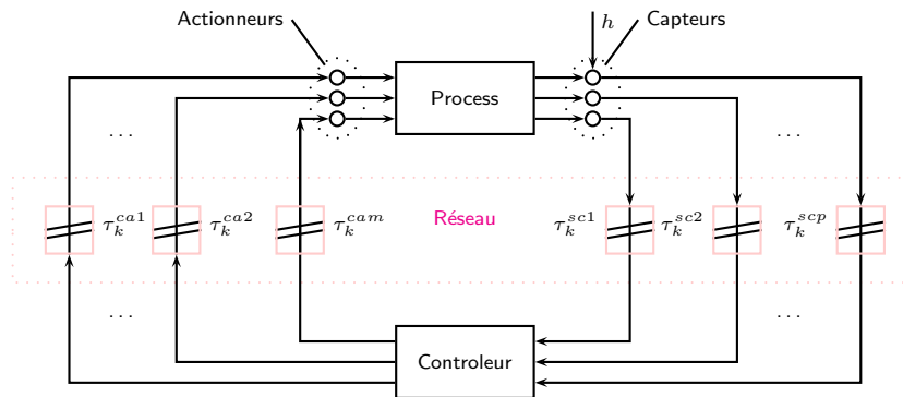
FIG. 1.7: Modèle d'asservissement distribué à multiples entrées et sorties (Nilson, 1998)
