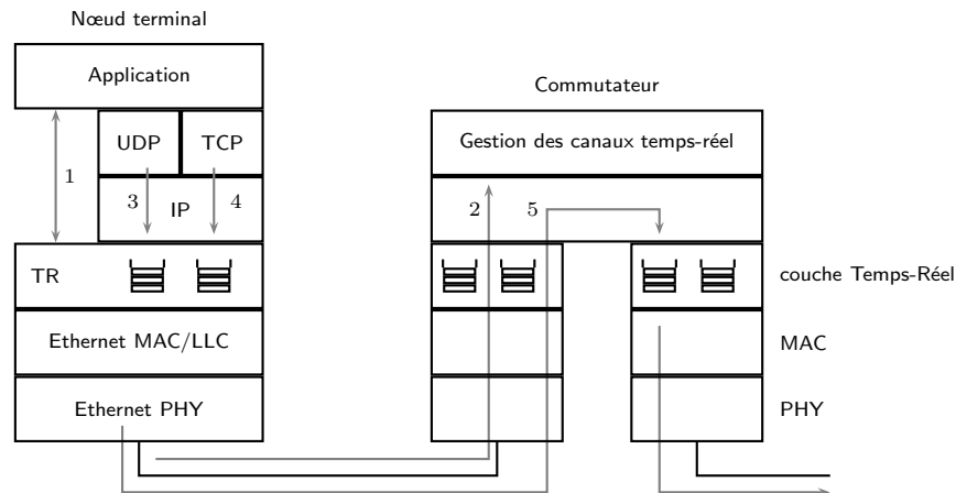
FIG. 2.5: La couche temps-réel
