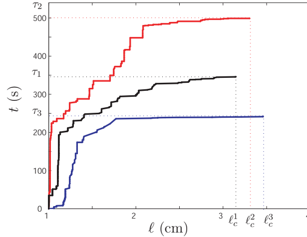
FIG. 2.3 – Temps courant t en fonction de la longueur de la fissure l pour trois expériences réalisées dans des conditions expérimentales identiques ( l_i = 1\text{cm} et F = 270\text{N} ).
