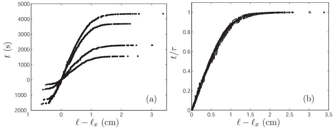
FIG. 4.18 – (a) temps en fonction de l - l_x avec un changement d'origine en temps et en longueur, (b) temps remis à l'échelle par le temps restant jusqu'à la rupture en fonction de l - l_x avec un changement d'origine en temps et en longueur, pour quatre expériences réalisées dans les mêmes conditions expérimentales ( l_i = 1.5\text{cm} , F = 900\text{N} ).
