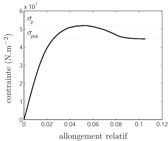
FIG. 3.4 – Contrainte nominale en fonction de l'allongement relatif pour un échantillon de polycarbonate ( 24 \times 21\text{cm}^2 ) initialement intact en traction à vitesse constante ( 46.25\mu\text{m.s}^{-1} ).
