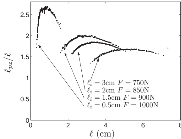
FIG. 4.13 – Rapport l_{pz}/l pour quatre expériences réalisées dans des conditions expérimentales différentes en fonction de la longueur de la fissure.
