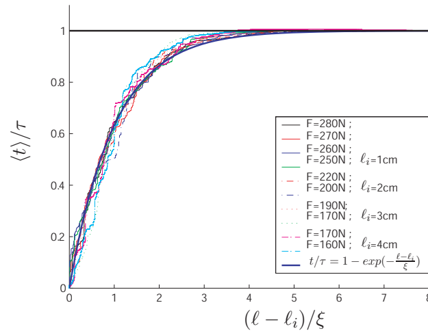
FIG. 2.4 – Temps moyen \langle t \rangle pour que la fissure atteigne une longueur l en fonction de (l - l_i) / \xi . La moyenne est effectuée sur dix à vingt expériences réalisées dans des conditions expérimentales identiques. La courbe continue représente l'ajustement des données par t/\tau = 1 - e^{-\frac{l-l_i}{\xi}} avec \xi comme unique paramètre libre.
