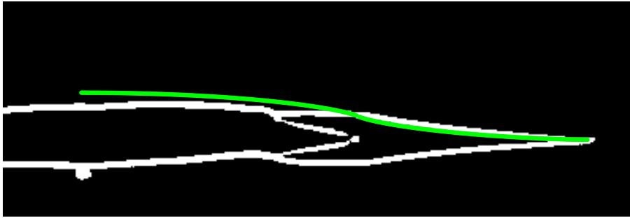
FIG. 4.16 – Image traitée illustrant la fissure et sa zone plastique lors d'une expérience de fluage ( \ell_i = 1.5\text{cm} et F = 900\text{N} ). La courbe en vert/gris est la prédiction théorique de l'ouverture de la fissure et de la zone plastique à partir de l'expression théorique de l'équation 4.4.
