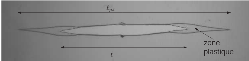
FIG. 4.8 – Image d'une fissure dans un film de polycarbonate avec ses zones plastiques à chaque extrémité; l est la longueur de la fissure et l_{pz} la longueur d'une extrémité d'une zone plastique à l'autre.
