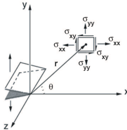
FIG. 1.4 – Base de projection du tenseur des contraintes dans le voisinage de la pointe d'une fissure.
