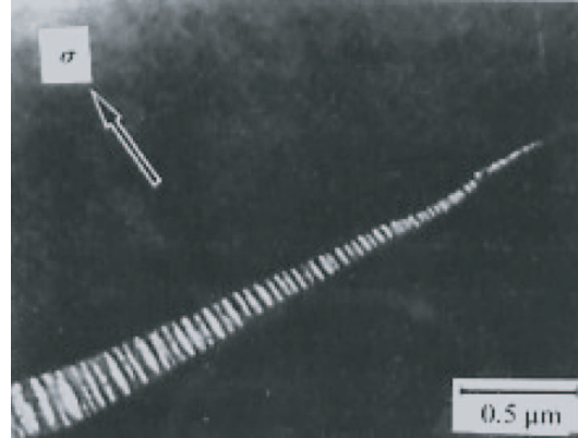
FIG. 4.14 – Zone de craquelage à la pointe d'une fissure dans un échantillon de PolyStyrène [85].
