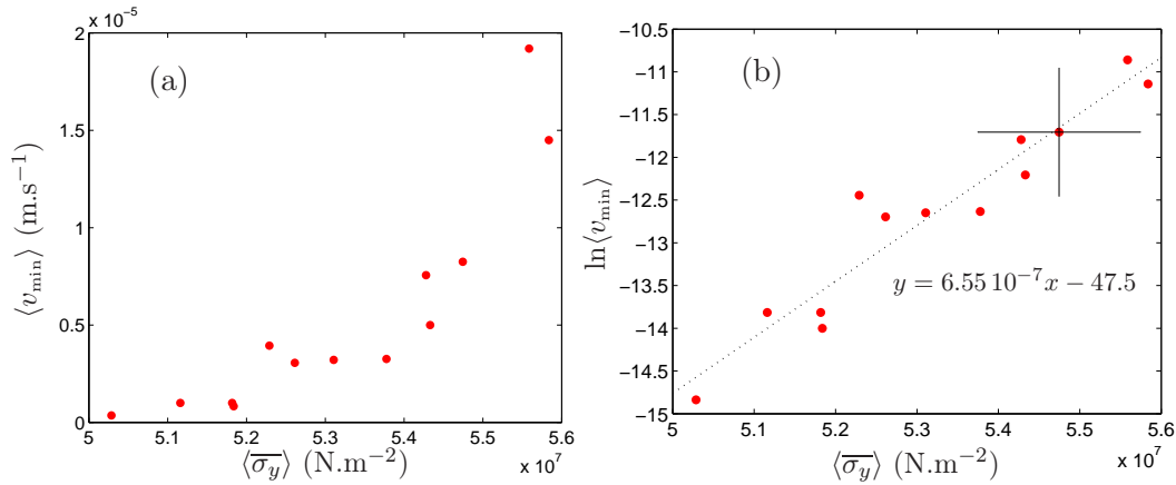
FIG. 4.24 – (a) Vitesse minimale \langle v_{\min} \rangle et (b) son logarithme en fonction de la contrainte plastique moyenne \langle \overline{\sigma}_y \rangle . Chacun des points est le résultat du calcul de la moyenne statistique de v_{\min} et de \overline{\sigma}_y sur une série d'expériences à \ell_i et \sigma donnés. Les conditions expérimentales sont variées ( \ell_i = 1.5, 2, 3\text{cm} et 2.9 < \sigma < 3.8 \cdot 10^7 \text{N.m}^{-2} ). Pour donner une idée de la dispersion des données pour \ell_i et \sigma fixés, on indique des barres d'erreurs typiques sur un point de la figure (b).
