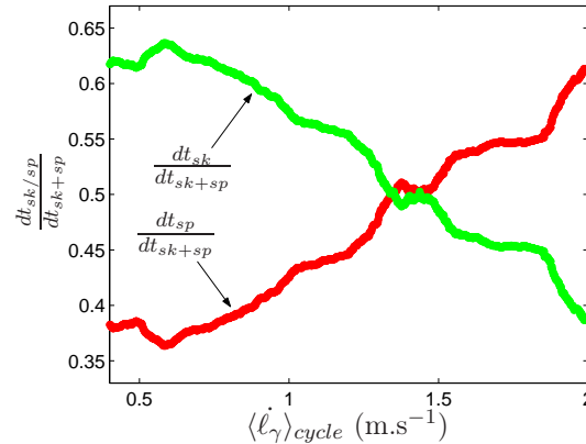
FIG. 5.17 – Rapport de la durée des phases de stick (gris clair/vert) et de slip (gris foncé/rouge) sur la durée du stick-slip en fonction de la vitesse moyenne de pelage pour une expérience de stick-slip spontanée réalisée avec m = 245\text{g} .
