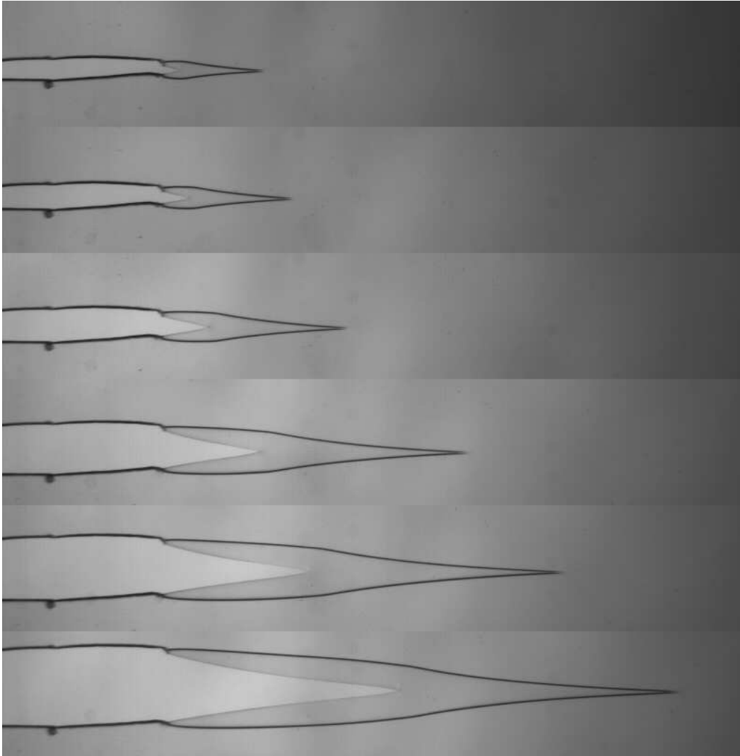
FIG. 4.9 – Série d'images illustrant la croissance d'une fissure lors d'une expérience de fluage ( l_i = 1.5\text{cm} et F = 900\text{N} ). Les images ne sont pas espacées régulièrement en temps.
