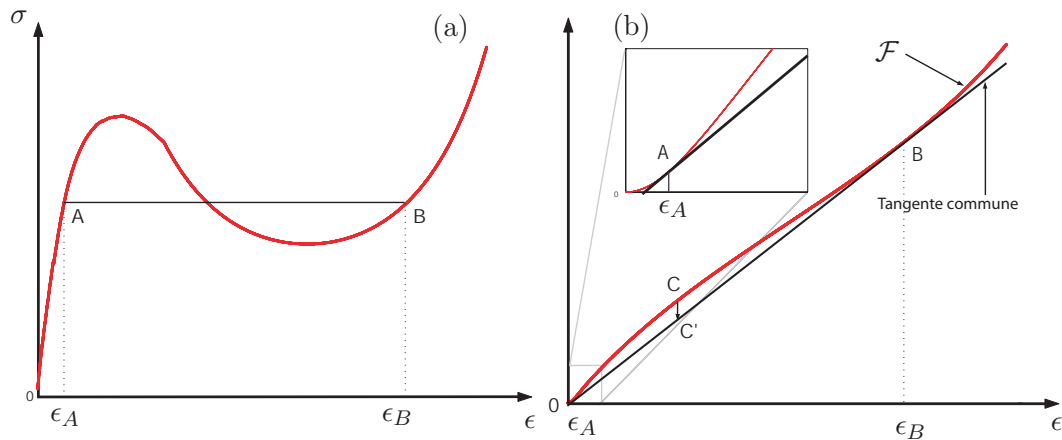
FIG. 3.10 – (a) Courbe schématique de la contrainte \sigma(\epsilon) en fonction de la déformation relative pour un polymère amorphe; (b) énergie libre \mathcal{F}(\epsilon) obtenue par intégration de la contrainte \sigma(\epsilon) représentée en (a).
