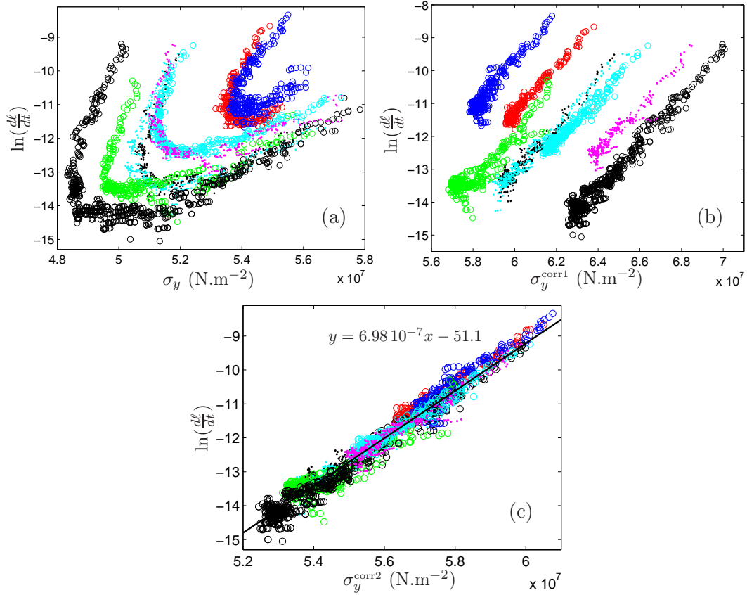
FIG. 4.27 – Logarithme de la vitesse de croissance de la fissure en fonction, (a) de la contrainte de Dugdale-Barenblatt, (b) de cette même contrainte corrigée \sigma_y^{\text{corr1}} selon l'équation 4.22 et (c) de cette même contrainte corrigée \sigma_y^{\text{corr2}} selon l'équation 4.24, au cours de huit expériences réalisées dans des conditions expérimentales variées ( \ell_i = 1.5, 2, 3\text{cm} et 2.9 < \sigma < 3.8 \cdot 10^7 \text{N.m}^{-2} ). Sur la figure (c), la droite noire est le résultat de l'ajustement linéaire de l'ensemble des données.
