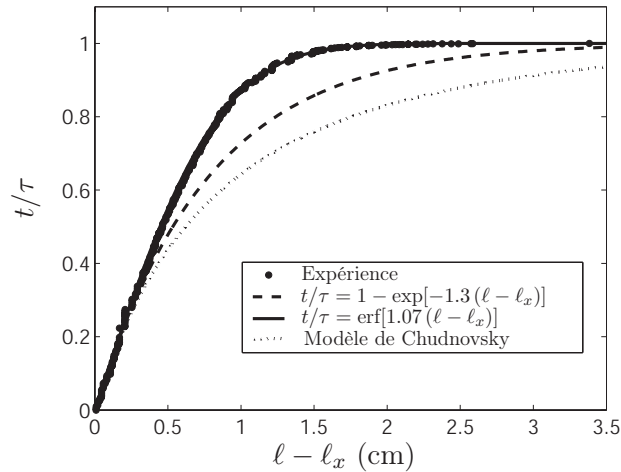
FIG. 4.19 – Temps remis à l’échelle par le temps restant jusqu’à la rupture en fonction de \ell - \ell_x pour une expérience à contrainte imposée ( \ell_i = 1.5\text{cm} , F = 900\text{N} ) et ses ajustements par le modèle de Chudnovsky, le modèle de croissance thermiquement activée et une fonction erreur.
