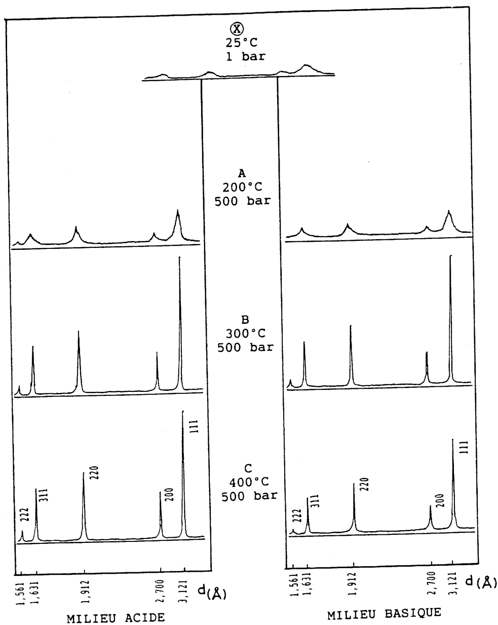
Fig.38 : Diffractogrammes des poudres de dioxyde de cérium élaborées à différentes températures par recristallisation solvothermale en milieu acide ( \text{pH}\approx 1 ) ou basique ( \text{pH}\approx 9 ) à partir d'un "sol" de dioxyde de cérium à 250 g/l.
