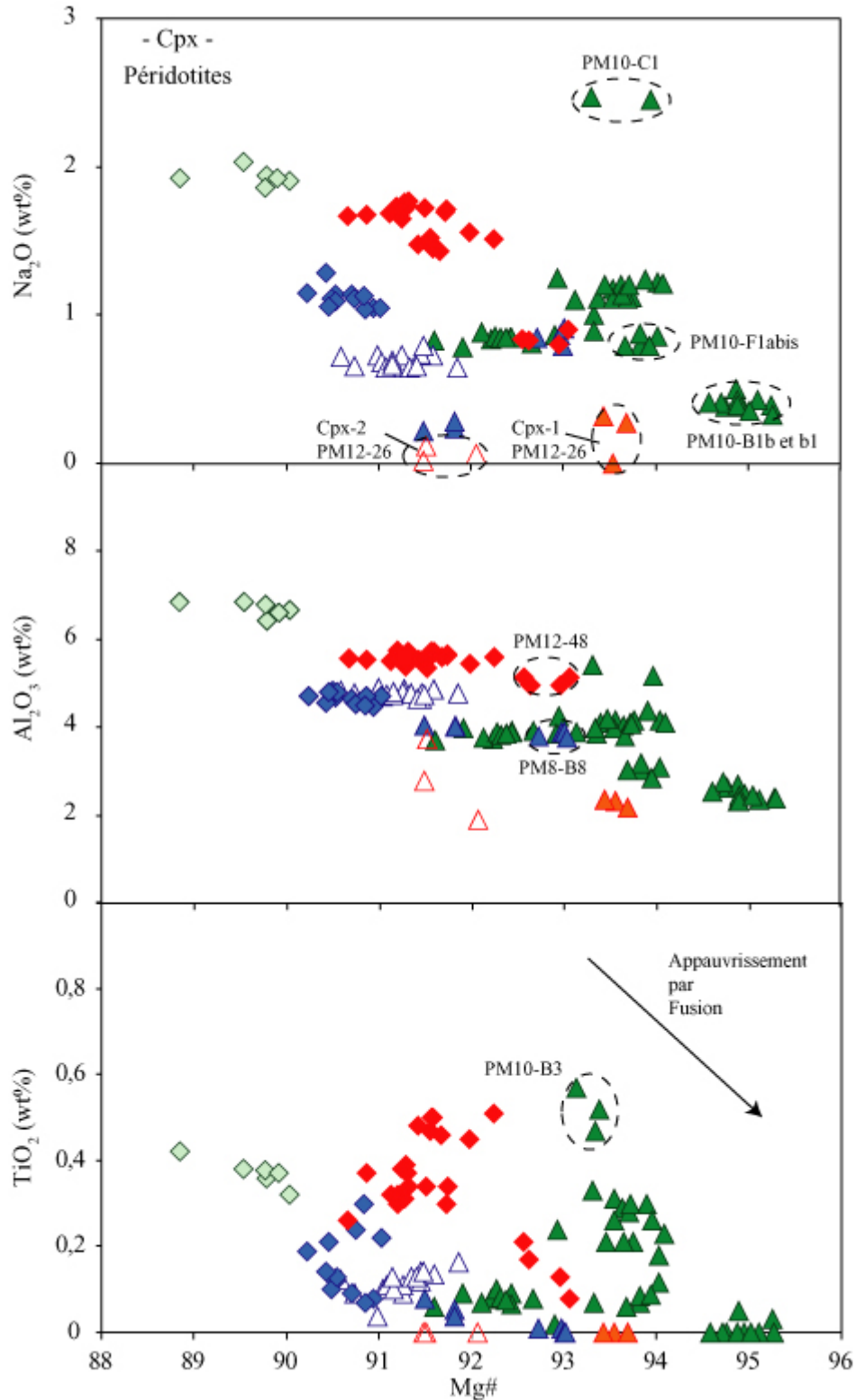
Figure IV-15 : Diagrammes \text{Na}_2\text{O} , \text{Al}_2\text{O}_3 , \text{TiO}_2 vs \text{Mg}\# [(\text{Mg}/(\text{Mg}+\text{FeTot})) \times 100] dans les clinopyroxènes des péridotites. Rappel des légendes : les triangles correspondent aux harzburgites et les losanges, aux lherzolites. En bleu sont représentés les échantillons de PM8, en vert ceux de PM10 et en rouge-orangé, ceux de PM12. La flèche noire marque le trend d'appauvrissement contrôlé par la fusion partielle (Norman, 1998).
