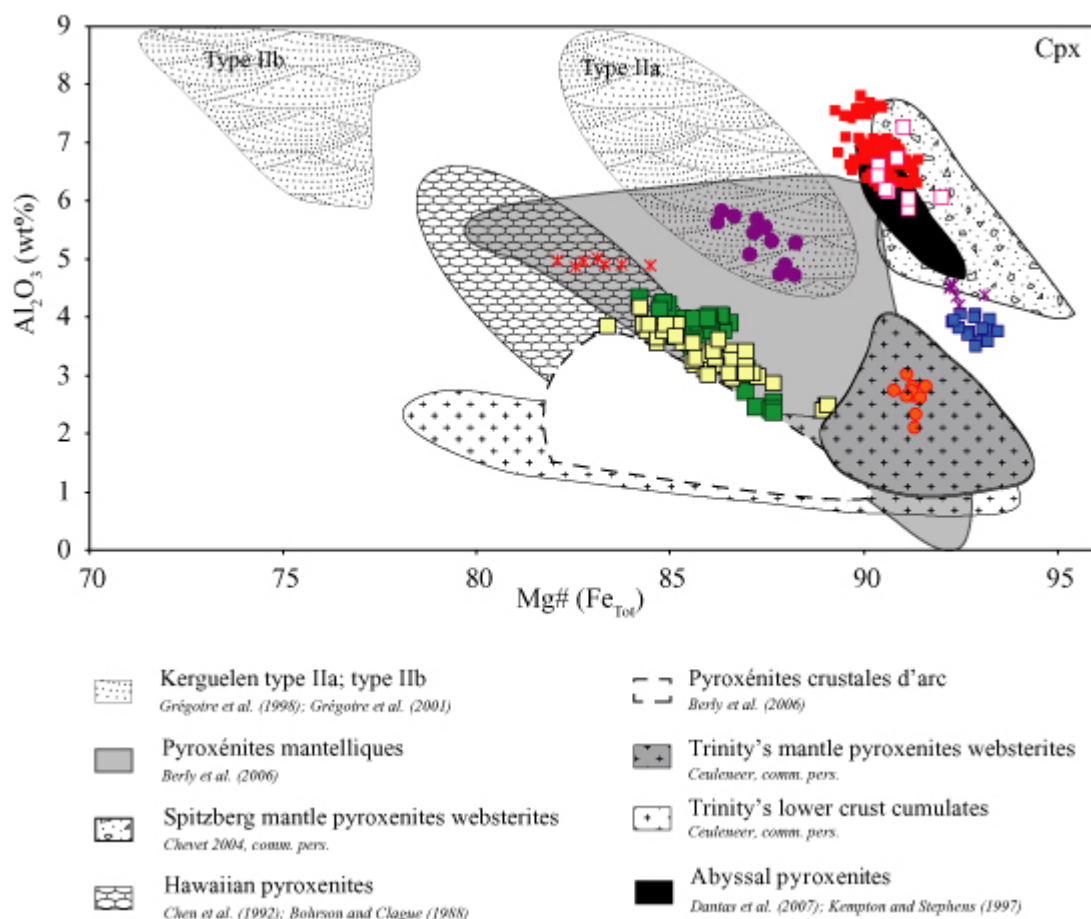
Figure IV-25 : Diagramme Al_2O_3 vs Mg\# des clinopyroxènes des pyroxénites de Patagonie, en comparaison aux pyroxénites provenant de plusieurs sites et de plusieurs contextes géodynamiques (abyssales, ophiolites, arc et intraplaque océanique) à travers le monde. Carré (webstérite) en Jaune de PM6 ; en bleu de PM8 ; en vert de PM10, en rouge de PM12 et en blanc de PM24. Les croix violettes et rouges correspondent aux clinopyroxénites de Cerro Clark (PM24) à spinelle et sans spinelle, respectivement. Les ronds (orthopyroxénite) sont orange pour Cerro de los Chenques (PM12) et violet pour Pali Aike (PM18).
