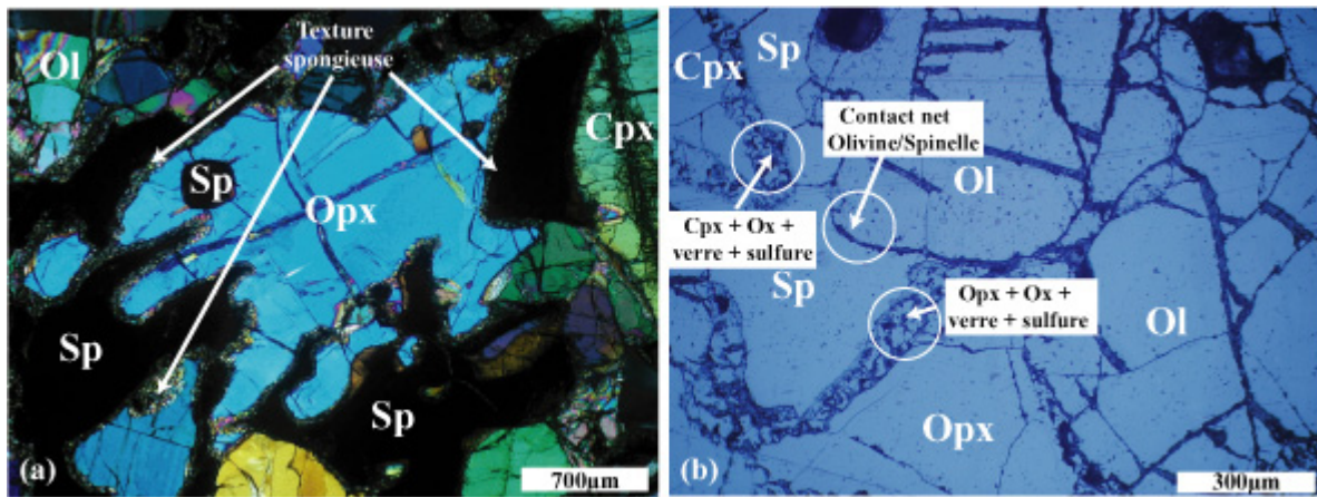
Figure V-3 : Microphotographies dans la lherzolite à spinelle PM24-09. Le contact entre les spinelles interstitiels et les pyroxènes, est souligné par une accumulation de minéraux (a et b) de petites tailles (<10µm). Ces minéraux sont des opaques, des sulfures, et des pyroxènes qui sont piégés dans du verre.
