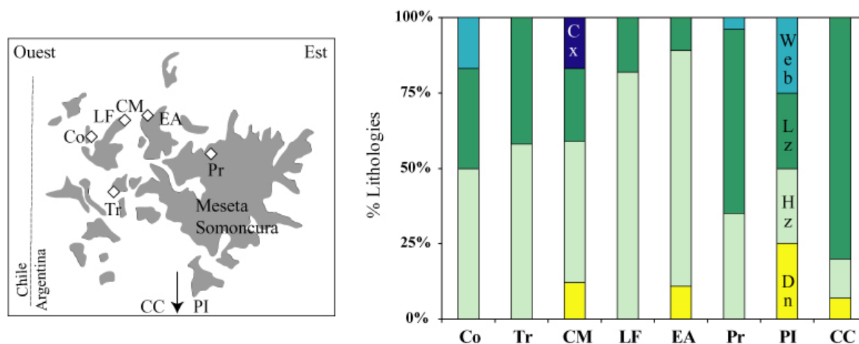
Figure IV-1 : Synthèse des différentes lithologies d'enclaves mantelliques étudiées dans les localités de la Meseta de Somoncura (carte de gauche) et de Canquel (CC et PI, Figure II-9, 13), dans les travaux de Ntaflos et al. (2001, 2002), Mallmann (2004), Rivalenti et al. (2004) et Bjerg et al. (2000a, b, 2005). Dn : Dunite ; Hz : Harzburgite ; Lz : Lherzolite ; Web : Websterite ; Cx : Clinopyroxénite.
