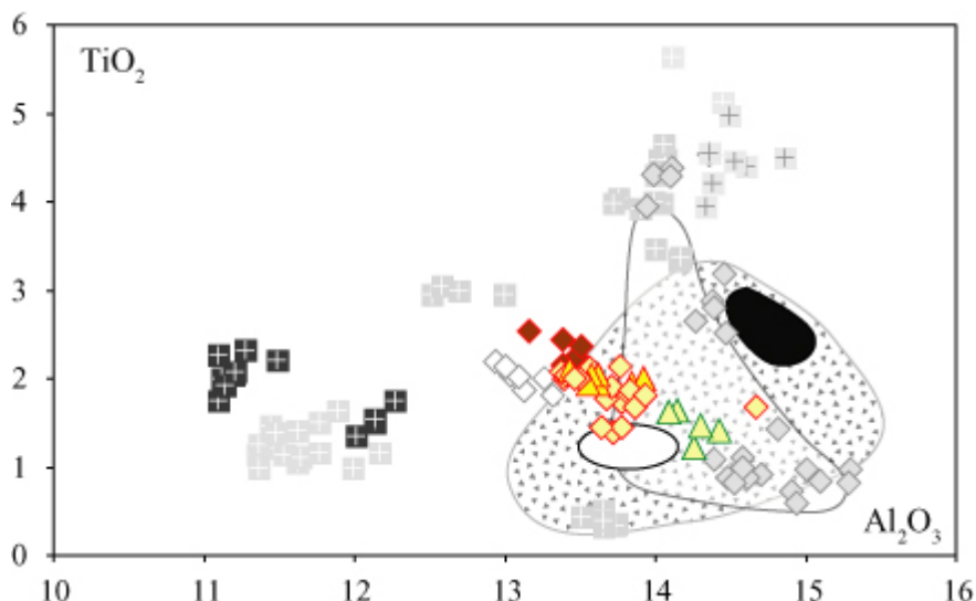
Figure VI-19: Diagrammes binaires \text{TiO}_2 vs \text{Al}_2\text{O}_3 et \text{Cr}_2\text{O}_3 , \text{Na}_2\text{O} et \text{K}_2\text{O} vs \text{Mg\#} [(\text{Mg}/(\text{Mg}+\text{FeTot})) \times 100] des amphiboles des péridotites de Pali Aike. Les symboles en gris représentent les compositions des amphiboles des lherzolites (triangles) et des wehrlites (croix + carrés) de Gobernador Gregores (voir Chapitre V). Le champ noir plein correspond aux amphiboles d'une lherzolite à spinelle contenant des amphiboles disséminées de Cerro Clark (PM24, Comm. Pers. Ntaflos) et le champ noir vide illustre les amphiboles d'une lherzolite à spinelle de Cerro el Mojon, de la zone Nord Patagonienne (CM, PM4-C2, Mallmann, 1998).
