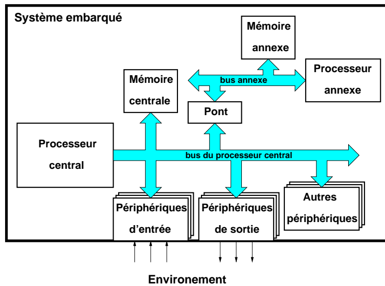
FIG. 1.3 – Architecture embarquée de deuxième génération
