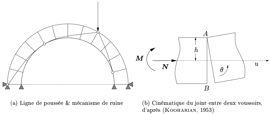
FIGURE 2.1 – Voûte &amp; analyse limite
