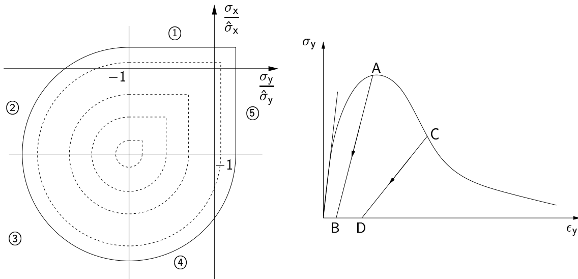
(a) Surface limite d'écoulement
