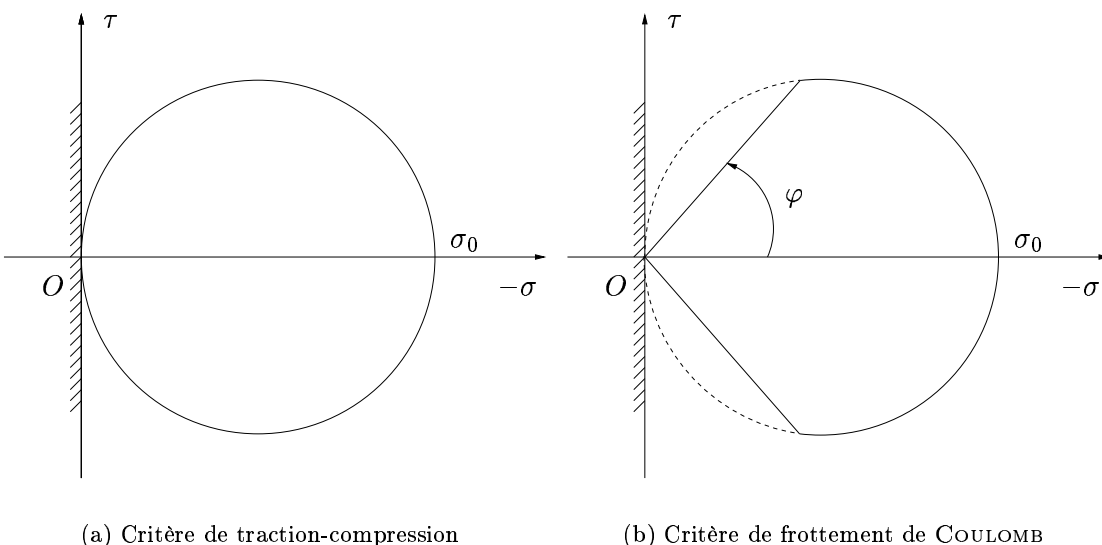
FIGURE 2.3 – Critère de rupture des maçonneries, d'après (DELBECQ, 1982)
