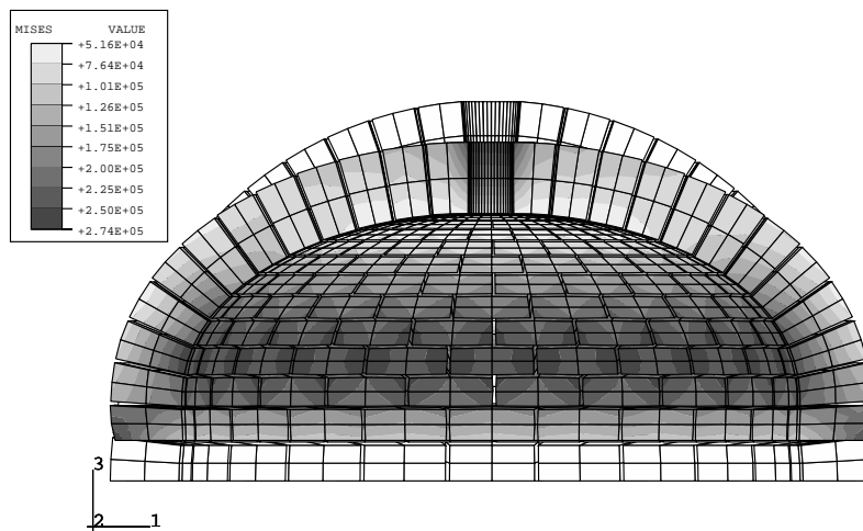
(b) Contraintes de VON MISES dans un plan de coupe ( \times 2.5 \cdot 10^6 )
