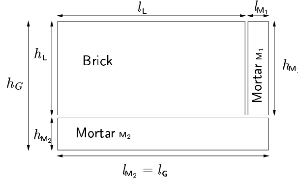
FIGURE 4.7 – Volume élémentaire représentatif
