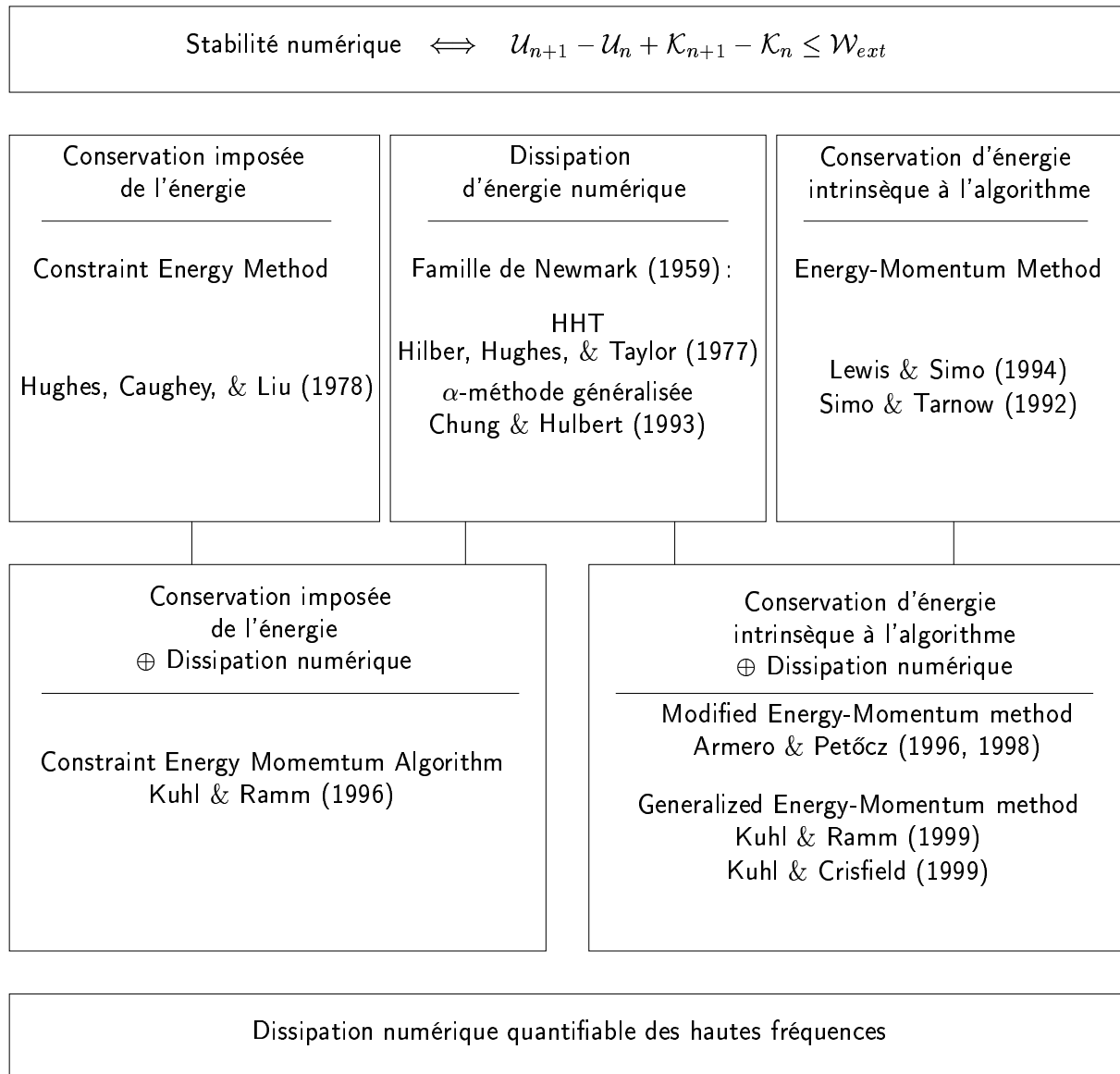
FIGURE 6.3 – Revue des schémas d'intégration qui satisfont le critère énergétique de stabilité, inspirée de KUHL & CRISFIELD (1999)
