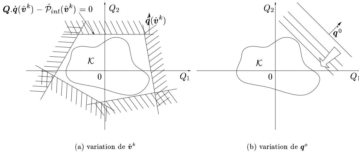
FIGURE A.1 – Approche de \mathcal{K} par l'extérieur
