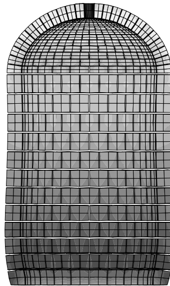
(d) Contraintes de VON MISES dans un plan de coupe
