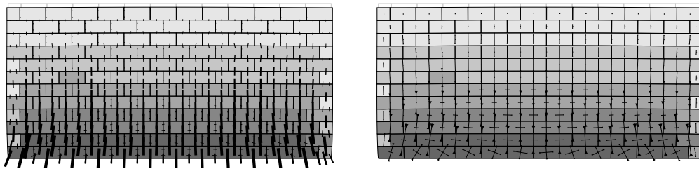
(d) Réactions et contraintes pour h = 0.1 \cdot 10^{-01} s
