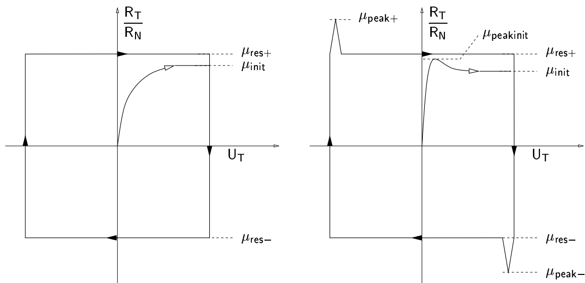
(a) Pression normale faible, vitesse faible
