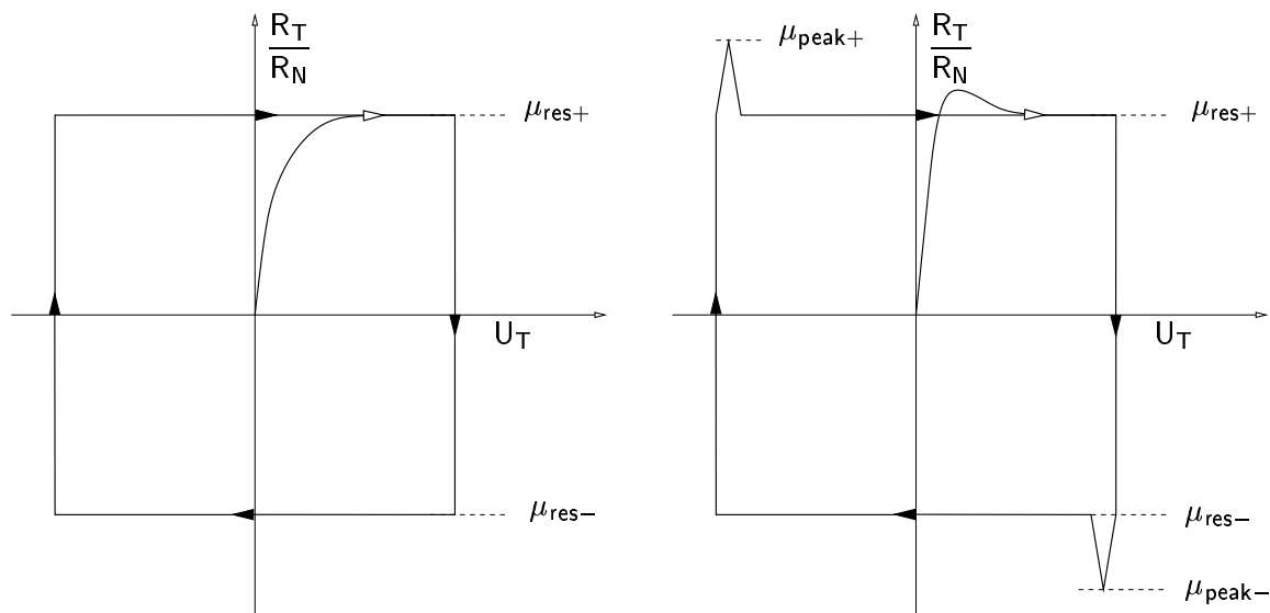
(c) Pression normale élevée, vitesse faible
