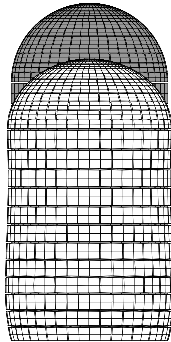
(b) Déformée sous gravité
