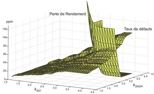
FIG. 4.14 – Le Taux de défauts et la Perte de rendement vs. les limites de test.
