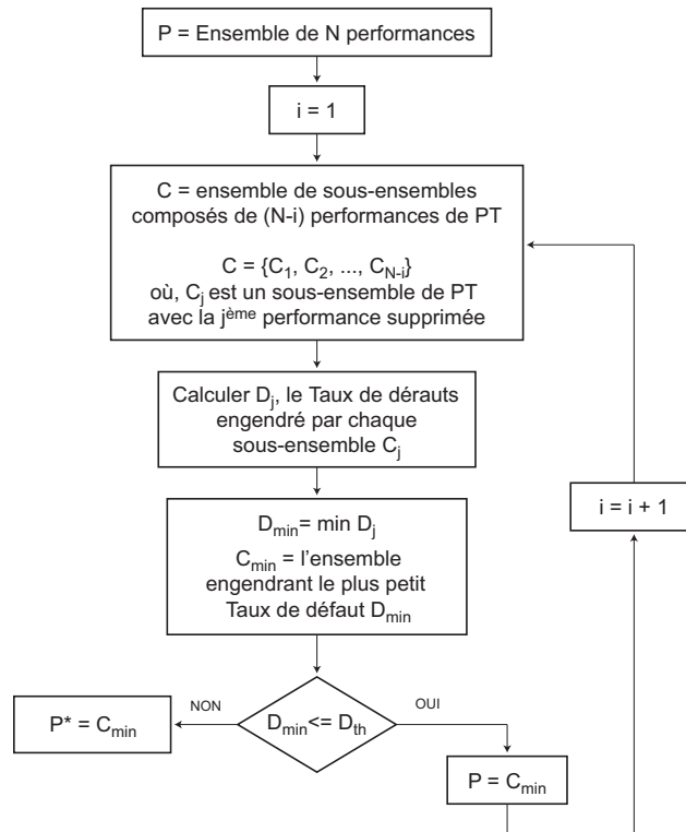
FIG. 6.1 – Algorithme de la méthode de réduction du nombre des performances.
