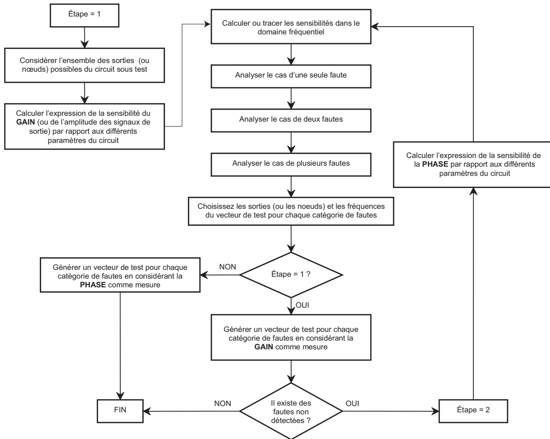
FIG. 3.24 – Algorithme de génération de vecteurs de test structurel en considérant l’analyse de sensibilité.
