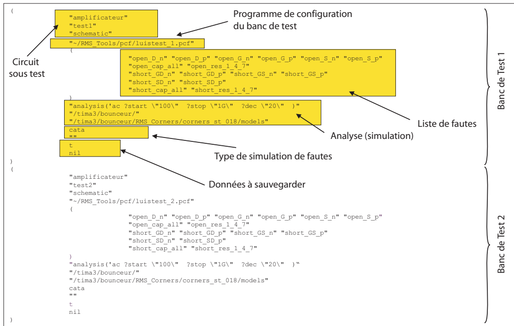
FIG. 5.17 – Exemple d’un Programme de Configuration à Plusieurs Bancs de Test pour l’amplificateur (banc de test 1 et 2).
