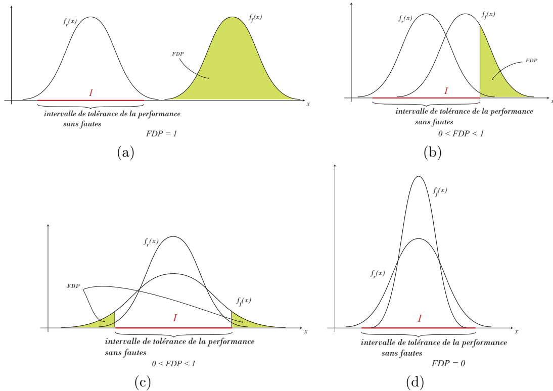
FIG. 3.9 – Les différentes valeurs de la Probabilité de Détection de Fautes FDP .
