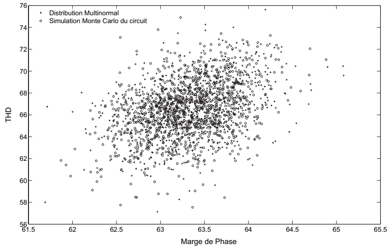
FIG. 4.10 – Distribution de 1000 circuits générés par la simulation Monte Carlo du circuit et de la loi multinormale.
