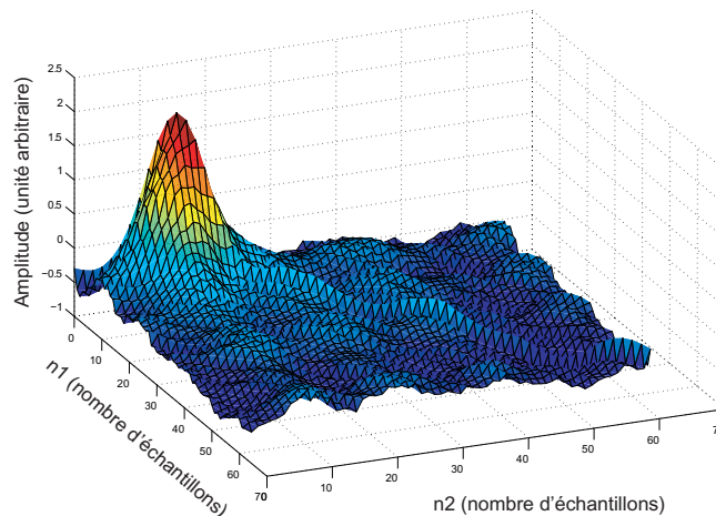
FIG. 6.16 – Le 2 ème noyau de Volterra d'un MEMS.
