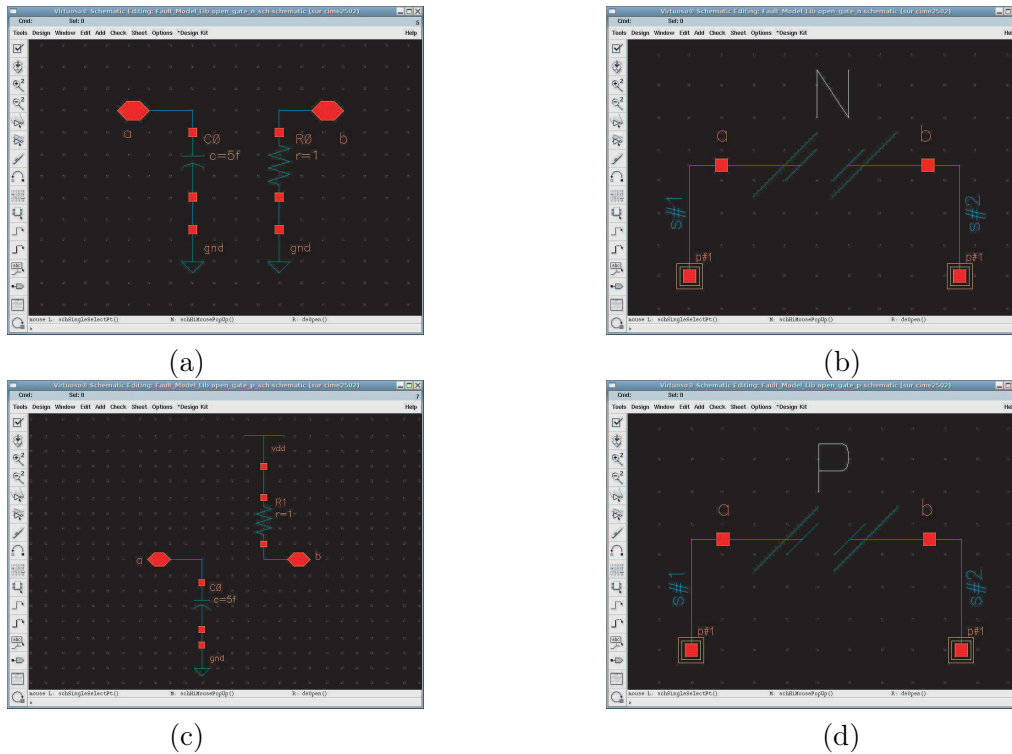
FIG. 5.20 – Exemple de modèles de fautes : (a) Circuit-ouvert à la grille d’un NMOS (forme Schématique), (b) Circuit-ouvert à la grille d’un NMOS (forme FMDL), (c) Circuit-ouvert à la grille d’un PMOS (forme Schématique) et (d) Circuit-ouvert à la grille d’un PMOS (forme FMDL).
