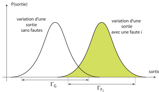
FIG. 3.11 – Les valeurs d'un critère de test d'un circuit sans fautes et avec une faute.
