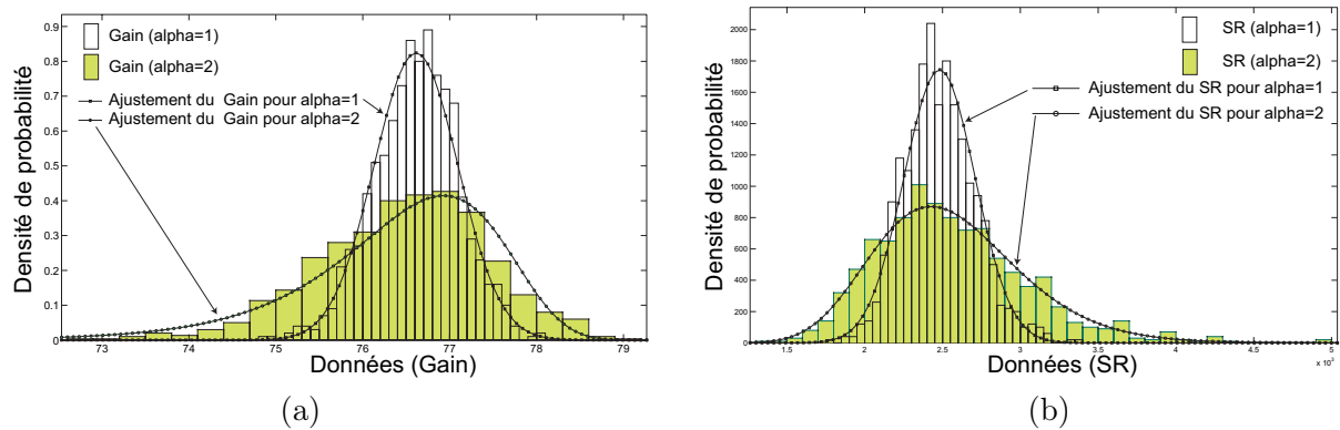
FIG. 4.8 – La distribution (a) du Gain et (b) du SR de l'amplificateur pour \alpha = 1 qui représente le cas normal et \alpha = 2 qui représente le cas d'un élargissement.
