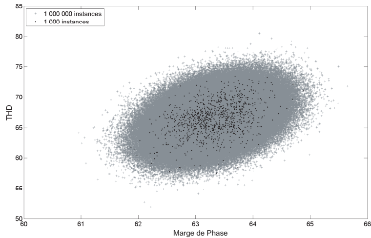
FIG. 4.11 – Génération de 1000 et 1 million de circuits ayant une distribution multinormale.
