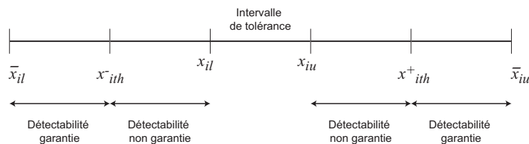
FIG. 3.27 – Intervalles de tolérance, de détectabilité et acceptables d'un paramètre du circuit.
