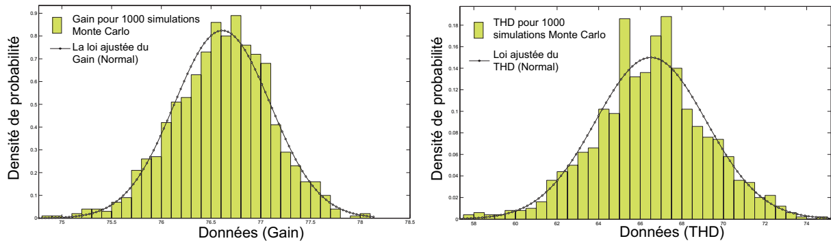
FIG. 4.3 – La distribution (a) du Gain et (b) du THD de l’amplificateur.
