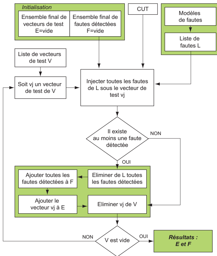
FIG. 2.5 – Principe de base de la génération automatique de vecteurs de test (ATPG).
