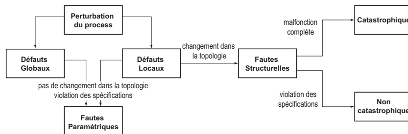
FIG. 2.2 – Classification des fautes analogiques.
