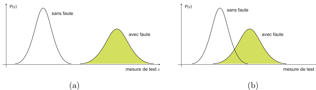
FIG. 2.12 – Faute (a) totalement détectée et (b) partiellement détectée.
