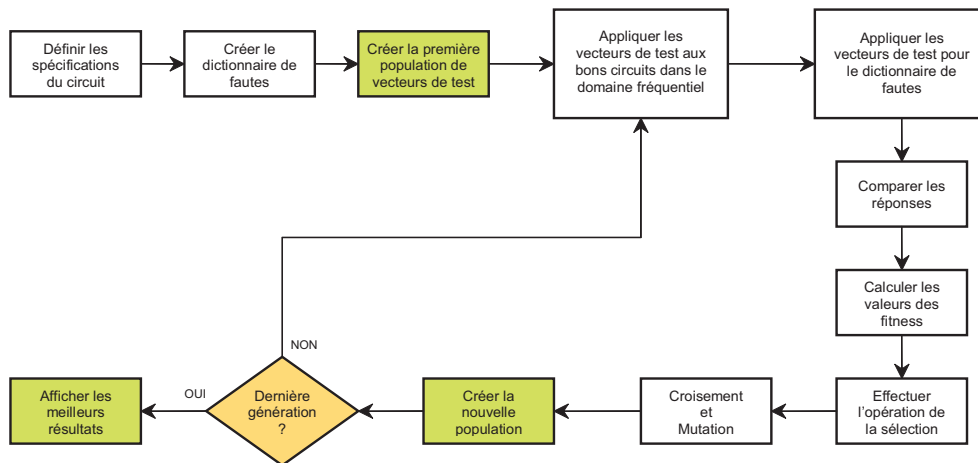
FIG. 3.25 – Génération de vecteurs de test par les Algorithmes Génétiques.
