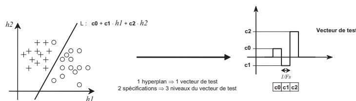
FIG. 3.15 – Vecteur de test dérivé des hyperplans.
