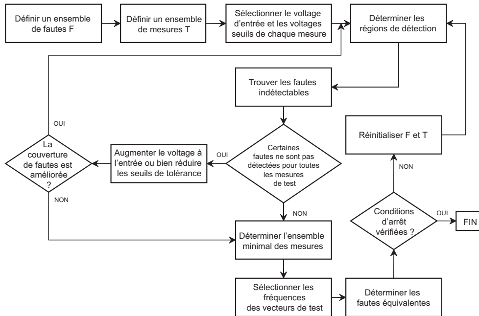
FIG. 3.21 – Génération de vecteurs de test par minimisation de l'ensemble des mesures de test et de fréquences de détection de fautes.
