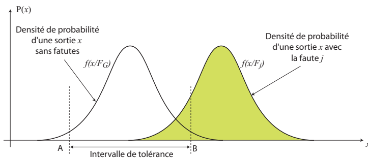
FIG. 3.26 – Densités de probabilité d'un circuit sans faute et d'un autre avec faute.
