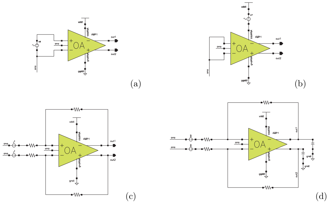
FIG. 5.19 – Exemple des configurations des bancs de test (a) : n°1, (b) : n°4, (c) : n°6 et (d) : n°7 de l’amplificateur.
