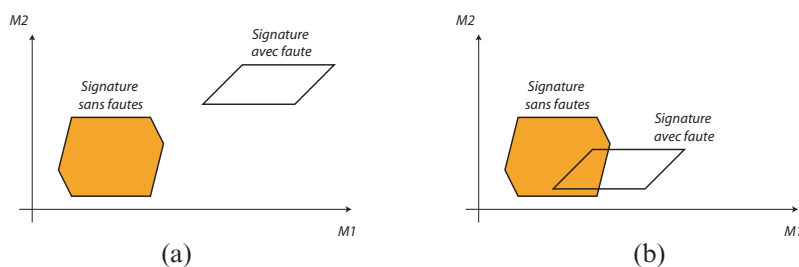
FIG. 3.19 – Signature d'un circuit sans fautes et d'un circuit avec (a) fautes détectées et (b) fautes non détectées.
