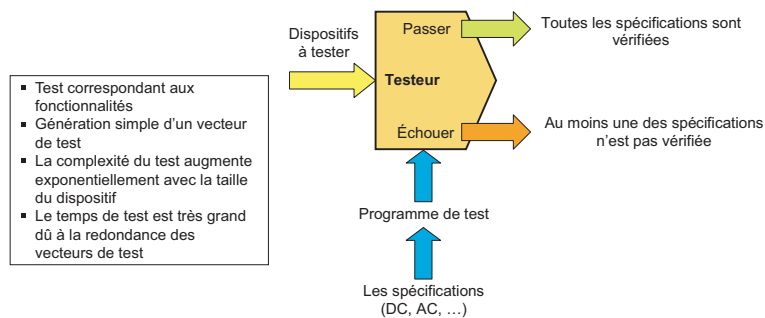
FIG. 2.9 – Principe d'un test fonctionnel [79].
