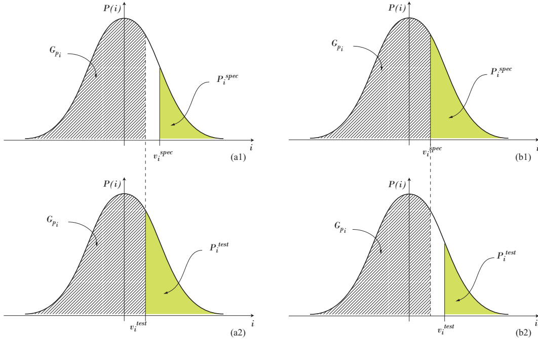
FIG. 2.14 – Probabilité de détection d'une faute (a1 et b1) et probabilité d'occurrence d'une faute (a2 et b2).
