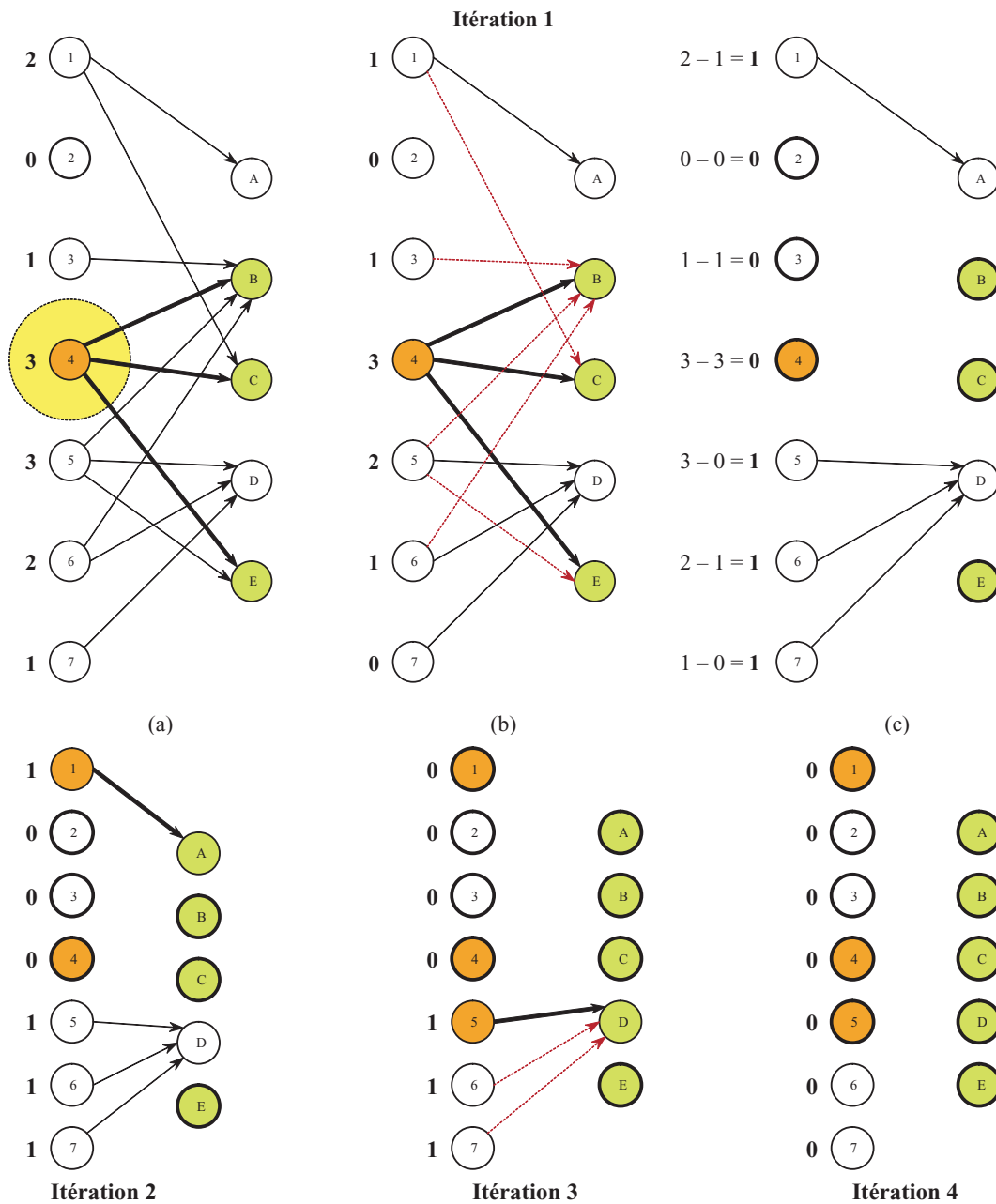
FIG. A.4 – Algorithme de résolution du problème de minimum de region de détection ou de diagnostic.
