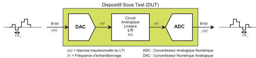
FIG. 3.14 – Structure d'un test numérique pour les circuits analogiques.
