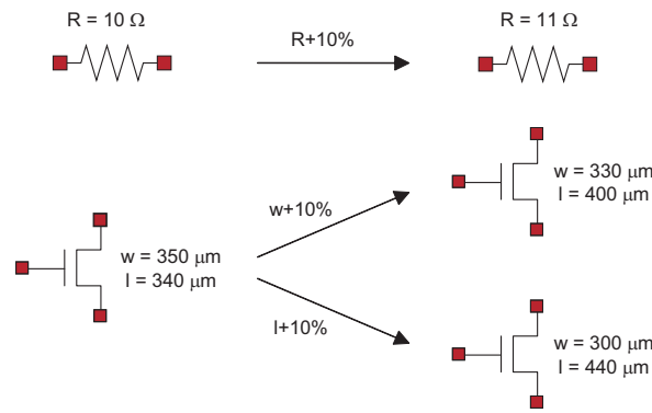
FIG. 5.3 – Modèles de fautes paramétriques locales.
