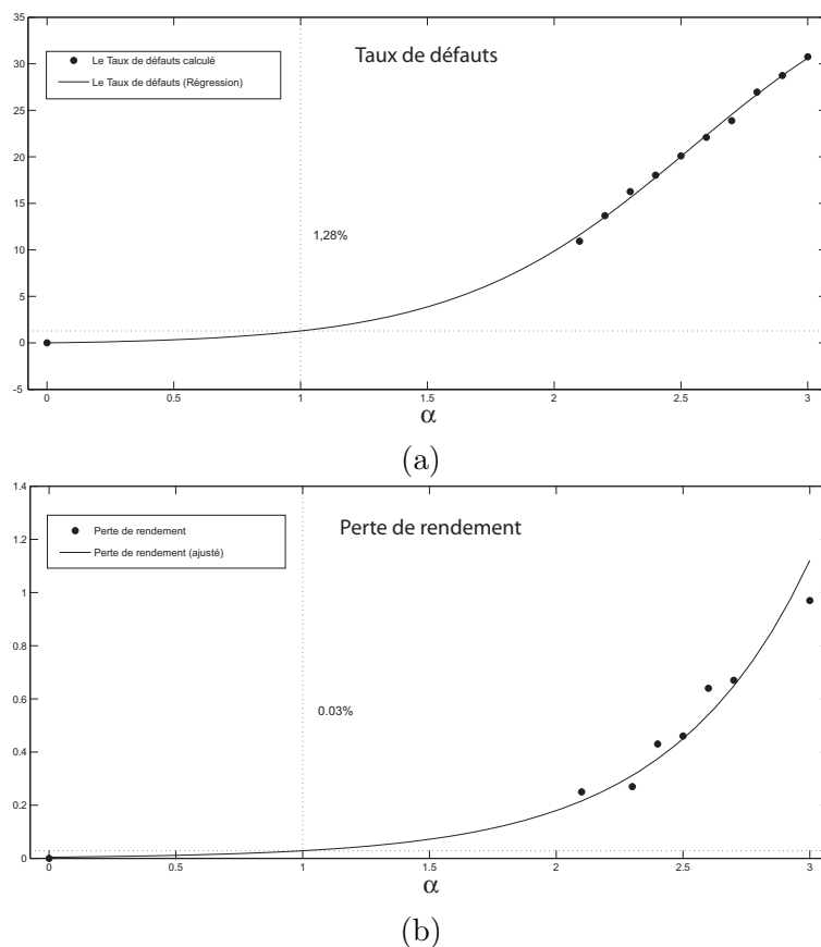
FIG. 4.4 – Calcul des métriques (a) Taux de défauts et (b) Perte de rendement par régression.
