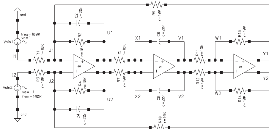
FIG. 6.3 – Filtre biquadratique.
