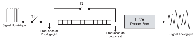
FIG. 6.9 – Génération sur-puce d'un signal analogique à partir d'un signal numérique.
