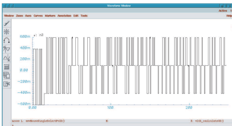
FIG. 6.15 – Vecteur de test multi-niveau ( Mu=4 , N=2 et Alpha=1 ).
