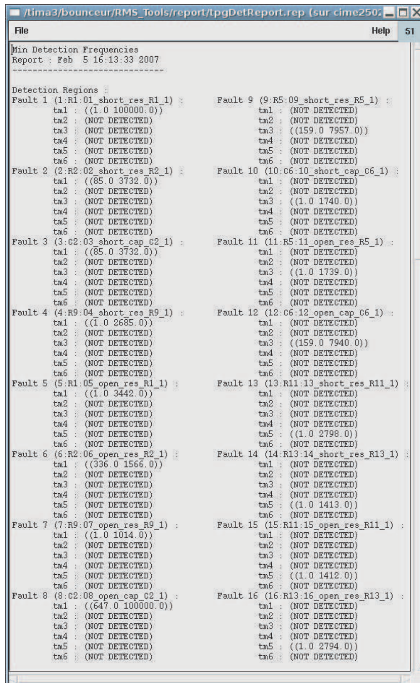
FIG. 6.6 – Intervalle fréquentiel de détection de chaque faute injectée dans le filtre.
