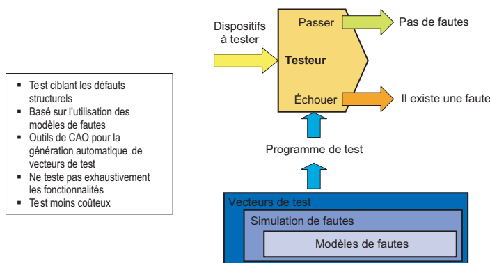
FIG. 2.10 – Principe d'un test structurel [79].
