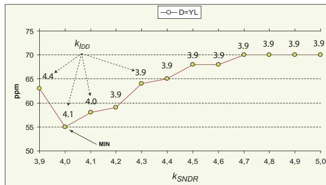
FIG. 4.15 – Points où le Taux de défauts est égal à la Perte de rendement vs. les limites de test.
