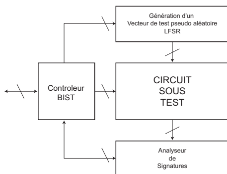
FIG. 2.7 – BIST typique pour un test pseudo aléatoire.
