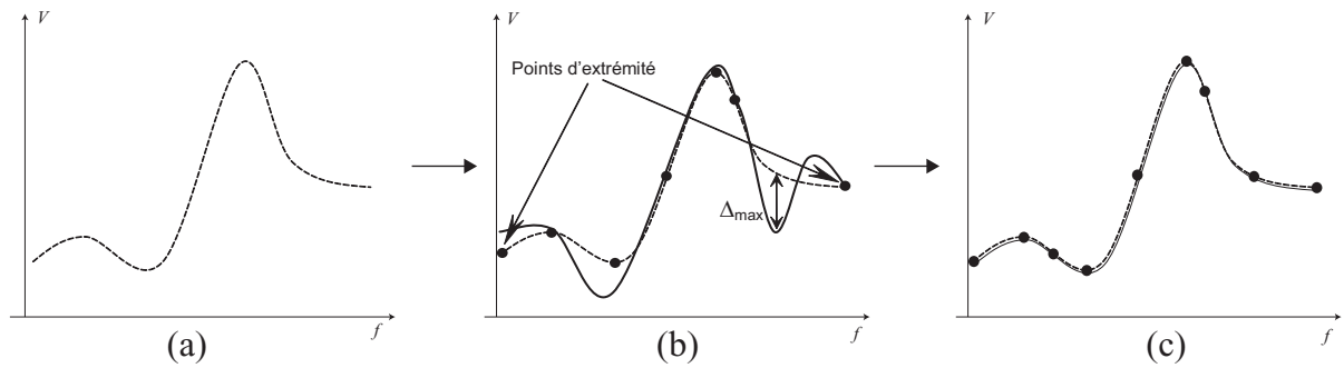
FIG. 3.22 – Reproduction de la fonction de transfert par interpolation.
