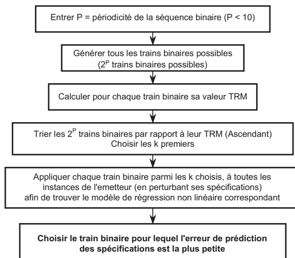
FIG. 3.28 – Génération d'un vecteur de test pour le test alternatif d'un émetteur RF.
