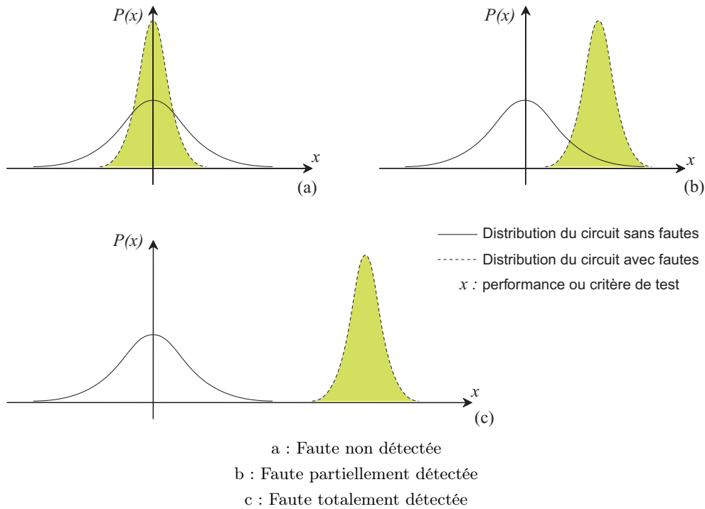
FIG. 3.8 – Performance d'un circuit sans faute et avec faute.
