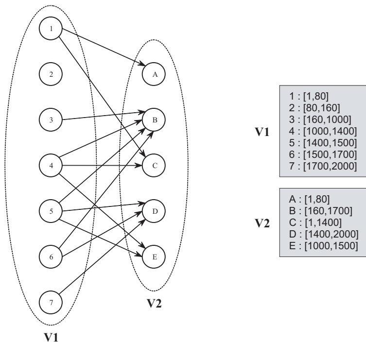
FIG. A.3 – Graphe bipartie du problème de minimum de region de détection ou de diagnostic.
