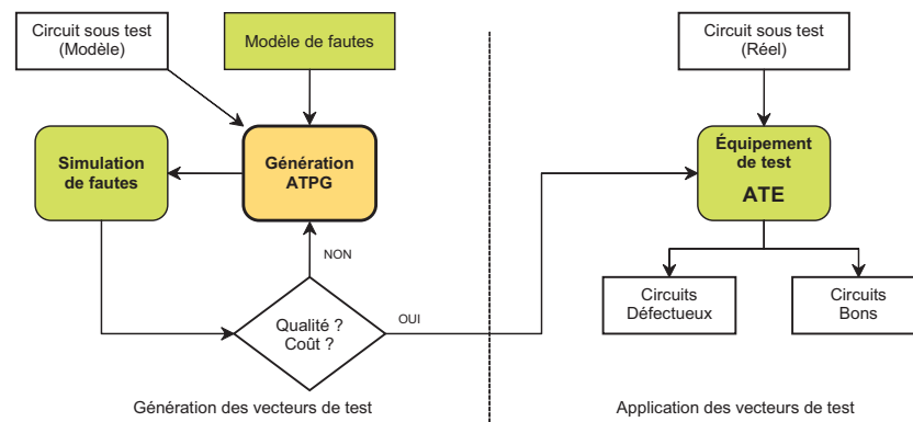
FIG. 2.4 – Génération et application des vecteurs de test [63].
