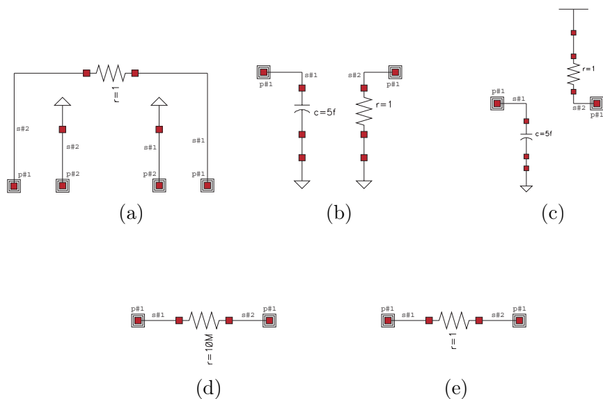
FIG. 5.2 – Modèles de fautes catastrophiques conçus sous Cadence (Virtuoso).
