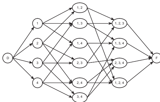
FIG. 3.17 – Graphe pour ordonner quatre performances.
