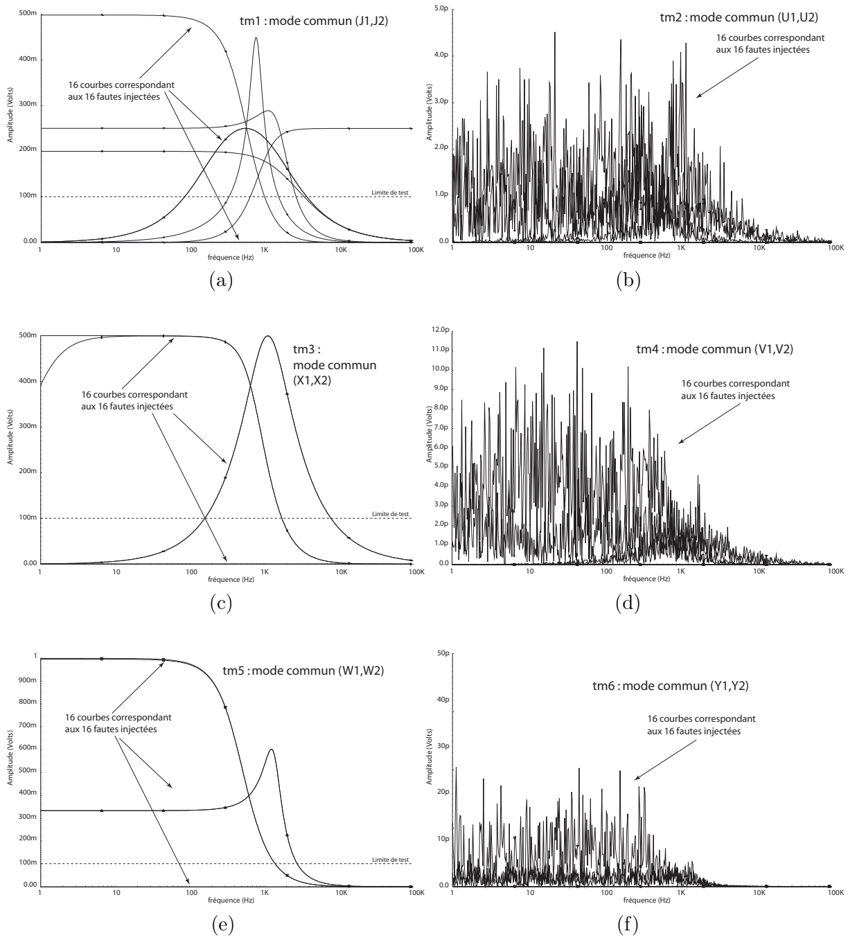
FIG. 6.5 – Les modes communs sous les effets des fautes : (a) tm1, (b) tm2, (c) tm3, (d) tm4, (e) tm5 et (f) tm6.
