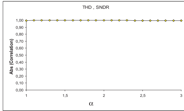
FIG. 4.7 – Corrélation absolue entre la THD et le critère de test SNDR en fonction du rapport d'augmentation de l'écart-type \alpha .
