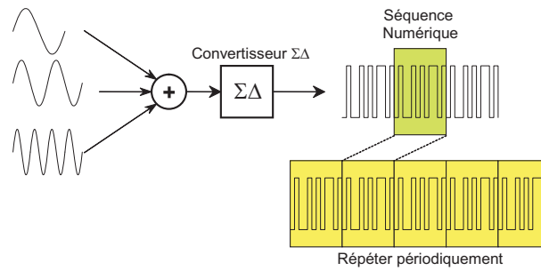
FIG. 6.10 – Génération d’un vecteur de test numérique d’une bonne qualité.
