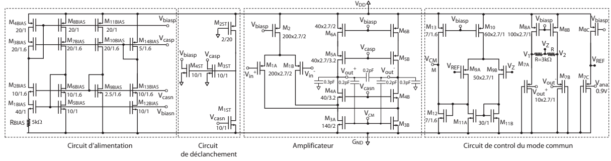
FIG. 4.2 – Amplificateur opérationnel complètement différentiel. Les dimensions de chaque transistor W/L sont de multiples de la taille unité de transistor ( W_{UNIT} = 0.28\mu\text{m} et L_{UNIT} = 0.18\mu\text{m} ).
