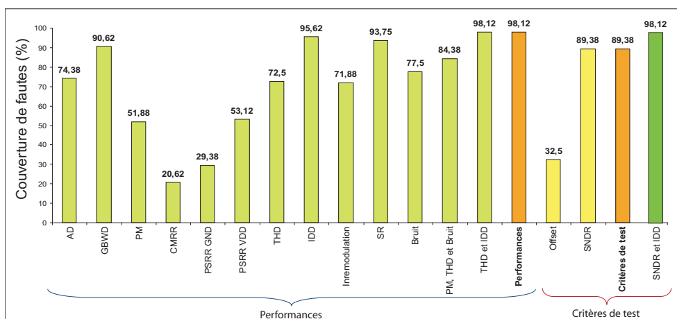
FIG. 5.23 – La Couverture de fautes catastrophiques des performances et des critères de test.
