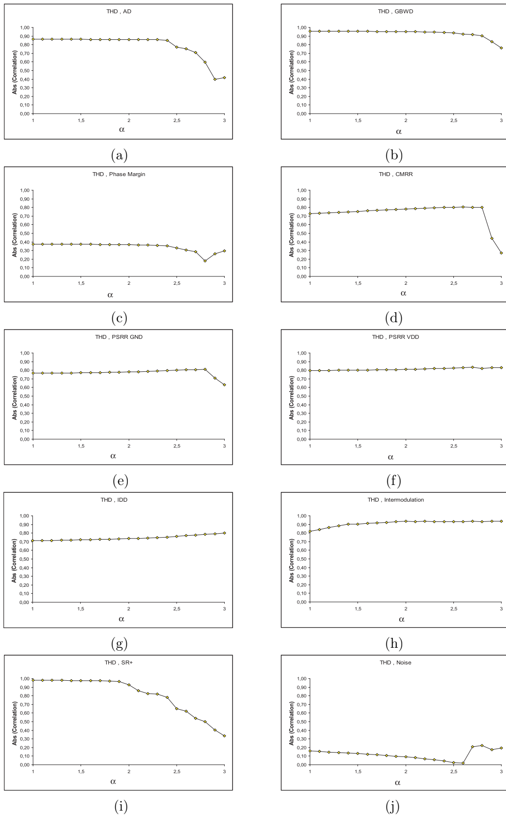
FIG. 4.6 – Coefficients de corrélation en valeurs absolue entre le THD et les autres performances du circuit en fonction du rapport d'augmentation de l'écart-type \alpha .
