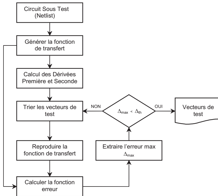
FIG. 3.23 – Génération de vecteurs de test par interpolation.
