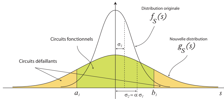
FIG. 4.5 – Exemple d'une performance élargie.
