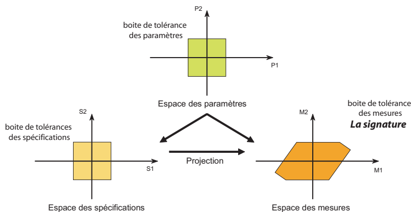
FIG. 3.18 – Calcul de l'espace de la signature.
