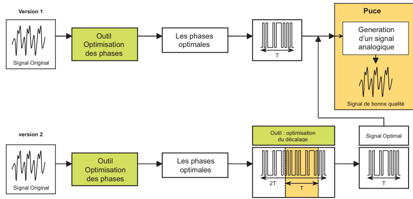
FIG. 6.12 – Technique d’optimisation de la qualité de vecteurs de test numériques.
