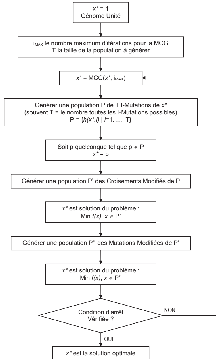
FIG. A.2 – L'algorithme MCMGA.
