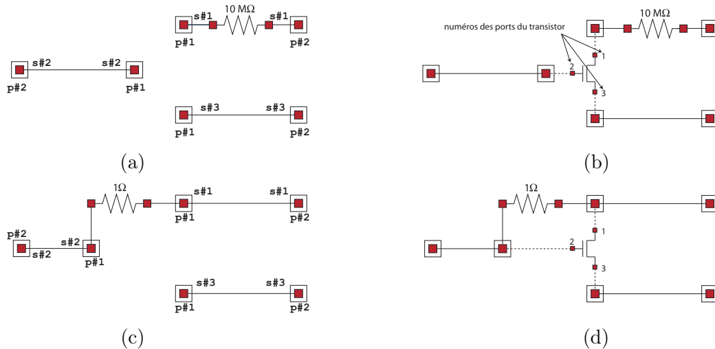
FIG. 5.1 – Construction d’un modèle de fautes : (a) et (c) représentation en format FMDL, (b) et (d) exemples d’injections des modèles de fautes pour le cas d’un transistor.
