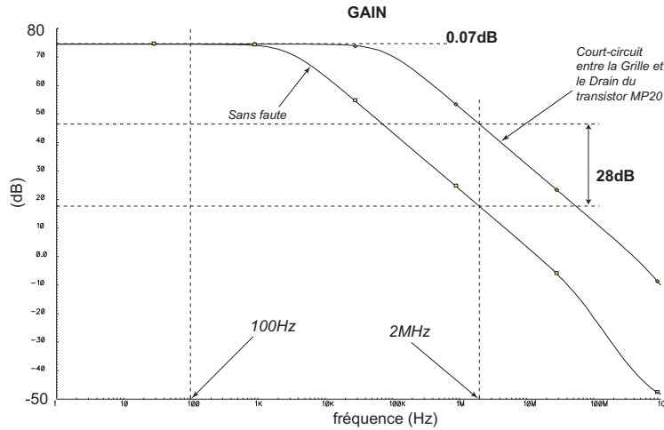
FIG. 6.8 – La performance Gain avec une fréquence qui ne permet pas de détecter une faute (a) et une fréquence qui permet de détecter cette faute (b).
