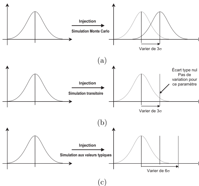
FIG. 5.5 – Différentes injections de fautes paramétriques.
