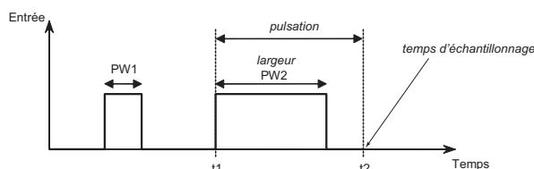
FIG. 3.16 – Vecteur de test composé d'une série de pulsations.
