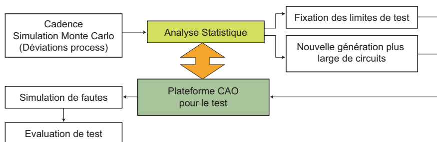
FIG. 4.1 – Méthode d'évaluation de test par modélisation statistique du circuit sous test.
