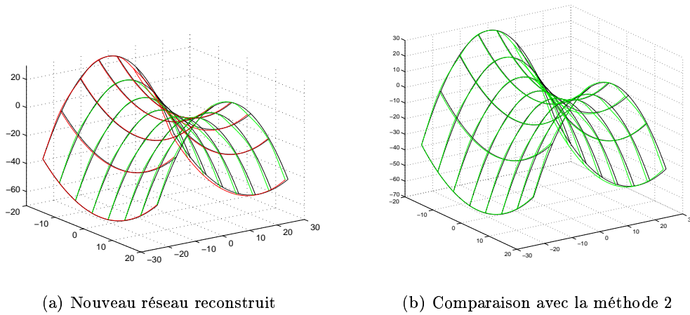
FIG. 3.25 – Selle : Reconstruction du réseau avec contraintes dans une direction ( noir ) : réseau réel, ( gauche, rouge ) : courbes reconstruites avec contraintes de longueur, ( gauche vert ) : courbes reconstruites avec contraintes de positions
