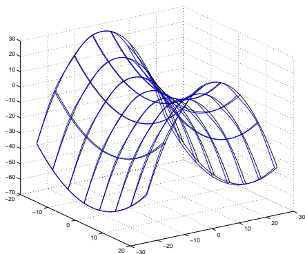
(a) Réseau de courbes indépendantes (non fermé)
