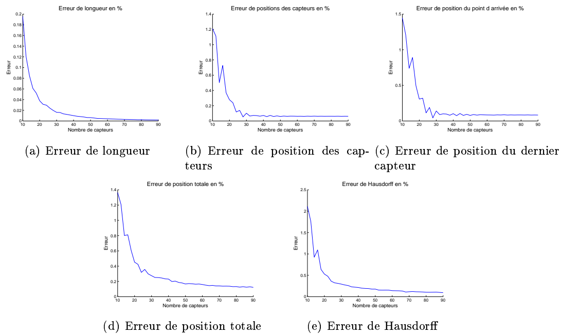
FIG. 1.35 – Erreurs pour la spline 3D
