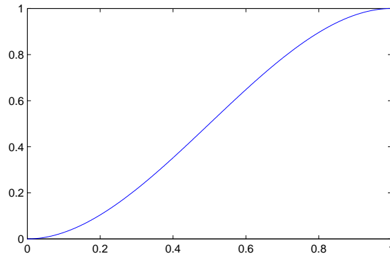
FIG. 3.5 – fonction de Hermite \varphi_1
