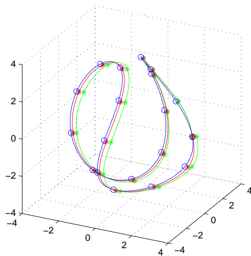
FIG. 1.46 – Reconstruction bruitée pour la courbe fermée, (bleu) : courbe initiale, (rouge) : courbe reconstruite à partir de données non bruitées, (vert) : courbe reconstruite à partir de données bruitées
