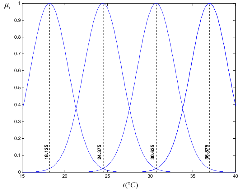
FIG. 4.6 – Fonctions d'activation en fonction de la température
