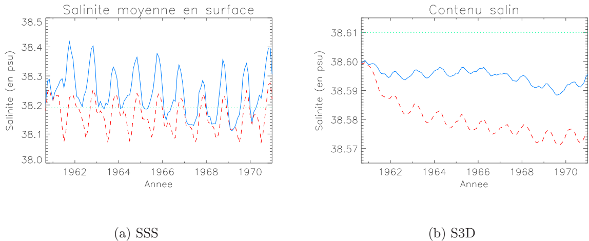
FIG. 2.7 – Evolution temporelle de (a) la salinité de surface et (b) la salinité moyenne de la colonne d'eau à partir de deux simulations de 10 ans, l'une avec rappel newtonien pour la SSS (pointillés) et l'autre avec des fleuves explicites et sans rappel pour la SSS (trait plein).
