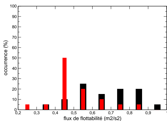
FIG. 4.40 – Distribution statistique de la perte de flottabilité hivernale par classes pour OM8-ARP (noir) et CAM (rouge).
