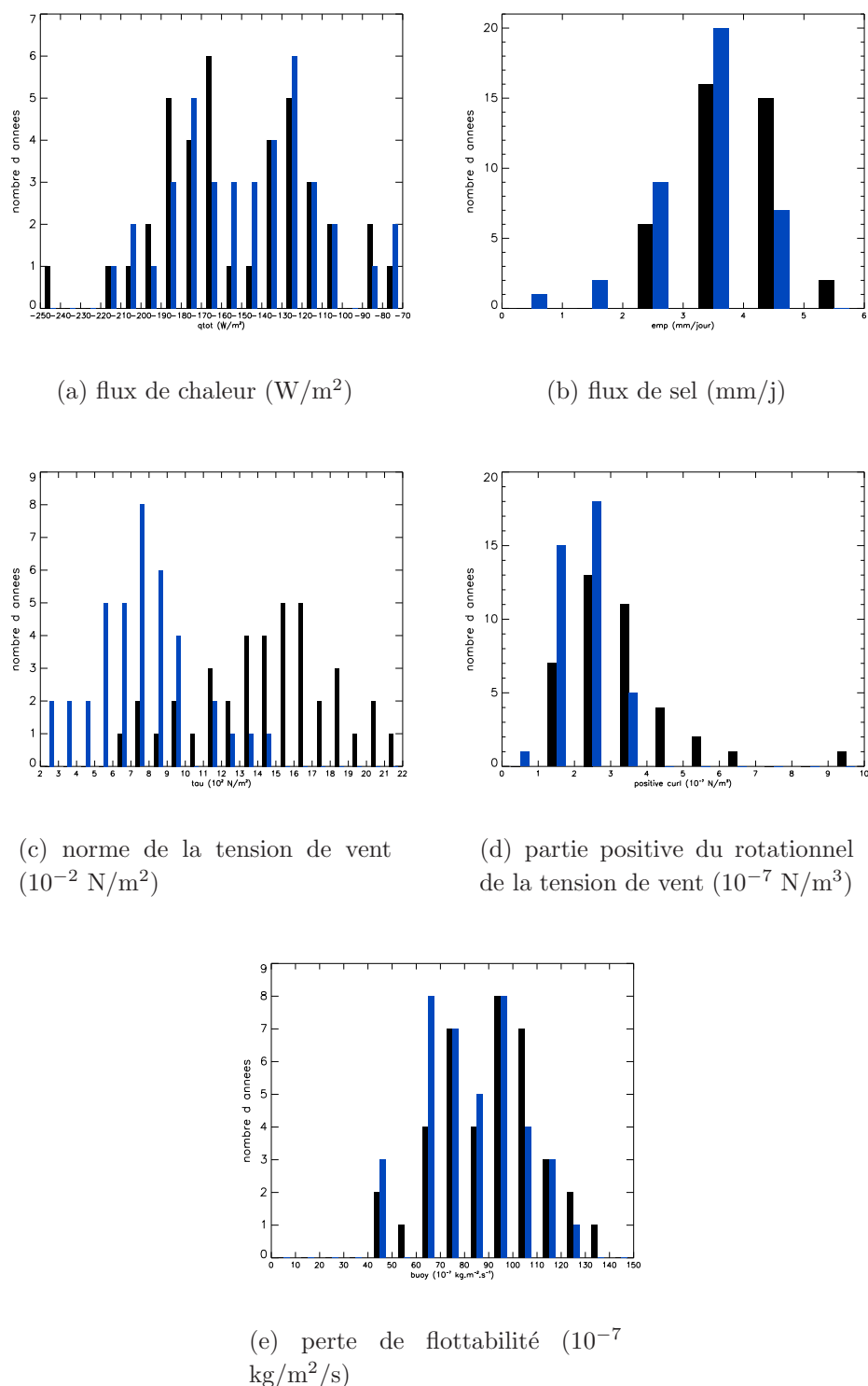
FIG. 3.32 – Histogrammes sur 39 ans pour OM8-ERP (en noir) et OM8-ERA (en bleu) sur la zone LION4 en moyenne sur DJF pour les flux air-mer.
