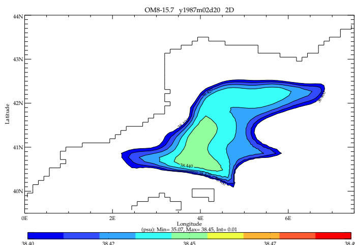
FIG. 3.7 – Salinité de surface le 20 février 1987 pour l'expérience de référence OM8-15.7. Selon le critère donné par (Leaman and Schott, 1991), la zone de convection profonde est délimitée par l'isoligne 38.40 psu.
