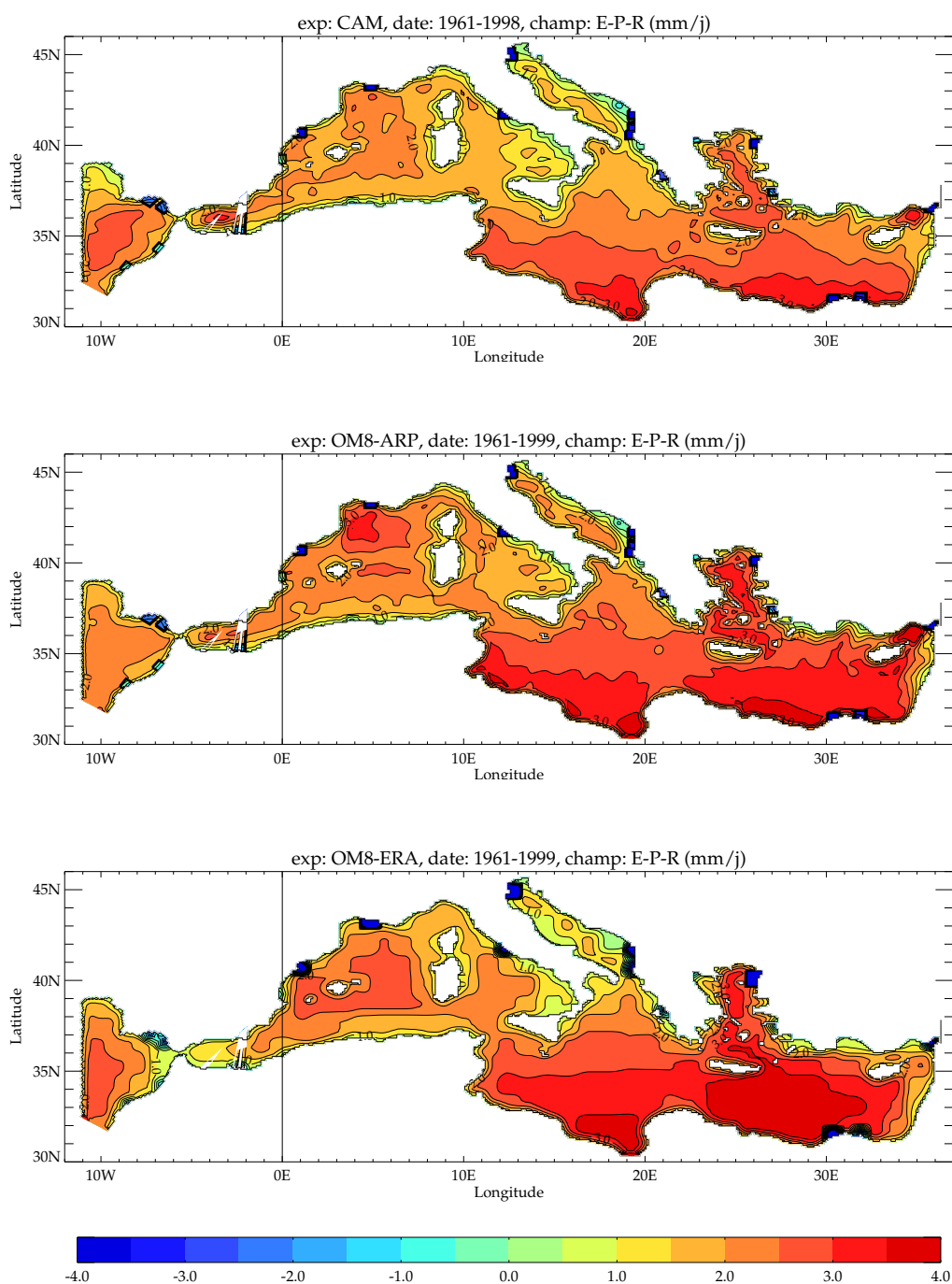
FIG. 4.6 – Même légende que la figure 4.5 pour le flux d'eau (mm/j). Notons que le terme correctif utilisé pour OM8-ERA est inclus.
