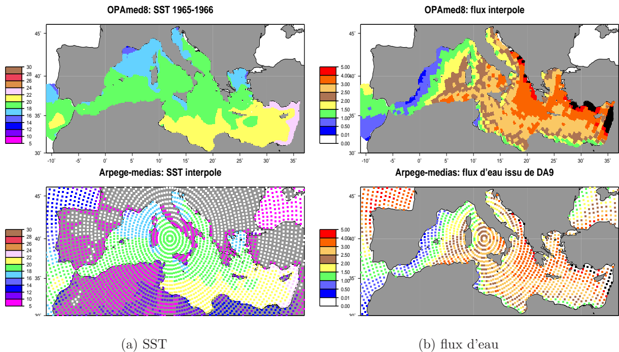
FIG. 2.11 – Exemple d'interpolation dans le modèle couplé régional SAMM (a) d'un champ de SST et (b) d'un champ de flux d'eau (E-P). Champs d'OPAMED8 en haut et d'ARPEGE-Climat Medias en bas.
