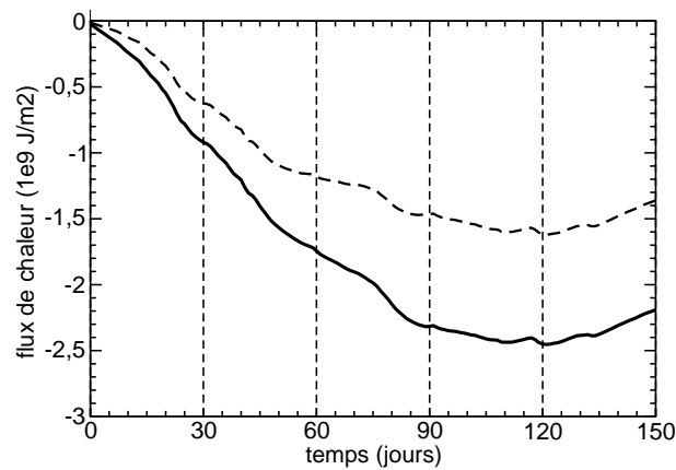
FIG. 3.2 – Série temporelle du flux de chaleur cumulé quotidiennement de début décembre à fin avril (en 10^9 \text{ J.m}^{-2} , moyenne sur LION4). Le flux issu de la réanalyse ERA40 avant correction en tiret, après correction en trait plein.
