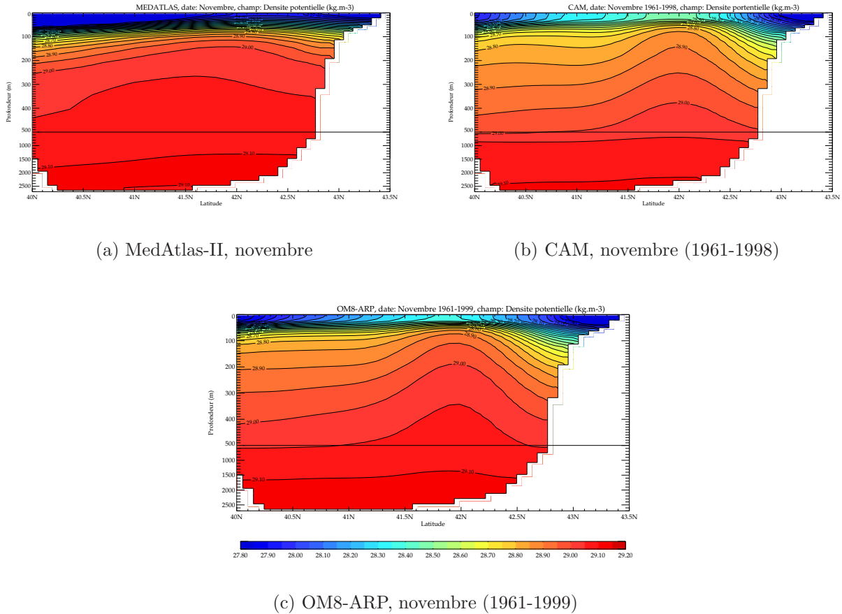
FIG. 4.29 – Section verticale à 4.5^{\circ}\text{E} de la densité potentielle en novembre pour (a) la climatologie MedAtlas-II, (b) la simulation CAM (moyenne sur 1961-1998) et (c) la simulation OM8-ARP (1961-1999).
