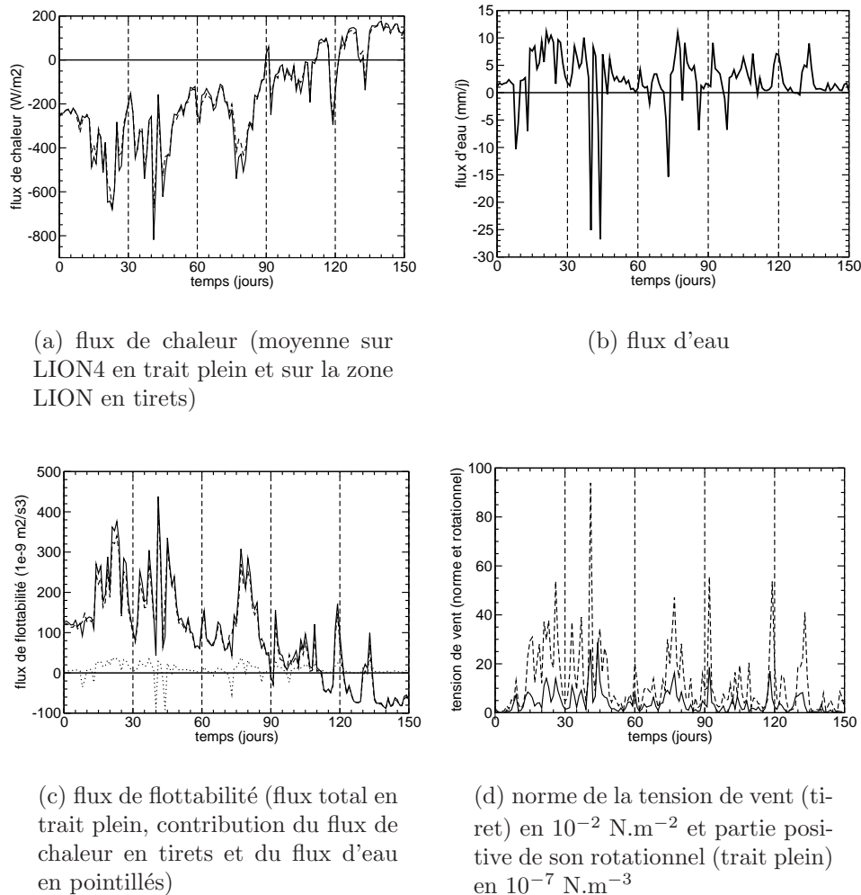
FIG. 3.3 – Série temporelle (en jours) de début décembre à fin avril pour les différents flux océan-atmosphère moyennés sur la zone LION4.
