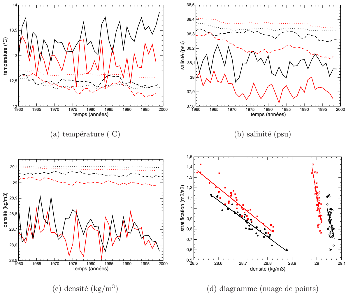
FIG. 4.26 – Evolution temporelle pour 3 couches de la zone LION4 (a) de la température, (b) de la salinité et (c) de la densité pour le mois de novembre pour OM8-ARP en noir et CAM en rouge. Les couches sont la couche de surface (0-150 m, trait plein), la couche intermédiaire (150-1000 m, tirets) et la couche profonde (sous 1000 m, pointillés). La figure (d) représente, sous forme de nuage de points (OM8-ARP en noir et CAM en rouge), la corrélation de la stratification verticale en novembre avec la densité des couches de surface (symbole plein) et intermédiaires (symbole vide).
