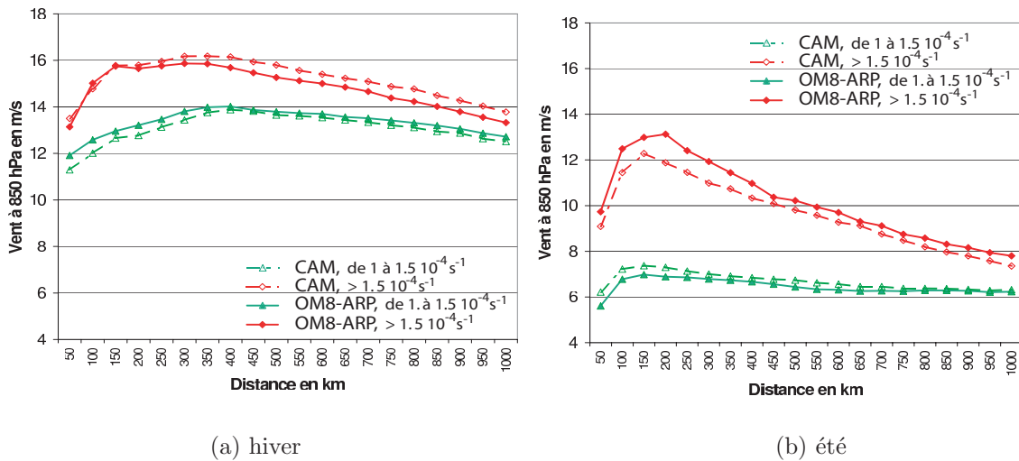
FIG. 5.26 – Composites de vent moyen à 850 hPa (en m/s) pour les trajectoires qui naissent dans le golfe de Gênes (a) en hiver et (b) en été pour ARP (symboles et traits pleins) et CAM (symboles vides et tirets).
