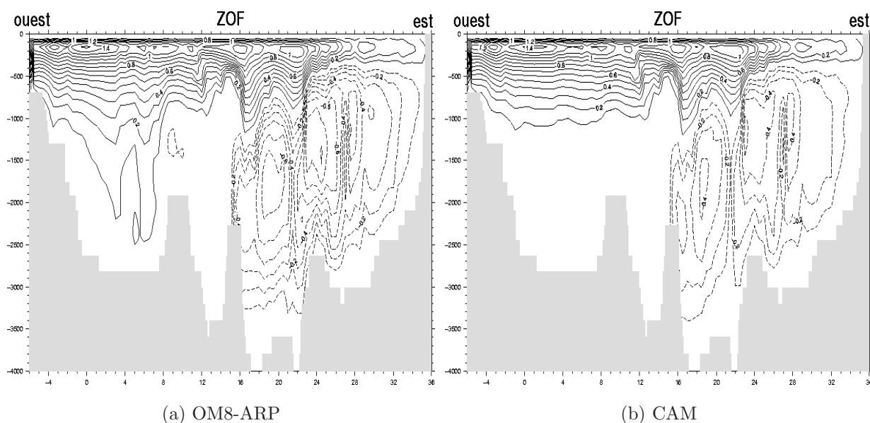
FIG. 4.13 – Fonction de retournement zonale intégrée sur l'ensemble de la Méditerranée pour (a) OM8-ARP (moyenne sur 1961-1999) et (b) CAM (moyenne sur 1961-1998).
