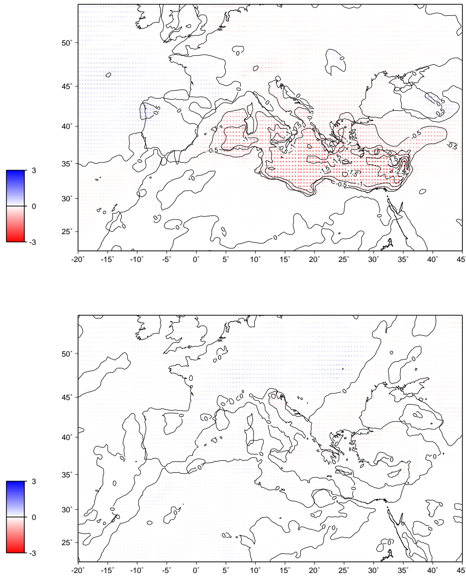
FIG. B.7 – Différence de précipitations moyennes (en mm/jour) CAM-ARP, en hiver (en haut) et en été (en bas).
