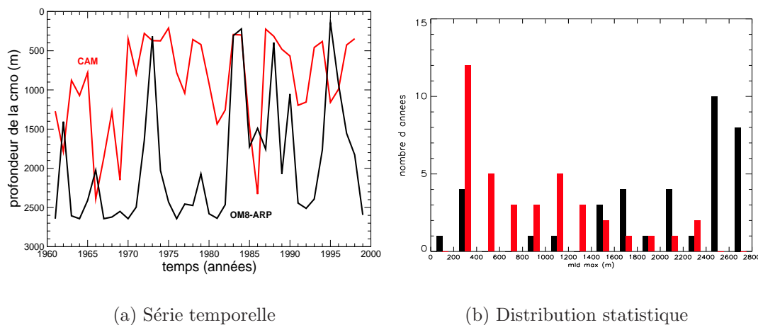
FIG. 4.21 – Série temporelle du maximum de la profondeur de la couche mélangée (maximum sur la zone LION4 et sur les mois de janvier, février et mars à partir de fichiers mensuels) pour les simulations OM8-ARP (en noir) et CAM (en rouge). Le champ est montré sous (a) la forme d'une série temporelle et (b) d'un histogramme.
