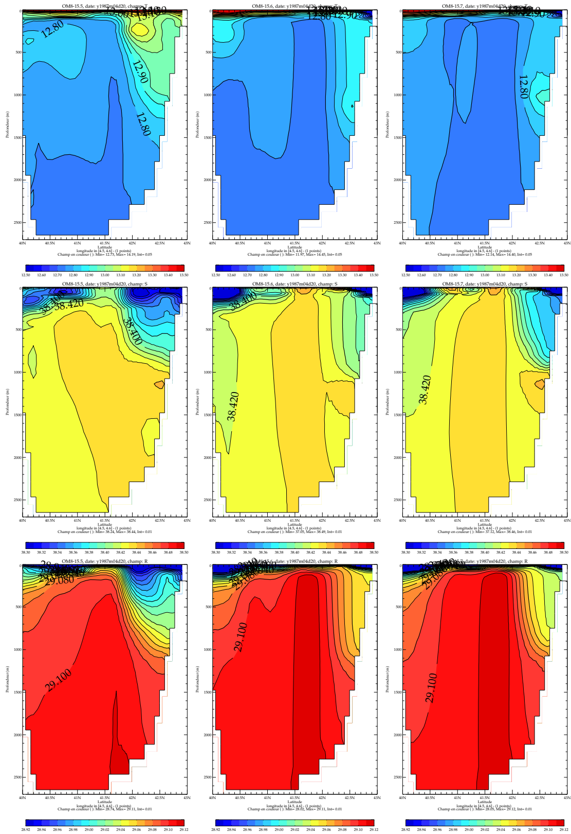
FIG. 3.12 – Comme la figure 3.8 mais pour le 20 avril 1987.
