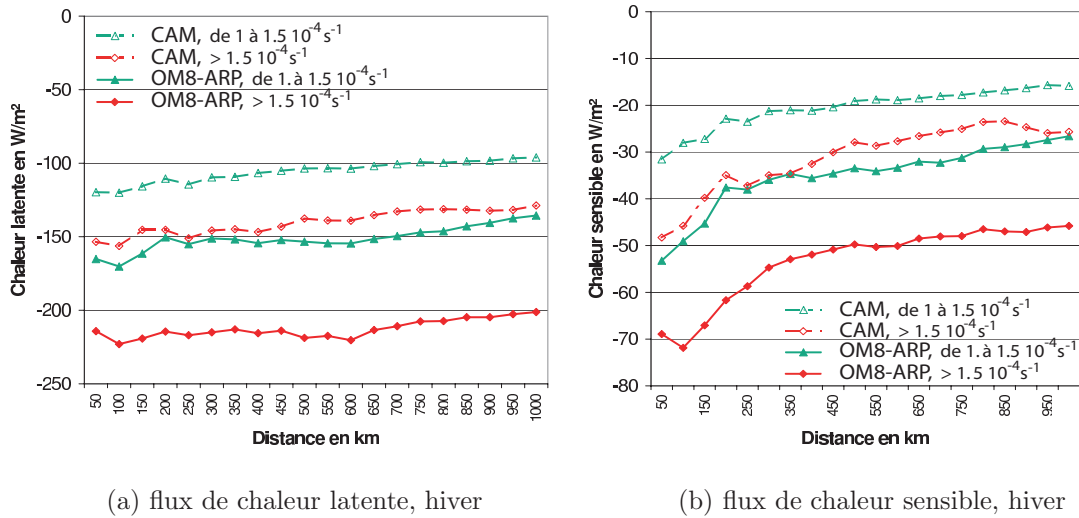
FIG. 5.27 – Composites de flux de chaleur latente et sensible (en W/m^2 ) pour les trajectoires qui naissent dans le golfe de Gênes, pour ARP (symboles et traits pleins) et CAM (symboles vides et tirets), en hiver.
