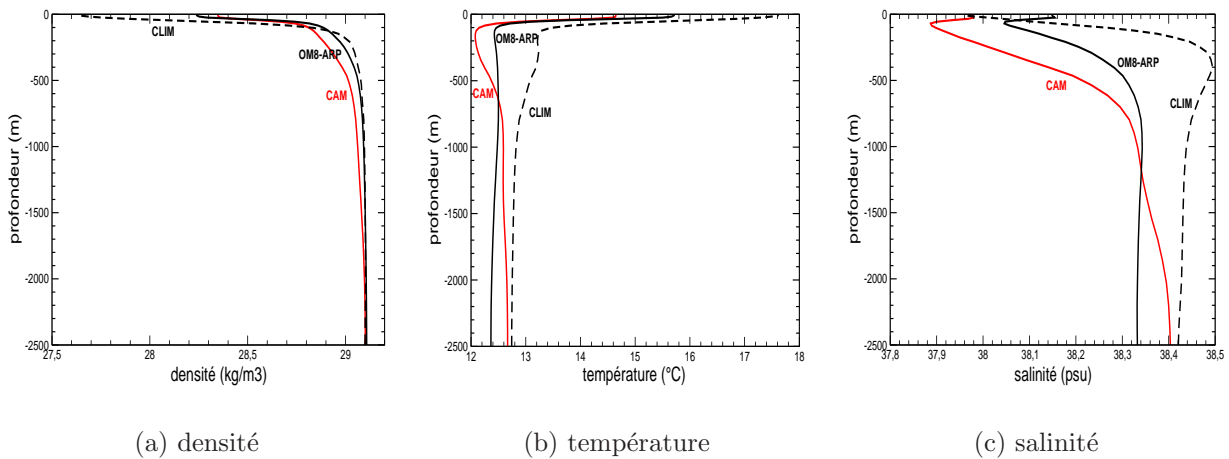
FIG. 4.23 – Profil vertical moyen de (a) densité, (b) température et (c) salinité sur la zone LION4 en moyenne sur le mois de novembre et sur l'ensemble de la simulation. OM8-ARP en noir, CAM en rouge et MedAtlas-II en tiret noir.
