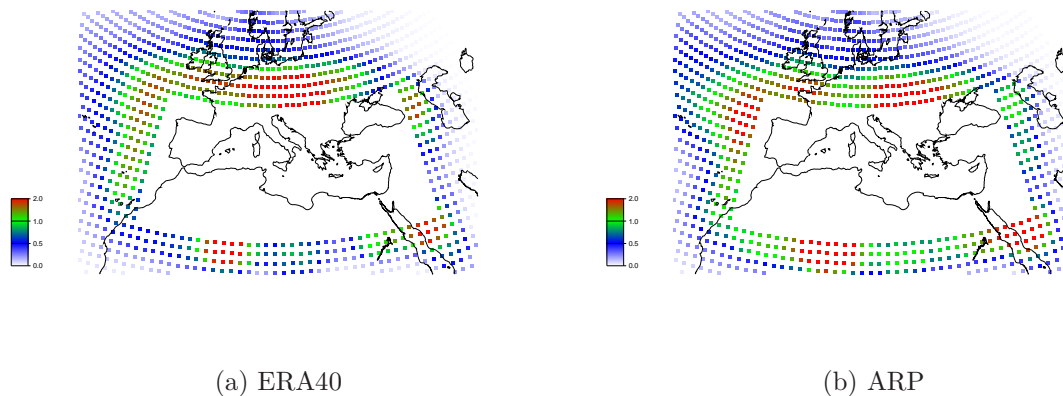
FIG. 5.9 – Densités de cyclogénèse des trajectoires entrant dans le domaine méditerranéen, en moyenne sur l'année, pour (a) ERA40 et (b) ARP (nombre moyen par mois dans un rayon de 380 km).
