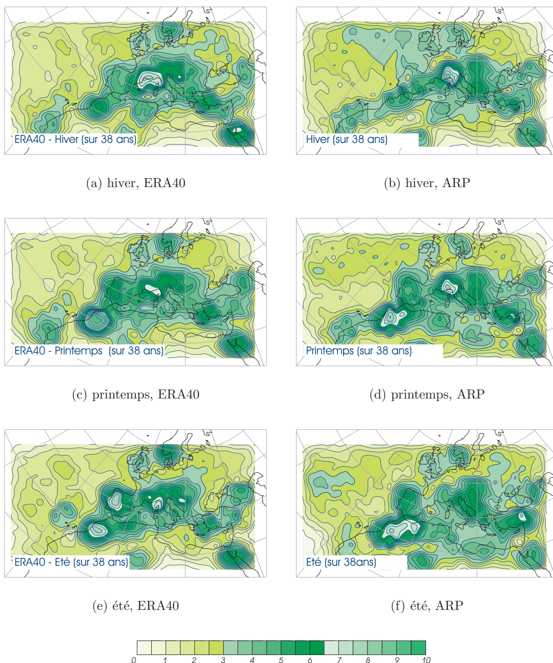
FIG. 5.8 – Densités de cyclogénèse pour ERA40 (droite) et ARP (gauche) sur les 38 années d'étude (a,b) en hiver, (c,d) au printemps et (e,f) en été (nombre moyen par mois dans un rayon de 380 km; l'isoligne en gras correspond à la valeur 3).
