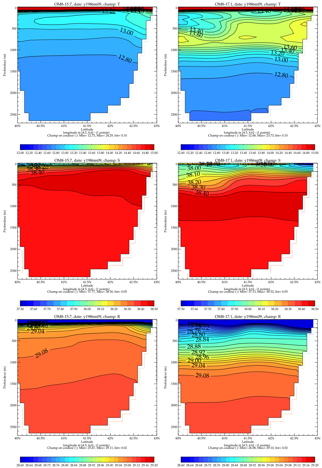
FIG. 3.25 – Section verticale à 4,5°E (de 40 à 43°N) de température (haut), salinité (milieu) et densité (bas) pour les simulations OM8-15.7 (gauche) et OM8-17.1 (droite). Moyenne mensuelle pour septembre 1986.
