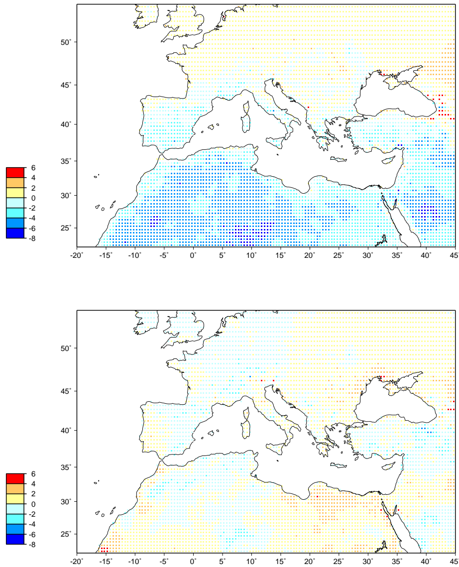
FIG. B.2 – Différence de température moyenne à 2m (en °C) ARP-CRU, en hiver (en haut) et en été (en bas).
