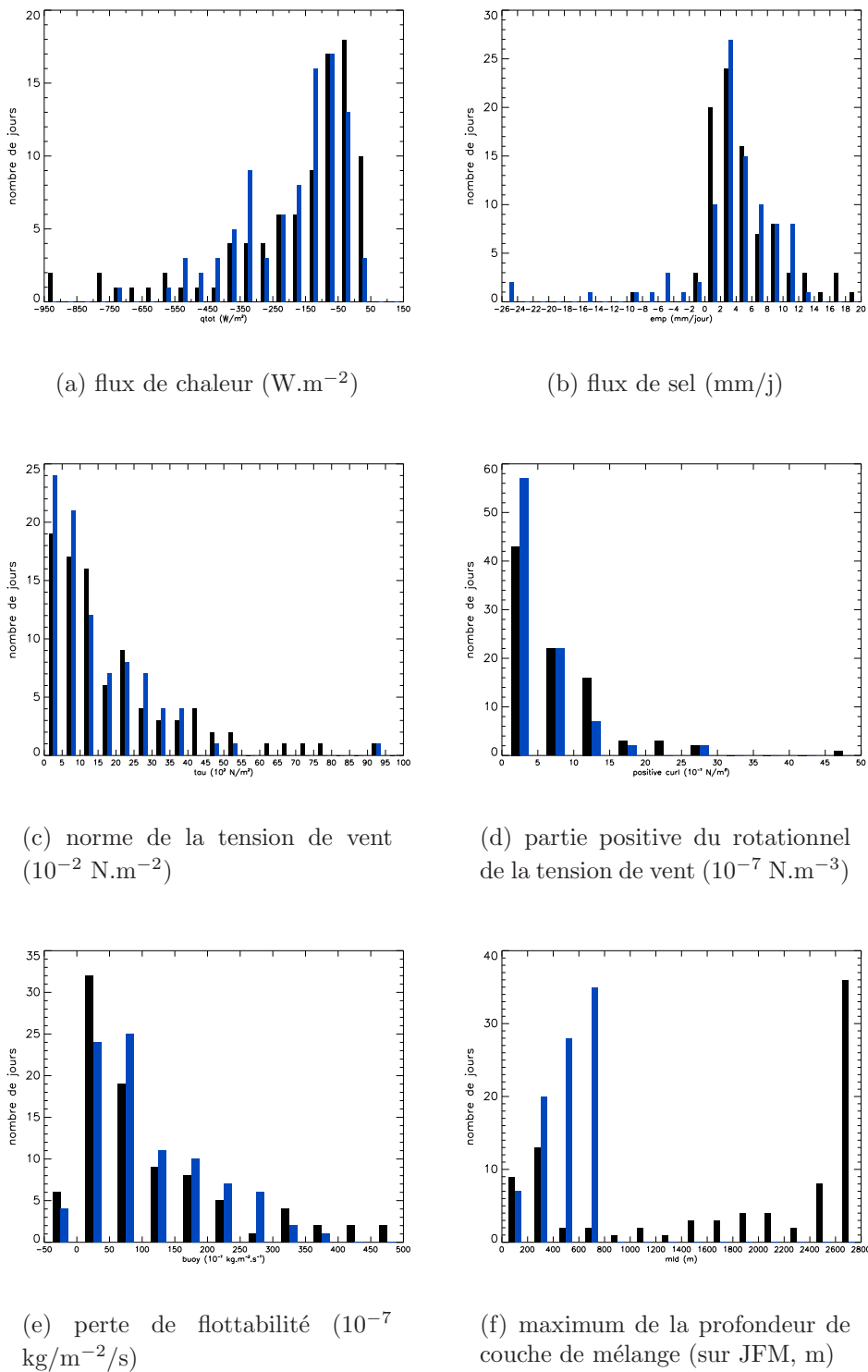
FIG. 3.33 – Histogrammes à partir des valeurs quotidiennes sur la période hivernale DJF pour l’année 1979-80 d’OM8-ARP (en noir) et l’année 1986-87 d’OM8-ERA (en bleu) sur la zone LION4.
