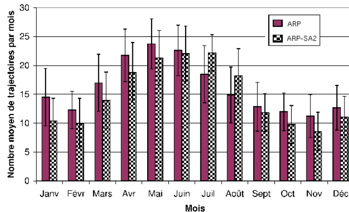
FIG. 5.17 – Histogramme du nombre moyen mensuel de trajectoires pour les trajectoires dont \zeta_{max} > 1.10^{-4}s^{-1} , dans le domaine méditerranéen, pour ARP (rouge) et ARP-SA2 (noir et blanc).
