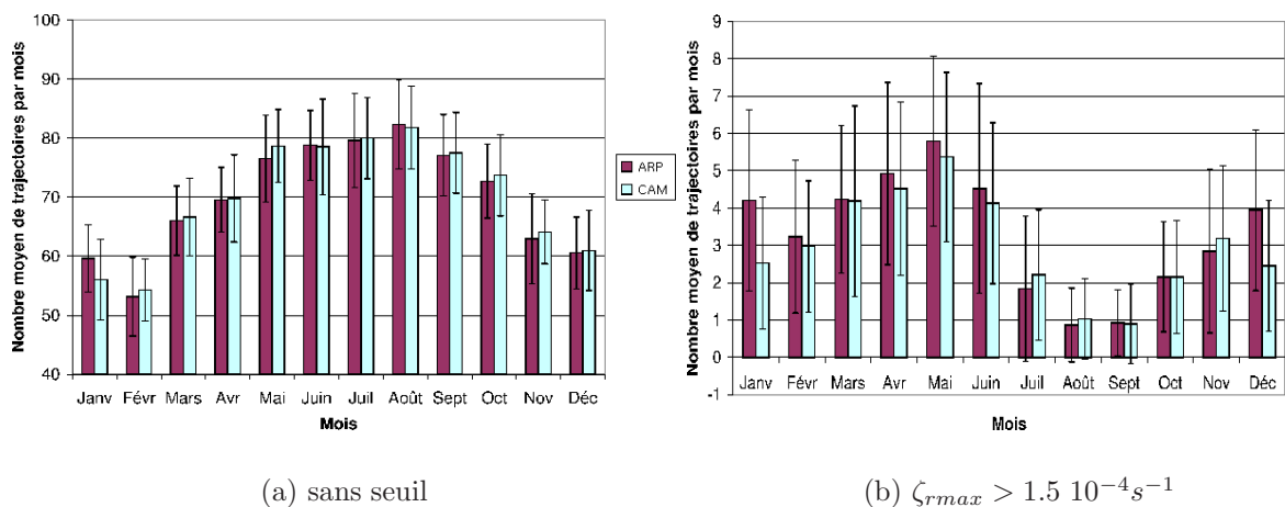
FIG. 5.11 – Histogramme du nombre moyen mensuel de trajectoires (a) sans seuil d'intensité et (b) pour les trajectoires dont \zeta_{rmax} > 1.5 \cdot 10^{-4} s^{-1} . Moyenne sur 38 ans, dans le domaine méditerranéen, pour ARP (rouge) et CAM (bleu).
