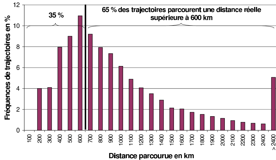
FIG. 5.4 – Répartition des trajectoires dont la distance entre positions de début et de fin est inférieure à 600 km en fonction de la distance réellement parcourue pour l'expérience ARP, sur le domaine méditerranéen et sur la période 1960-1998.
