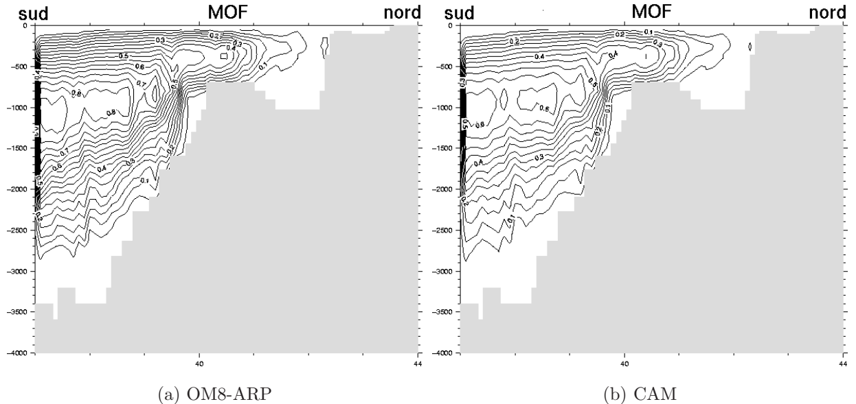
FIG. 4.15 – Fonction de retournement méridionale intégrée sur la mer Adriatique et le Nord de la mer Ionienne (limitée à 37°N) (a) OM8-ARP (moyenne sur 1961-1999) et (b) CAM (moyenne sur 1961-1998).
