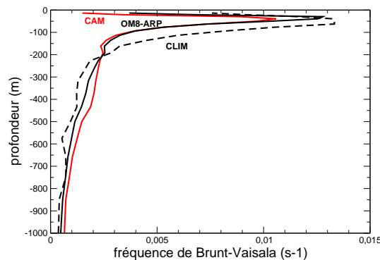
FIG. 4.24 – Même légende que la figure 4.23 mais pour la fréquence de Brunt-Vaisala.
