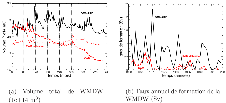
FIG. 4.30 – Evolution temporelle pour la zone LION (a) du volume total de WMDW (eau plus dense que 29.08 \text{ kg/m}^3 pour OM8-ARP et que 29.06 \text{ kg/m}^3 pour CAM) et (b) du taux annuel de formation de la WMDW (mêmes seuils). OM8-ARP en noir, CAM en rouge et la courbe débiaisée de CAM en tirets rouge.
