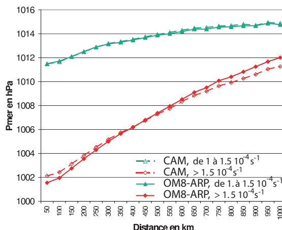
FIG. 5.24 – Composites de pression réduite au niveau de la mer (en hPa) pour les trajectoires qui naissent dans le golfe de Gênes, pour ARP (symboles pleins) et CAM (symboles vides et tirets), en hiver.
