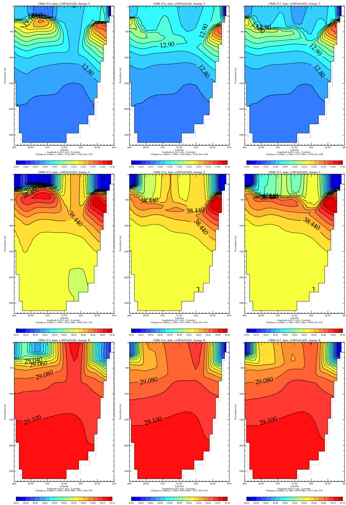
FIG. 3.9 – Comme la figure 3.8 mais pour le 20 janvier 1987.
