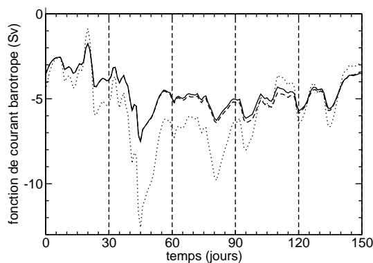
FIG. 3.14 – Série temporelle de début décembre à fin avril de la fonction de courant barotrope moyennée sur la zone LION_4 , c'est-à-dire au coeur du gyre cyclonique entourant la zone de convection. L'expérience de référence avec correction du flux de chaleur (OM8-15.7) en trait plein, avec correction du flux de chaleur et de sel (OM8-15.6) en tirets, avec correction du flux de chaleur, du flux de sel et du flux de quantité de mouvement (OM8-15.5) en pointillés.
