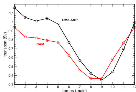
FIG. 4.35 – Cycle saisonnier moyen du transport net (Sv) vers l'Ouest au Nord de la Corse pour OM8-ARP (en noir) et CAM (en rouge).
