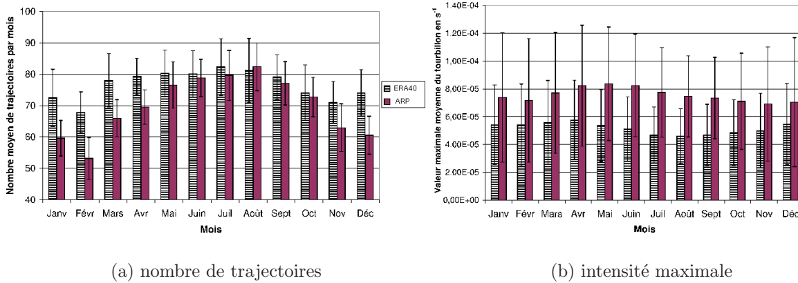
FIG. 5.6 – Histogramme (a) du nombre moyen mensuel de trajectoires et (b) de l'intensité maximale moyenne mensuelle sur 38 ans, dans le domaine méditerranéen, pour ERA40 (en rayé blanc et noir) et ARP (en rouge).
