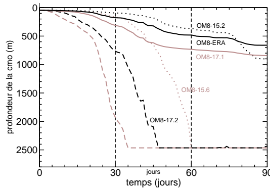
FIG. 3.28 – Série temporelle de la profondeur de couche de mélange calculée avec le modèle 0D. En trait noir, sans correction de flux de chaleur et en gris avec. En trait plein, CI=OM8-ERA ; en tirets, CI=OM8-ARP et en pointillés CI=OM8-R3D.
