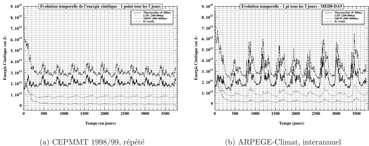
FIG. 2.8 – Energie cinétique en J (un point tous les 5 jours) dans deux simulations de 10 ans et pour différentes couches de la mer Méditerranée, (a) simulation avec forçage perpétuel par l’année 1998-99 du CEPMMT et (b) simulation avec forçage interannuel issu d’ARPEGE-Climat.
