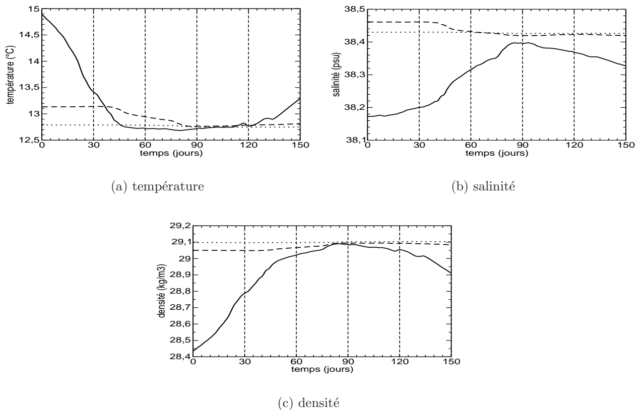
FIG. 3.13 – Séries temporelles de (a) la température, (b) la salinité et (c) la densité, moyennées sur LION4 et intégrées sur 3 couches. La couche de surface (de la surface à 150 m) en trait plein, la couche intermédiaire de (150 à 600 m) en tirets et la couche profonde (au-delà de 600 m) en pointillés.
