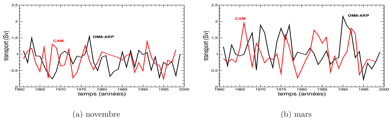
FIG. 4.36 – Série temporelle du transport total (Sv) vers l'Ouest à travers le détroit situé entre la Corse et le continent à 9.5^\circ\text{E} (a) en novembre et (b) en mars pour les simulations OM8-ARP (en noir) et CAM (en rouge).
