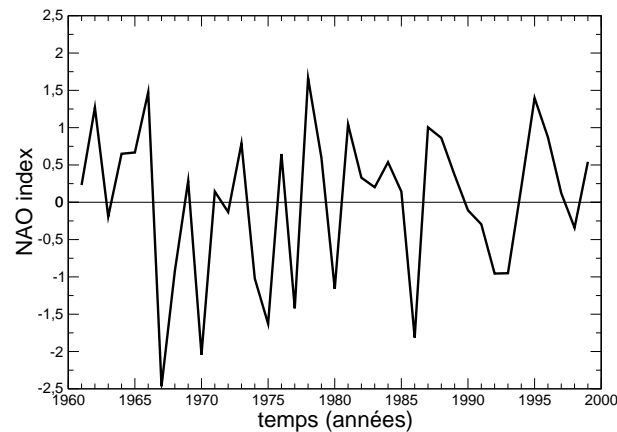
FIG. 4.43 – Série temporelle de l'indice NAO calculé pour l'expérience OM8-ARP (données fournies par Terray, communication personnelle).
