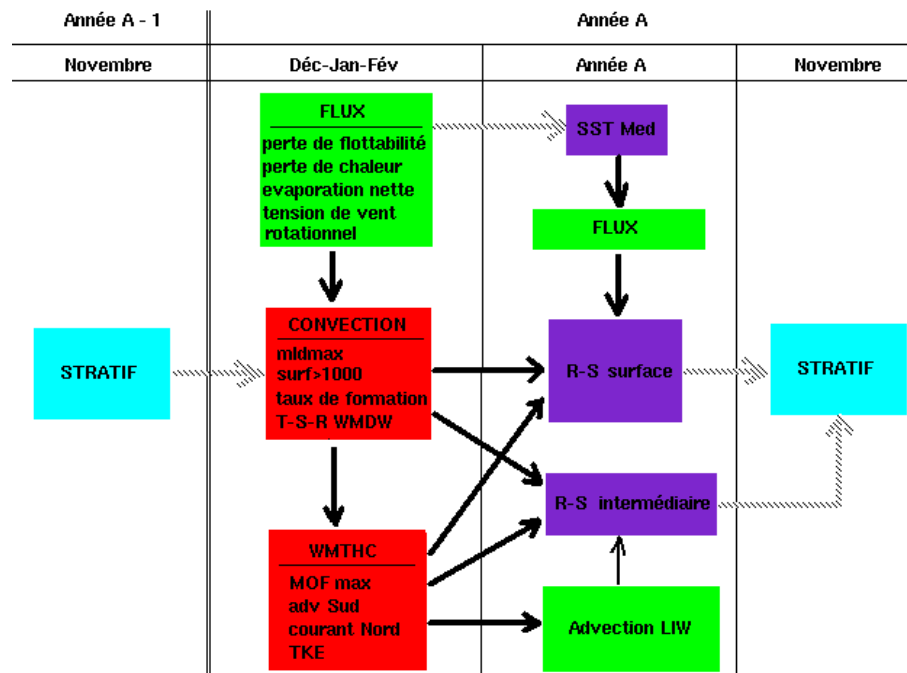
FIG. 4.42 – Schéma de synthèse des liens entre variables physiques concernant la variabilité interannuelle de la formation de la WMDW dans la simulation CAM. Les flèches noires (respectivement rayées) représentent des corrélations positives (respectivement négatives). R représente la densité, S la salinité. Lorsque ce n'est pas précisé, les grandeurs sont calculées pour la zone de convection (LION4).
