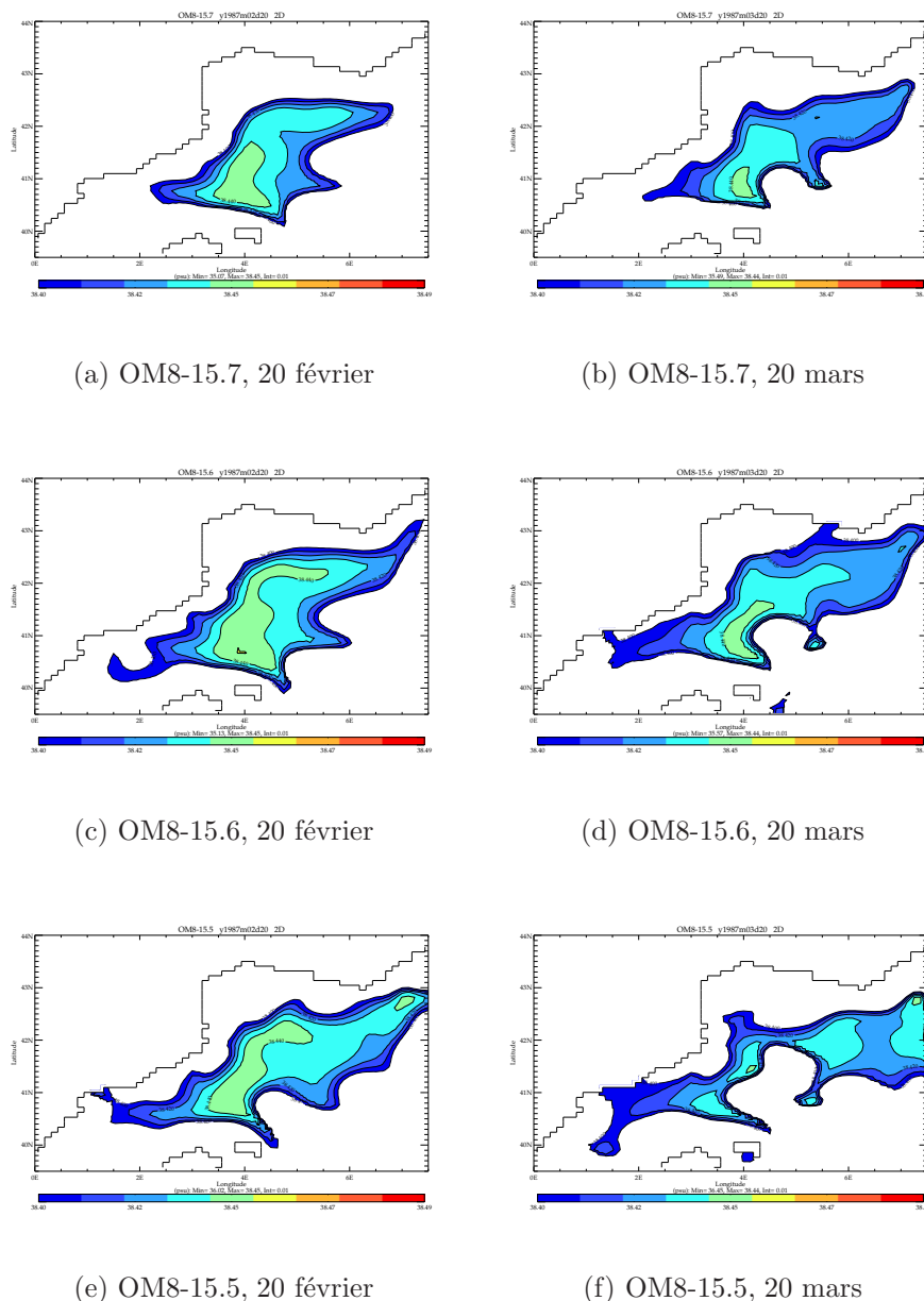
FIG. 3.21 – Moyenne quotidienne (20 février et 20 mars) de la salinité de surface (en psu) pour OM8-15.7, 15.6 et 15.5. La salinité est seuillée à 38.40 psu pour que la zone colorée représente la zone de convection profonde suivant le critère de MS98.
