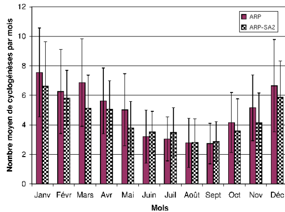
FIG. 5.30 – Histogrammes du nombre moyen mensuel de cyclogénèses pour les trajectoires dont \zeta_{rmax} > 1.10^{-4} s^{-1} pour ARP (rouge) et ARP-SA2 (noir et blanc), golfe de Gênes.
