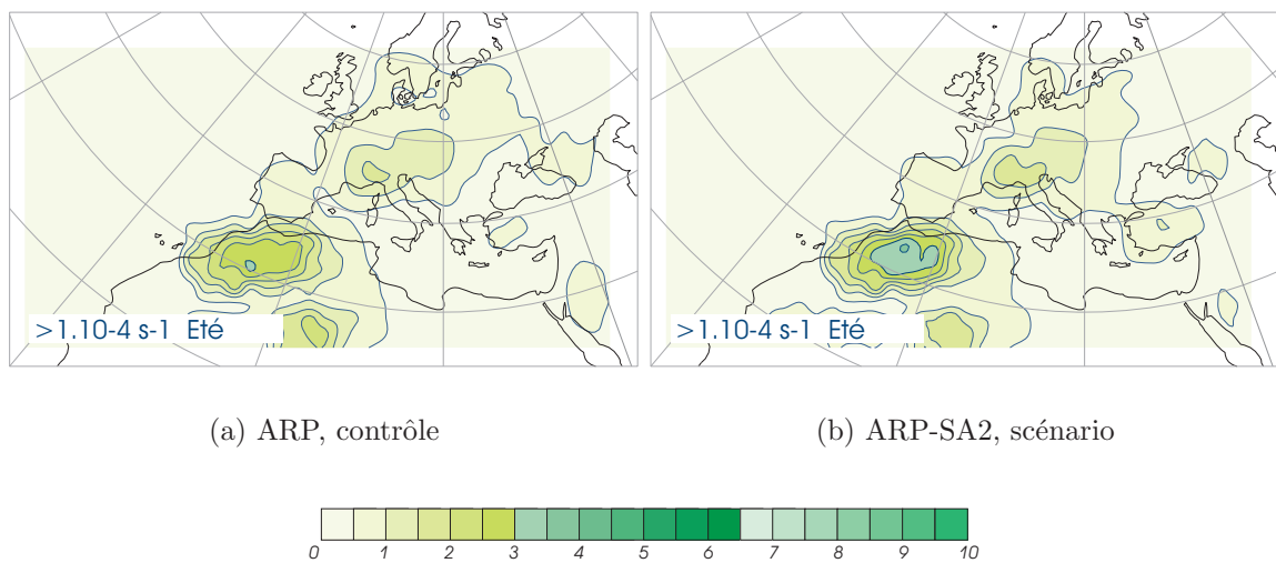
FIG. 5.19 – Même légende que la figure 5.18 mais en été.
