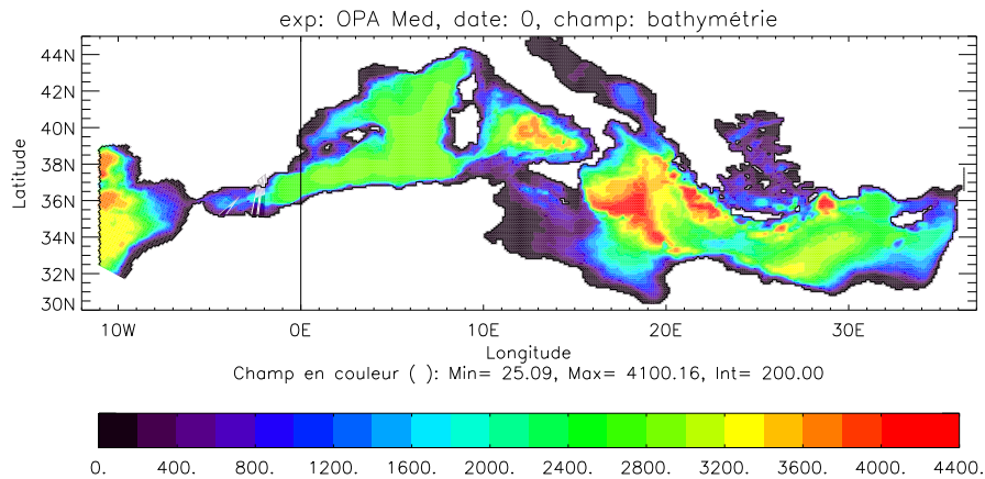
FIG. 2.5 – Bathymétrie et trait de côte d'OPAMED8.
