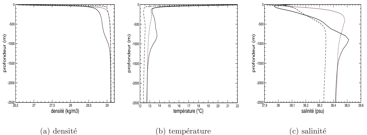
FIG. 3.27 – Profil vertical moyen en (a) densité, (b) température et (c) salinité sur la zone LION 4 en juillet, c'est-à-dire juste avant le démarrage des expériences OM8-17.2 (tirets), OM8-15.X (pointillés) et OM8-ERA (noir). On a ajouté les profils issus de la climatologie MEDATLAS-II (gris) qui sont confondus avec ceux d'OM8-15.X.
