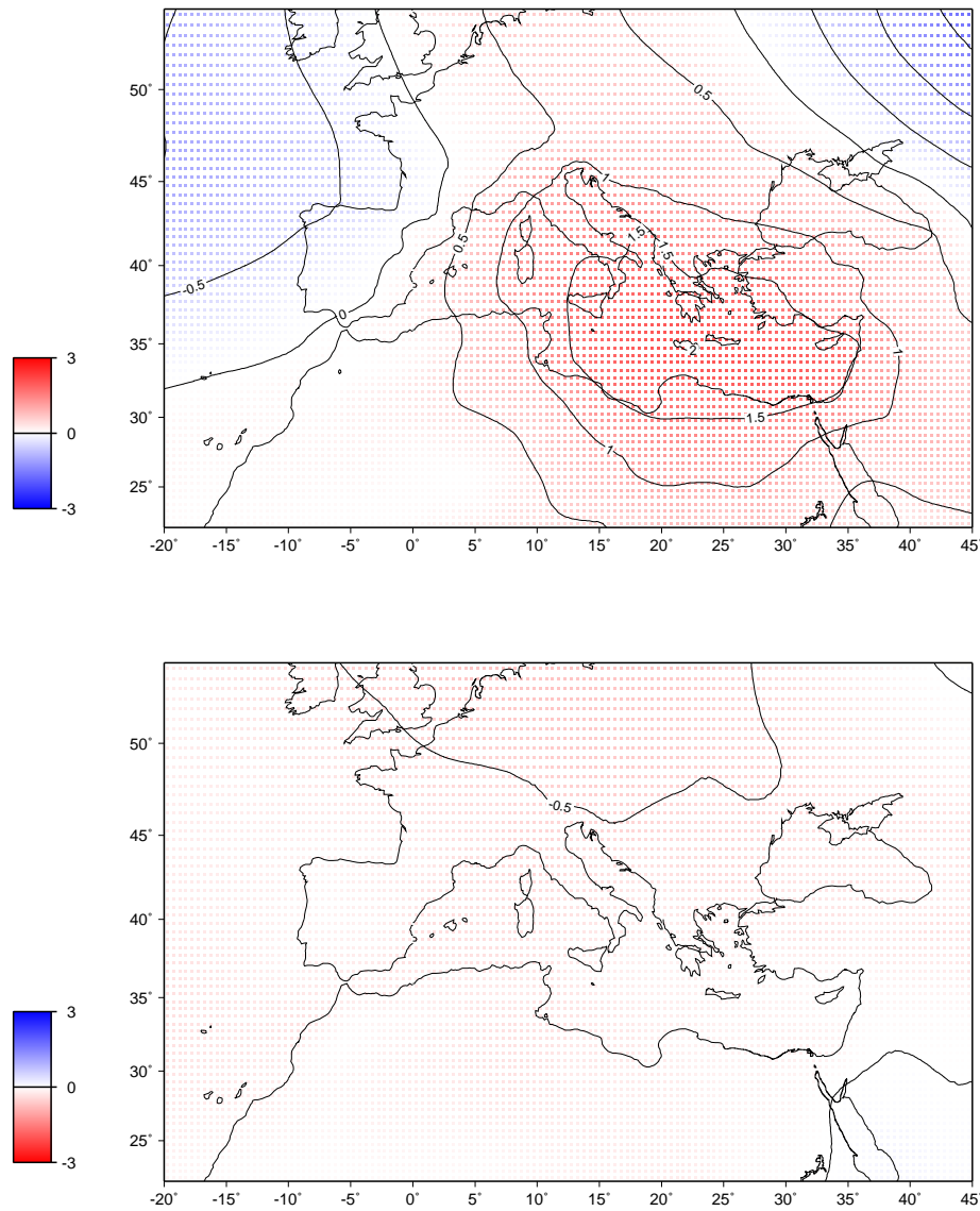
FIG. B.5 – Différence de pression réduite au niveau de la mer moyenne (en hPa) CAM-ARP, en hiver (en haut) et en été (en bas).
