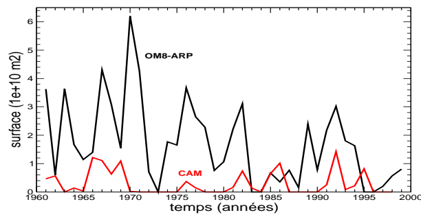
FIG. 4.22 – Série temporelle de la surface pour laquelle la profondeur de la couche de mélange dépasse 1000 m dans la zone LION (moyenne sur JFM de chaque année) pour les simulations OM8-ARP (en noir) et CAM (en rouge).
