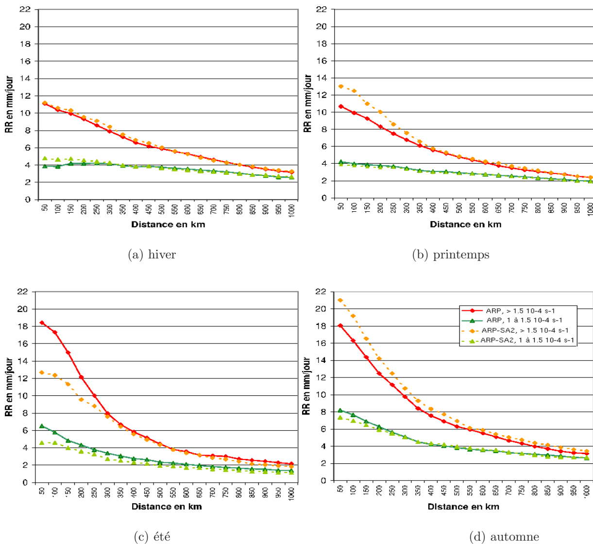
FIG. 5.32 – Composites de précipitations (en mm/jour) pour les trajectoires qui naissent dans le golfe de Gênes, pour ARP (trait plein) et ARP-SA2 (tirets courts) pour les 4 saisons.
