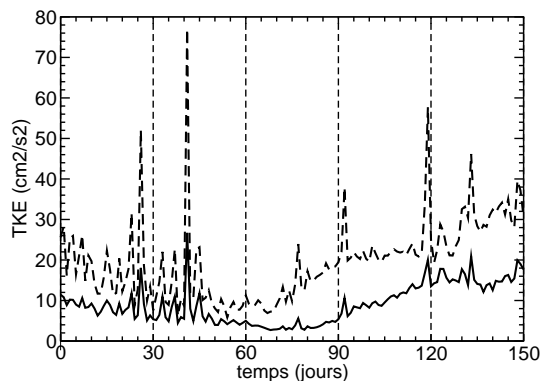
FIG. 3.23 – Série temporelle de l'énergie cinétique turbulente ( TKE , en \text{cm}^2.\text{s}^{-2} ) moyennée sur la zone LION4 et sur les 150 premiers mètres du modèle. Simulation OM8-15.7 en trait plein et OM8-15.5 en pointillés.
