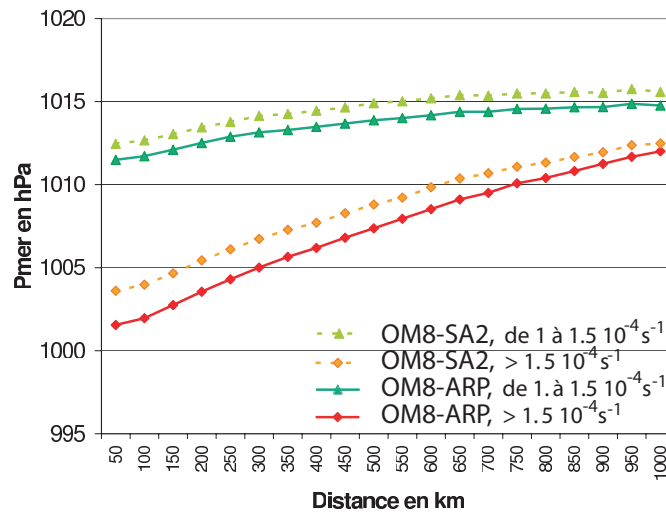
FIG. 5.31 – Composites de pression réduite au niveau de la mer (en hPa) pour les trajectoires qui naissent dans le golfe de Gênes, pour ARP (trait plein) et ARP-SA2 (tirets courts), en hiver.
