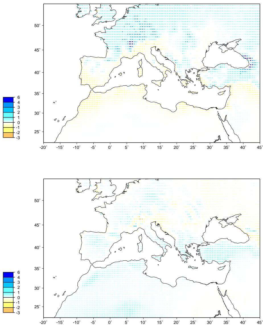
FIG. B.3 – Différence de précipitations moyennes (en mm/jour) ARP-CRU, en hiver (en haut) et en été (en bas).
