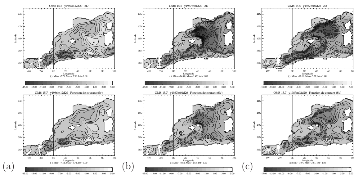
FIG. 3.15 – Fonction de courant barotrope pour les expériences OM8-15.5 (en haut) et OM8-15.7 (en bas) pour la moyenne quotidienne de (a) le 20 décembre ; (b) le 20 janvier et (c) le 20 février.
