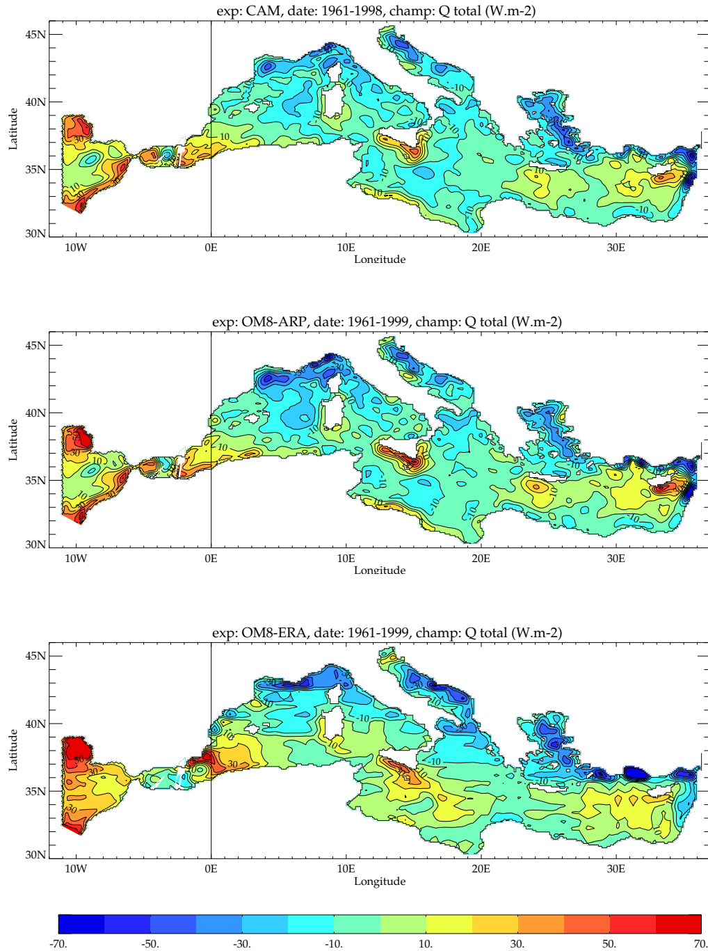
FIG. 4.5 – Carte du flux de chaleur ( W/m^2 ) en moyenne annuelle pour CAM (en haut), OM8-ARP (au milieu) et OM8-ERA (en bas). Les grandeurs sont moyennées sur l'ensemble des simulations et incluent le terme de rappel pour les expériences forcées.
