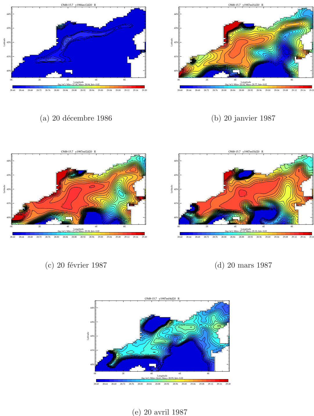
FIG. 3.5 – Moyenne quotidienne du champ de densité en surface pour l'expérience OM8-15.7.
