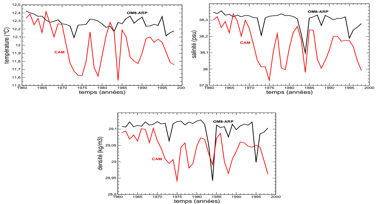
FIG. 4.32 – Série temporelle des caractéristiques (température potentielle, salinité, densité potentielle) de l'eau formée en février au point de profondeur de couche de mélange maximale sur la zone LION pour les simulations OM8-ARP (en noir) et CAM (en rouge).
