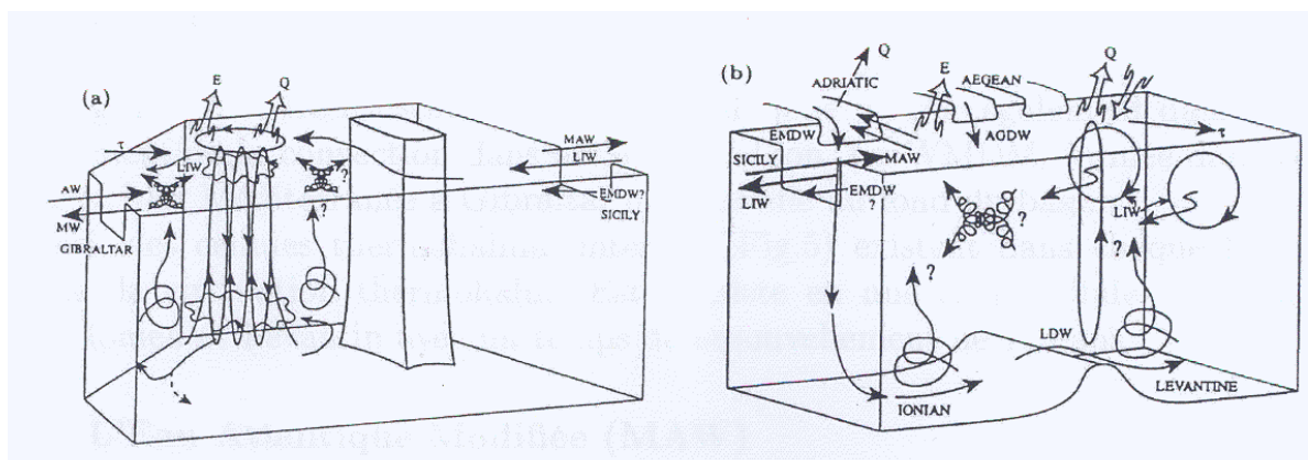
FIG. 1.3 – Schéma de la mer Méditerranée montrant la formation, le cheminement et le mélange des différentes masses d'eau en Méditerranée. Figure extraite de Robinson et al. (2001) avec E l'évaporation, Q le flux net de chaleur et \tau la tension de vent.
