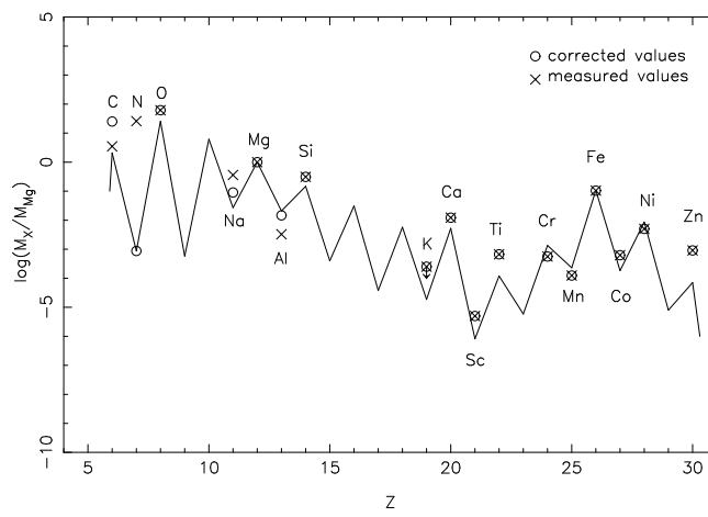
FIG. 4.22 – Rapport logarithmique des masses des éléments par rapport au magnésium. Comparaison des valeurs mesurées dans CS 22949–037 aux valeurs prédites par Woosley et Weaver (1995) modifiées par Heger et Woosley (2002). Les mesures d’abondances sont corrigées d’effets hors-ETL (Na et Al) et de mélanges internes (C et N).
