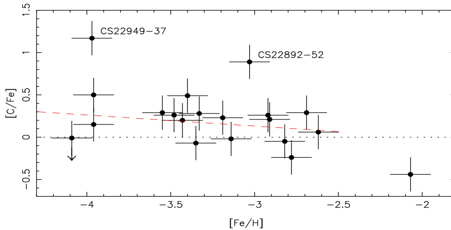
FIG. 4.5 – Évolution de l’abondance du carbone en fonction de la température. L’étoile la plus déficiente n’a qu’une limite supérieurs en carbone.
