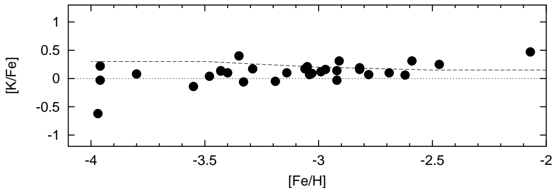
FIG. 5.9 – Évolution de l'abondance du potassium avec la métallicité. Les • sont nos mesures, corrigées des effets hors ETL, les + celles de Johnson (2002), la courbe en tirets représente les prédictions de Goswami et Prantzos (2000).
