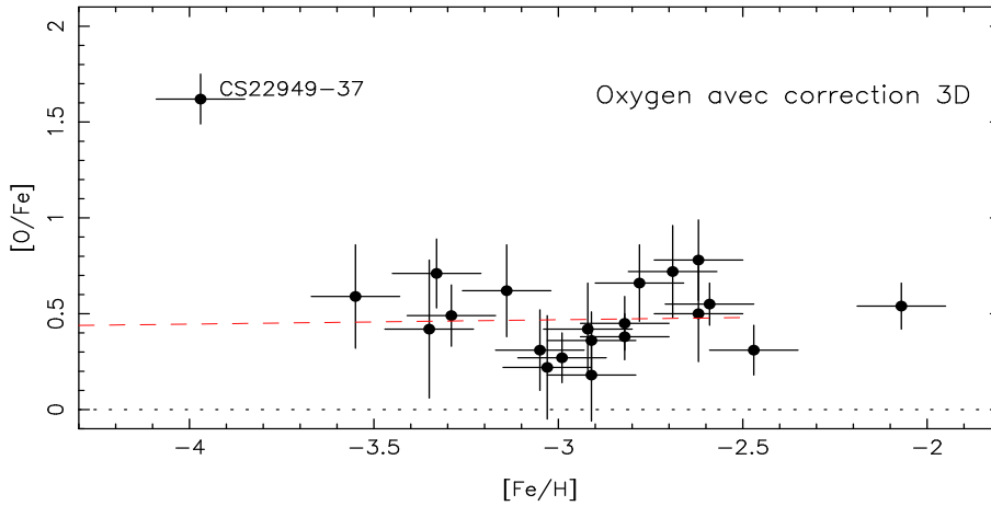
FIG. 4.7 – Évolution de l'abondance de l'oxygène en fonction de la métallicité avec les corrections 3D dans les modèles. L'abondance de CS 22949-037 est discutée à la section 4.6 page 58.
