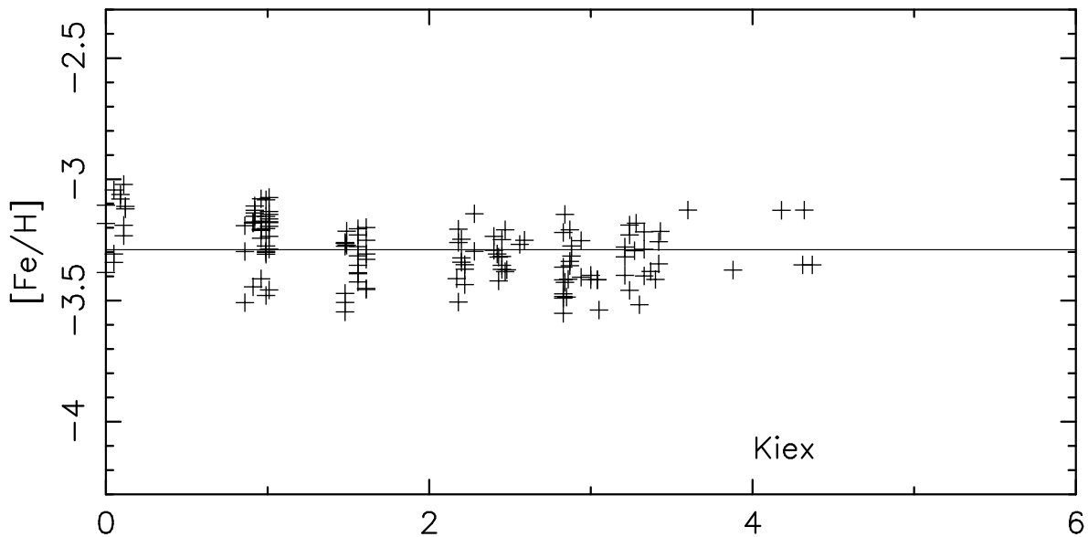
FIG. 3.1 – Étude de l’abondance en fer ( raies de Fe I) en fonction du potentiel d’excitation des raies mesurées dans l’étoile CS 22878–101. Le rapport [Fe/H] devrait être indépendant de la raie choisie, quel que soit le potentiel d’excitation de celle-ci. On remarque en général que les raies à très faible potentiel d’excitation donnent une valeur légèrement supérieure. Cela peut s’interpréter par une plus grande sensibilité de ces raies aux écarts à l’ETL.
