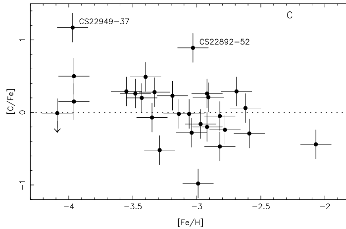
FIG. 4.1 – Abondance du carbone dans les étoiles géantes de notre échantillon. L'abscisse est le rapport de l'abondance du fer Fe/H rapporté à l'abondance solaire. L'ordonnée est le rapport des abondances du carbone et du fer, rapporté au rapport solaire. Les deux coordonnées sont en échelles logarithmiques. L'amplitude des barres d'erreurs représente l'erreur totale du [Fe/H] et [C/Fe]
