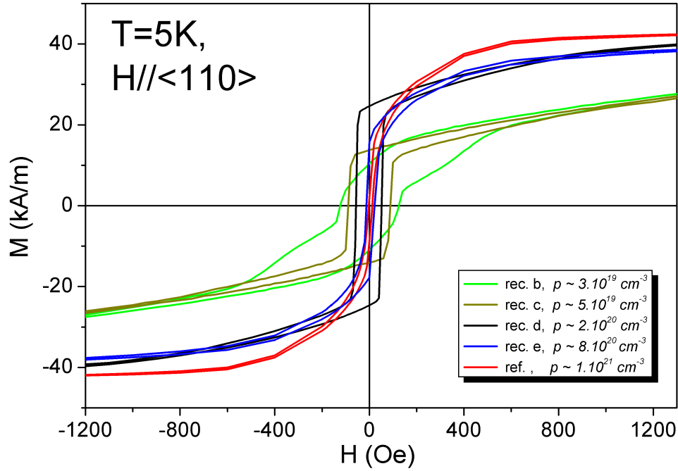
FIG. II.13 – Cycles d'hystérésis obtenus à T=5\text{ K} en magnéto-métrie SQUID avec le champ magnétique le long des axes cristallo-graphiques. Les densités de porteurs indiquées sont celles trouvées par effet Hall à haut champ.
