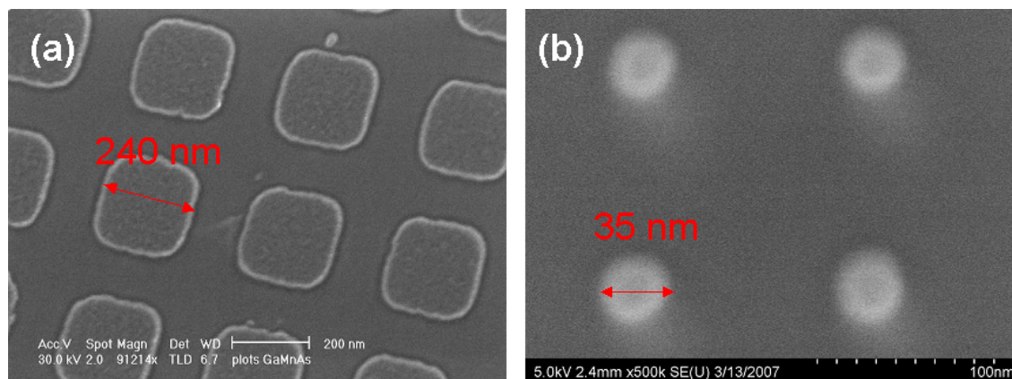
FIG. III.9 – Images MEB de plots de (\text{Ga},\text{Mn})\text{As} réalisés par gravure (N. Vernier et E. Cambril) : (a) Plots de 240 nm (dimension nominale : 200 nm). (b) Plots de 35 nm (dimension nominale : 20 nm).
