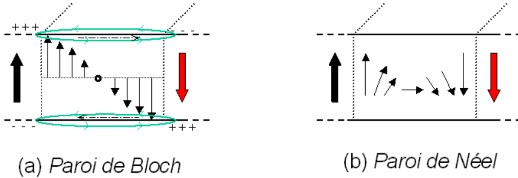
FIG. I.3 – Pour un film à forte anisotropie uniaxiale, la paroi de "Néel" (b) sera défavorable par rapport à une configuration de type "Bloch" (a). L'aimantation tourne alors parallèlement à la paroi, en envoyant les lignes de champ démagnétisant à l'infini, dans l'épaisseur de la couche. On parle de "paroi à 180°" entre deux domaines d'aimantation opposée. Un faible champ démagnétisant apparaît néanmoins aux extrémités de la paroi de Bloch, la transformant localement en paroi de Néel [98].
