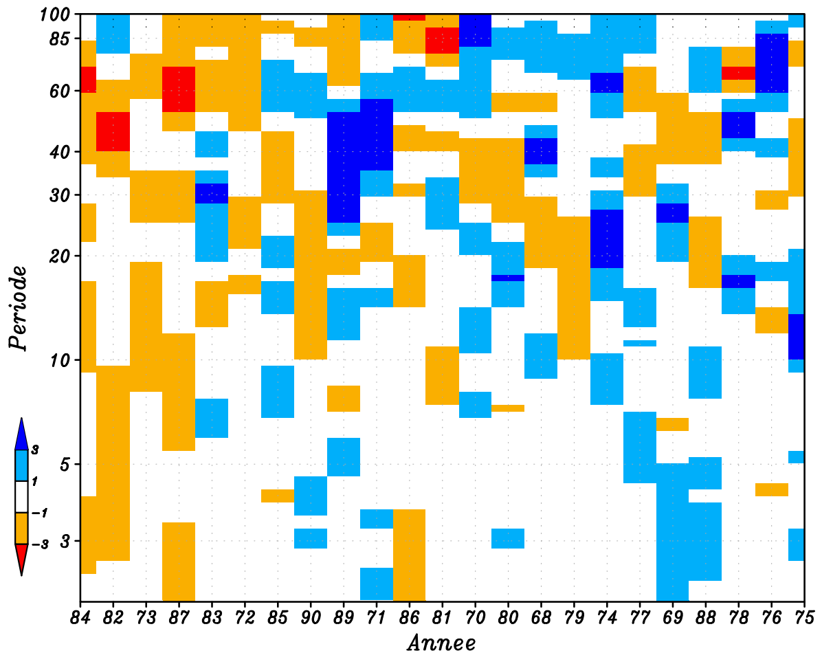
FIG. 6.6: Anomalies des densités spectrales moyennes des précipitations sur le point de grille de Niamey. Les années sont classées par ordre croissant de cumul annuel, et précisées sur l'axe des abscisses.
