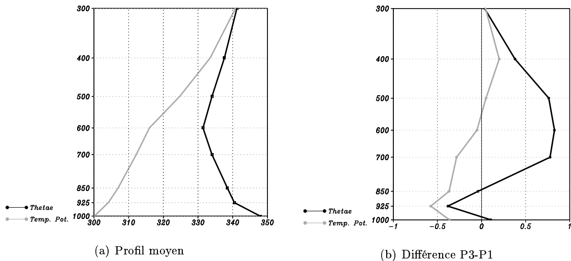
FIG. 9.14: Profil vertical de la température potentielle équivalente moyenne ( \theta_e , en ^{\circ}\text{K} ) ( noir ) et de la température potentielle ( \theta , en ^{\circ}\text{K} ) ( gris ) sur la maille de Niamey, (a) . Anomalie de \theta_e ( noir ) et de \theta ( gris ) lors du renforcement des précipitations (P3-P1), (b) .
