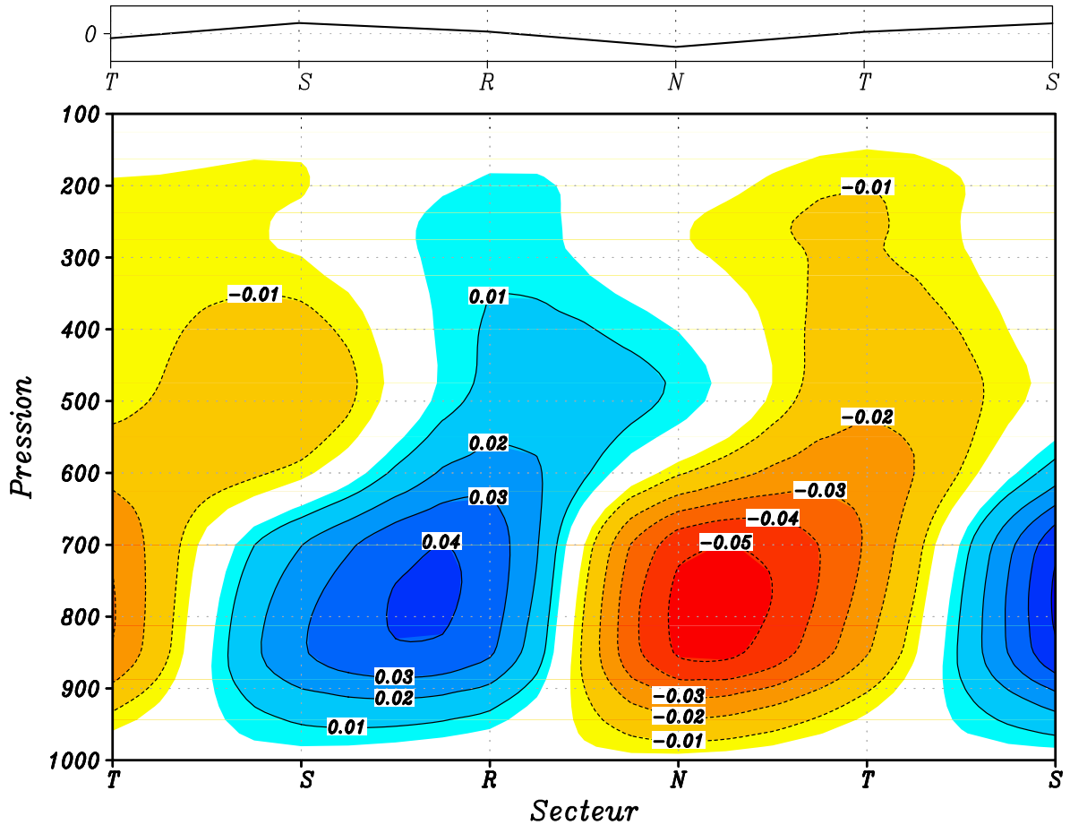
FIG. 9.7: Profil vertical des vitesses verticales suivant les secteurs sur la maille de Niamey (en Pa \cdot s^{-1} ). Les secteurs sont identifiés par le vent meridien ( haut )
