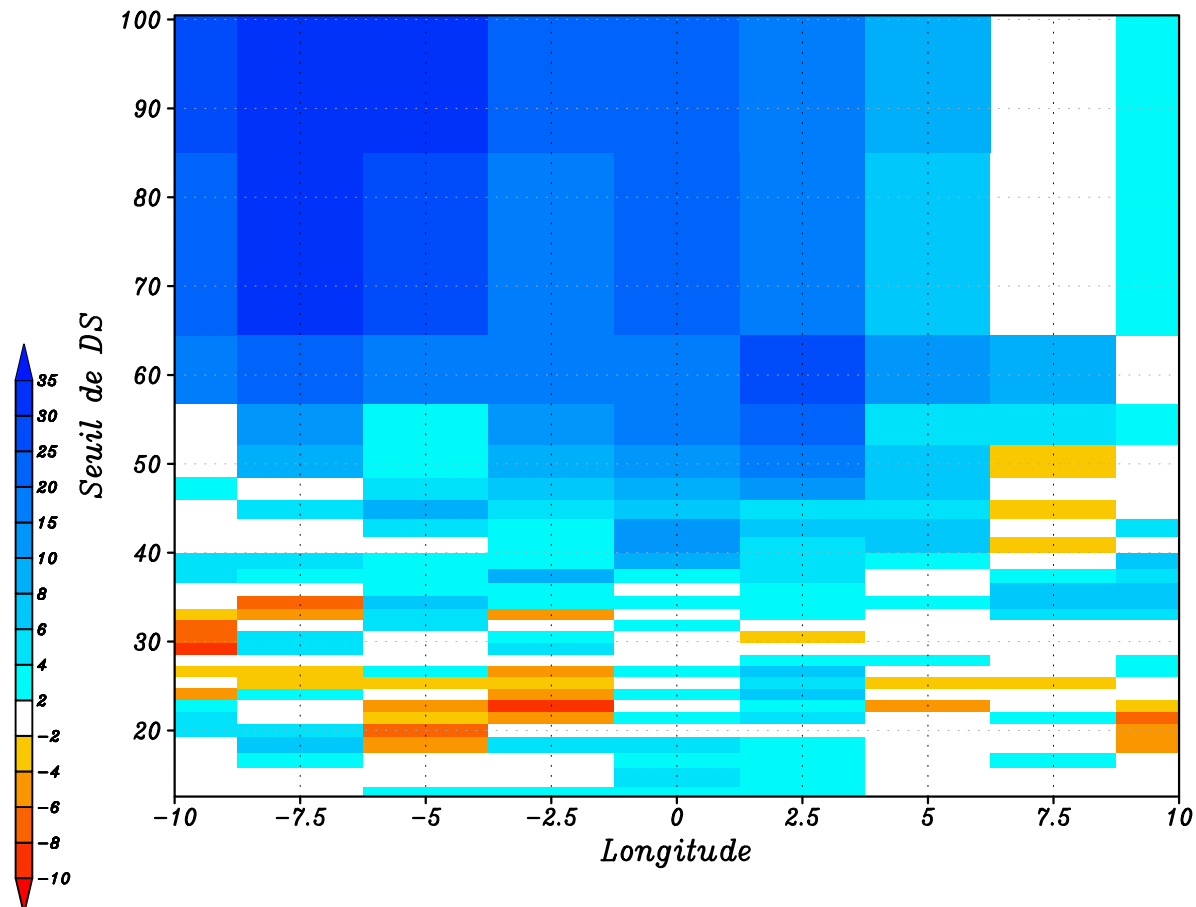
FIG. 8.6: Distribution longitudinale, entre 10°Ouest et 10°Est, de la différence de contribution (en %) du cumul des P3 entre les secteurs propices et les secteurs inhibiteurs.
