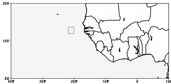
(a) Référence de J_0 à 20^\circ Ouest
