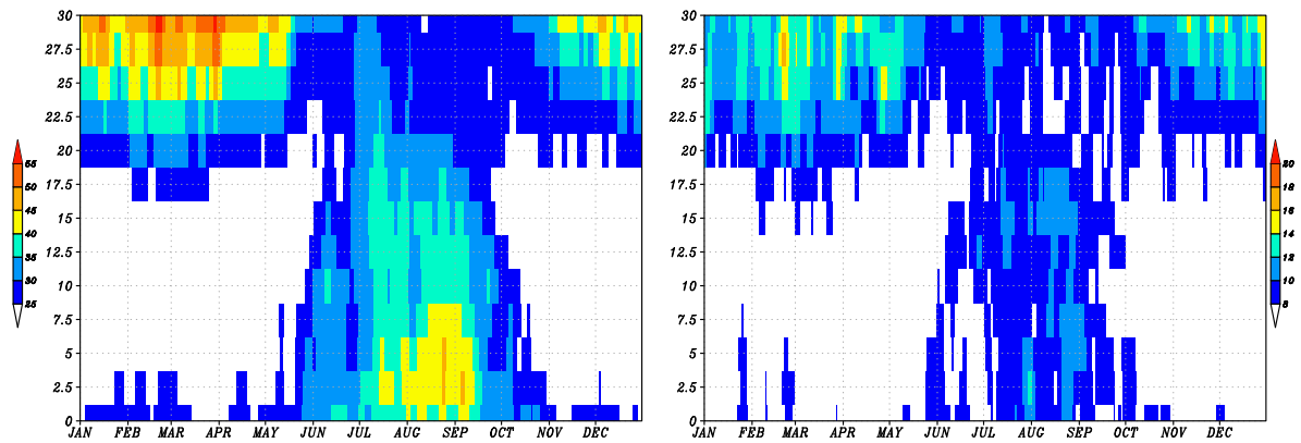
FIG. 5.3: Évolution entre 0^{\circ} et 30^{\circ} Nord, de l'indice DS détectée à 700 hPa et moyennée sur [10^{\circ}\text{W};10^{\circ}\text{E}] et dans la période 1968-1990 (a), en m^2.s^{-2} , idem pour l'écart type de DS (b).
