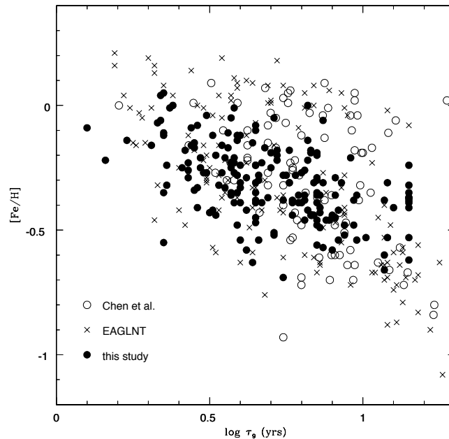
FIG. 1.8 – Relation âge-métallicité dans le disque mince d’après Reddy et al. (2003)
