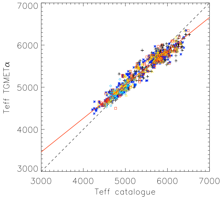
FIG. 3.3 – T_{\text{eff}} de \text{TGMET}\alpha en fonction de T_{\text{eff}} de la littérature. “Plus”: Soubiran & Girard (2005): +, Ramírez & Meléndez (2005): *, Blackwell & Lynas-Gray (1998): \Delta , Di Benedetto (1998): \square , Mishenina et al. (2006): \diamond .
