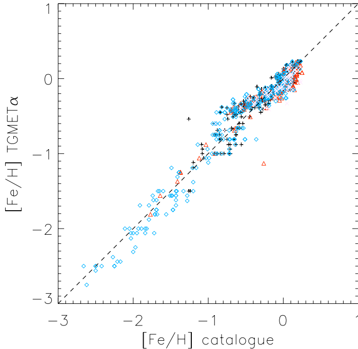
FIG. 3.5 – [Fe/H] de TGMET\alpha en fonction de [Fe/H] de la littérature. Les auteurs sont indiqués avec des symboles différents, Soubiran & Girard (2005): +, Mishenina et al. (2006): ◇, Heiter & Luck (2003): ×, Valenti & Fischer (2005): △.
