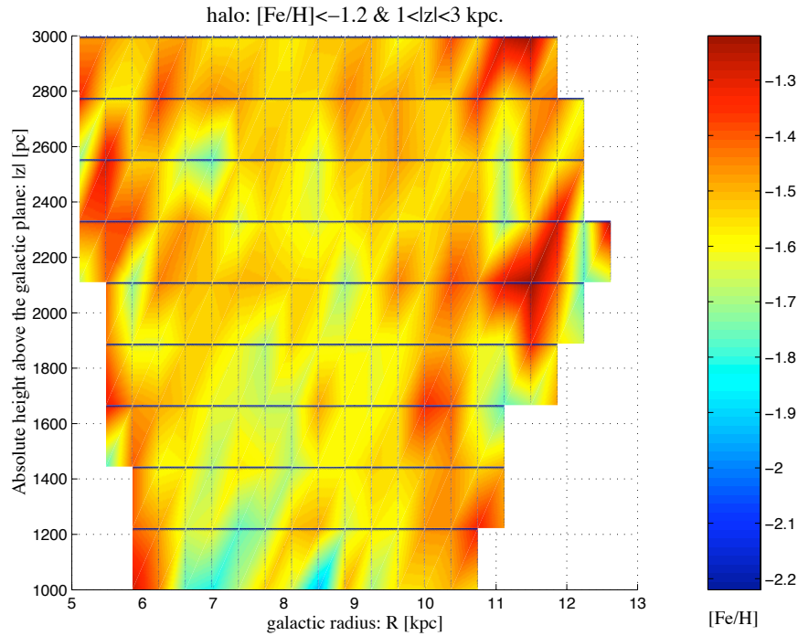
FIG. 4.14 – Distribution de [\text{Fe}/\text{H}] en fonction de |z| (par intervalles de \sim 200 pc) et R (par intervalles de \sim 0.5 kpc) pour l'échantillon du halo.
