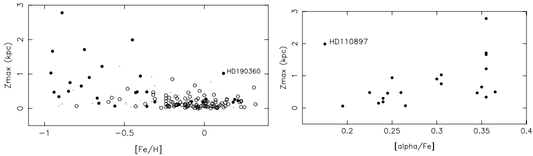
FIG. 1.13 – Z_{\text{max}} en fonction de [\text{Fe}/\text{H}] (à gauche) et de [\alpha/\text{Fe}] (à droite) d’après Mishenina et al. (2004). Les symboles sont les mêmes que ceux de la figure 1.12
