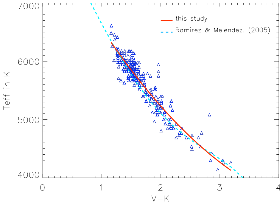
FIG. 3.4 – T_{\text{eff}} de TGMET\alpha , corrigé, en fonction de l'indice V-K . L'ajustement avec un polynôme de degré 2 est représenté par une courbe en trait plein. La relation pour les étoiles naines donnée by Ramirez & Melendez (2005) est représentée avec une courbe en pointillée.
