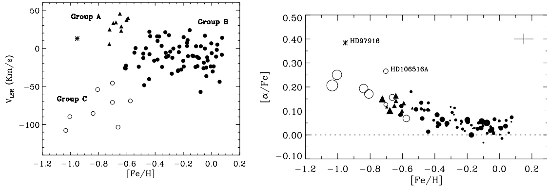
FIG. 1.4 – V_{LSR} et [alpha/Fe] en fonction de [Fe/H] pour l'échantillon de Chen et al. (2000). Les différents symboles représentent les différents groupes d'étoiles. Le groupe C est le groupe d'étoiles du disque épais. L'astérisque correspond à une étoile du halo. La taille des symboles sur la figure de droite est proportionnelle à l'âge des étoiles.
