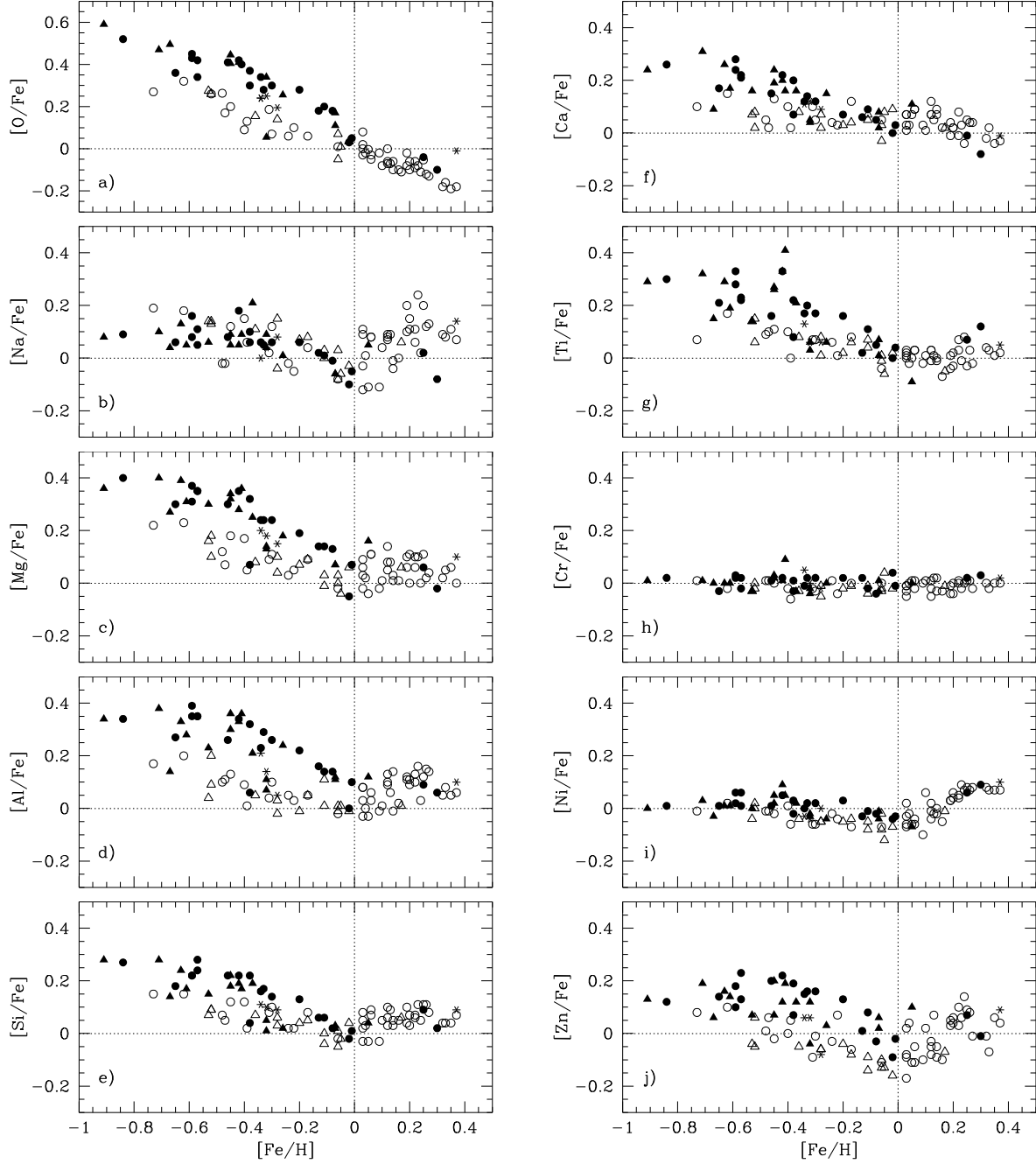
FIG. 1.9 – [X/Fe] en fonction de [Fe/H] d'après Bensby et al. (2005). Les symboles vides sont les étoiles appartenant au disque mince, les symboles noirs au disque épais et les astérisques sont des objets de transitions.
