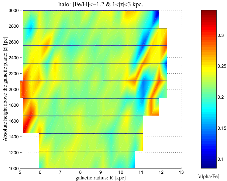
FIG. 4.12 – Distribution de [\alpha/\text{Fe}] en fonction de |z| (par intervalles de \sim 200 pc) et R (par intervalles de \sim 0.5 kpc) pour l'échantillon du halo.
