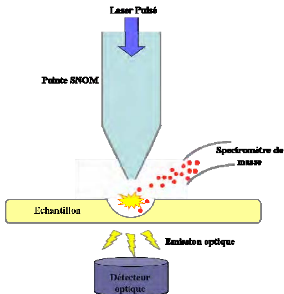
Figure 2.5 : Schéma du SNOM
