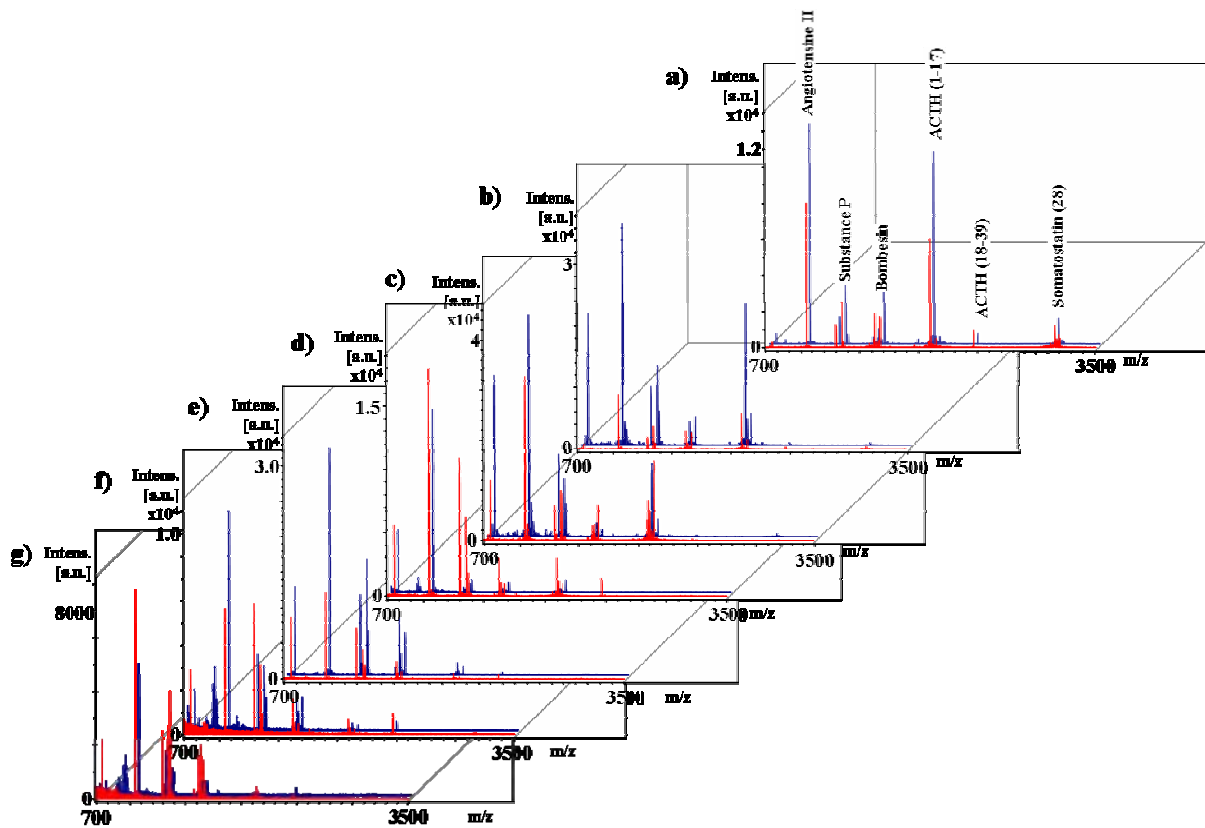
Figure 5.6 : Comparaison de la sensibilité entre lame Ni 10 (rouge) et lame ITO (bleu) pour des concentrations de 4 \mu M, 1 \mu M, 0,4 \mu M, 0,1 \mu M, 4nM, 1nM, 0,4nM (respectivement a), b), c), d), e), f) et g))
