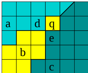
FIG. 4.2 –: Erreur de la transformée de DANIELSSON sur un voisinage en 4–connexité (algorithme 4SED de DANIELSSON 1980.) : les points a, b et c sont des points du complémentaire et q, d et e des points de l’objet. Lors de la propagation en 4–connexité, d est plus proche de a que de b, c et e est plus proche de c, q sera noté “plus proche de a ou de c” alors que le résultat exact serait b.
