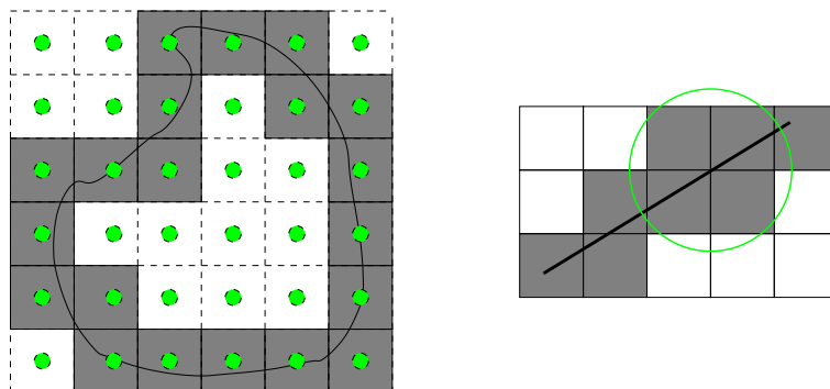
FIG. 1.11 —: Discretisation par supercouvertures : (gauche) discrétisation d'une courbe quelconque et illustration d'une bulle pour la discrétisation d'une droite.
