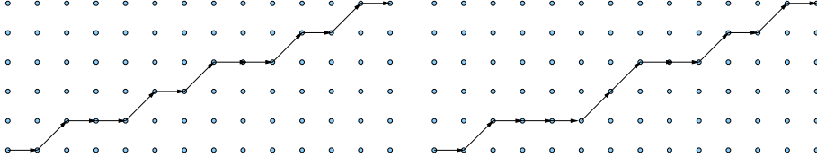
FIG. 2.3 – : Propriété de FREEMAN : (gauche) le codage est 0 - 1 - 0 - 0 - 1 - 0 - 1 - 0 - 0 - 1 - 0 - 1 - 0 , les codes “1” apparaissent isolés et uniformément répartis ; (droite), le codage est 0 - 1 - 0 - 0 - 0 - 1 - 1 - 0 - 0 - 1 - 0 - 1 - 0 , dans ce cas, ni le code “0” ni le code “1” sont isolés, cet arc n’est pas un segment discret.
