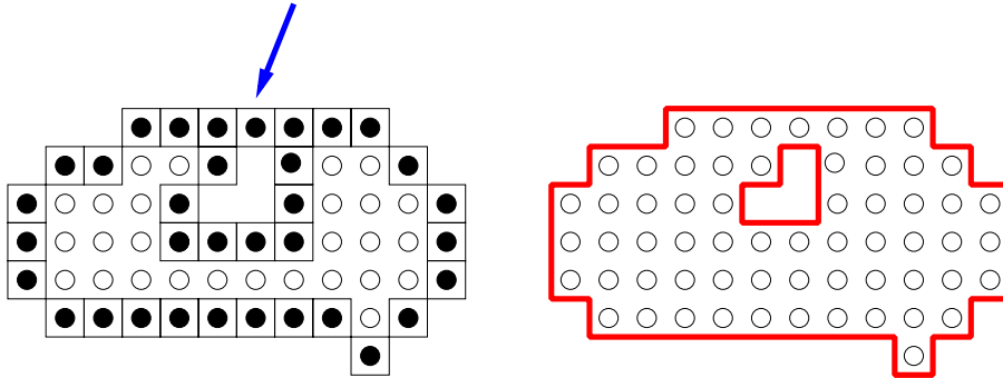
FIG. 1.5 – : Défaut de la notion de bord en tant qu'ensemble de points discrets (points noirs à gauche) et surface de lignels basée sur une approche cellulaire (polygones en gras à droite).
