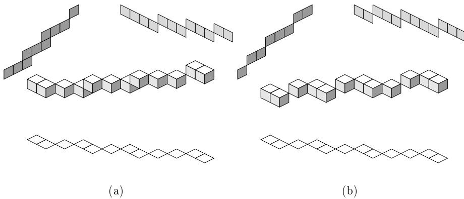
FIG. 2.23 –: Droites discrètes 3D 26-connexes : (a) droite naïve \mathcal{D}_{3D}(10, 7, 3, 0, 0, 0) et (b) droite naïve \mathcal{D}_{3D}(10, 7, 3, -5, 0, 0) (DEBLED-RENNESON, 1995).
