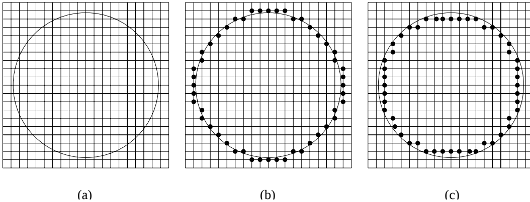
FIG. 3.1 — Discretisation de cercles euclidiens : (a) cercle euclidien superposé sur une grille discrète, (b) discrétisation GIQ de NAKAMURA et AIZAWA et (c) discrétisation de KIM.
