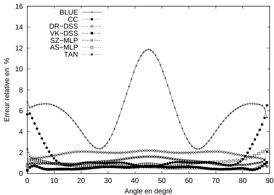
FIG. 5.25 —: Erreur relative sur un carré de taille fixe sur lequel une rotation est effectuée : en abscisse se trouve l'angle de rotation entre 0 et 90 degrés et en ordonnée, l'erreur relative des différents estimateurs.
