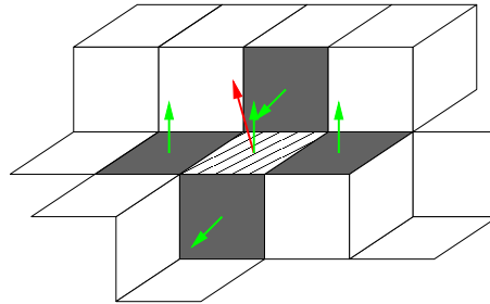
FIG. 5.11 – : Approche de CHEN ET AL. (1985) pour l'estimation de la normale basée sur une décomposition cellulaire de la surface discrète.
