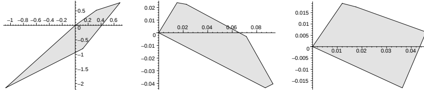
FIG. 3.14 —: Exemples d'évolution de l'acd sur un cercle de rayon 100 quand on considère un nombre croissant d'arêtes de \Gamma .
