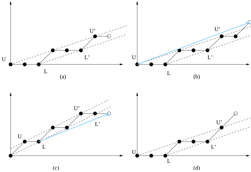
FIG. 2.19 —: Différents cas de figure lors de l'ajout d'un point à une droite discrète : (a) ajout d'un point ne changeant pas les paramètres, (b) ajout d'un point faiblement extérieur supérieur, dans ce cas le vecteur clair indique les nouveaux paramètres du segment discret, (c) ajout d'un point faiblement extérieur inférieur, le vecteur clair indique toujours le nouveau paramétrage de la courbe et (d) ajout d'un point fortement extérieur et mise en échec de la reconnaissance.
