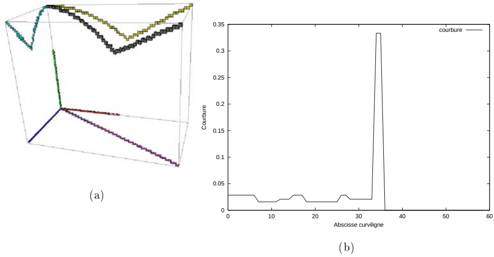
FIG. 5.43 —: Exemple de calcul de courbure sur une courbe discrète 3D avec une estimation du cercle osculateur : (a) courbe discrète 26-connexe composée d'un arc de cercle et d'un segment de droite discrète 3D, (b) graphe de courbure obtenu.
