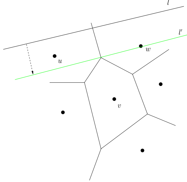
FIG. 4.7 – : Illustration de la preuve : C_v n'intersecte pas l et on calcule une paire de sites cachant v en translatant la droite l vers un sommet de C_v . Les sites adjacents à ce sommet du diagramme sont solutions du problème.
