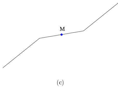
FIG. 2.46 –: Illustration du test statistique : (a) exemple où le segment central est plus petit (25 pixels avec les mêmes paramètres) que dans la figure 2.45, (b) cas pathologique où les segments à l'extrémité ont la même loi et où M est au milieu du segment central ; (c) illustration géométrique de ce cas pathologique.
