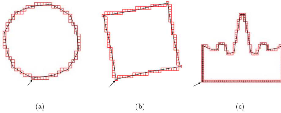
FIG. 2.21 –: Exemples de segmentation d'une courbe discrète en droites discrètes avec l'algorithme de DEBLED-RENNESON et REVEILLÈS (1995) : la courbe polygonale noire correspond au résultat de la segmentation et la flèche indique le point départ, (a) un cercle discret, (b) un carré avec une rotation de 10 degrés et (c) sur une courbe construite par une fonction sinus cardinale.
