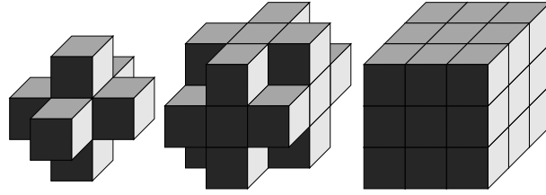
FIG. 1.3 –: Différentes connexités en 3D sur un pavage par cubes.
