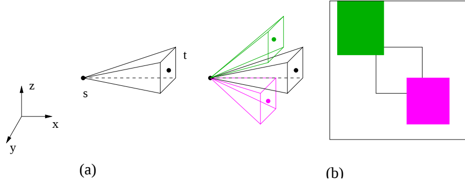
FIG. 4.38 —: Illustration de la visibilité restreinte en 3D : (a) domaines de visibilité restreinte dans l'espace primal et (b) illustration du test de visibilité par projection dans le plan (Oyz) contenant t des carrés associés aux voxels bloquants.
