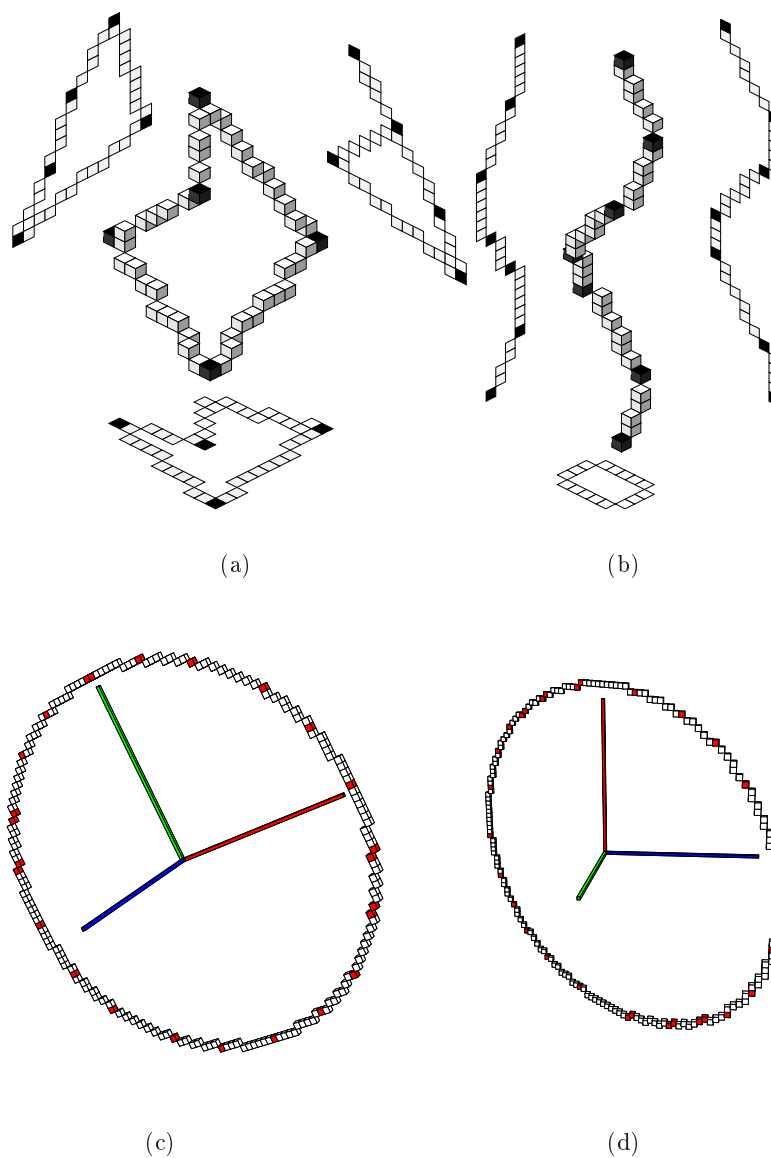
FIG. 2.25 – : Exemples de segmentation de courbes 26-connexes en segments de droite naïve 3D : les voxels sombres correspondent aux sommets de la segmentation, (a) et (b) courbes 26-connexes synthétiques, (c) segmentation d'un cercle 3D et (d) segmentation d'une ellipse 3D (DEBLED-RENNESON, 1995; COEURJOLLY ET AL., 2001a)
