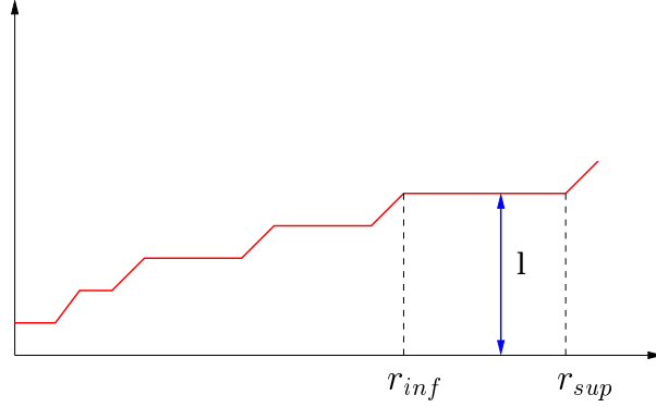
FIG. 5.38 –: Illustration de la première parabole des cercles arithmétiques et calcul de l'ensemble des cercles de hauteur l .
