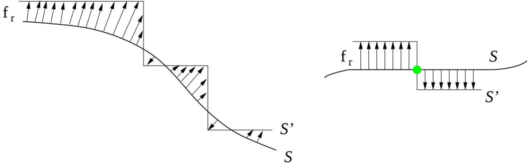
FIG. B.5 – : Illustration de la construction de f_r dans le cas 2D : à gauche une courbe continue \mathcal{S} et sa discrétisation \mathcal{S}' avec la fonction f_r . À droite, présentation d'un cas pathologique : \mathcal{S} est orthogonale à \mathcal{S}' .
