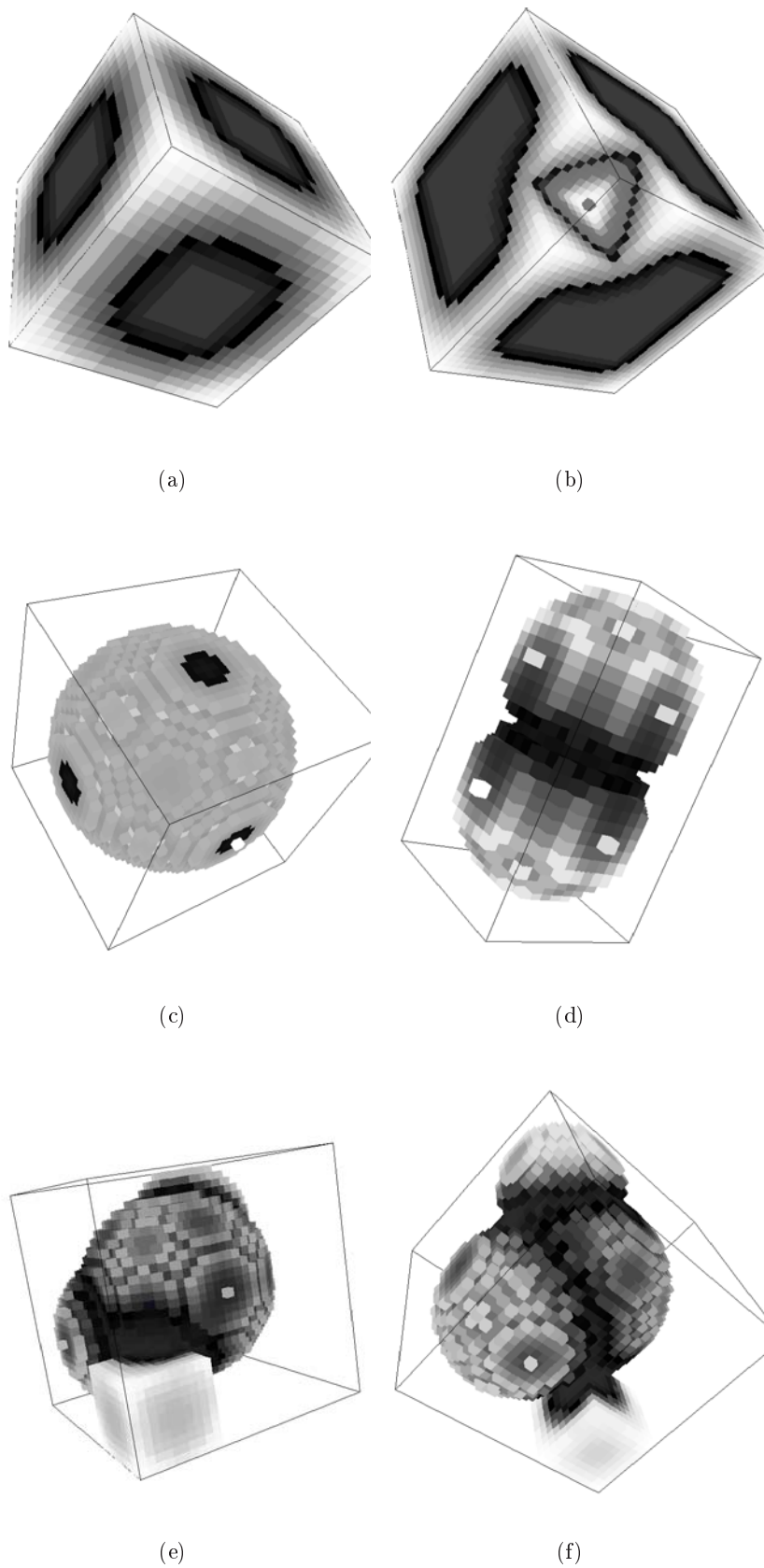
FIG. 5.45 – : Exemples de calcul de courbure moyenne avec l'estimateur de BULLARD ET AL. (1995) : (a) sur un cube discret, (b) sur un cube dont un coin est chanfreiné, (c) sur une sphère discrète, (d) sur un objet composé de deux sphères connexes et (e) – (f) sur un objet composite.
