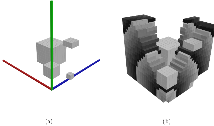
FIG. 4.39 —: Exemple d'étiquetage en distance géodésique 3D : (a) domaine 3D défini par les obstacles gris et (b), étiquetage en distance géodésique de la première classe de visibilité uniquement. Le voxel source est à l'origine du repère.
