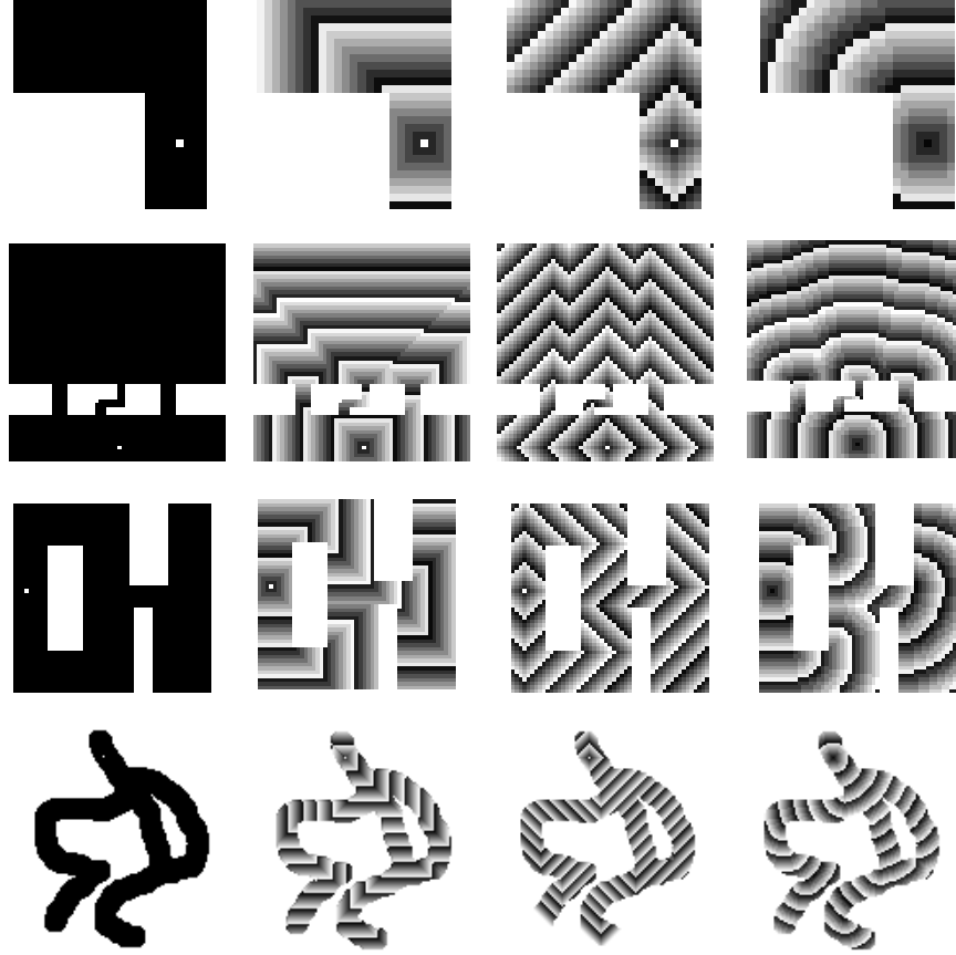
FIG. 4.35 —: Analyse expérimentale de l'étiquetage en distance géodésique : de gauche à droite, les domaines discrets et le point source (pixel blanc isolé), l'étiquetage avec la distance d_8 , avec la distance d_4 et enfin avec la distance géodésique proposée.
