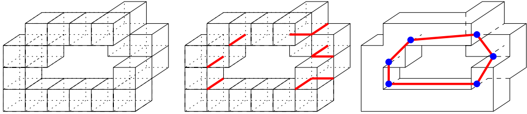
FIG. 5.27 — : Illustration du calcul du polygone de longueur minimale associé à une courbe discrète 6-connexe : courbe discrète initiale, sélection des arêtes critiques et calcul du polygone de longueur minimale.
