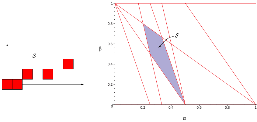
FIG. 2.11 –: Ensemble de pixels S et domaine des droites euclidiennes y = \alpha x + \beta associées, noté \tilde{S} .
