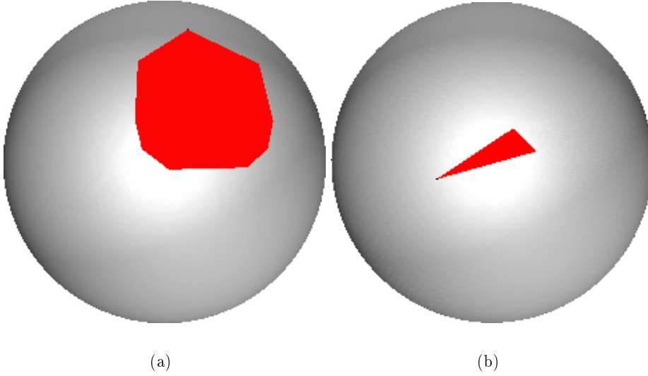
FIG. 5.49 –: Exemples de calcul d'enveloppes convexes sphériques : (a) représentation sur la sphère unité du polygone obtenu sur un voisinage v provenant d'une sphère discrète et (b) provenant d'un morceau de cylindre.
