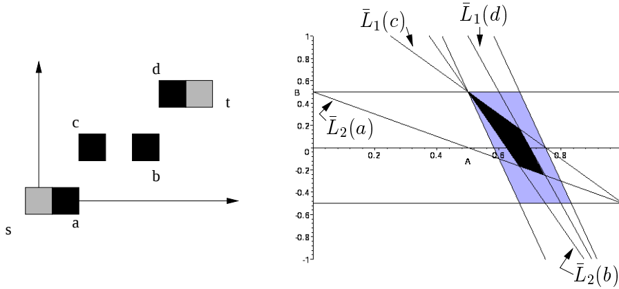
FIG. 4.32 – : Domaine de visibilité associé à un ensemble de pixels : le domaine en gris clair correspond à \mathcal{S}(s, t) et le polygone noir au domaine de visibilité associé à s , t et aux pixels bloquants a , b , c et d . Les contraintes non tracées correspondent aux contraintes n'intersectant pas \mathcal{S}(s, t) .
