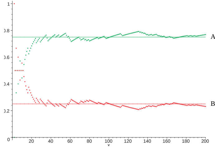
FIG. 2.42 —: Liens entre droite discrète et loi de BERNOULLI : en ordonnée se trouvent les fréquences d'apparition des codes "0" (courbe A) et "1" (courbe B) lors d'un tirage aléatoire d'un code dans le mot infini issu de la droite naïve \mathcal{D}(1, 4, 0) . L'abscisse correspond aux tirages successifs.
