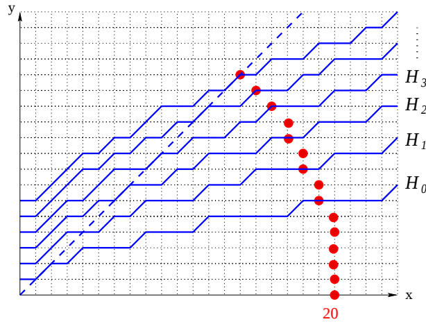
FIG. 3.3 —: Exemple de construction d'un cercle de Pitteway plancher de rayon 20.
