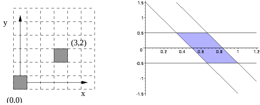
FIG. 4.31 – : Exemple de domaine \mathcal{S}(s, t) des pixels (0, 0) et (3, 2) : le domaine \mathcal{S}(s, t) est défini par les inéquations \{\beta < 1/2, \beta \geq -1/2, \beta < -3\alpha + 5/2, \beta \geq -3\alpha + 3/2\} .
