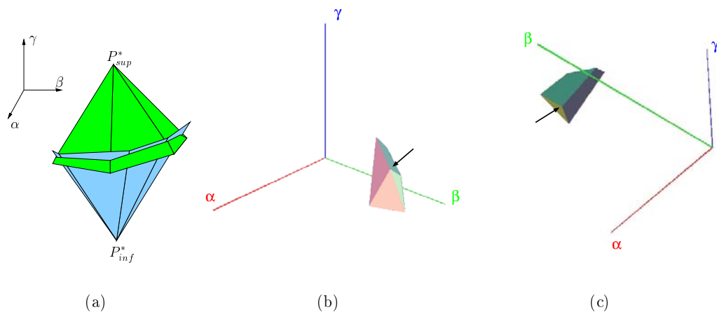
FIG. 2.37 –: Illustration du polyèdre avec la notion de double-cône : (a) illustration schématique du double-cône et (b)-(c) le polyèdre dans l'espace dual du morceau de plan P(1, 3, 4, 0) (voir figure 2.35), les flèches indiquent respectivement les sommets P_{sup}^* et P_{inf}^* .
