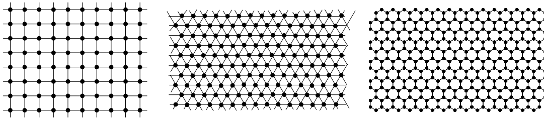
FIG. 1.2 —: Représentation duale par maillage en dimension 2.
