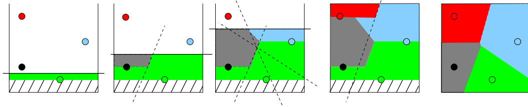
FIG. 4.6 – : Balayage de l'image en y croissant (4 premières images) avec les diagrammes de Voronoï partiels. Chaque cellule a la couleur du site auquel elle correspond, la partie hachurée correspond aux pixels non-étiquetés et les droites en pointillés sont des médiatrices entre sites.
