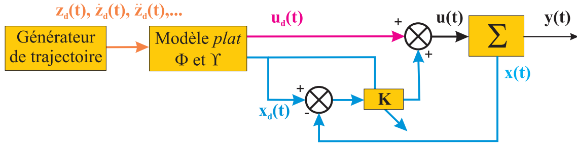
FIG. III.8 – Architecture du contrôleur en suivi de trajectoire.
