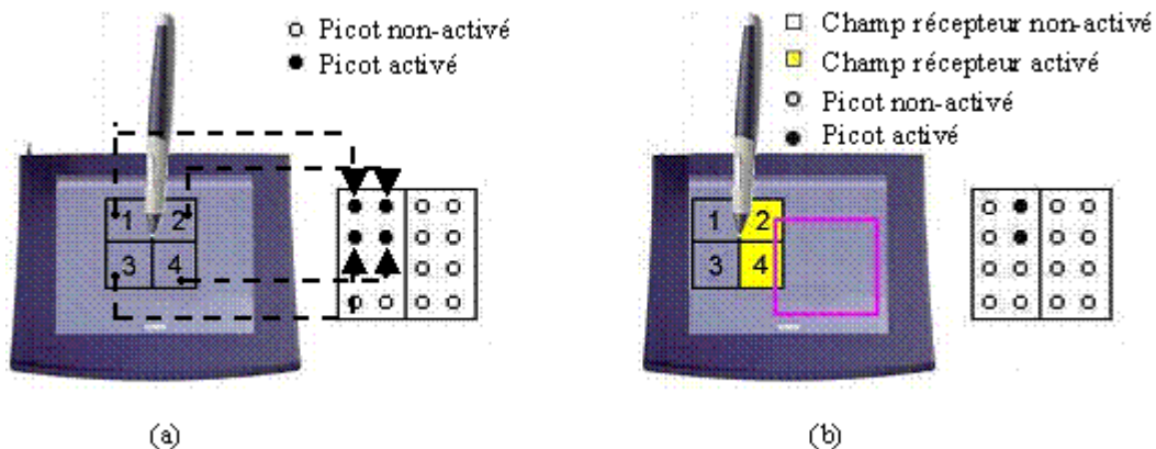
Figure 20 : a) Relation entre la matrice de champs récepteurs et la matrice de stimulateurs tactiles, b) principe du système de détection-stimulation. Schéma explicatif (d'après Sribunruangrit, 2004)
