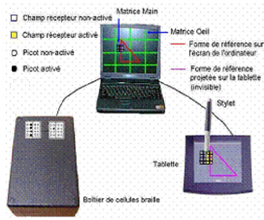
Figure 57 : Présentation du système œil-main, illustration (d'après Sribunruangrit, 2004)
