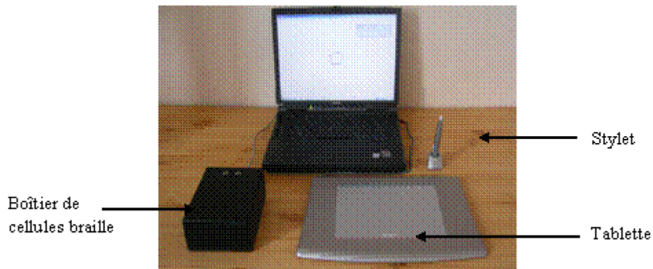
Figure 18 : Ensemble du dispositif de suppléance perceptive (version III)
