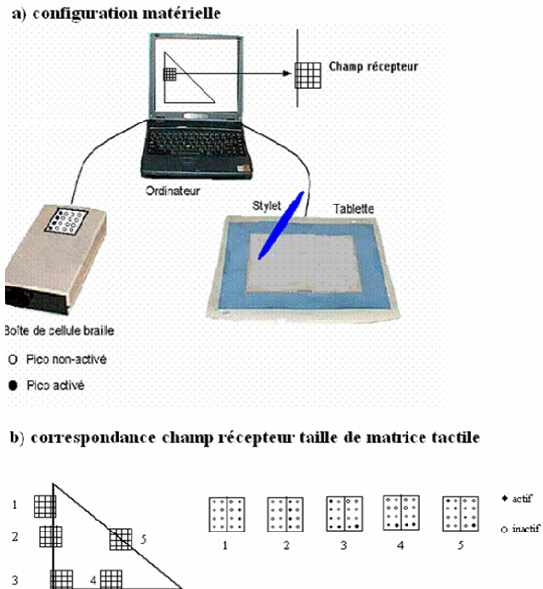
Figure 21 : Relation entre le champ récepteur et la stimulation tactile pendant l'exploration du triangle. Schéma illustratif (d'après Sribunruangrit, 2004).
