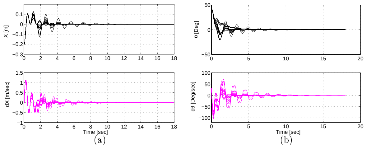
FIG. 3.28 – Application 3 (robustesse vis-à-vis des incertitudes paramétriques): position et vitesse de la coordonnée actionnée (a), position et vitesse de la coordonnée non actionnée (b)
