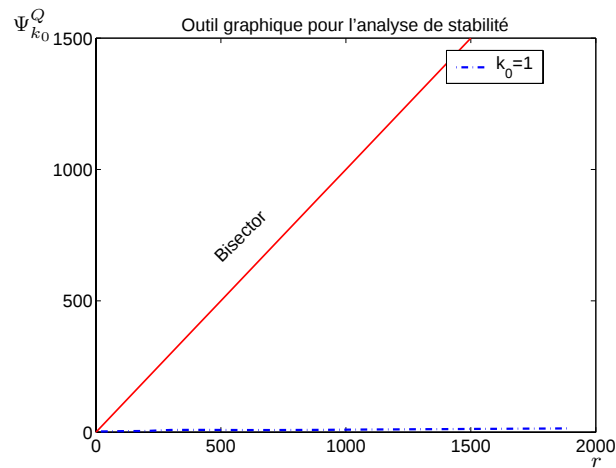
FIG. 3.35 – Application 4 (génération de cycles limites) courbe d'analyse de stabilité: les conditions suffisantes du point 2 de la proposition 1 sont vérifiées pour k_0 = 1
