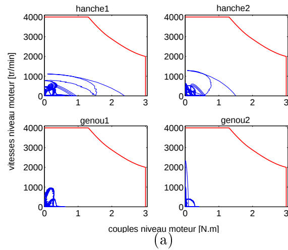
FIG. 5.60 – Approche 2 : évolution des vitesses angulaires des moteur en fonction des couples niveau moteurs, superposées au gabarit constructeur délimitant la puissance maximale
