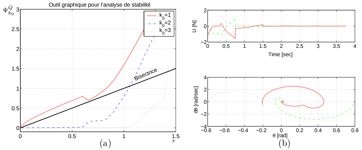
FIG. 3.26 – Application 3 (stabilisation): courbe d'analyse de stabilité (a): les conditions suffisantes de stabilité du point 1 de la proposition 1 sont vérifiées pour k_0 = 2, 3 , évolution de l'entrée de commande et plan de phase de la dynamique interne (b)
