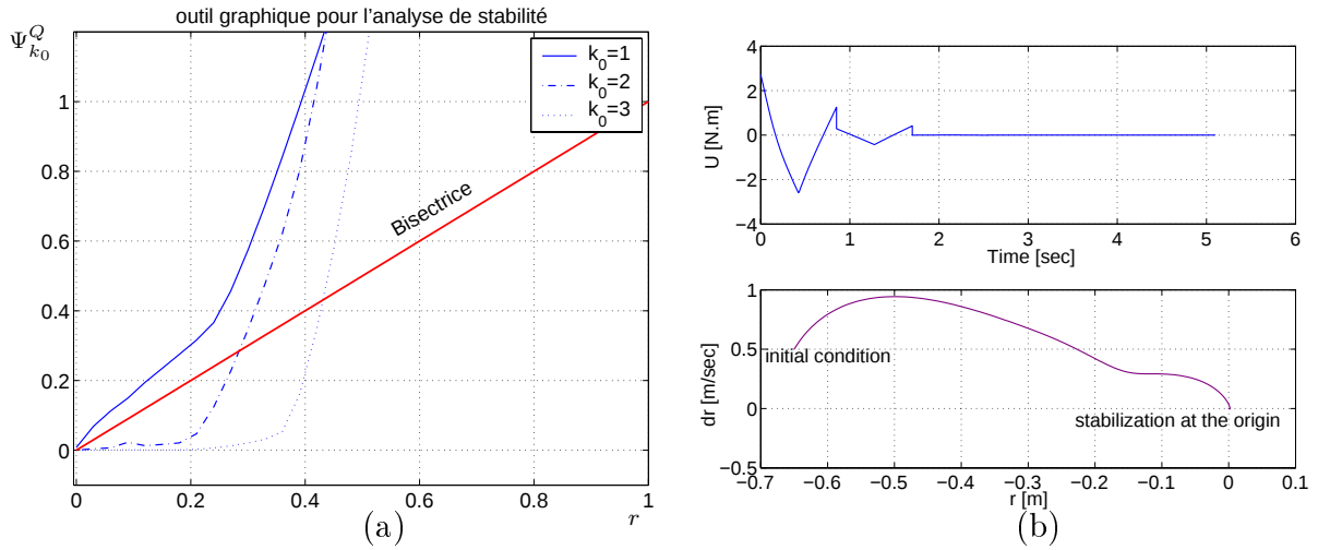
FIG. 3.16 – Application 2 (stabilisation): courbe d'analyse de stabilité: les conditions suffisantes du point 1 de la proposition 1 sont satisfaites pour k_0 = 2, 3 (a), évolution dans le temps de l'entrée de commande (b) haut, plan de phase de \eta (b) bas
