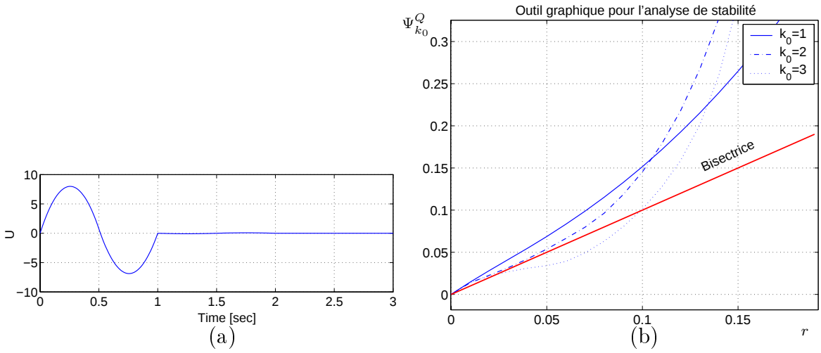
FIG. 3.8 – Application 1 (stabilisation): évolution dans le temps de l'entrée de commande (a), courbe d'analyse de stabilité (b): les conditions suffisantes du point 2 de la proposition 1 sont satisfaites pour k_0 = 3
