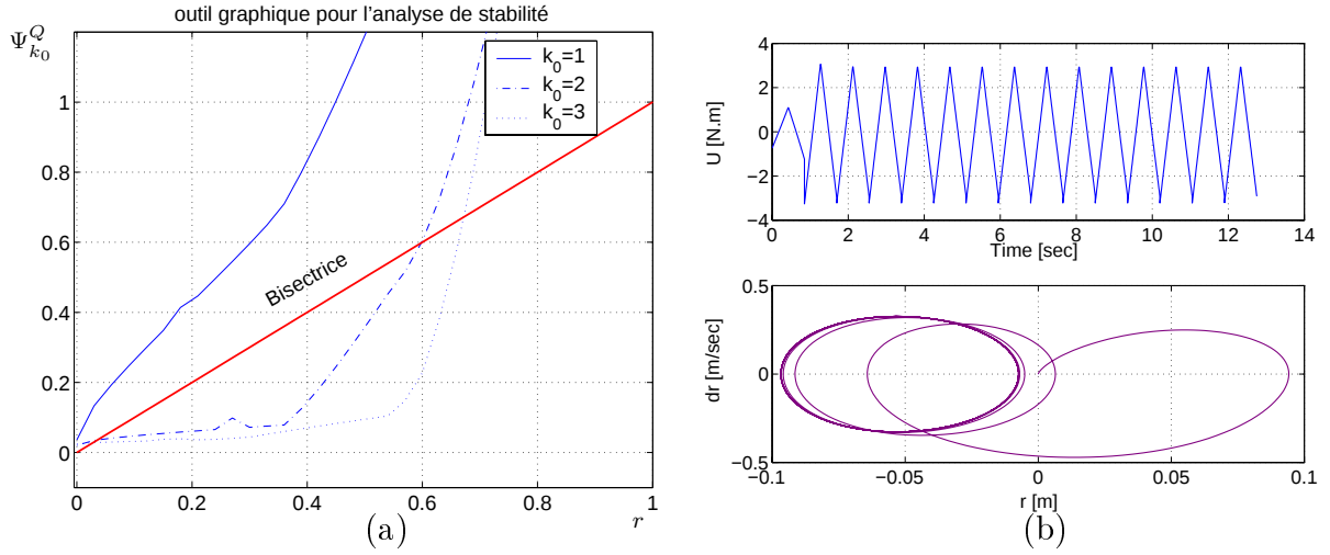
FIG. 3.19 – Application 2 (génération de cycles limites): courbe d'analyse de stabilité (a): les conditions suffisantes du point 2 de la proposition 1 sont vérifiées pour k_0 = 2,3 , évolution de l'entrée de commande (b) haut, plan de phase de \eta (b) bas
