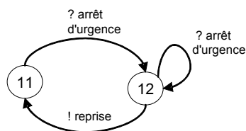
figure 1.14 Représentations de l'arrêt d'urgence et de la reprise
