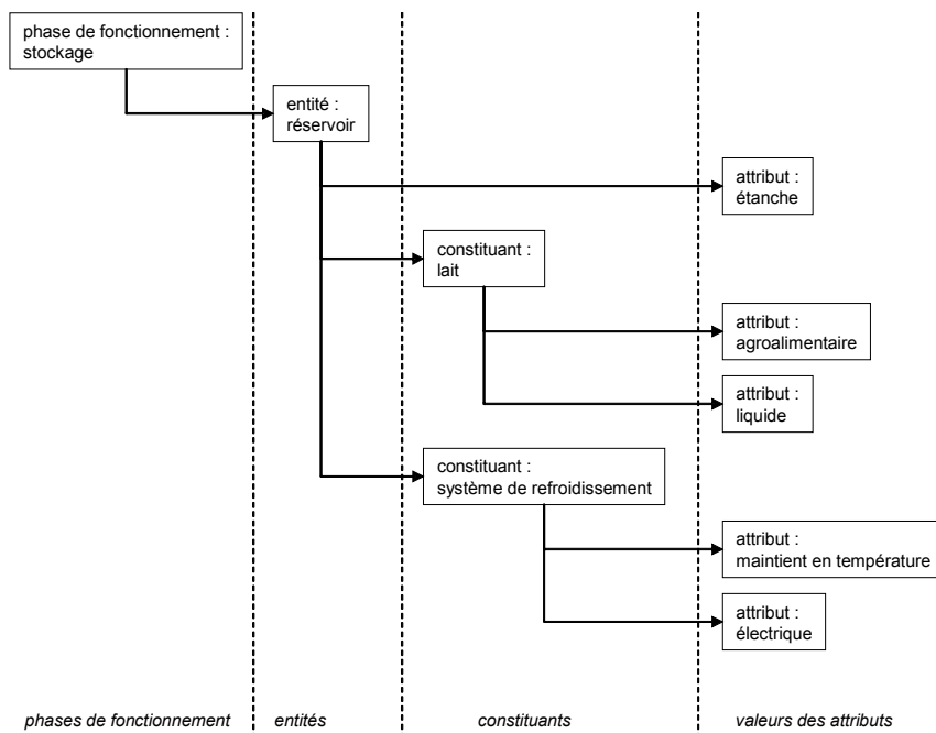
figure 2.24 Exemple : détail de la phase de fonctionnement stockage
