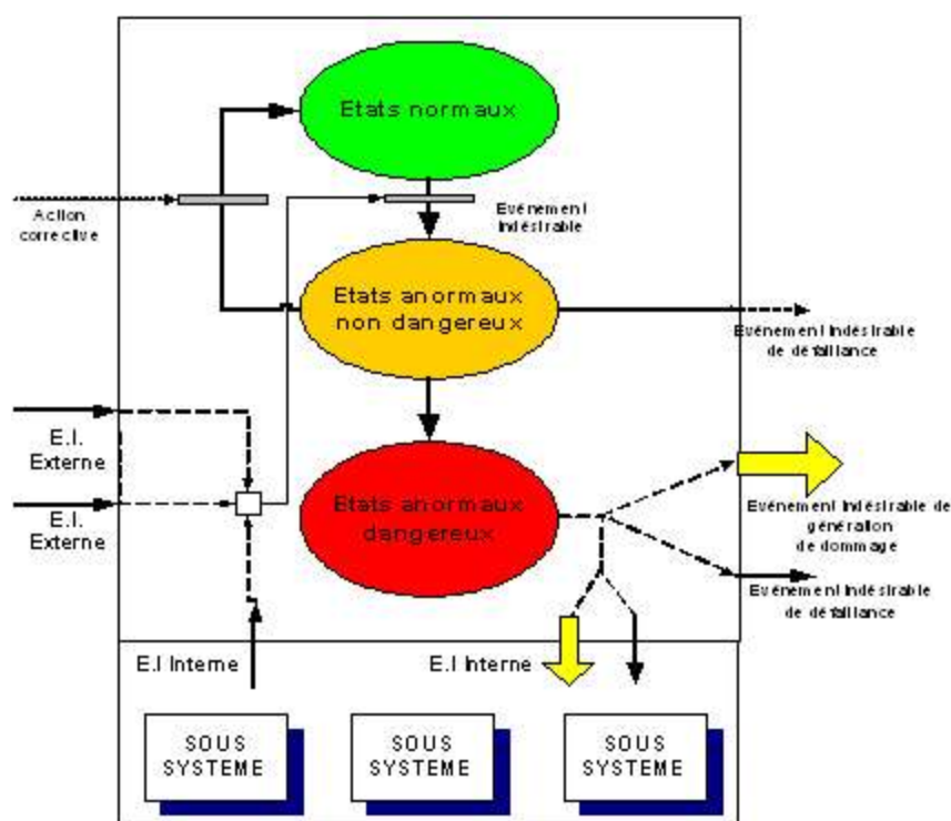
figure 1.4 Modèle dysfonctionnement d'une entité [Flaus 2003]
