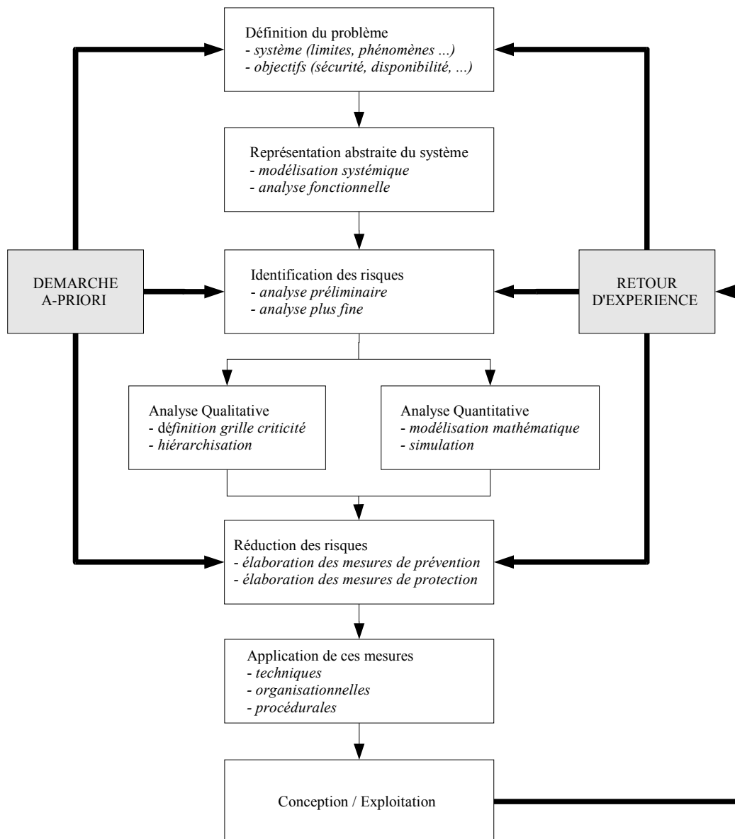
figure 1.6 Démarche d'analyse des risques [PRIHSE 2002]
