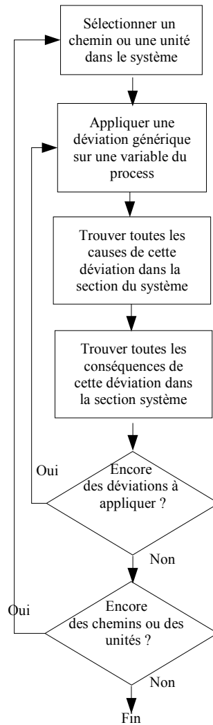
figure 1.8 Principe d'analyse de l'HAZOP
