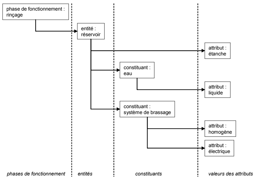
figure 2.26 Exemple : détail de la phase de fonctionnement rinçage
