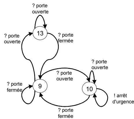
figure 1.15 Contacteur de la porte avec les états de défaillances
