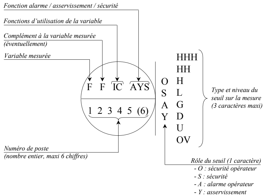
figure A2 Organe de mesure
