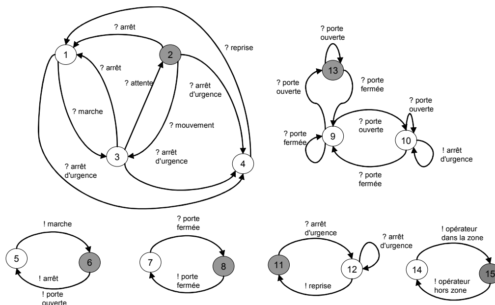
figure 1.17 Etat dangereux de l'installation
