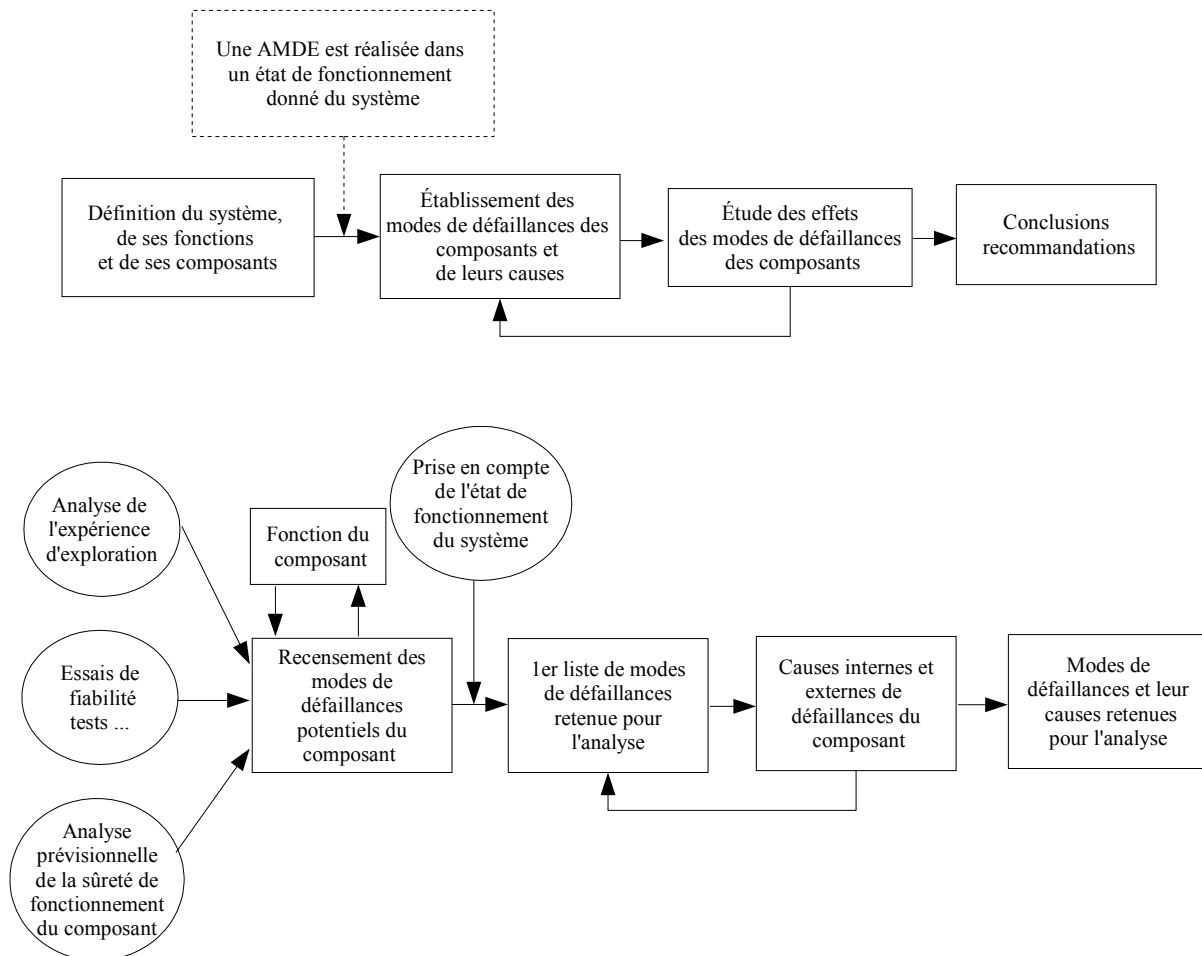
figure 1.7 Méthode de réalisation d'une AMDE [Villemeur 1988]
