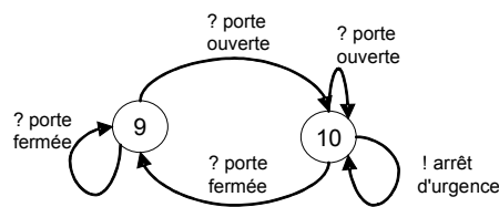
figure 1.13 Représentation du contacteur de la porte
