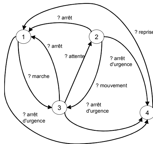
figure 1.10 Représentation du robot
