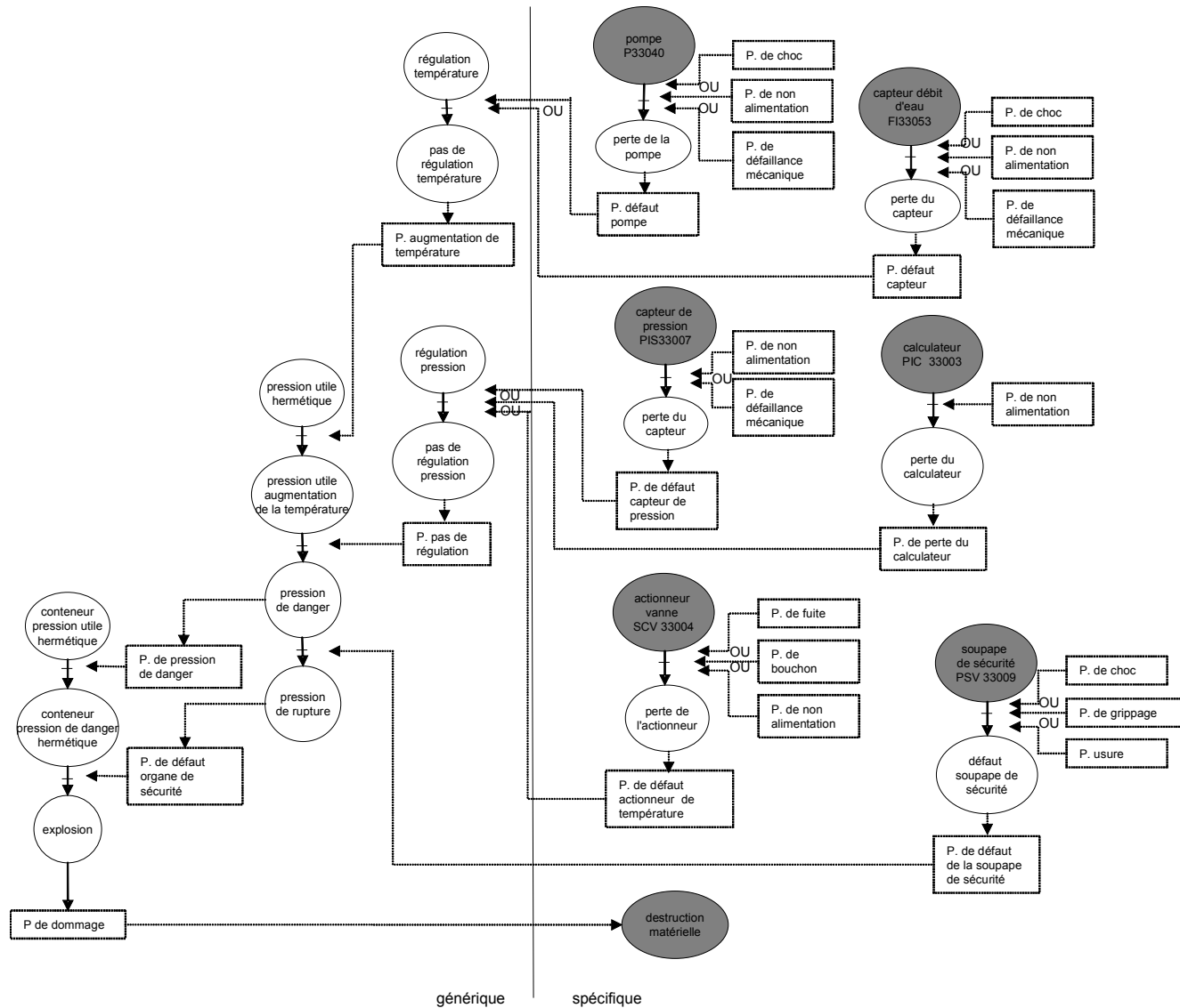
figure 3.14 Scénario de danger
