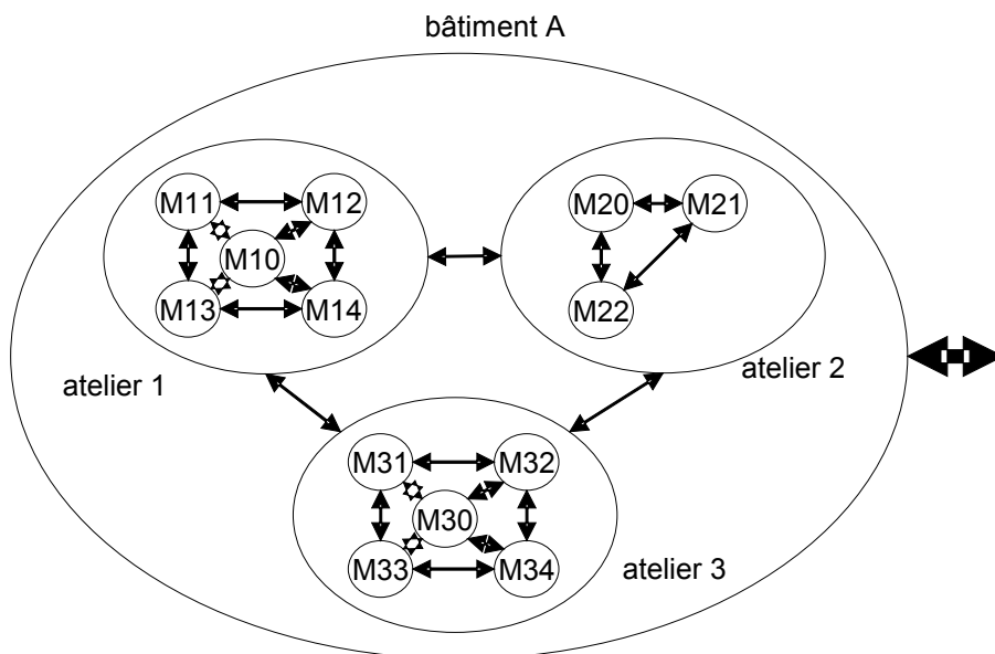
figure 1.5 Découpage systémique
