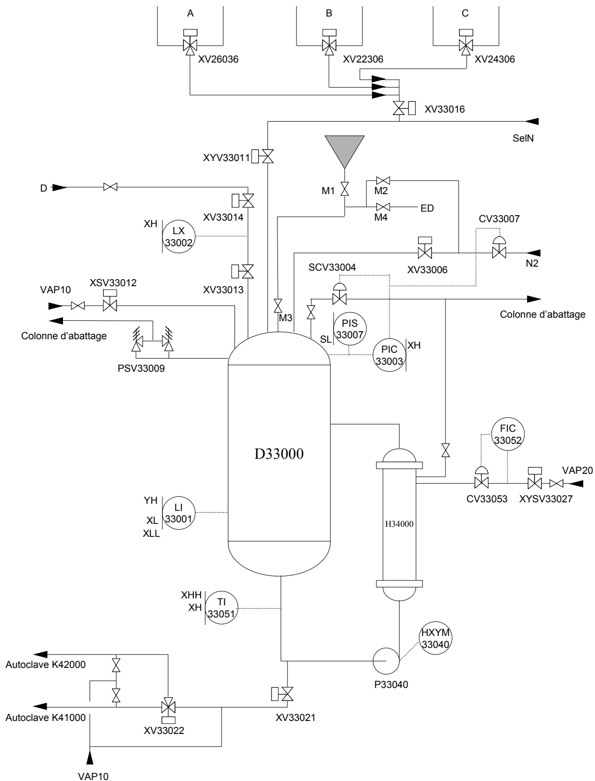
figure 3.1 Procédé industriel d'évaporation
