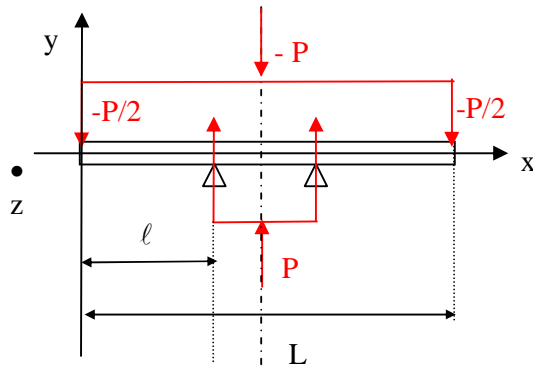
Figure III.14 : Modélisation de l'essai de flexion quatre points.
