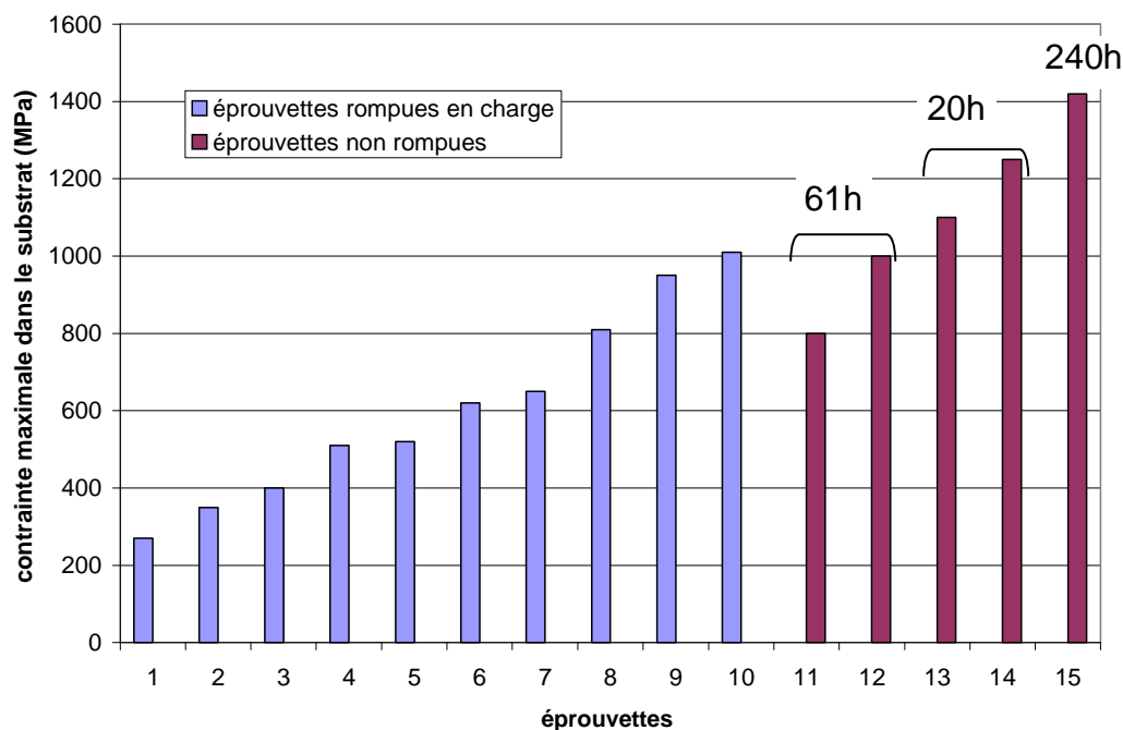
Figure IV.28 : Conditions de chargement en flexion quatre points des éprouvettes présentant un dépôt USG de 2 \mu\text{m} avec une sous-couche Al-Cu de 1,8 \mu\text{m} (contraintes maximales dans le substrat prime ) [Delette, 2005].
