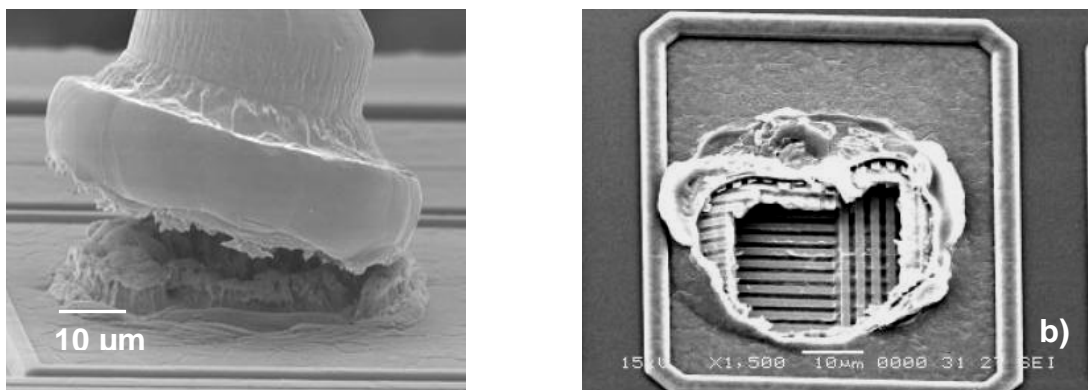
Figure I.13: Défaillances après pull test a) non adhésion du wire-bonding b) arrachement de la puce du au pull test [Crolles2 Alliance].
