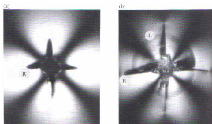
Figure III. 10 : Evolution des fissures latérales et radiales pour de la silice (a) lors de la charge apparition des fissures radiales, (b) pendant la décharge création du système de fissure radiales et latérales qui donnent naissance aux fissures de type half-penny [Lawn, 1975].
