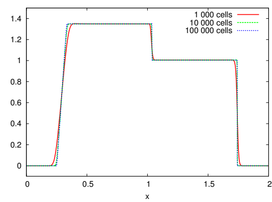
(g) Vitesse u_1 .
