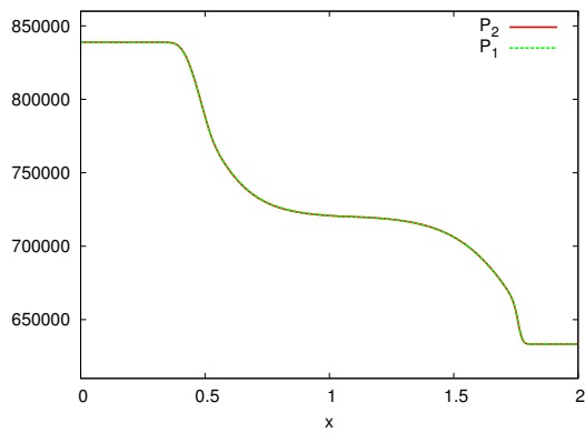
(g) Pressions en régime laminaire.
