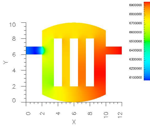
(d) Pression liquide P_2 .
