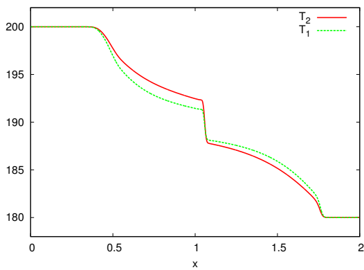
(i) Températures en régime laminaire.
