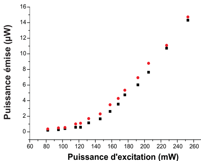
FIG. 3.14 – Puissance optique émise en \mu W en fonction de la puissance de pompe (mW). Ronds rouges : signal. Carrés noirs : complémentaire.
