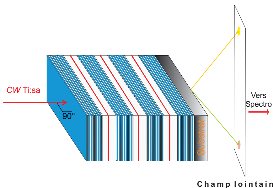
FIG. 3.6 – La microcavité est excitée à l'incidence normale par un laser Ti :Sa. On image le champ lointain de l'émission transmise sur une caméra CCD. L'excitation hors résonance permet d'obtenir la courbe de dispersion en tout point de l'échantillon.
