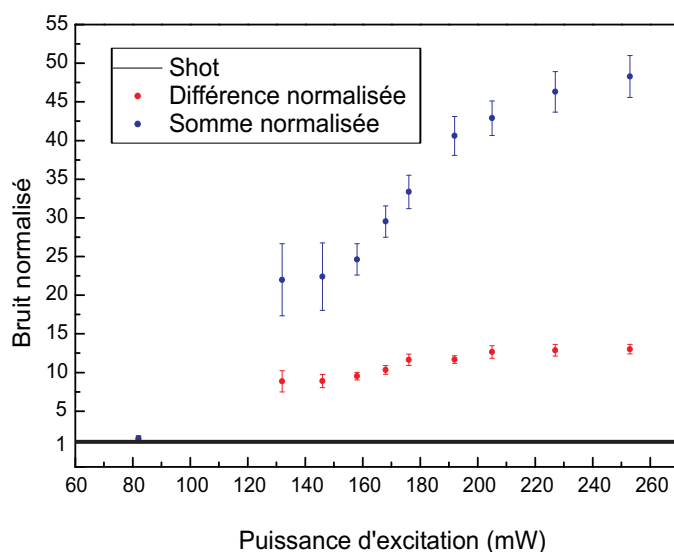
FIG. 3.15 – Bruit normalisé de la somme et de la différence des intensités du signal et du complémentaire en fonction de la puissance de pompe (mW). Ronds rouges : bruit normalisé de la différence. Ronds bleus : bruit normalisé de la somme.
