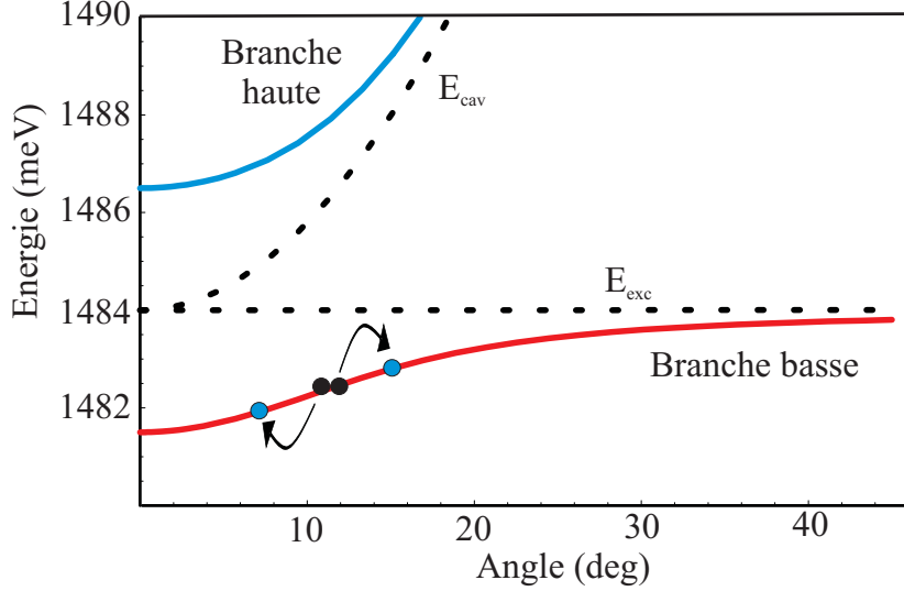
FIG. 2.2 – Représentation du terme d'interaction effective entre polaritons. Les états initiaux sont représentés par des cercles noirs, les états finaux par des cercles bleus.
