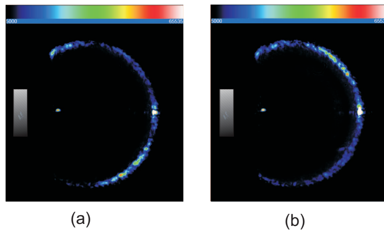
FIG. 4.12 – (a) : image en champ lointain résolue en polarisation circulaire droite ( \odot ) de la diffusion Rayleigh. (b) : image en champ lointain résolue en polarisation circulaire gauche ( \ominus ) de la diffusion Rayleigh. La pompe (à gauche) est masquée afin d'éviter la saturation de la CCD.
