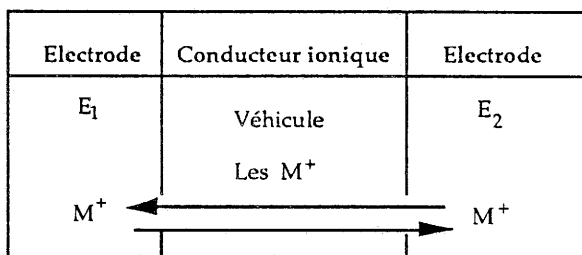
FIG. III - 1 : La chaîne électrochimique d'un dispositif électrochrome
