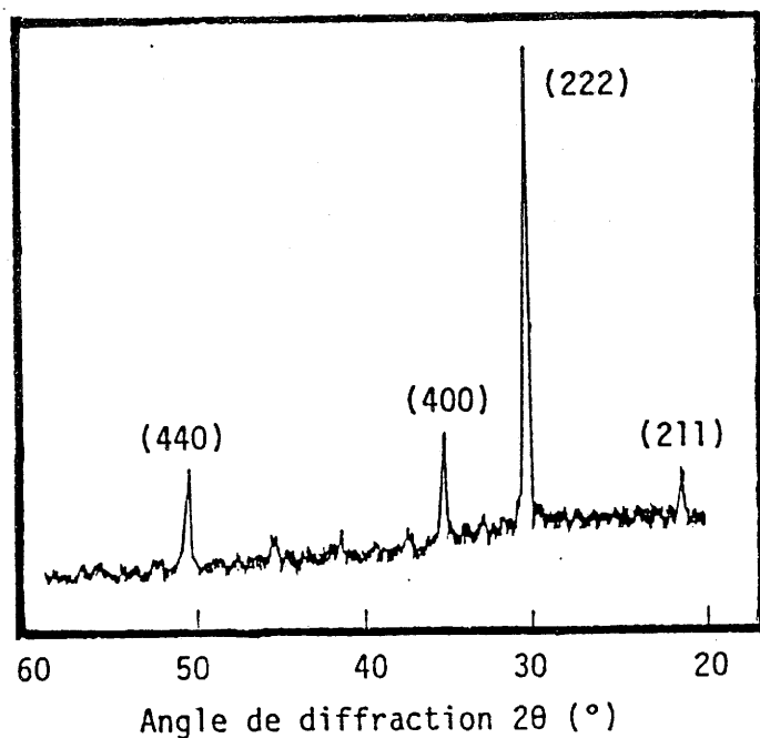
FIG. IV - 9 : Spectre de diffraction X d'un film d'ITO (60 W, T_S = 380^\circ \text{C} , plasma (Ar - O 2 5 %), pression 5 \cdot 10^{-3} mb
