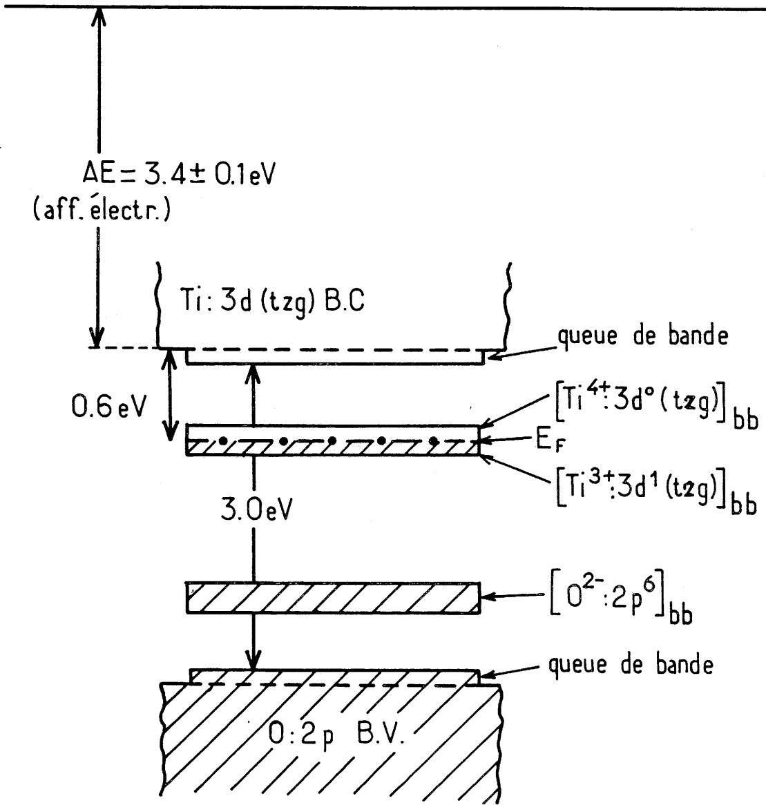
FIG. V - 4 : Mécanisme de transport dans les films amorphes de \text{SrTiO}_3 -n (8, publ. 1).
