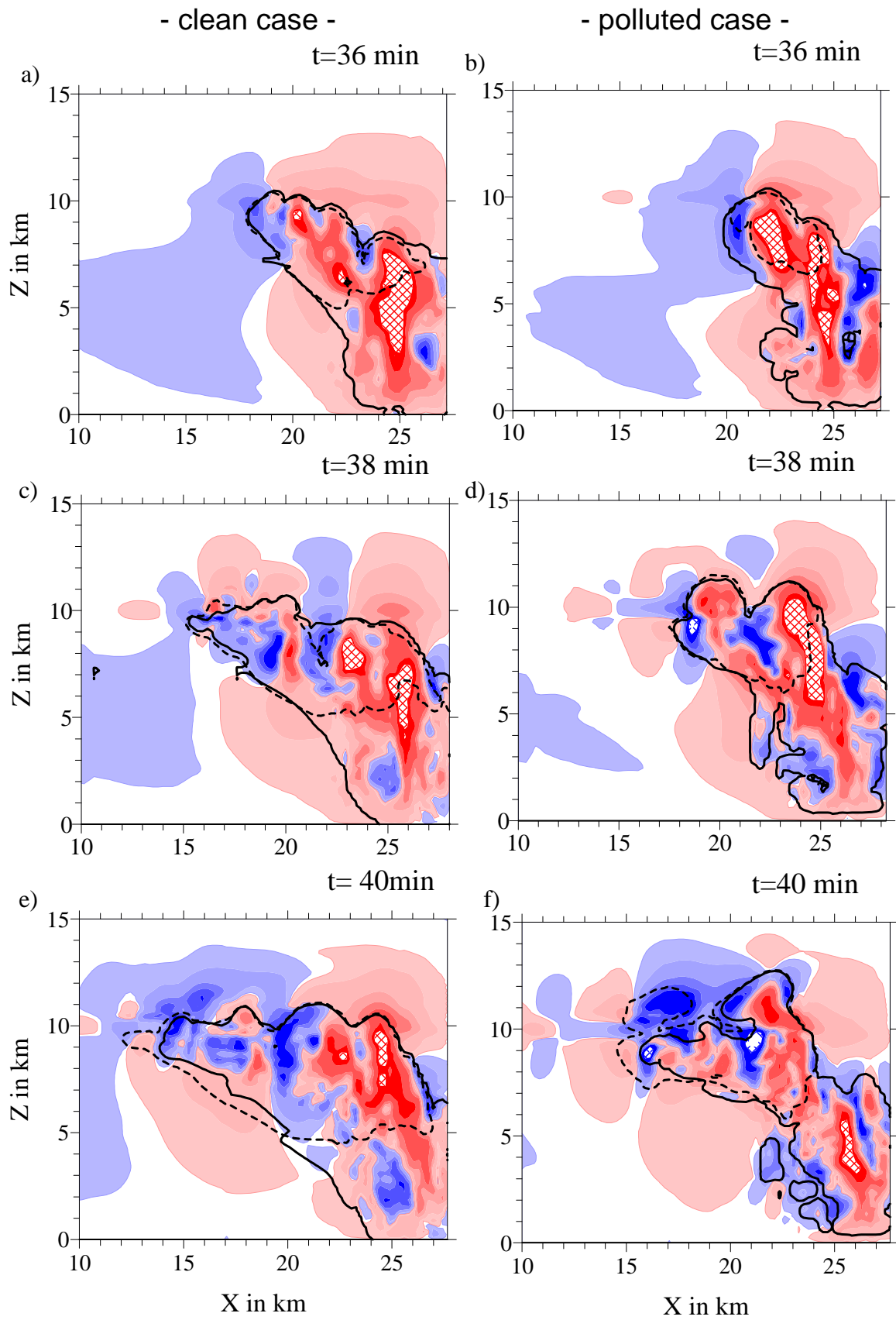
Figure 3.26 : Vent vertical ( \text{m s}^{-1} ) après 36, 38 et 40 minutes d'intégration pour une même coupe CC' à travers le domaine simulé (voir Fig. 3.29) et en fonction du spectre initial des particules d'aérosol (situation propre ou polluée). Les conventions de couleur sont les mêmes que pour les figures 3.16 ou encore 3.14.
