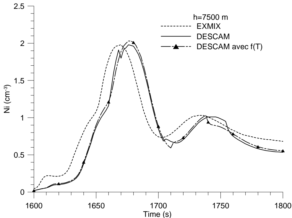
Figure 2.9 : Nombre des cristaux (cm -3 ) à 7.5 km en fonction du temps.
