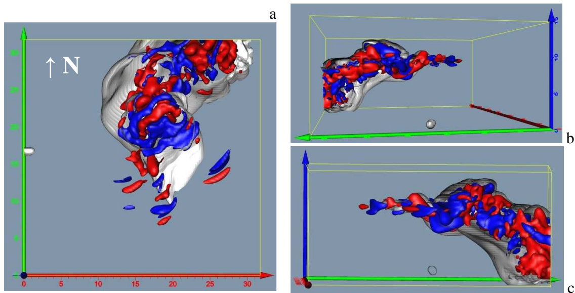
Figure 3.6 : Vent vertical simulé par DESCAM 3D après 41 minutes d'intégration. Les enveloppes bleues correspondent à -5 \text{ m s}^{-1} et les rouges à +5 \text{ m s}^{-1} . L'aspect général du nuage est rappelé à l'aide de l'enveloppe grise qui correspond, comme pour la figure 3.5 à 0.01 \text{ g m}^{-3} pour le contenu total en eau condensée (liquide + glace).
