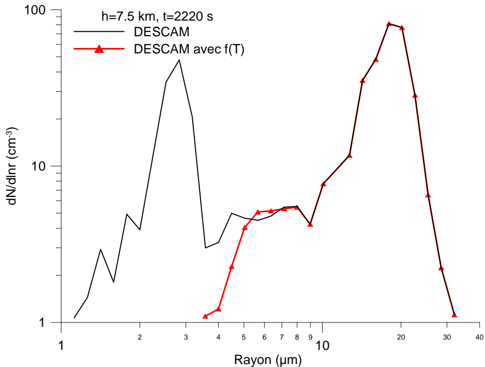
Figure 2.8 : Spectres des gouttes à 7.5 km après 37 minutes d'intégration pour le modèle DESCAM avec et sans correction de la nucléation des gouttes pour les basses températures.
