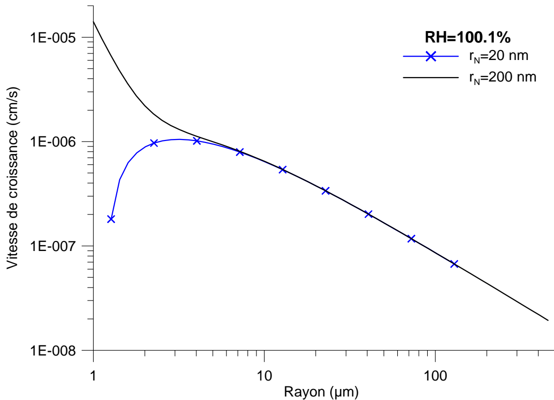
Figure 1.5 : Vitesse de croissance pour RH=100.1% en fonction du rayon humide pour deux particules d'aérosol sèches de tailles différentes (20 nm en bleu et 200 nm en noir).
