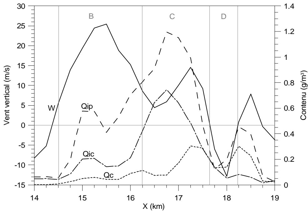
Figure 3.8 : Vitesse verticale ( w ), contenus en eau nuageuse ( Q_c ), en glace nuageuse ( Q_{ic} ) et en glace précipitante ( Q_{ip} ) simulés par DESCAM 3D à 10.25 km d'altitude et selon la direction AA' (cf. Fig. 3.7). Contrairement à la figure 3.2c, l'échelle adoptée pour les contenus est linéaire. L'évolution de la vitesse verticale sert à délimiter les différentes zones B, C et D.
