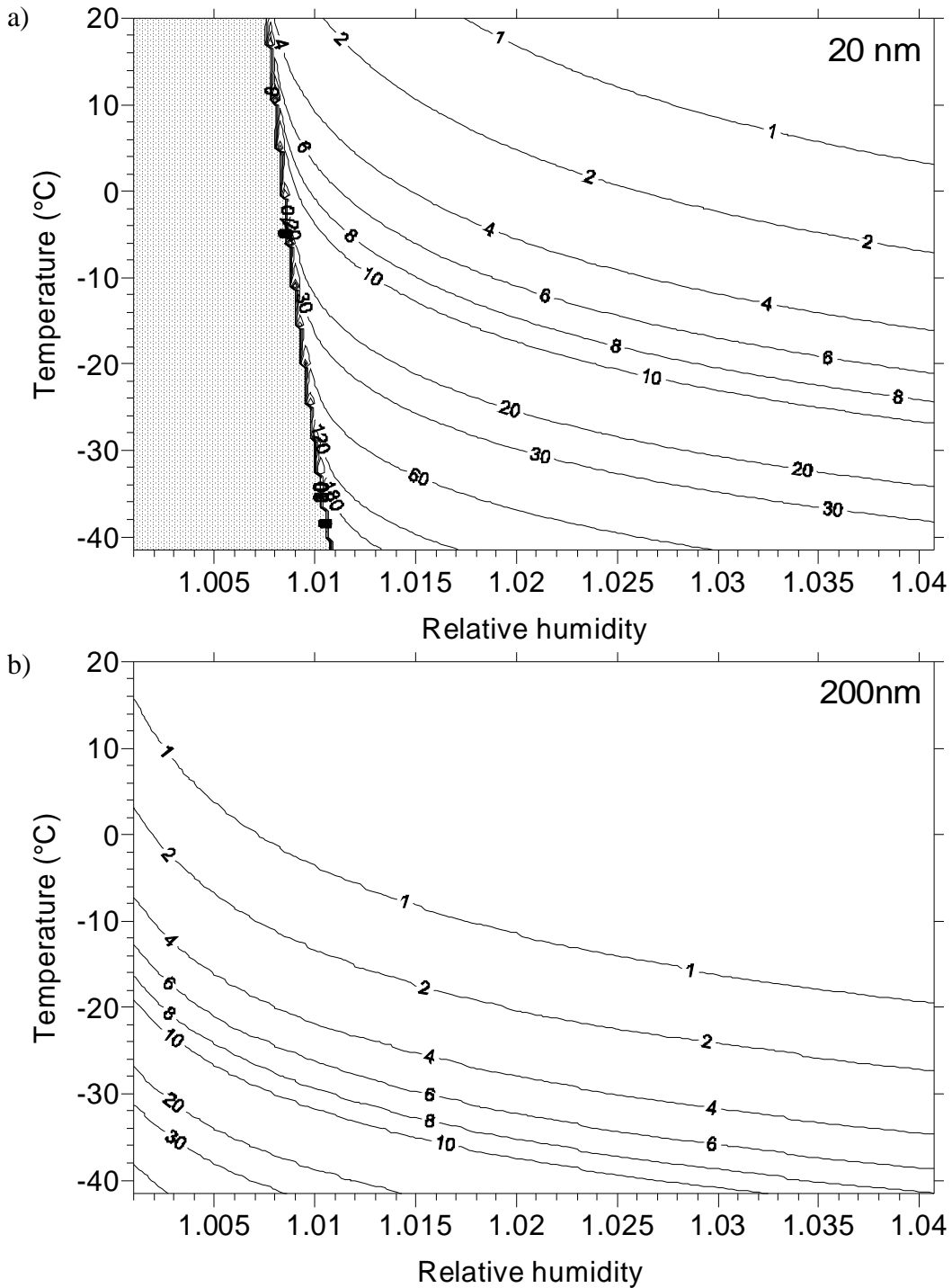
Figure 2.6 : Temps nécessaire (en s) pour que les particules d'aérosol de 20 nm (Fig. 2.6a) et de 200 nm (Fig. 2.6b) atteignent la taille 1\ \mu\text{m} par croissance par déposition de vapeur à partir de leur taille d'équilibre à 99%, en fonction de l'humidité relative et de la température. La zone en grisé sur la Fig. 2.6a correspond aux cas où l'humidité relative est trop faible pour que la particule soit activée.
