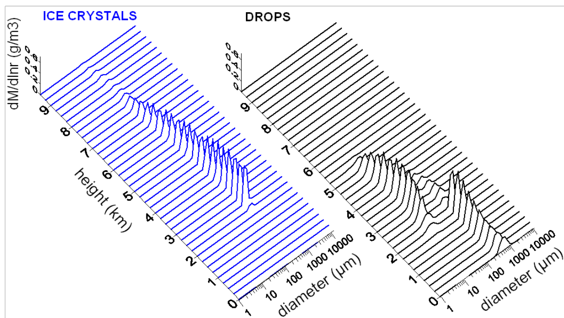
Figure 4.7 : Profil vertical des spectres en masse des cristaux (à gauche en bleu) et des gouttes (à droite en noir) pour le point (X=76 km et Y= 84 km) proche d'Alès.
