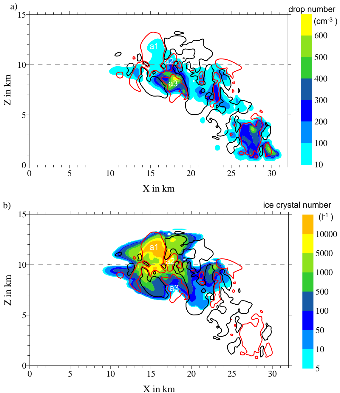
Figure 3.10 : a) Nombre des gouttes (cm -3 ) simulé par DESCAM 3D en coupe verticale selon la direction AA' (cf. Fig. 3.7). b) Idem pour le nombre des cristaux (l -1 ). Sur les deux figures, les zones d'ascendance verticales ( w > 2 \text{ m s}^{-1} ) sont signalées par les contours rouges et les zones de descendance ( w < -2 \text{ m s}^{-1} ) par les contours noirs.
