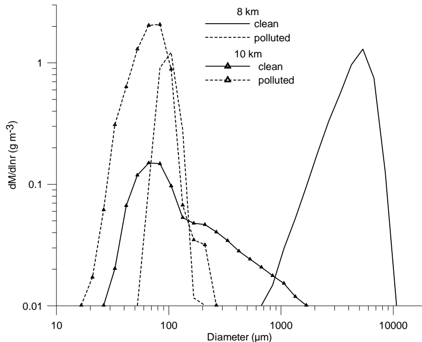
Figure 3.28 : Spectres moyens en masse des cristaux de glace à 8 et 10 km d'altitude et après 38 minutes d'intégration.
