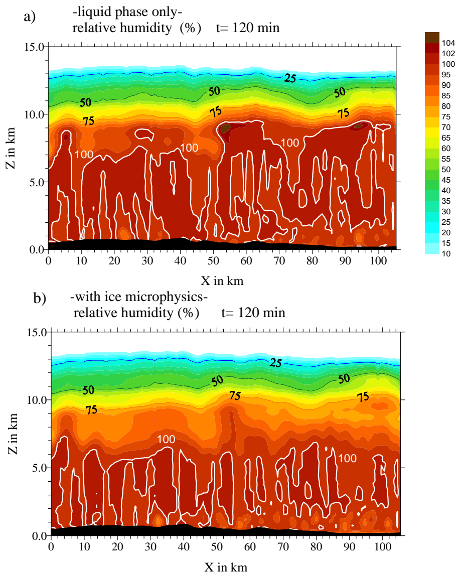
Figure 4.17 : Humidité relative (%) par rapport à l'eau le long de la coupe AA' (cf. Fig. 4.8a) pour le cas sans la microphysique froide (Fig. 4.17a) et avec la microphysique froide (Fig. 4.17b).
