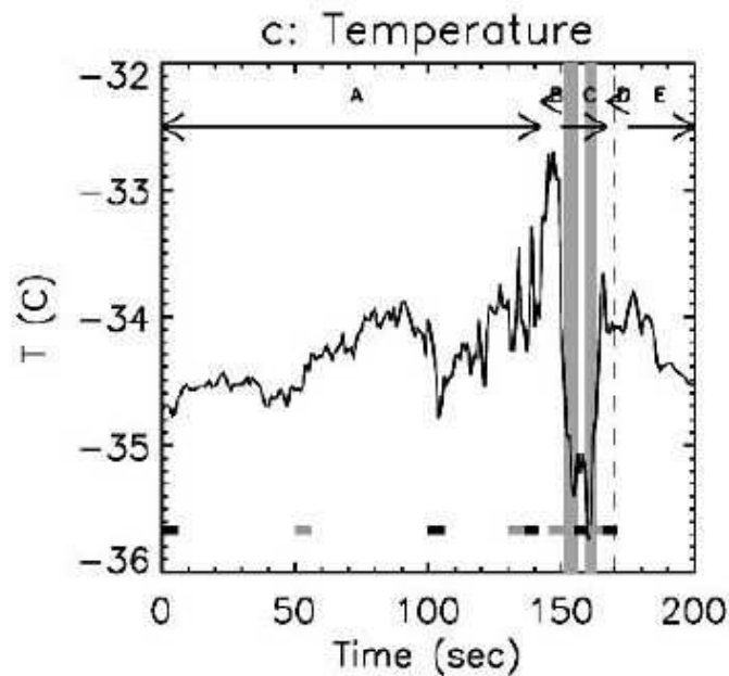
Figure 3.11 : Température (°C) mesurée lors du passage de l'avion dans le nuage.
