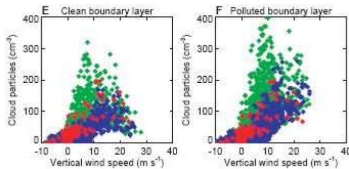
Figure 3.31 : Nombre total de particules (gouttes + cristaux) en fonction de la vitesse verticale simulé par Fridlind et al. (2004), pour les cas propre (E) et pollué (F). Comme pour la figure 3.24, les points rouges correspondent aux observations et les points verts et bleus sont les résultats du modèle respectivement à 9.9 et 10.3 km d'altitude.
