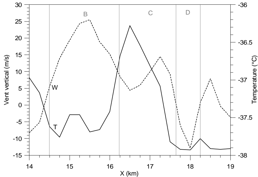
Figure 3.13 : Evolution de la vitesse verticale et de la température le long de la trajectoire AA' (cf. Fig. 3.7a et 3.12) à 10.25 km.
