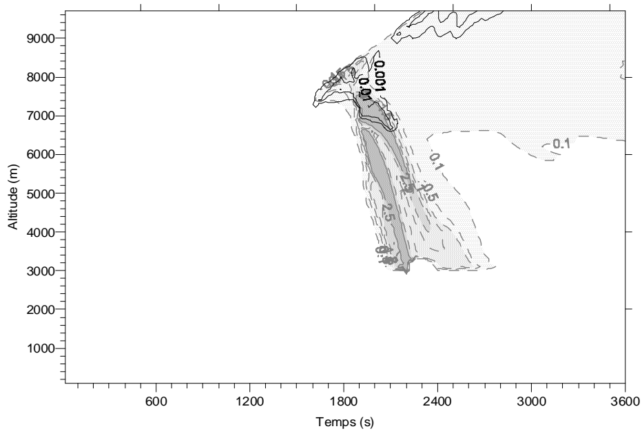
Figure D.3 : Contenu en glace nuageuse (traits noirs) et glace précipitante (zone et traits gris) en \text{g m}^{-3} pour la simulation du cas de CCOPE avec le modèle DESCAM avec trois formes possibles pour les cristaux.
