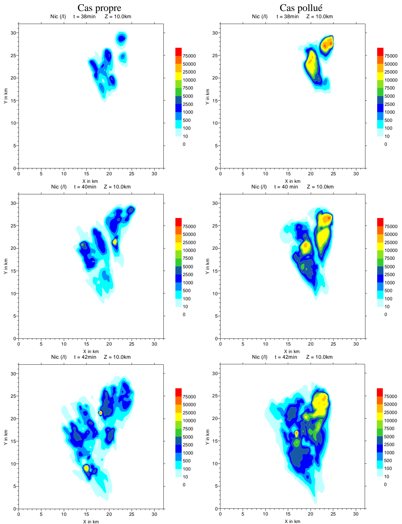
Figure 3.30 : Coupe horizontale à 10 km d'altitude du nombre des cristaux ( I^{-1} ) simulé par DESCAM 3D après 38, 40 et 42 minutes d'intégration dans les cas propre (à gauche) et pollué (à droite).
