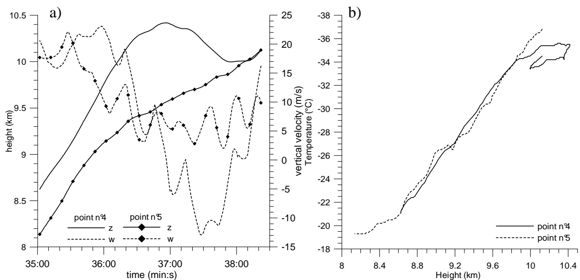
Figure 3.18 : a) Evolution de l'altitude et de la vitesse verticale le long des rétrotrajectoires calculées pour les points 4 et 5 arrivant à 10.125 km à t=38 min 20 s. b) Température en fonction de l'altitude pour les parcelles d'air 4 et 5.
