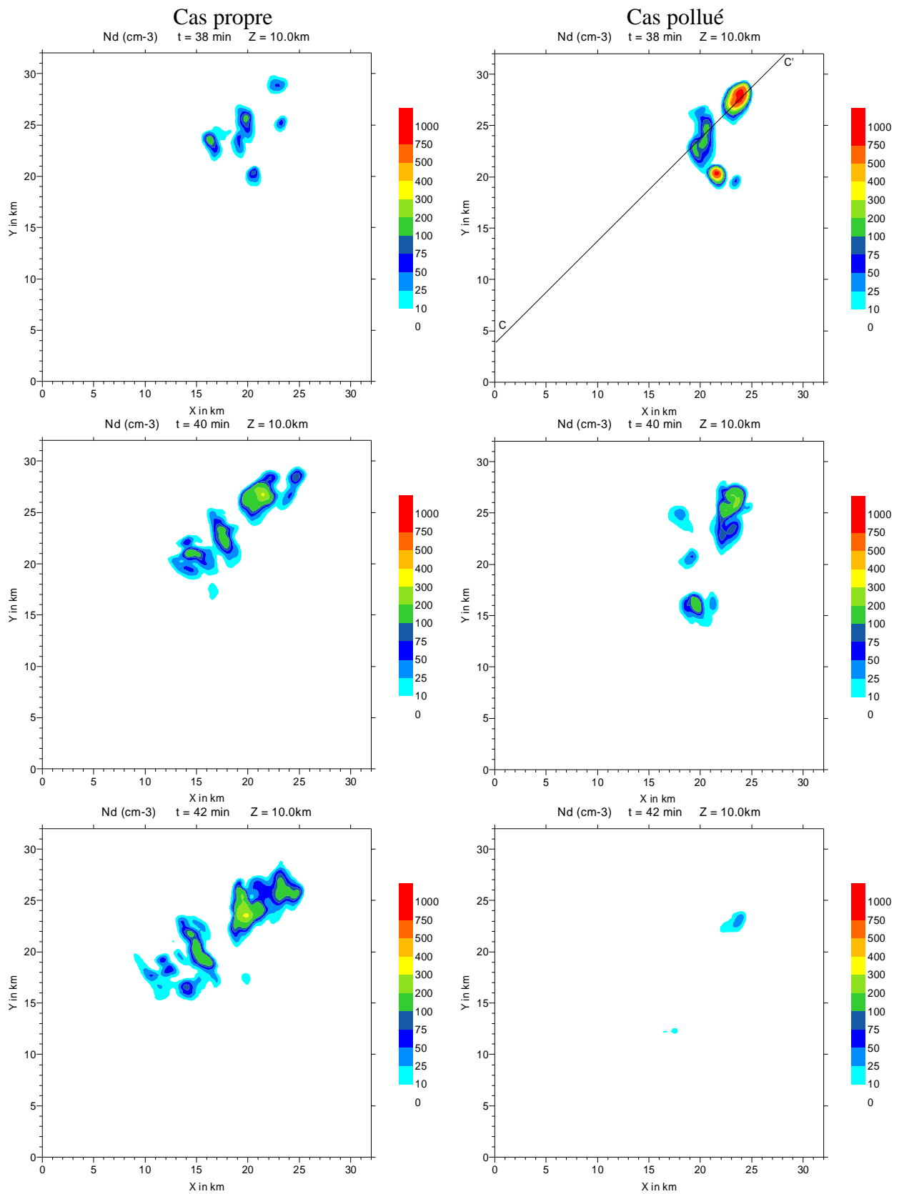
Figure 3.29 : Coupe horizontale à 10 km d'altitude du nombre des gouttes (cm -3 ) simulé par DESCAM 3D après 38, 40 et 42 minutes d'intégration dans les cas propre (à gauche) et pollué (à droite).
