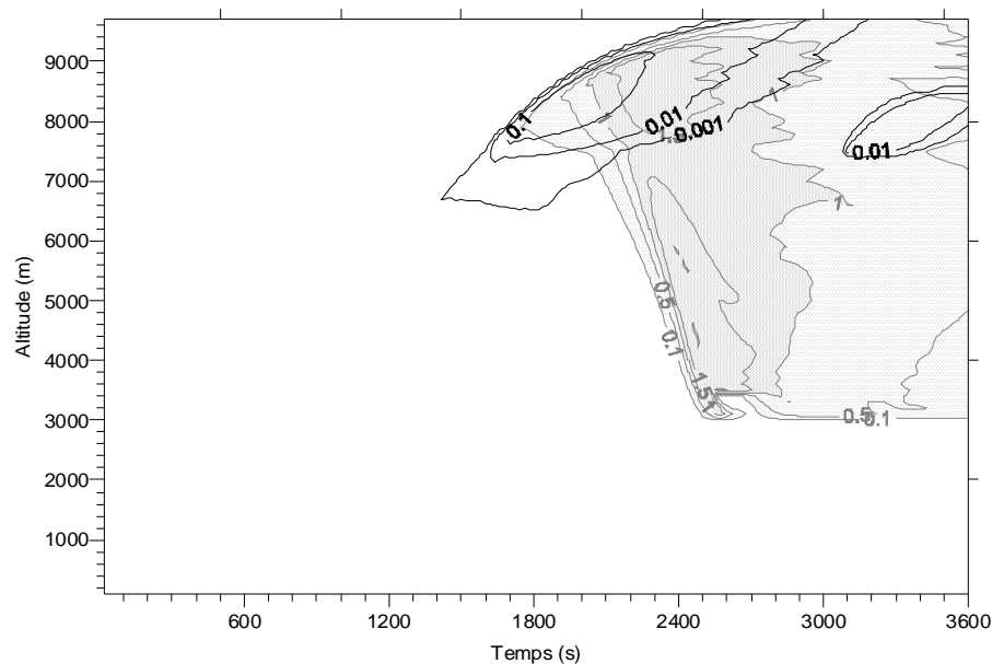
Figure 2.13 : Analogue à la figure 2.12 pour le modèle EXMIX.
