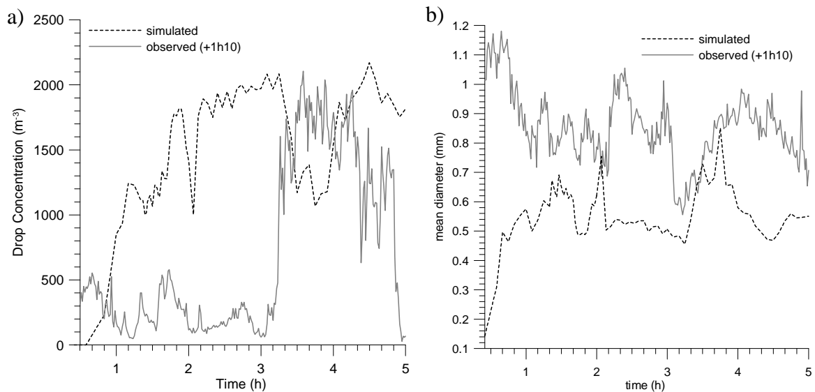
Figure 4.11 : Nombre (Fig. 4.11a) et diamètre moyen (Fig. 4.11b) des gouttes de pluie (diamètre > 64 \mu m ) à la surface calculés d'après les mesures du disdromètre (ligne continue) et simulés (ligne pointillée).
