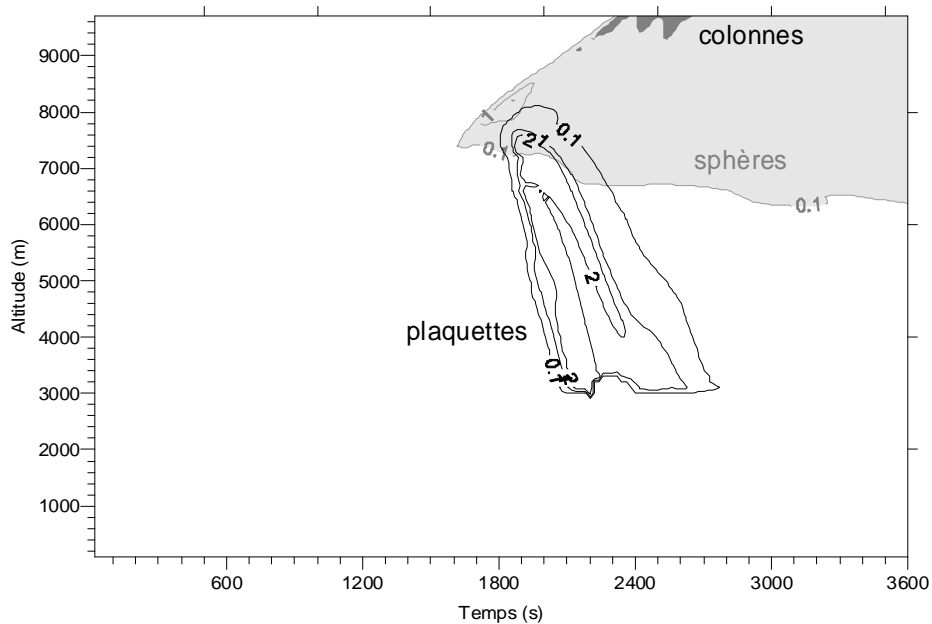
Figure D.4 : Contenus en glace en \text{g m}^{-3} pour les différentes formes considérées en fonction du temps et de l'altitude. Les couleurs noir, gris clair et gris foncé sont respectivement associées aux formes plaquettes hexagonales, sphères et colonnes. Pour les cristaux plaquettes et sphériques, le premier iso-contour correspond à 0.1 \text{ g m}^{-3} alors que pour les cristaux colonne la valeur de 0.01 \text{ g m}^{-3} a été choisie.
