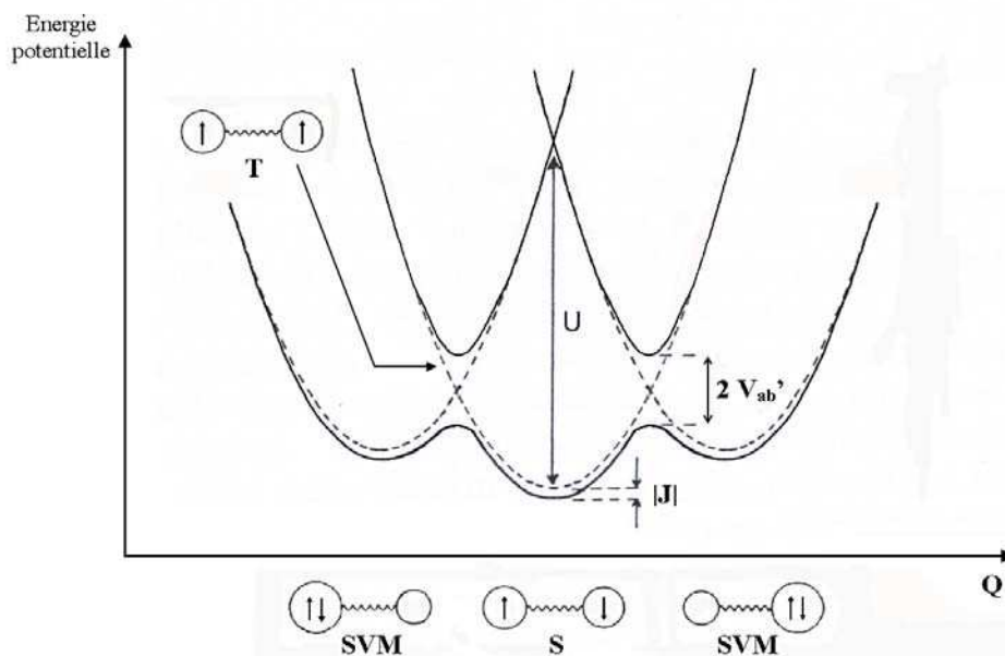
Figure I-16 : Courbes d'énergie potentielle pour un complexe dinucléaire homovalent dans le modèle du transfert de charge pour l'interaction antiferromagnétique.
