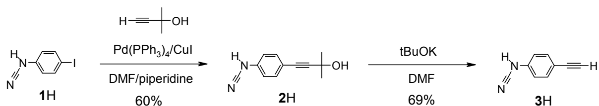
Schéma II-2 : Synthèse des ligands libres monocyanamides 2H et 3H sous leur forme protonée.
