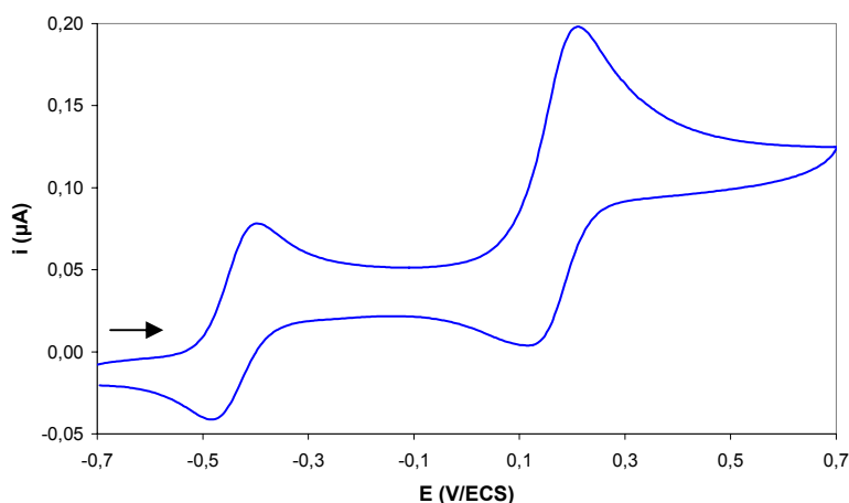
Figure II-2 : Voltamétrie cyclique de [\text{AsPh}_4]_2[\text{dicyd}] (dichlorométhane, 0.1 M TBAH, électrode de travail à disque de platine, vitesse de balayage : 0.1 \text{ V}\cdot\text{s}^{-1} , fenêtre d'étude : -0.7 \rightarrow 0.7 \rightarrow -0.7\text{V} )
