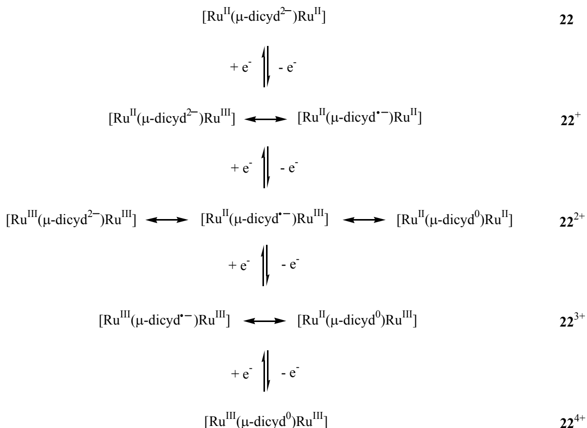
Schéma V-2 : Différentes structures électroniques envisageables selon le degré d'oxydation du complexe [\{Ru(tpy)(thd)\}_2(\mu\text{-dicyd})][PF_6] ( [22][PF_6] ).
