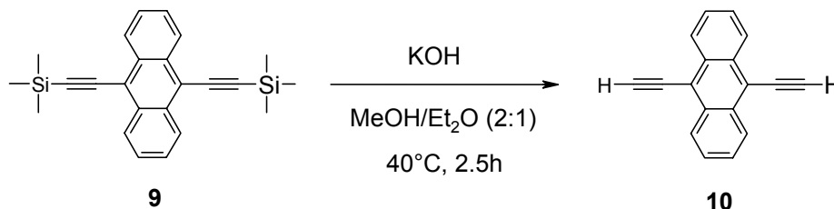
Schéma II-10 : Synthèse du 9,10-diéthynylantracène (10)
