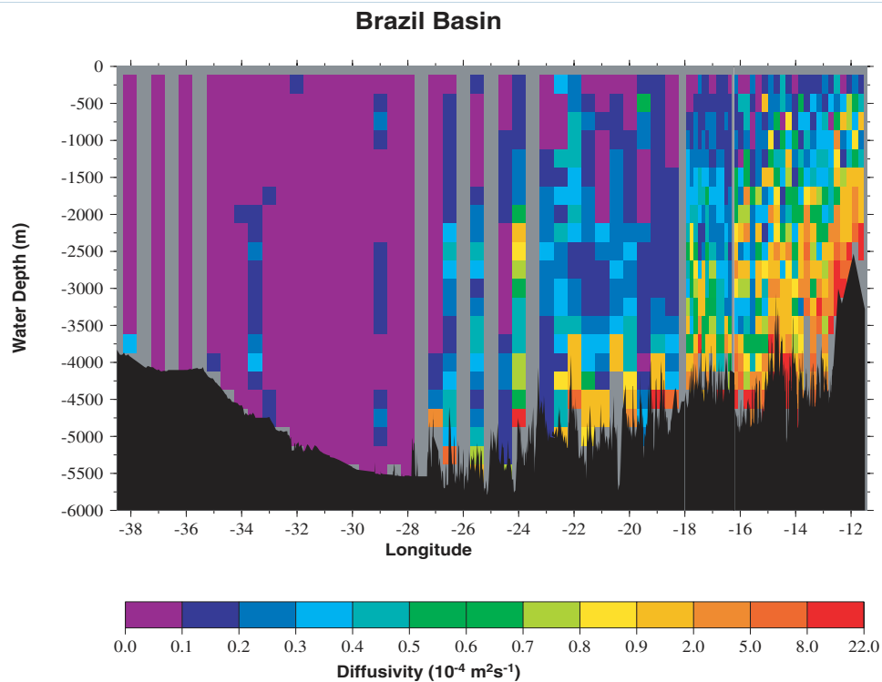
Figure 1.7 – Section zonale représentant la diffusivité verticale ( K_z ) à travers le bassin Brésilien ( m^2 \cdot s^{-1} ). Les valeurs du K_z sont faibles au dessus des topographies lisses ( i.e O(10^{-2}-10^{-1}) \text{ cm}^2 \cdot s^{-1} au dessus des plaines abyssales) et sont intensifiées par le fond au dessus des topographies plus rugueuses ( i.e O(1-10) \text{ cm}^2 \cdot s^{-1} au dessus des dorsales). D’après Mauritzen et al. (2002).
