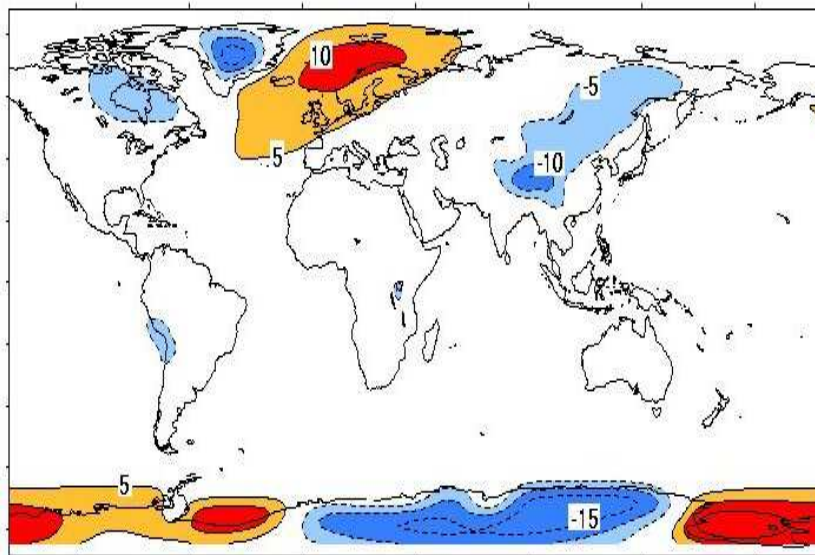
Figure 1.13 – Ecarts des températures de surface de l'air à la moyenne zonale, en moyenne annuelle. Ecarts en ^{\circ}C . Basé sur la climatologie NCAR des températures d'air de surface. D'après Rahmstorf et Ganopolski (1999).
