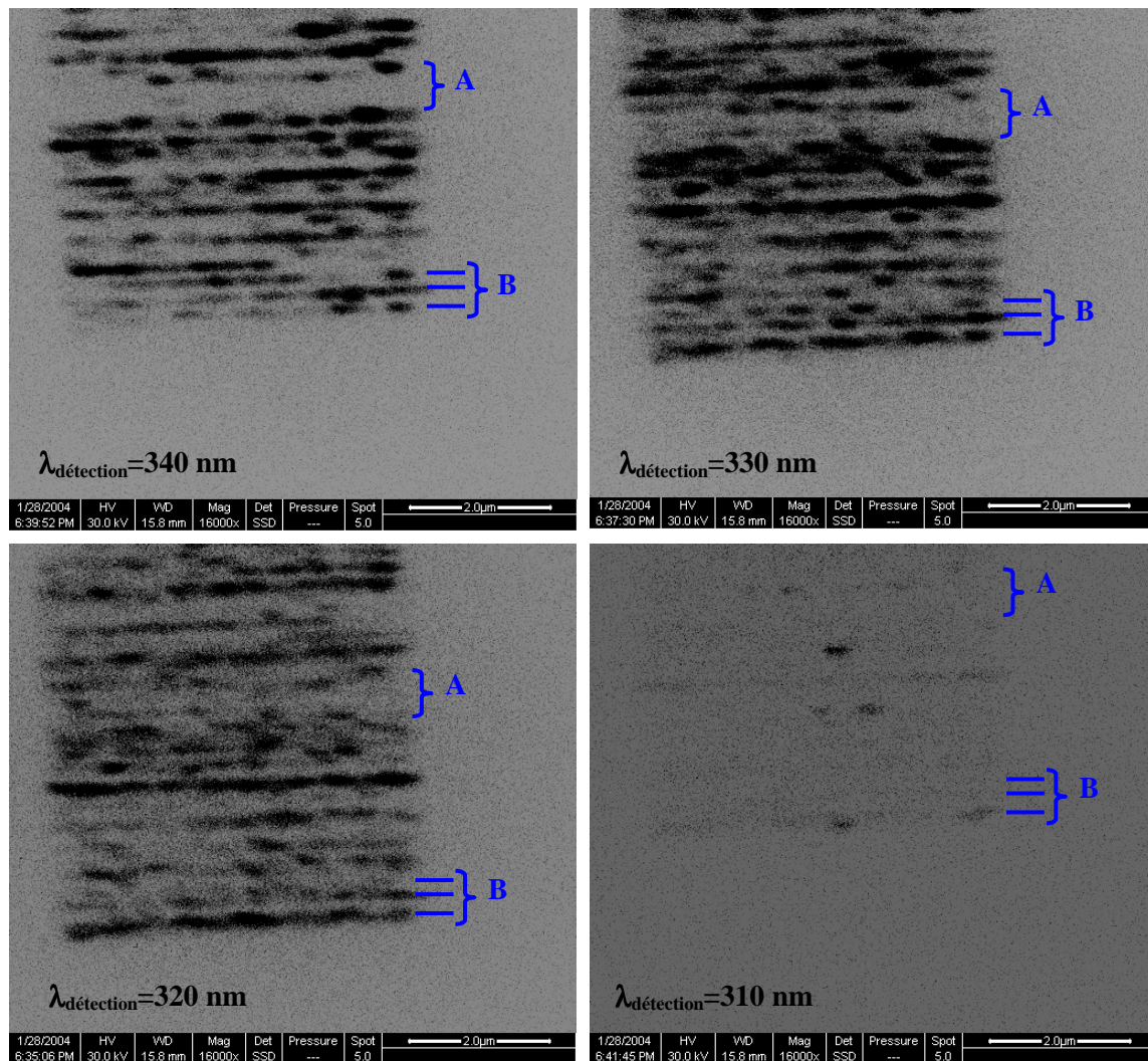
Figure 2.28 – Cartographies de CL d'une méssa de 5 \mu\text{m} de coté sur un échantillon de BQs de GaN (11-20), obtenues avec une tension d'accélération de 30 kV et filtrées à la longueur d'onde de (a) 340 nm, (b) 330 nm, (c) 320 nm, et (d) 310 nm.
