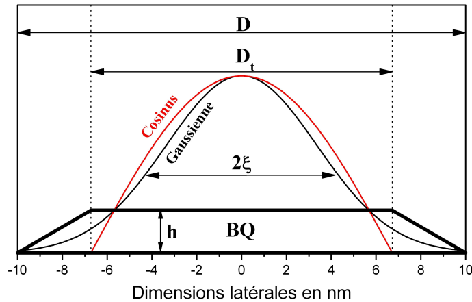
Figure 2.24 – Comparaison d'une fonction gaussienne de largeur à mi hauteur 2\xi = D/2 et de la fonction propre en cosinus du niveau fondamental d'un puits de potentiel infini de largeur D . Ce schéma permet de justifier qualitativement qu'une largeur à mi hauteur de 2\xi = D/2 est un choix raisonnable pour le paramètre de localisation de la gaussienne.
