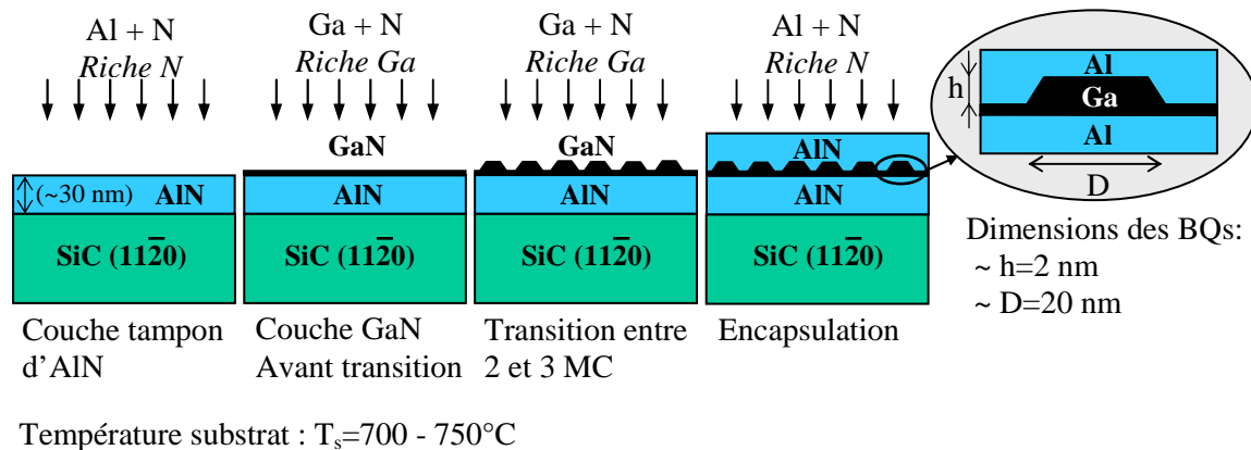
Figure 1.6 – Etapes de croissance d'un plan de BQs enterré de GaN/AlN
