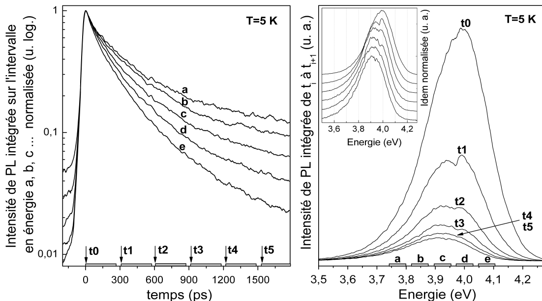
Figure 2.18 – Courbes de PL résolue en temps d'un PQ de GaN/AlN plan a, pour différentes énergies de transition, et évolution de la forme du spectre en fonction du temps. Contre toute attente, ce puits présente une luminescence lente aux temps longs, qui pourrait provenir d'un champ électrique interne lié à des ondulations de la couche épitaxiée. De plus, le déclin change avec l'énergie de transition, ce qui peut s'expliquer par des fluctuations d'épaisseur du puits.
