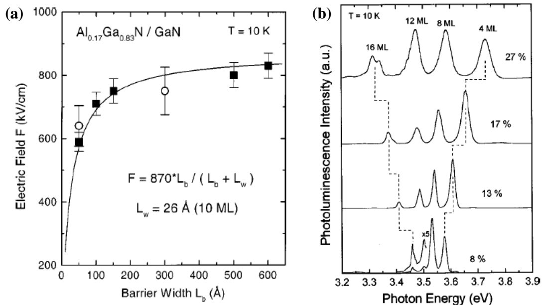
Figure 1.16 – (a) Evolution du champ électrique interne dans un super-réseau de PQs de GaN/AlGaN en fonction de l'épaisseur de barrières entre les puits. (b) Spectres de PL d'un ensemble de puits quantiques de GaN/AlGaN de 1, 2, 3 et 4 nm présentant chacun un pourcentage différent d'aluminium dans les barrières.
