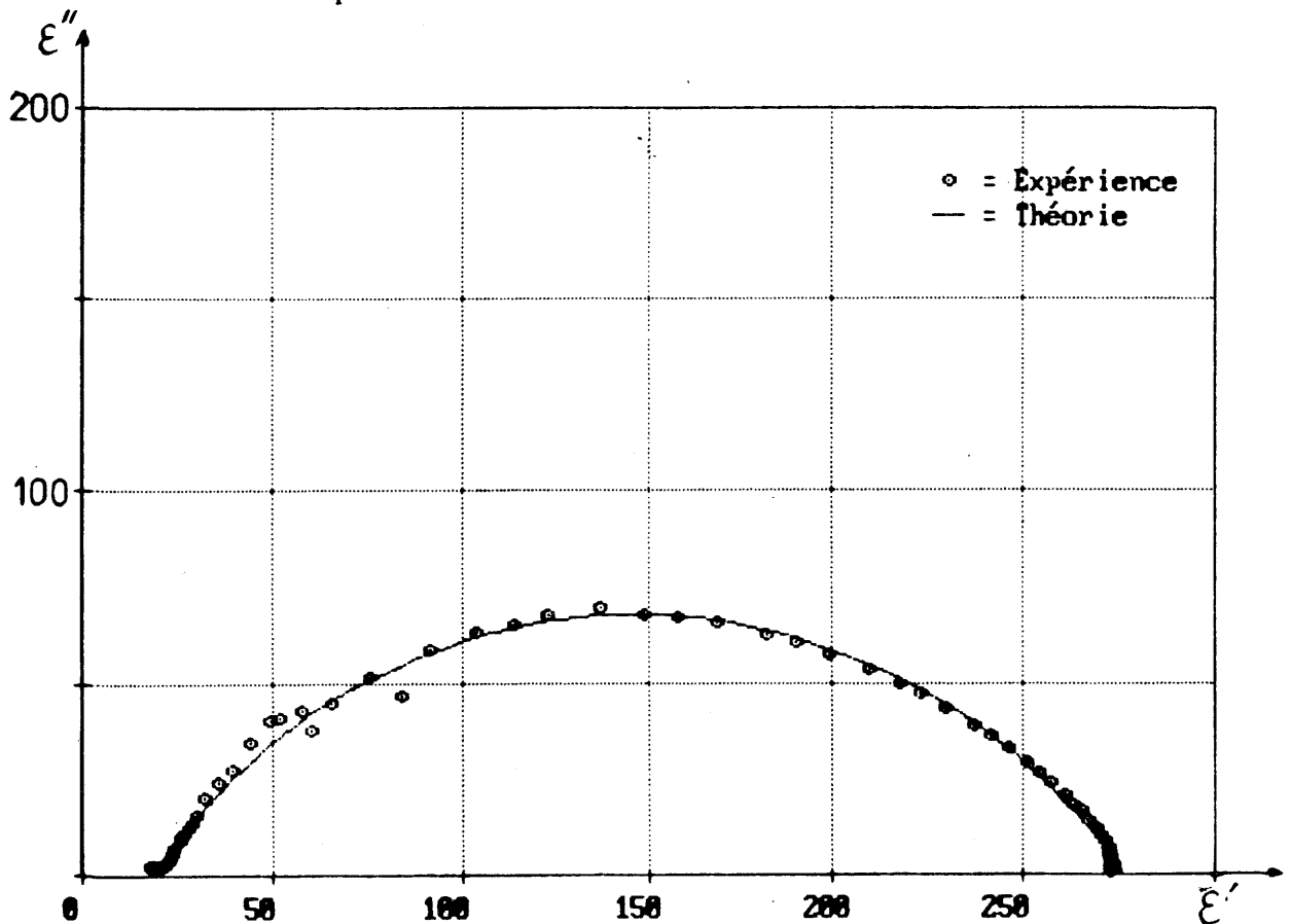
Fig.57 - Variations de \epsilon'' en fonction de \epsilon' pour un échantillon imprégné (après correction), ( I_a = 8\% , T_{\text{impr.}} = 1150^\circ\text{C} , \theta_{\text{impr.}} = 2\text{h} ).
