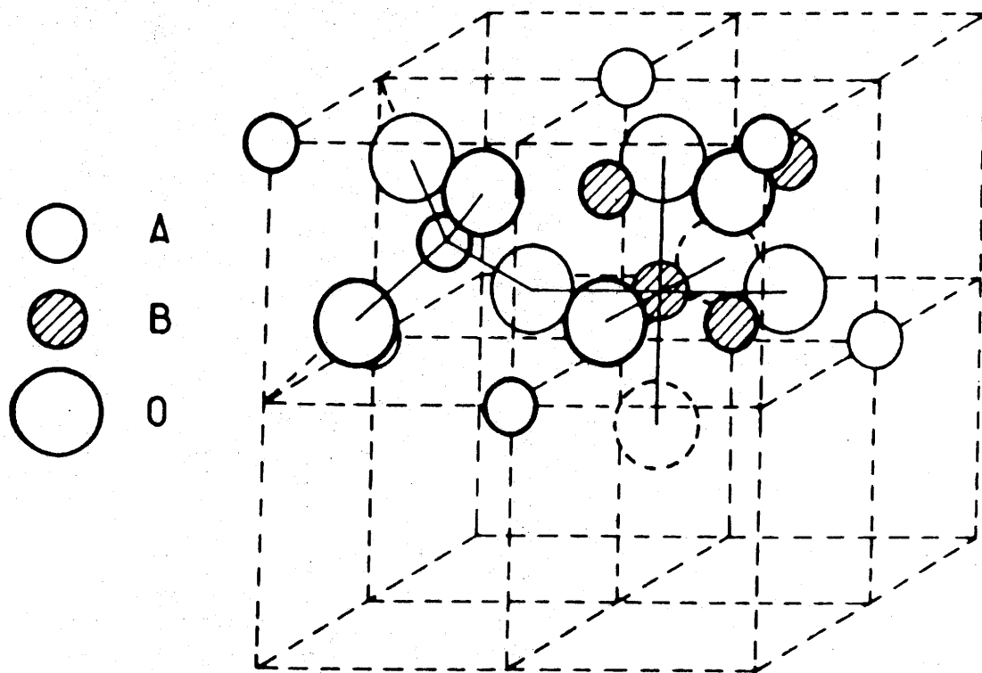
Fig.2 - Les deux octants de la maille spinelle.
