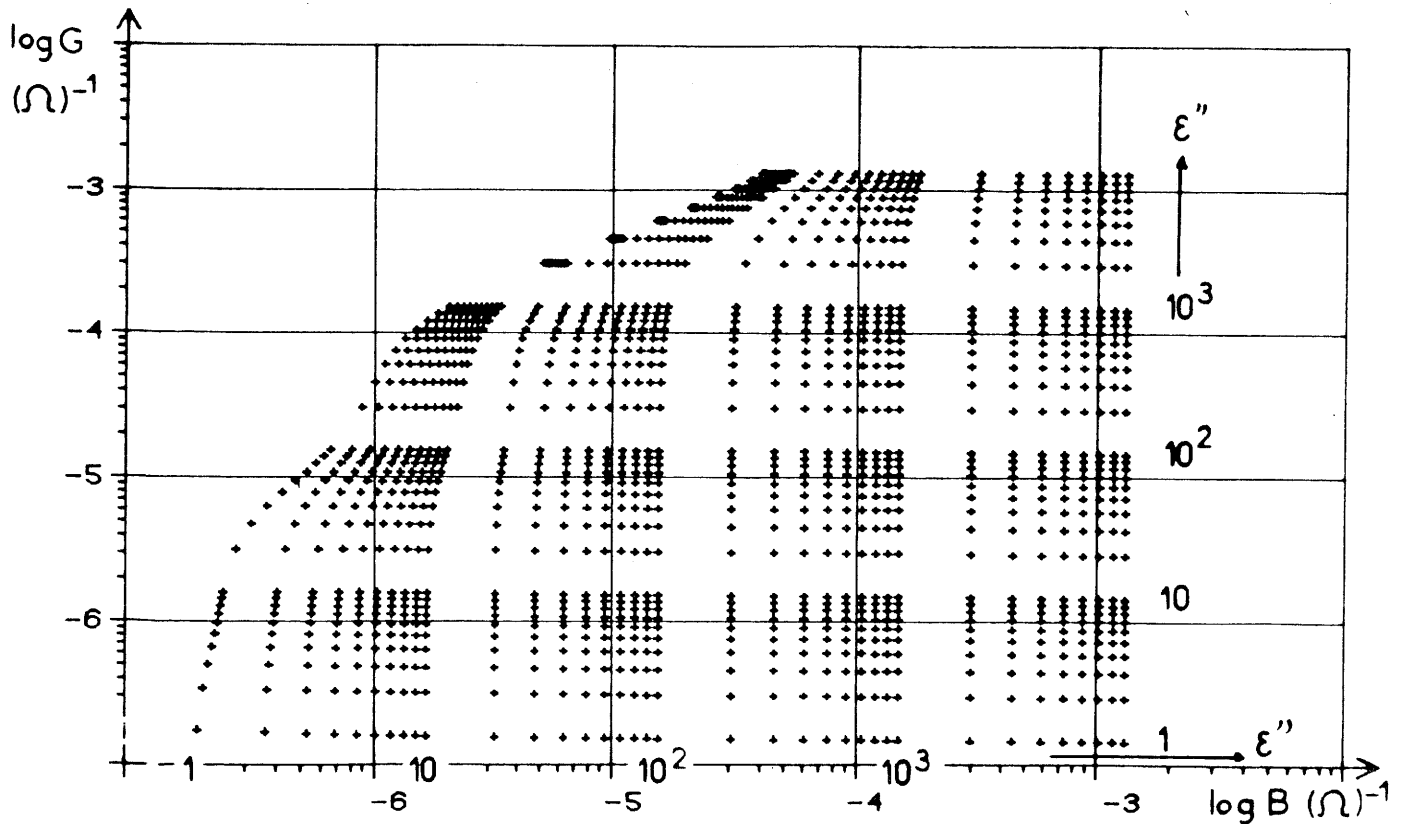
Fig. 98 - Abaque \epsilon' , \epsilon''=f(G,B) pour f=300 kHz, e=1,5 mm, NM=24 .
