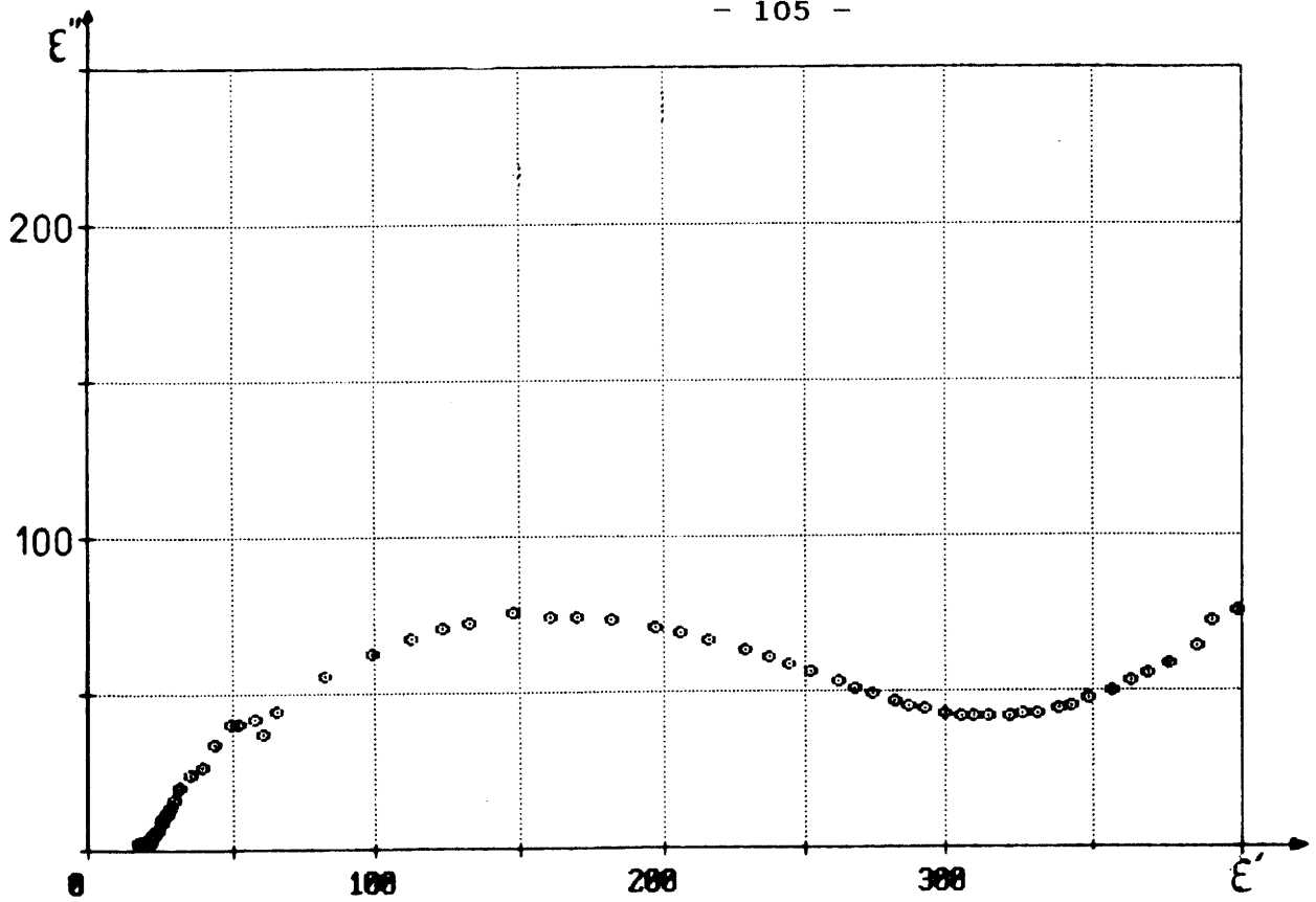
Fig.56 - Variations de \epsilon'' en fonction de \epsilon' pour un échantillon imprégné (sans correction), ( I_a = 8\% , T_{\text{impr.}} = 1150^\circ\text{C} , \theta_{\text{impr.}} = 2\text{h} ).
