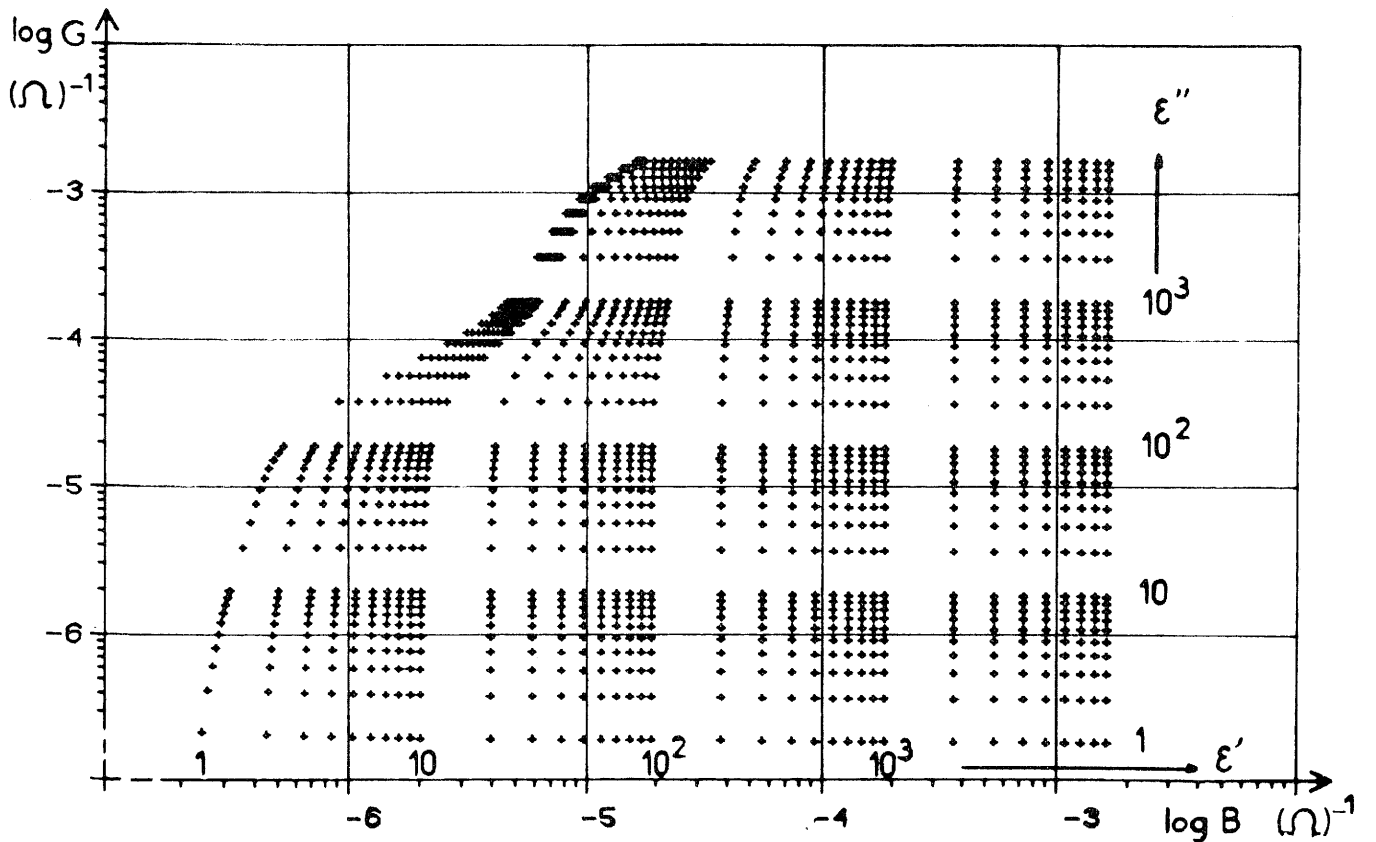
Fig. 92 - Abaque ε', ε''=f(G,B) pour f=300 kHz, e=1 mm, NM=30.
