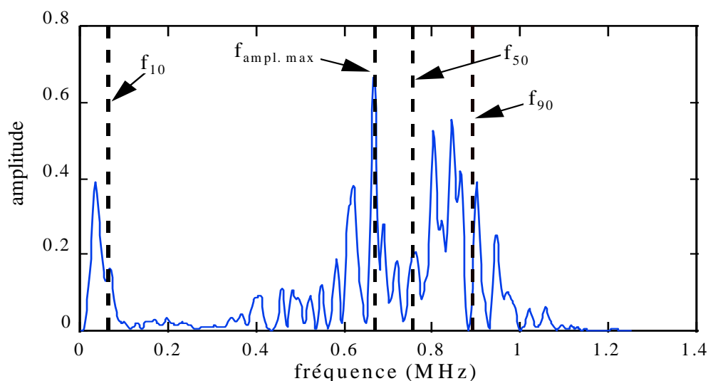
Figure 136 : Caractérisation du spectre déconvolué. f_{10} , f_{50} et f_{90} , : fréquences à 10%, 50% et 90% de l'énergie spectrale cumulée; f_{ampl\ max} : fréquence d'amplitude maximale.
