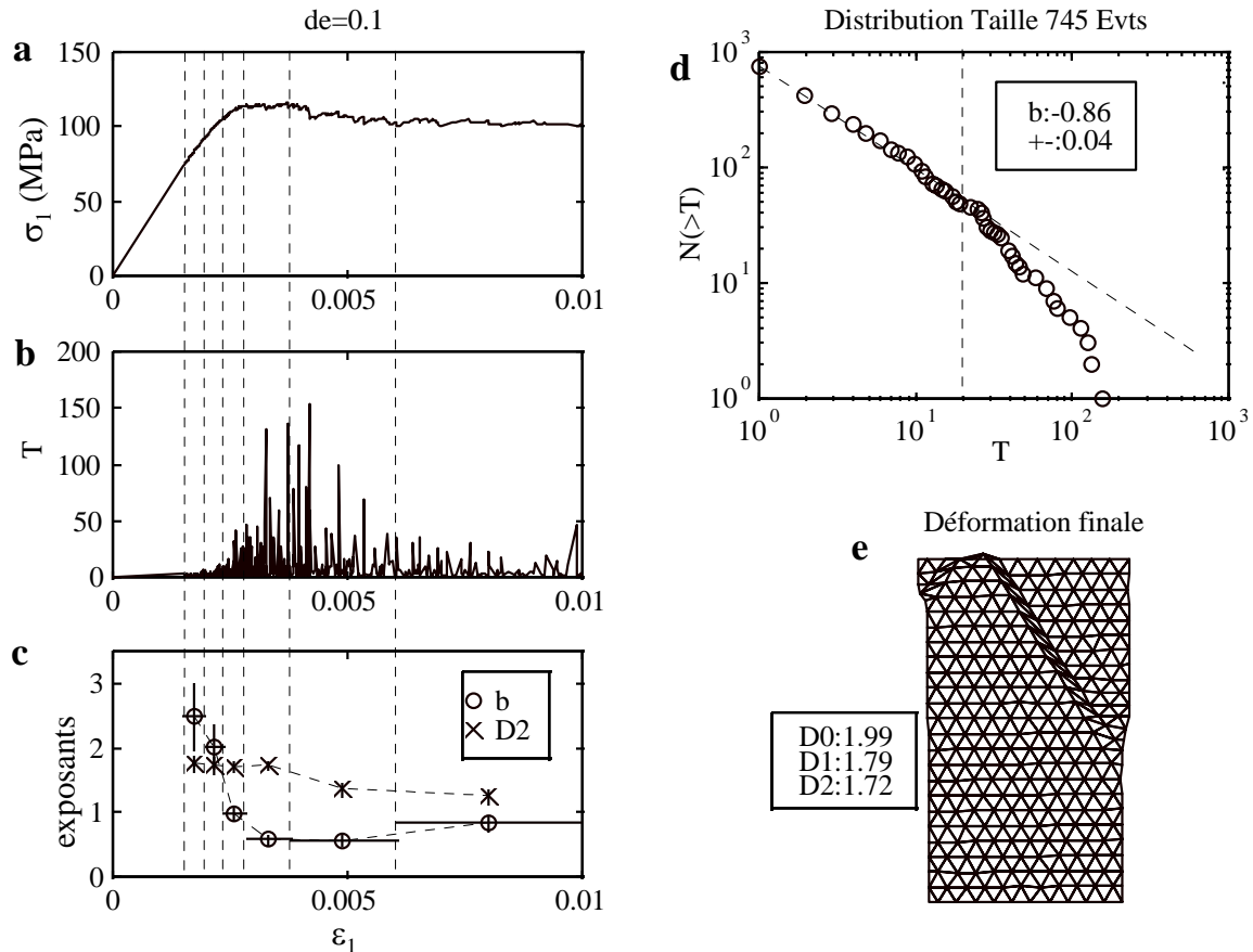
Figure 86: Résultats globaux de la simulation avec de = 0.1 , E = 50 GPa, \nu=0.25 , \tan(\phi)=0.5 et C=25-50 MPa. a) Courbe contrainte-déformation macroscopique, \sigma_1(\varepsilon_1) . b) Taille d'avalanche en fonction de \varepsilon_1 , T(\varepsilon_1) . c) exposants b ( T < 12 ) et D_2 pour des fenêtres successives contenant le même nombre d'avalanches (120). d) Distribution des tailles d'avalanches pour l'ensemble de la simulation. e) Déformation finale du modèle (amplifiée par 10).
