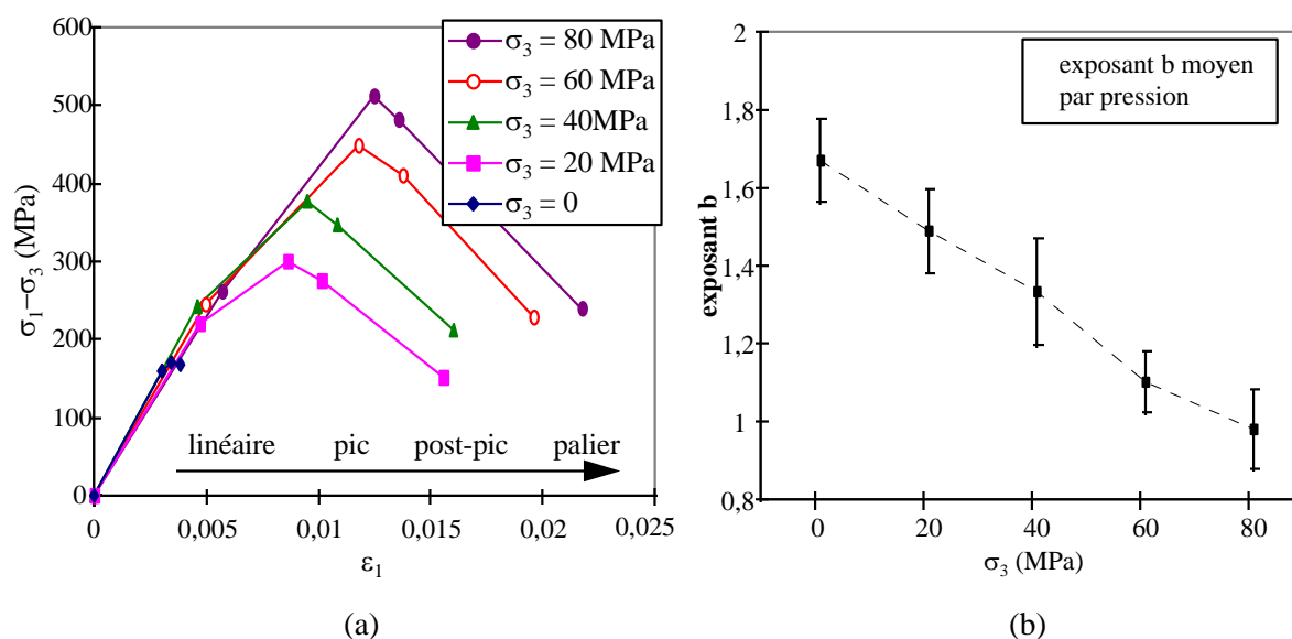
Figure 127 : Apparition de la ductilité et diminution de l'exposant b observés expérimentalement lors de l'augmentation de la pression de confinement. a) \sigma_1 - \sigma_3 moyen en fonction de \epsilon_1 moyen pour différentes valeurs de pression de confinement \sigma_3 . b) Exposant b moyen pour chaque valeur de pression de confinement, \sigma_3 . Les barres verticales indiquent l'écart type.
