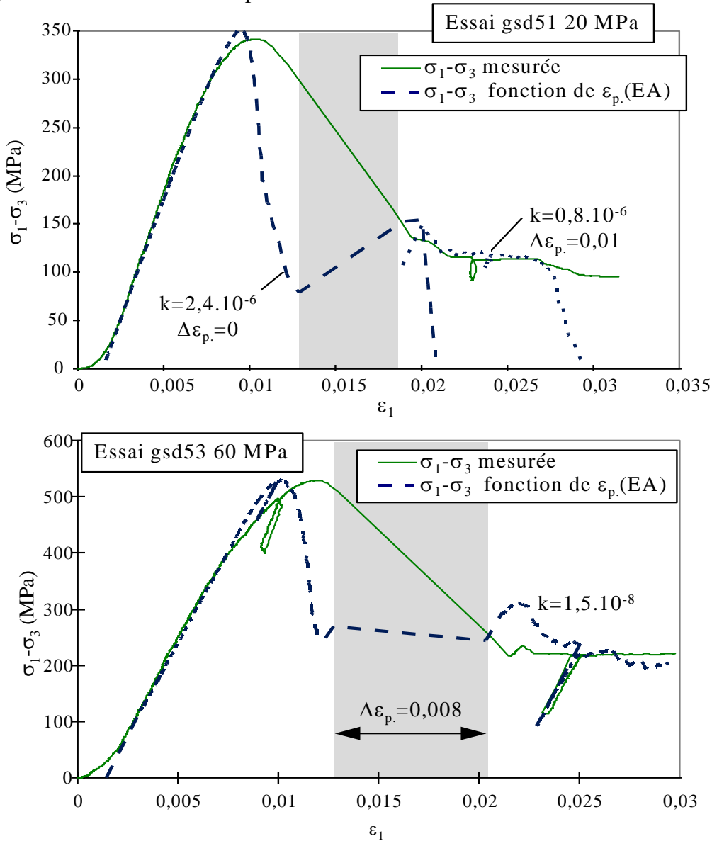
Figure 40 : Reconstruction de la courbe contrainte déformation à partir de la déformation permanente estimée par l'EA, pour deux essais de compression triaxiale. \Delta \epsilon_p est la déformation permanente due à la macrorupture.
