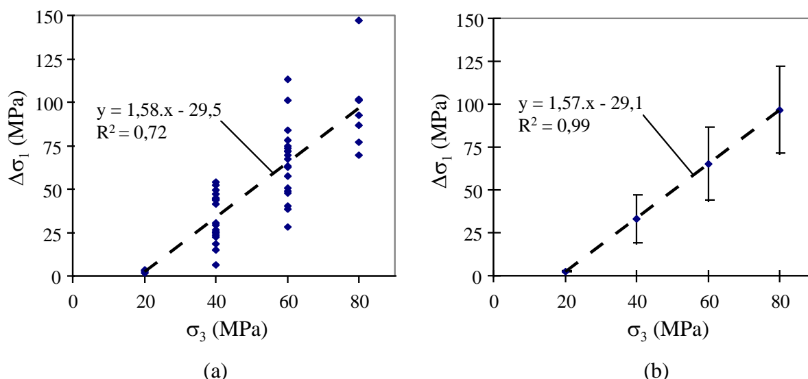
Figure 65 : Chute de la contrainte axiale au cours du glissement instable, \Delta\sigma_1 en fonction de la pression de confinement. a) ensemble des valeurs calculées. b) valeurs moyennes par pression de confinement. Les barres verticales indiquent l'écart type.
