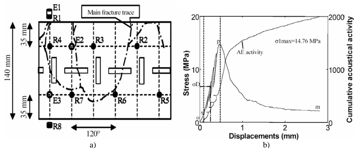
Figure 3 : a) Instrumentation acoustique et de déformation d'une éprouvette cylindrique de minerai de fer et trace de la surface de rupture (vue dépliée). b) Comportement mécanique et activité acoustique du même échantillon soumis à une compression uniaxiale.
