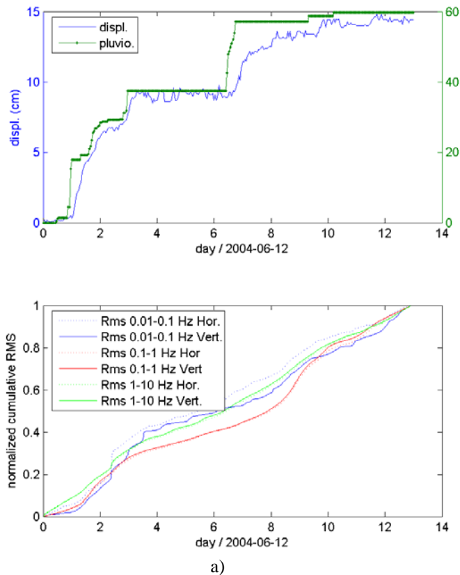
Figure 7 : a) Haut : déplacement et pluviométrie enregistrés sur le site de Super Sauze. Bas : RMS cumulée dans trois bandes de fréquence différentes. b) Haut : Stéphane Gaffet en phase d'installation de la station sismologique sur l'éperon rocheux autour duquel se déforme le glissement coulée. Bas : Stries de frottement entre la coulée et l'éperon.
