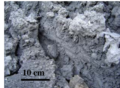
Figure 7 : a) Haut : déplacement et pluviométrie enregistrés sur le site de Super Sauze. Bas : RMS cumulée dans trois bandes de fréquence différentes. b) Haut : Stéphane Gaffet en phase d'installation de la station sismologique sur l'éperon rocheux autour duquel se déforme le glissement coulée. Bas : Stries de frottement entre la coulée et l'éperon.
