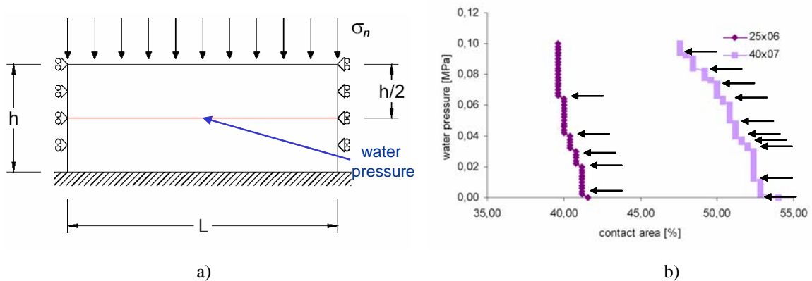
Figure 23 : a) Modélisation numérique par la méthode des éléments frontières de l'ouverture d'une fracture rugueuse sous l'effet d'une augmentation de pression de fluide. b) Proportion des aires de contact de la fracture en fonction de la pression de fluide, pour deux profils de rugosité différents. Les flèches horizontales indiquent les phases d'instabilité de l'ouverture, susceptibles d'induire de la sismicité.
