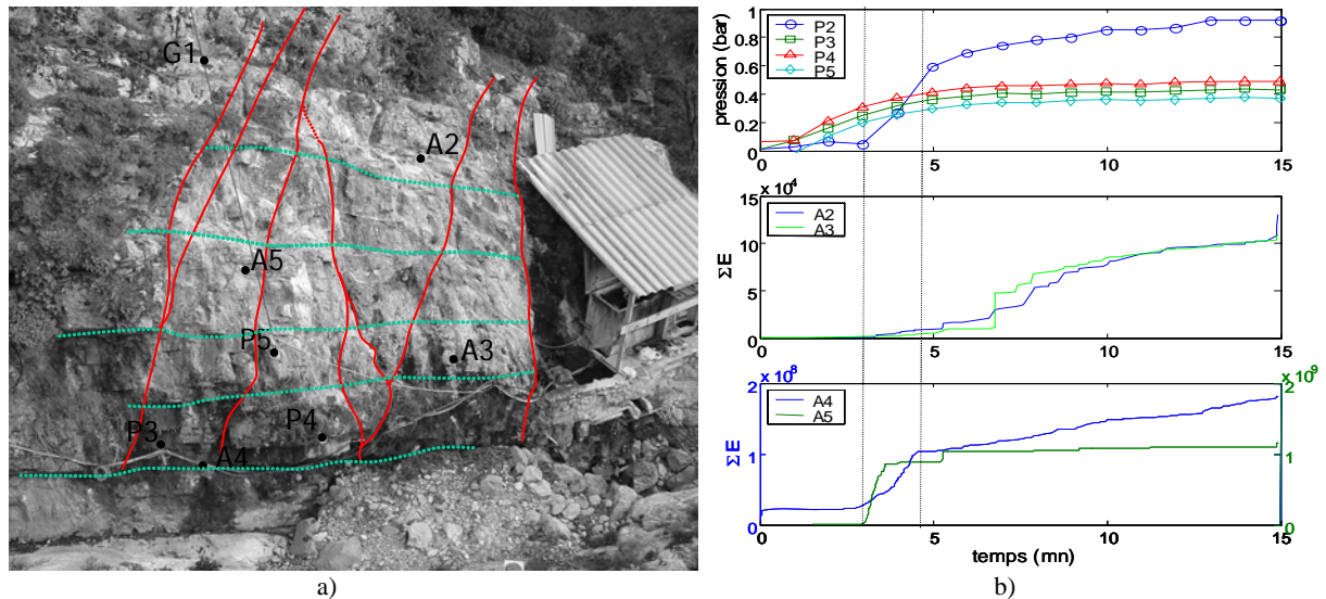
Figure 22 : a) Configuration du réseau sismique sur le site de Coaraze. G1 est un géophone tridirectionnel. A2, A3, A4, A5 sont des accéléromètres unidirectionnels. b) Pression hydraulique et énergie sismique cumulée sur les différents capteurs. P2 mesure la pression dans une fissure peu perméable, P3, P4 et P5 mesurent la pression dans des fractures fortement perméables (drains). Les accéléromètres A2 et A3 sont placés à distance des drains (1-1.5 m), A4 et A5 sont placés à proximité des drains (0.5 m).
